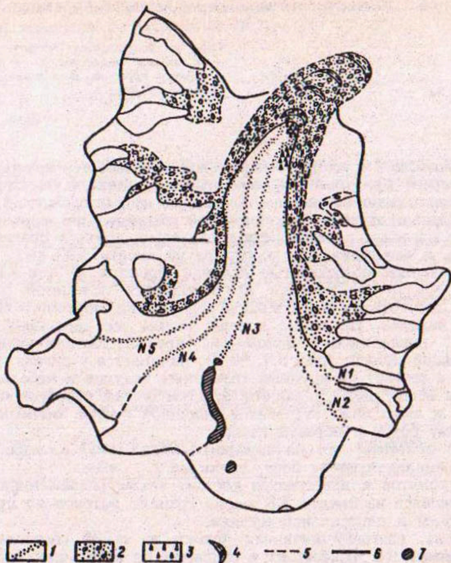
Рис. 6.4. Поверхностные и отложенные морены ледника Абрамова.
