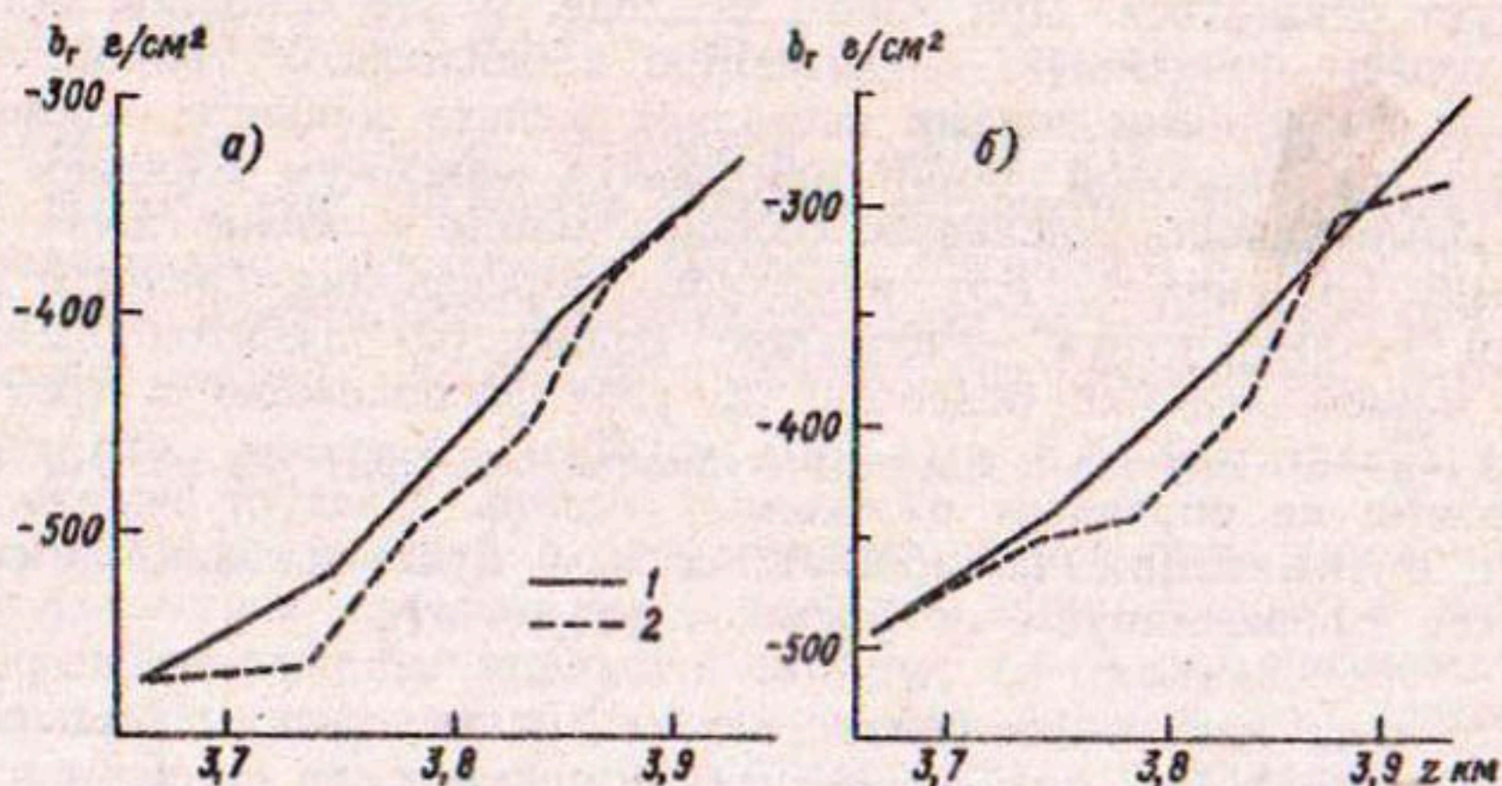
Рис. 3.5. Изменение годового удельного баланса массы ледника b_r с высотой z . а) 1979 г.; б) 1980 г.; 1 — рейки расположены по профилям, 2 — рейки расположены равномерно по площади ледника.
