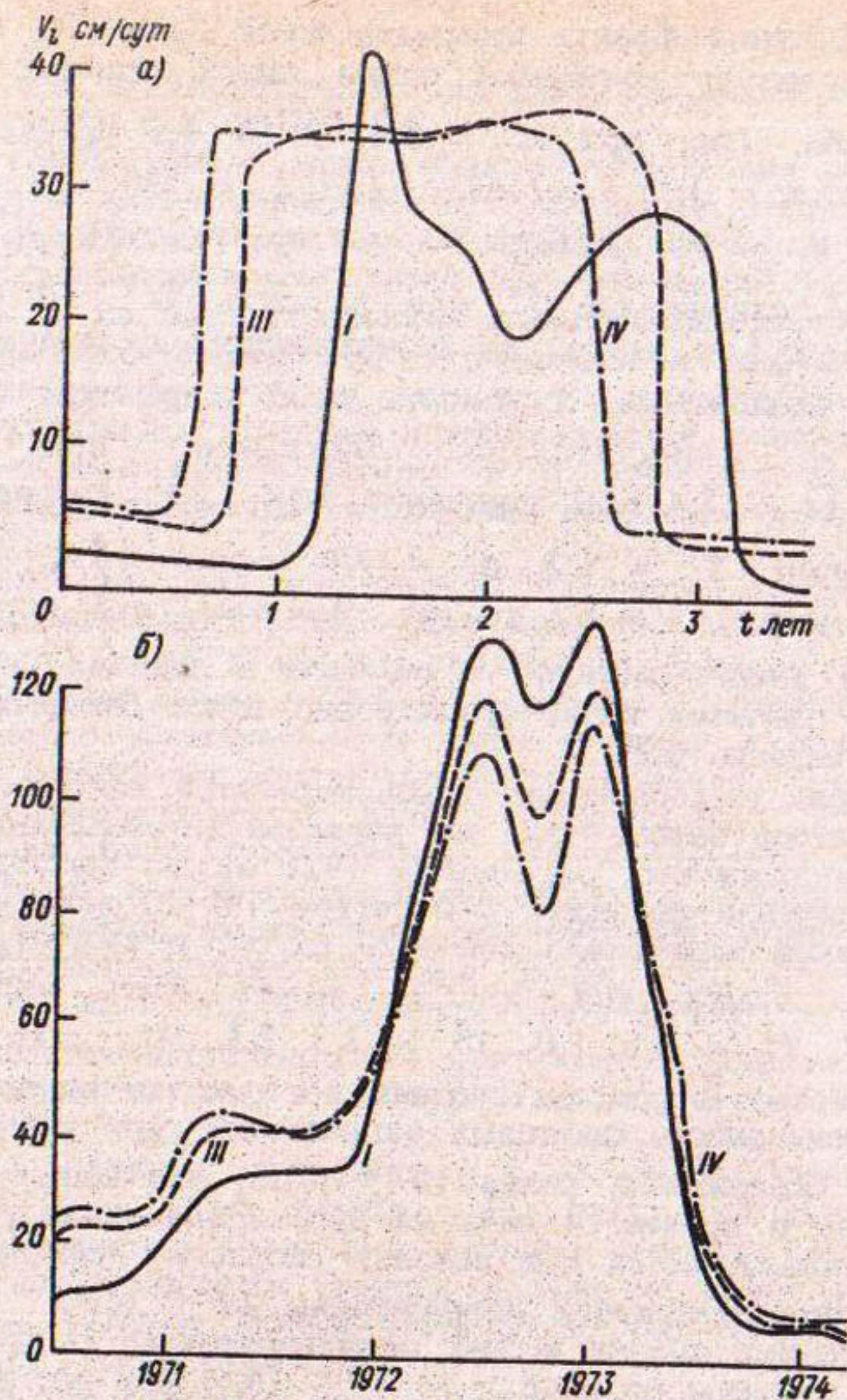
Рис. 5.11. Рассчитанное (а) и измеренное при по- движке 1971—1974 гг. (б) изменение поверхностной скорости движения льда V_i на леднике в поперечных створах I, III, IV.
