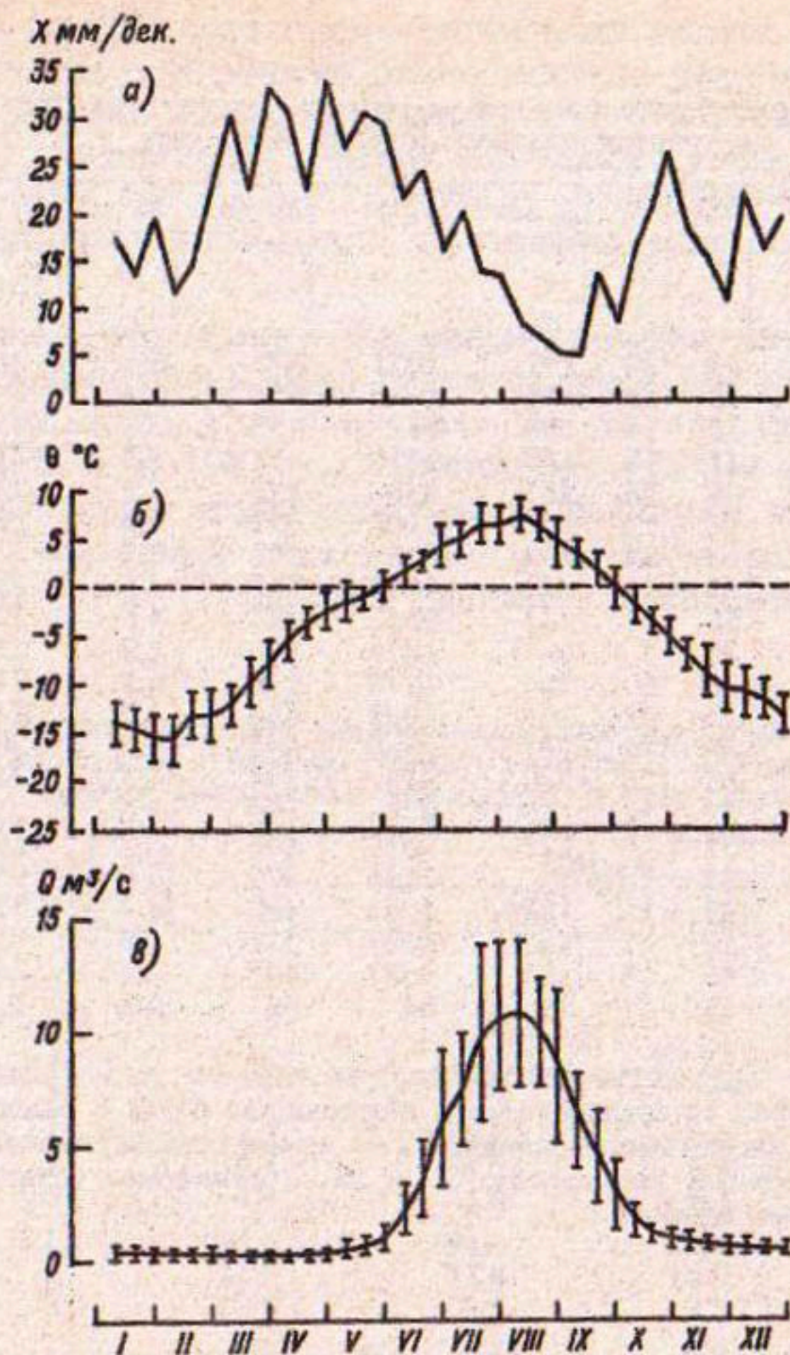
Рис. 2.1. Среднегодовое внутригодовое ход: а) выпадения осадков X , б) среднесуточной температуры воздуха \theta на ст. Ледник Абрамова, морена, в) расхода воды р. Коксу Q . Длина вертикальной линии соответствует стандарту отклонений.
