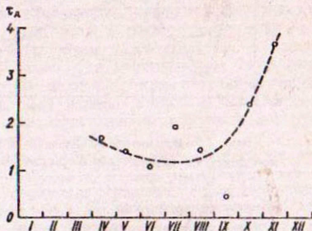
Рис. 4.3. Зависимость сдвига максимума взаимнокорреляционной функции поступления воды и стока \tau_d на леднике Абрамова от времени года.
