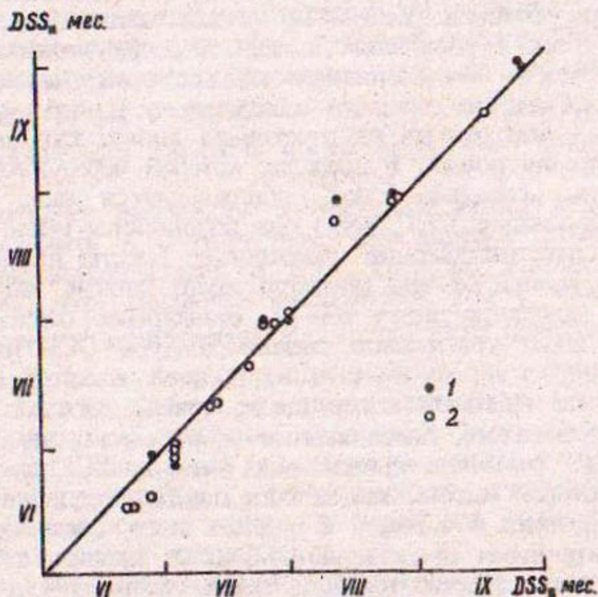
Рис. 4.11. Сравнение дат начала таяния льда в высотных зонах ледника Абрамова в 1985 и 1986 гг., рассчитанных ( DSS_1 ) с помощью формулы (4.7) и определенных по высоте снеговой границы ( DSS_2 ).
