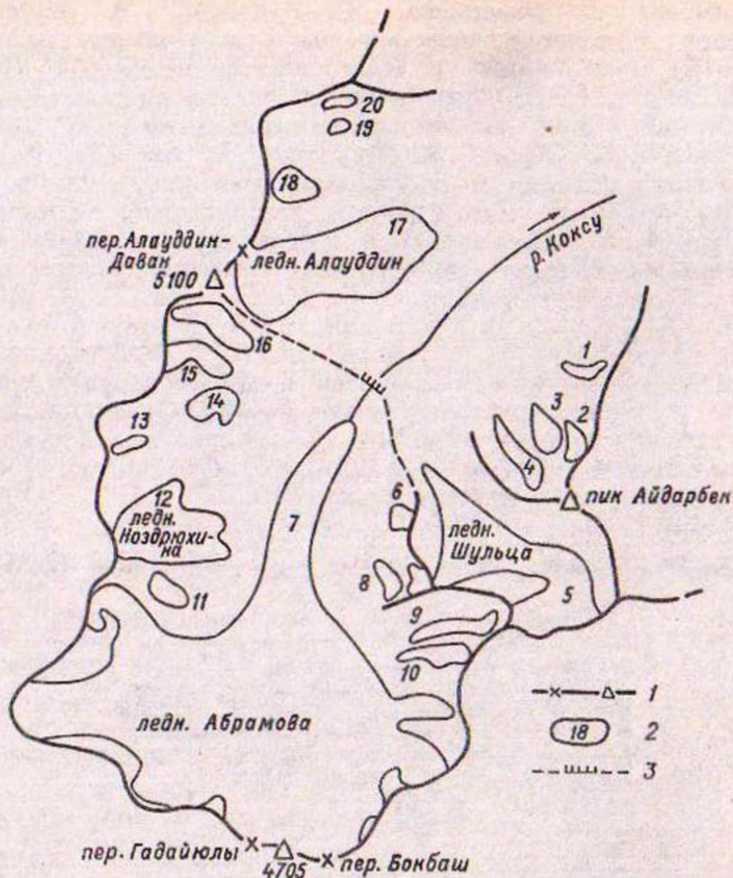
Рис. 1. 1. Схема оледенения верховьев р. Коксу.
