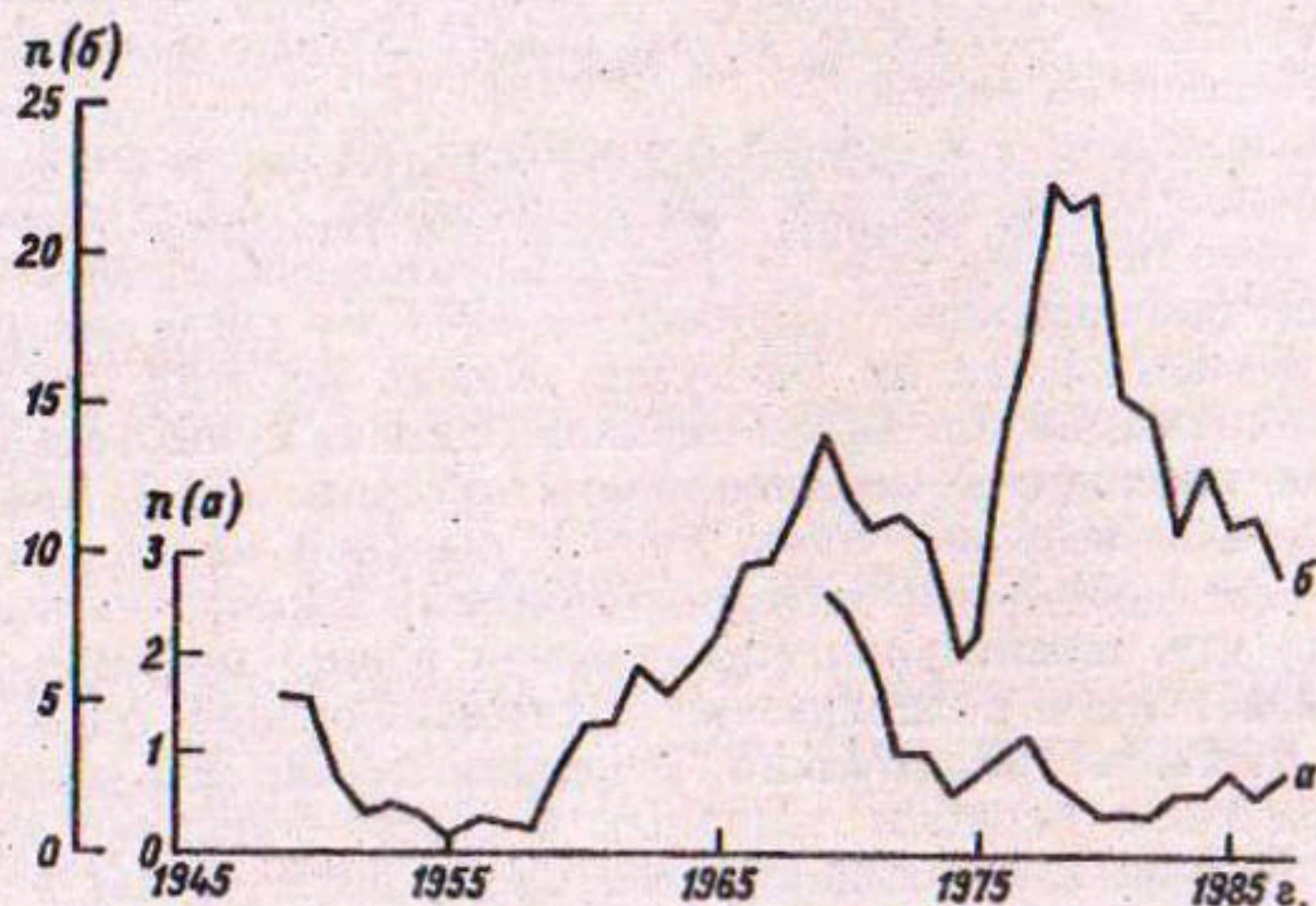
Рис. 2.7. Хронологические графики сглаженных по скользящим пятилетиям чисел дней с пыльной мглой n на станциях Ледник Абрамова ( a ) и Дараут-Курган ( b ).
