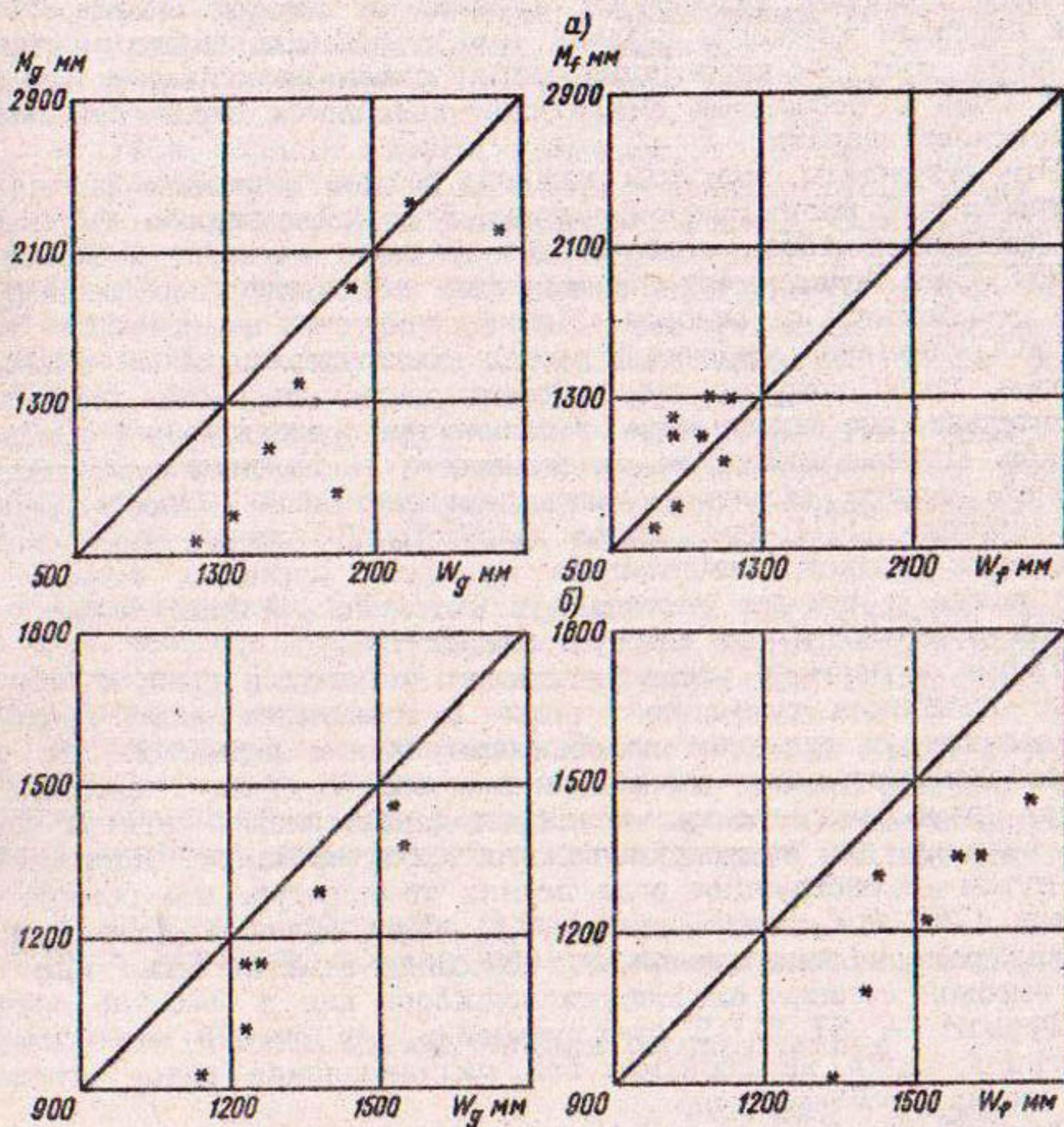
Рис. 4.5. Сравнение годового стока с ледников M_g и склонов M_f с годовым поступлением воды на эти поверхности ( W_g, W_p ).
