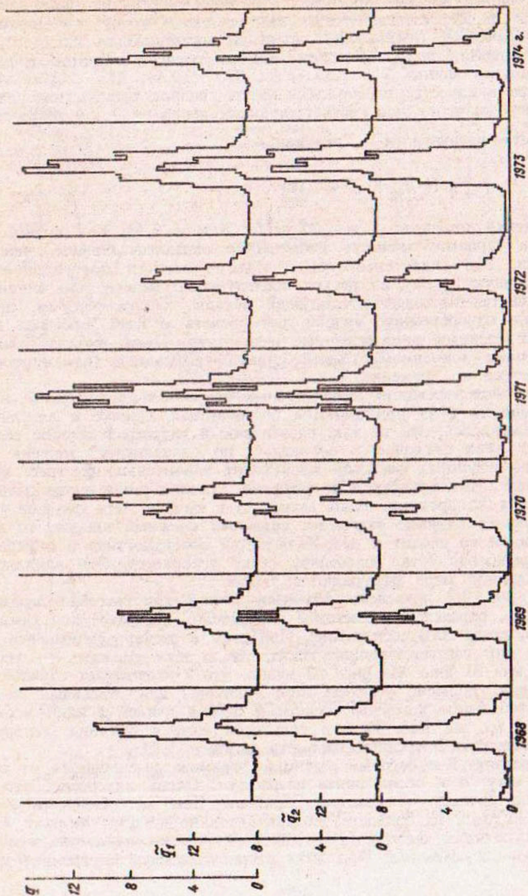
Рис. 4.1. Гидрографы среднего декадного стока с бассейна ледника Абрамова q — измеренный, \tilde{q}_1 — рассчитанный по q_{i-1} и \tilde{q}_2 — рассчитанный по q_{i-1} и \tilde{q}_{n_i}
