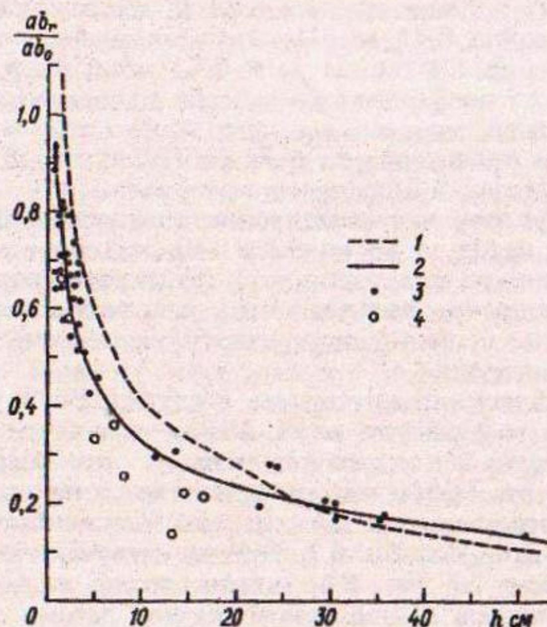
Рис. 6.6. Зависимость относительной величины таяния под мореной ab_r/ab_0 от толщины морены h .
