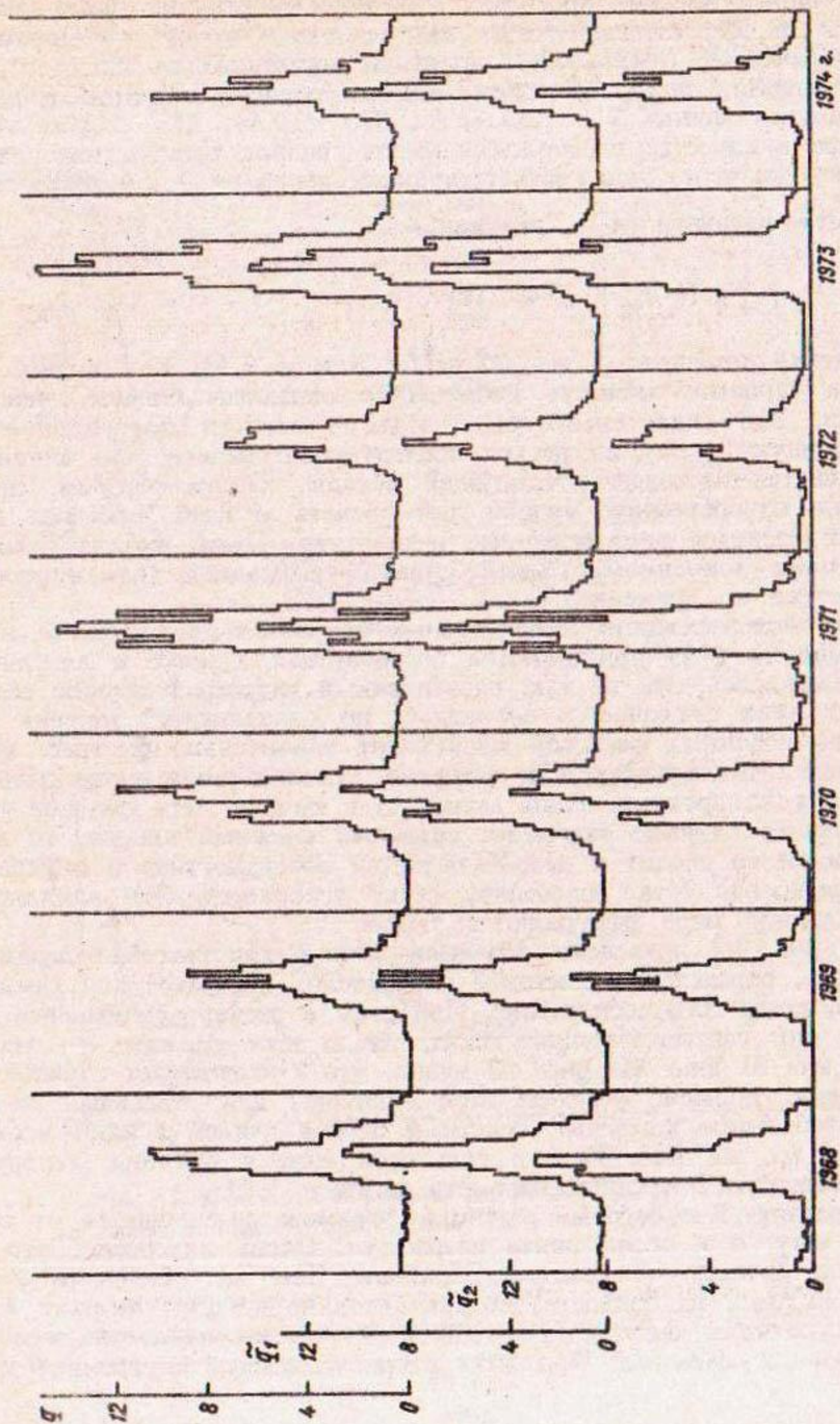
Рис. 4.1. Гидрографы среднего декадного стока с бассейна ледника Абрамова q — измеренный, \tilde{q}_1 — рассчитанный по q_{i-1} и \tilde{q}_{n_i-1} , \tilde{q}_2 — рассчитанный по q_{i-1} и \tilde{q}_{n_i}
