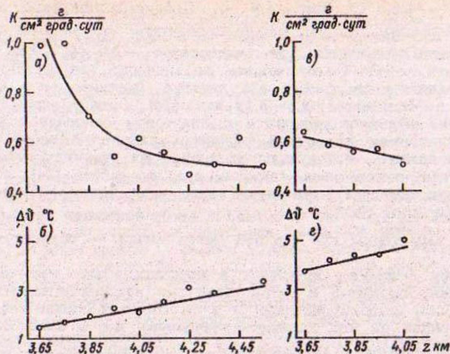
Рис. 4.9. Изменение параметров формул (4.7) с высотой z . а, б) — для таяния снега и фирна; в, г) — для таяния льда.
