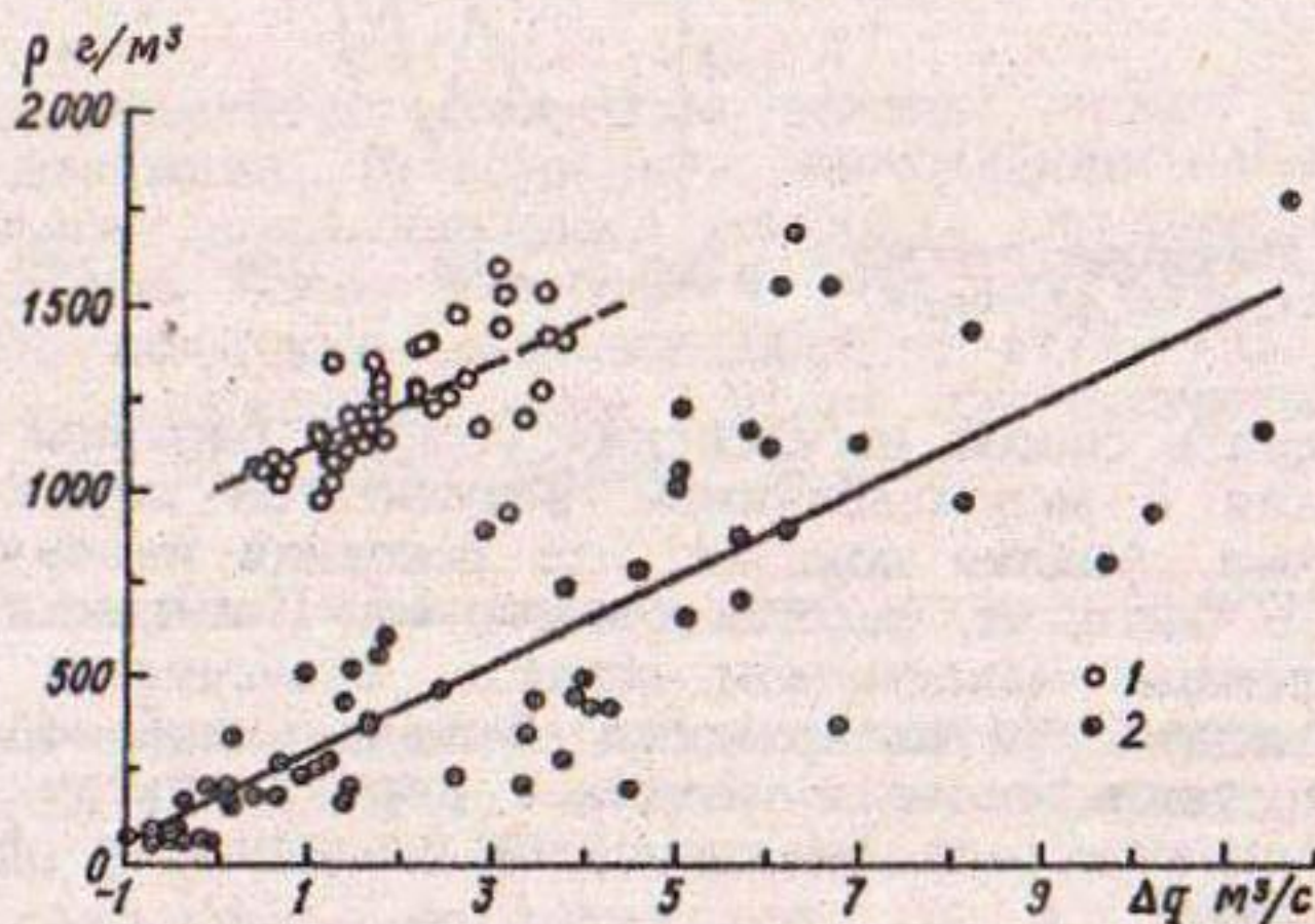
Рис. 4.29. Зависимость \rho(\Delta q) по данным за лето 1982 г.
