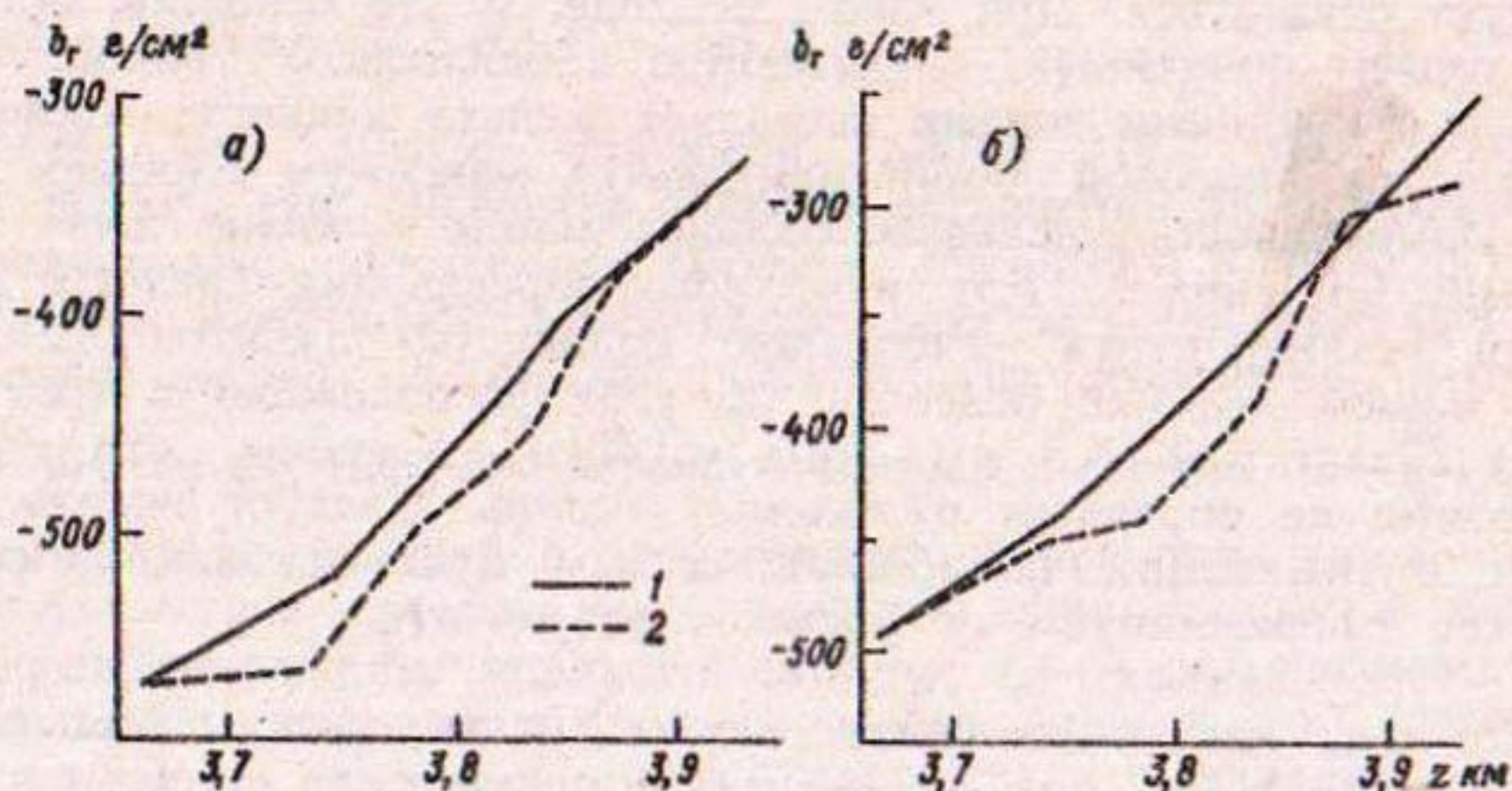
Рис. 3.5. Изменение годового удельного баланса массы ледника b_r с высотой z .
