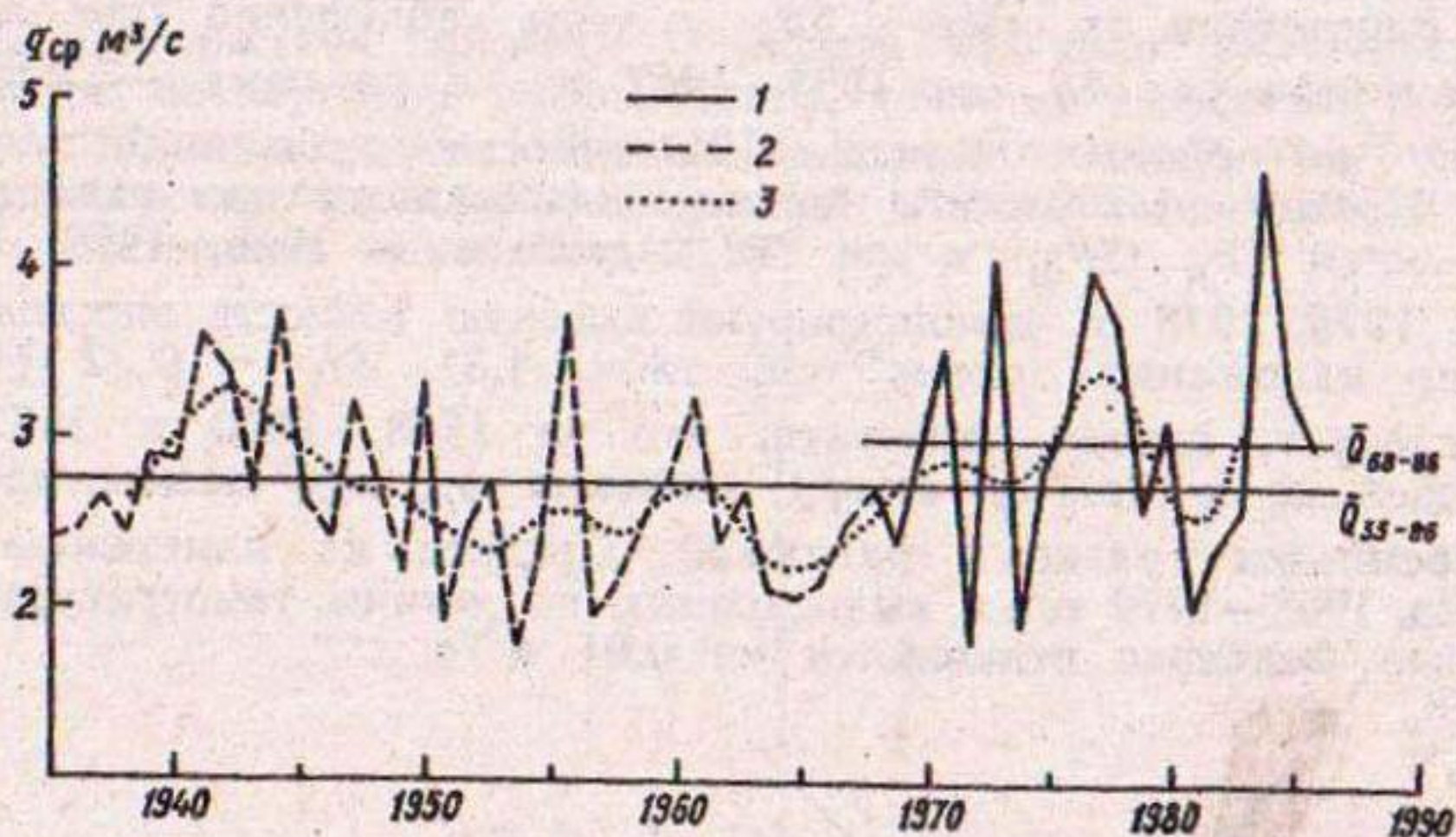
Рис. 4.26. Хронологический график хода среднегодовых расходов воды q_{\text{ср}} р. Коксу.
