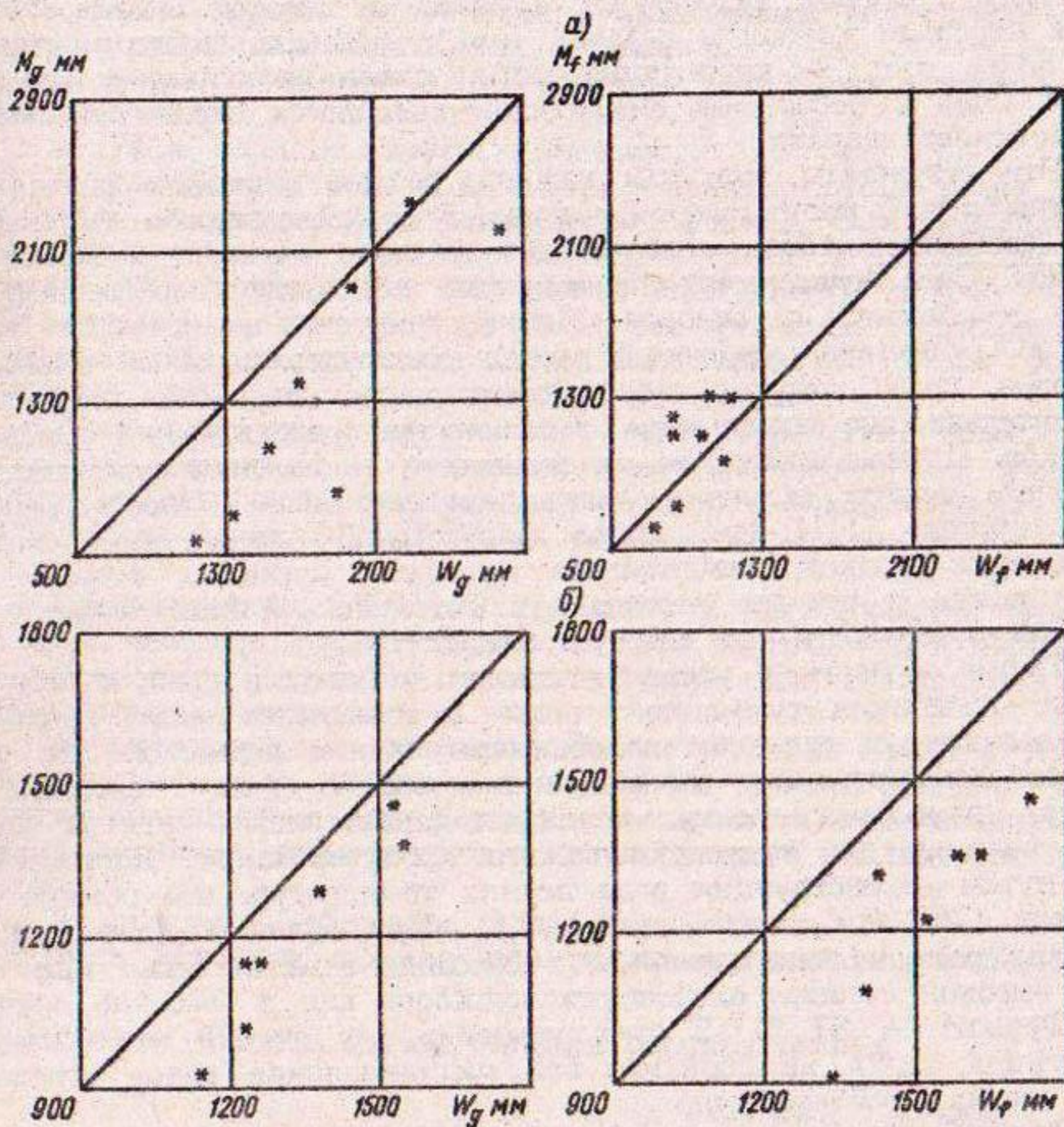
Рис. 4.5. Сравнение годового стока с ледников M_g и склонов M_f с годовым поступлением воды на эти поверхности ( W_g, W_f ).
