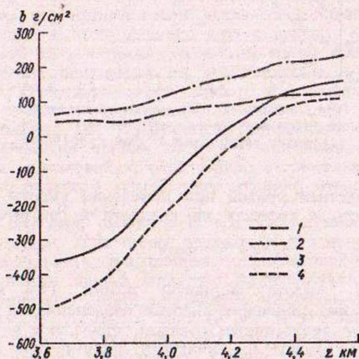
Рис. 3.3. Изменение удельного баланса массы ледника b с высотой z в различные месяцы 1990 г. 1, 2, 3, и 4 — январь, май, август и сентябрь.
