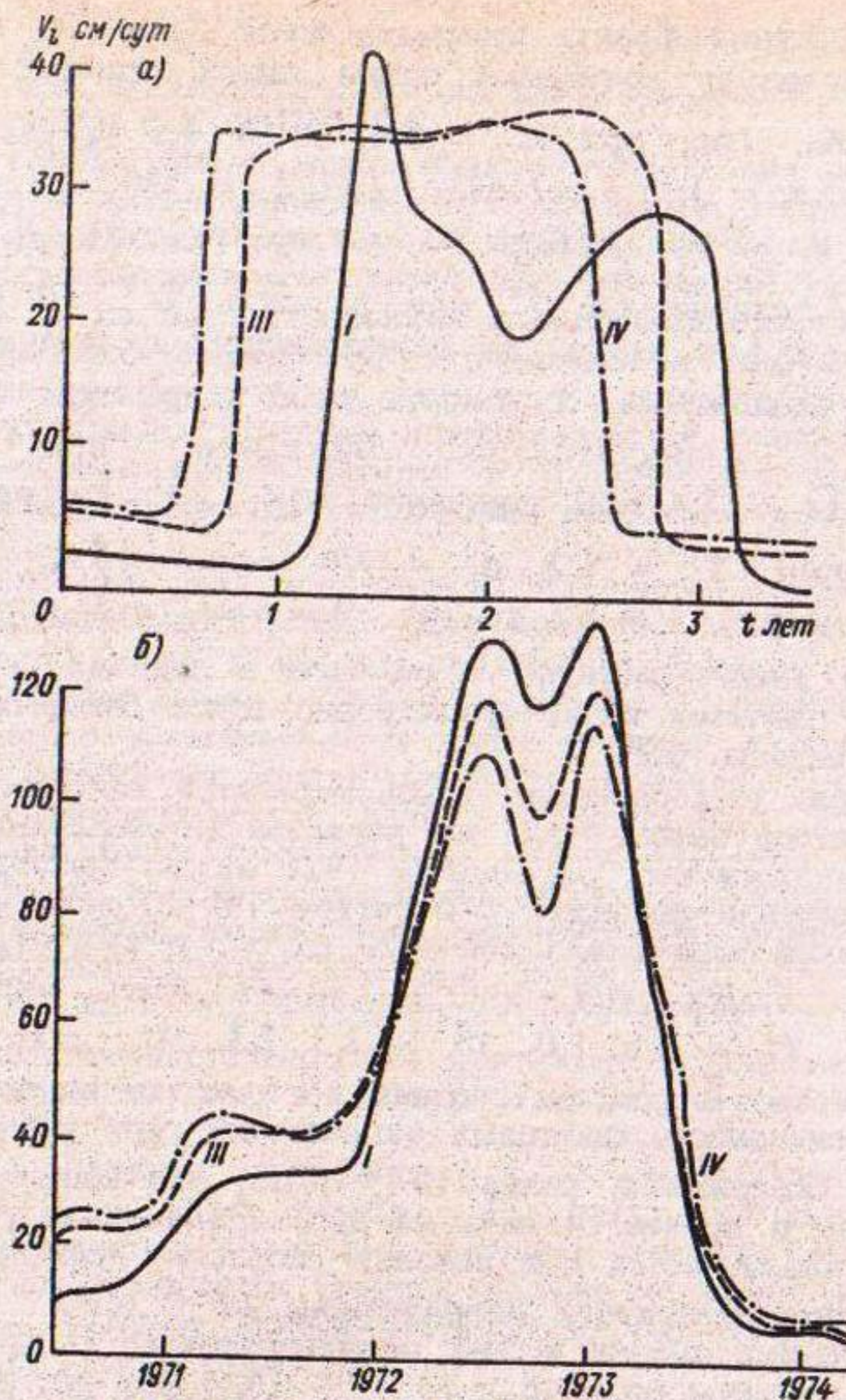
Рис. 5.11. Рассчитанное (а) и измеренное при по- движке 1971—1974 гг. (б) изменение поверхностной скорости движения льда V_1 на леднике в поперечных створах I, III, IV.
