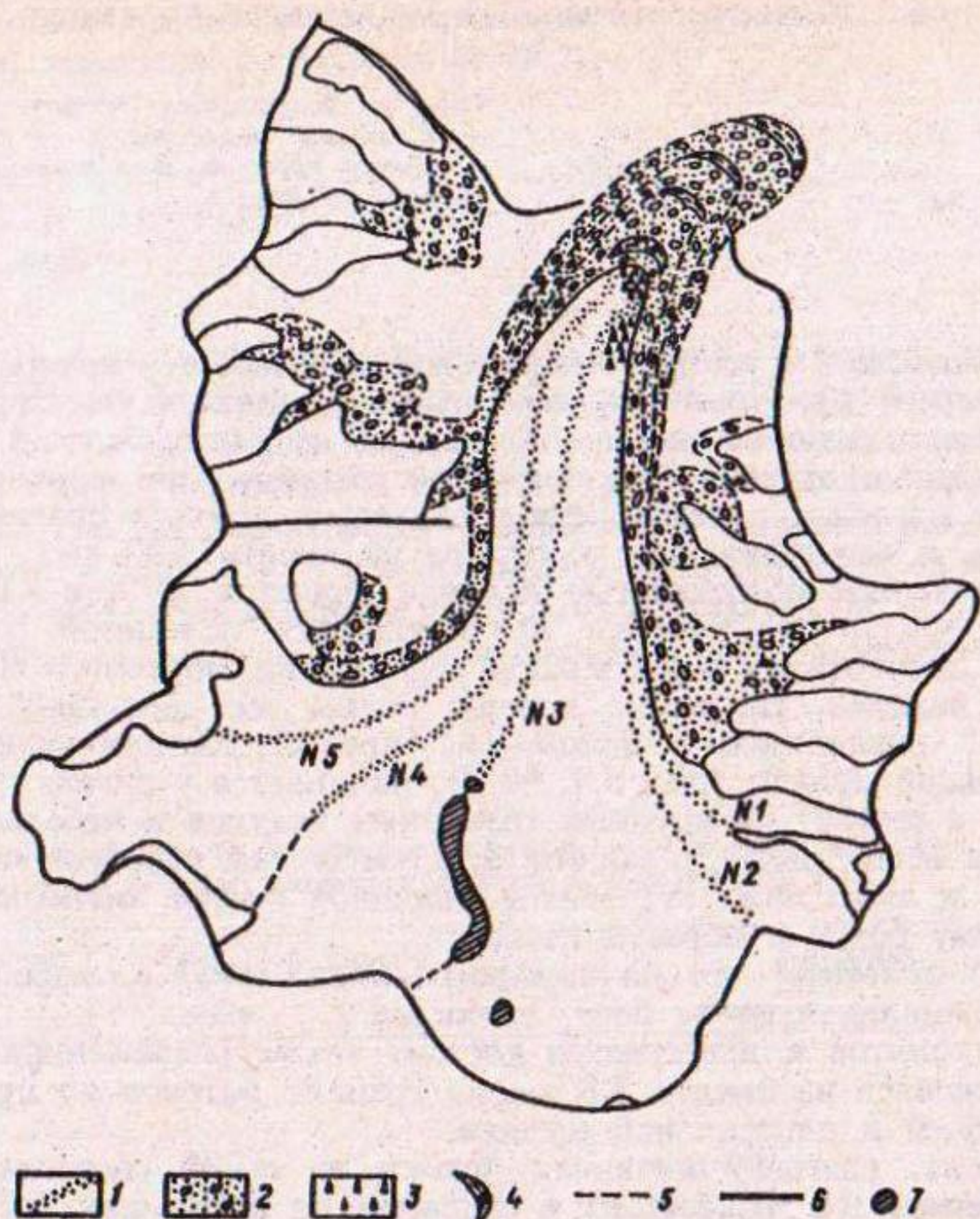
Рис. 6.4. Поверхностные и отложенные морены ледника Абрамова.
