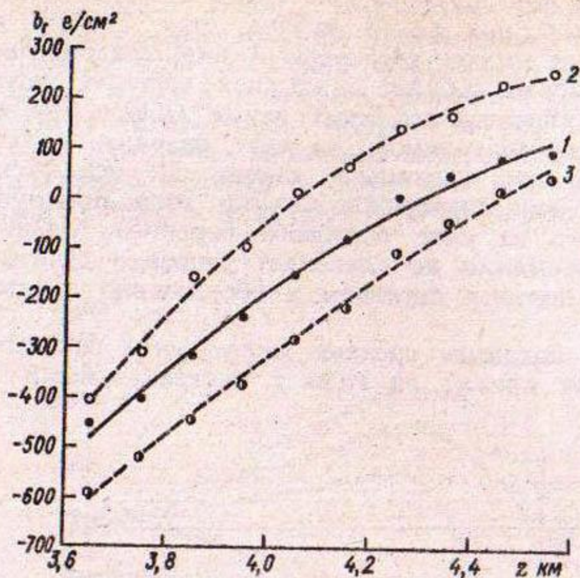
Рис. 3.4. Изменение годового удельного баланса массы ледника b_r с высотой ( z ). 1) среднее многолетнее; 2) 1969 г.; 3) 1984 г.
