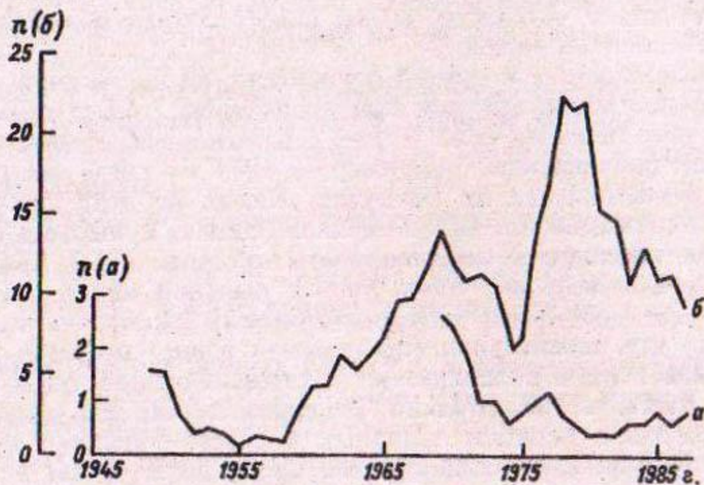
Рис. 2.7. Хронологические графики сглаженных по скользящим пятилетиям чисел дней с пыльной мглой n на станциях Ледник Абрамова (а) и Дараут-Курган (б).
