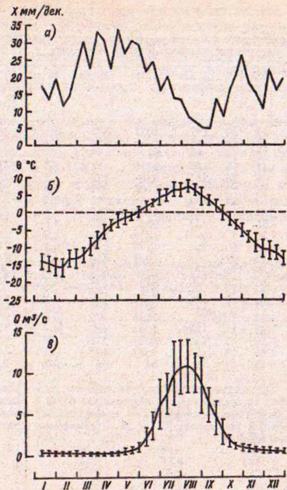
Рис. 2.1. Среднегодовой внутригодовой ход: а) выпадения осадков X , б) среднесуточной температуры воздуха \theta на ст. Ледник Абрамова, морена, в) расхода воды р. Коксу Q . Длина вертикальной линии соответствует стандарту отклонений.
