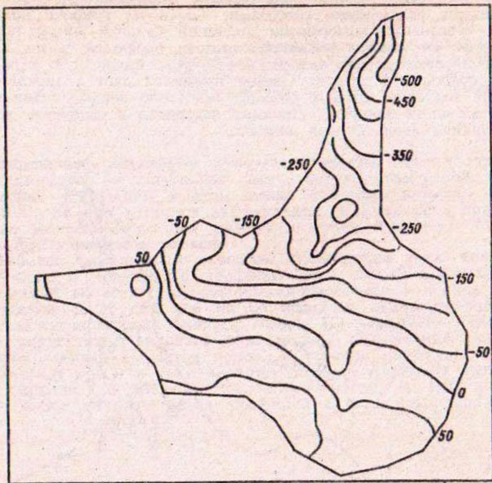
Рис. 3.7. Изолинии баланса массы ледника ( \text{г/см}^2 ). 1990 г.
