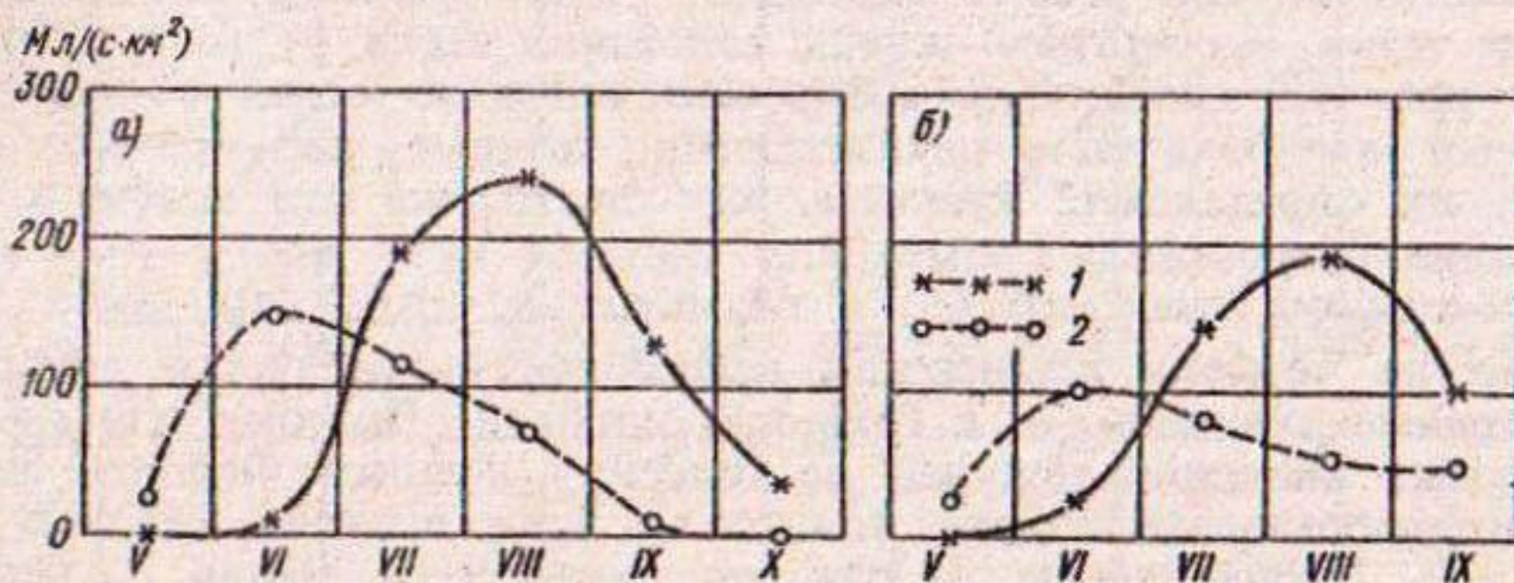
Рис. 4.4. Внутригодовой ход модулей стока M с ледников (1) и окружающих их склонов (2).
