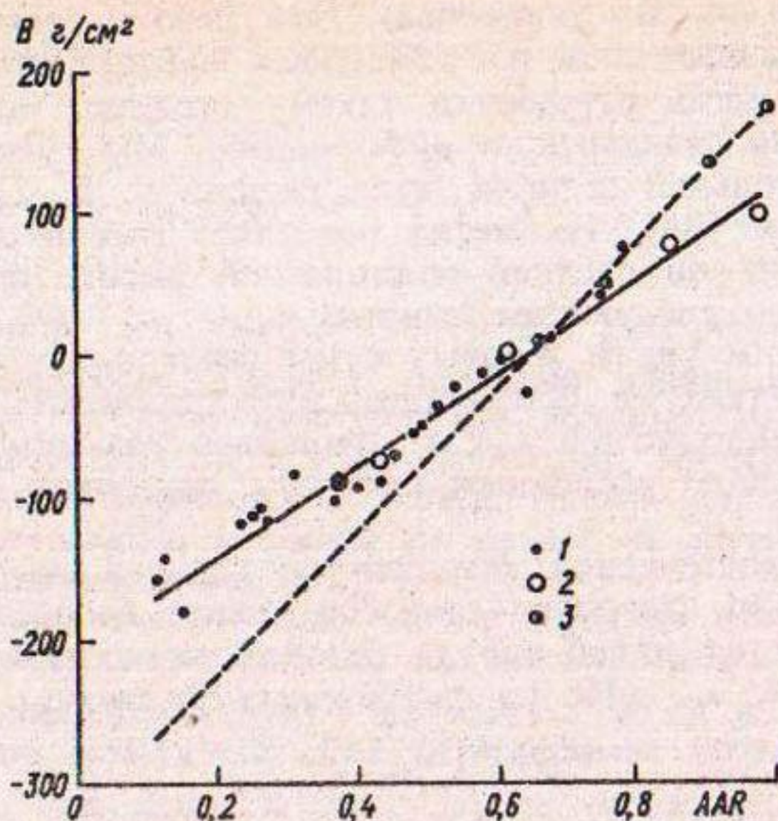
Рис. 3.12. Зависимость годового и текущих балансов массы ледника Абрамова B от доли площади ледника выше снеговой границы (AAR).
