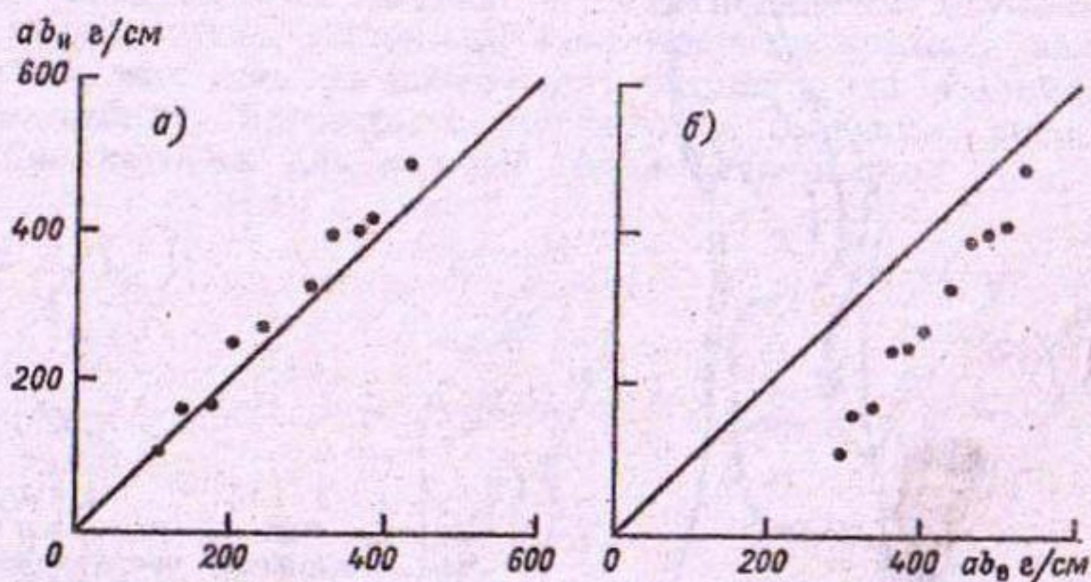
Рис. 4.8. Сравнение среднего по 50-метровым интервалам высоты измеренного удельного таяния ab_n на языке ледника Абрамова с рассчитанным ab_n .
