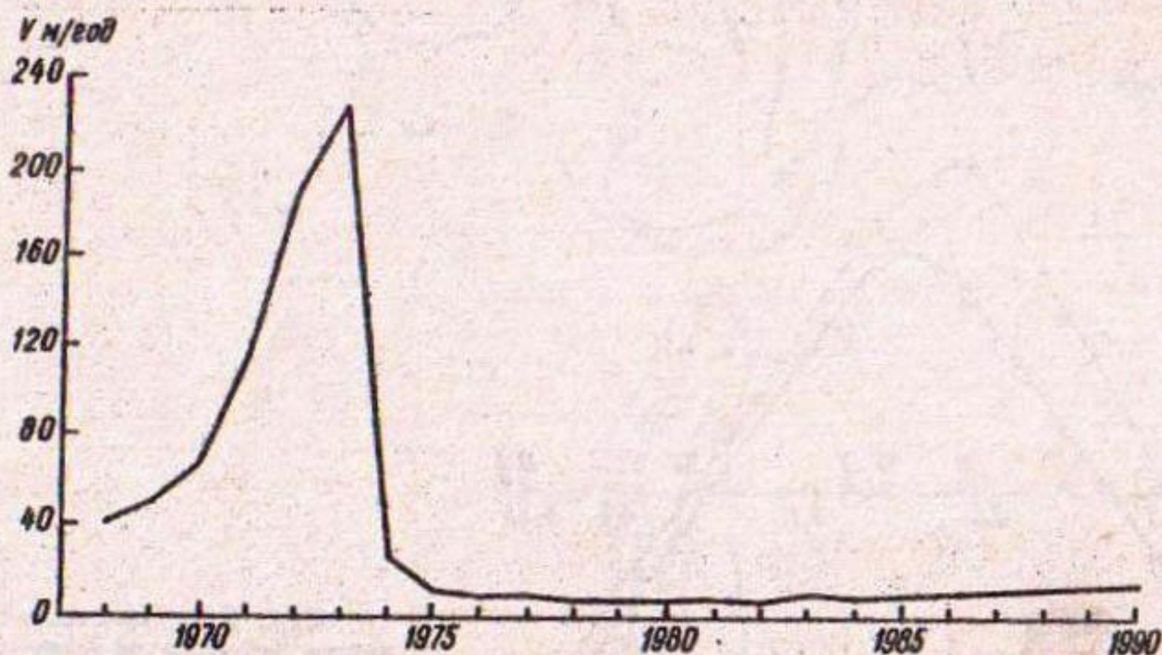
Рис. 5.3. Хронологические изменения средней поверхностной скорости движения льда V на 2-м поперечном профиле.
