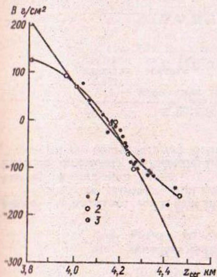
Рис. 3.11. Зависимость годового и текущих балансов массы ледника Абрамова B от высоты снеговой границы z_{csg} .
