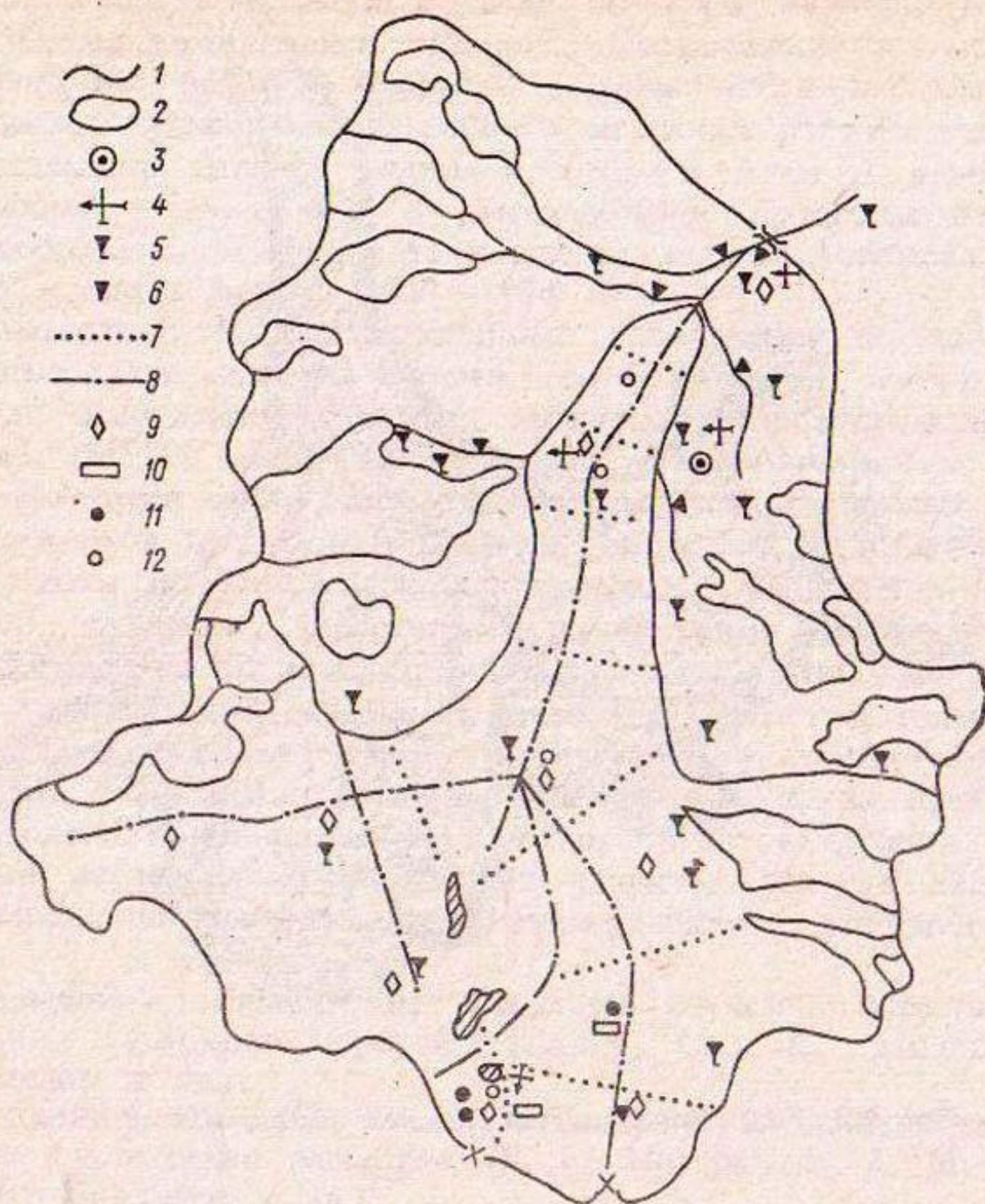
Рис. 1.2. Схема бассейна ледника Абрамова.
