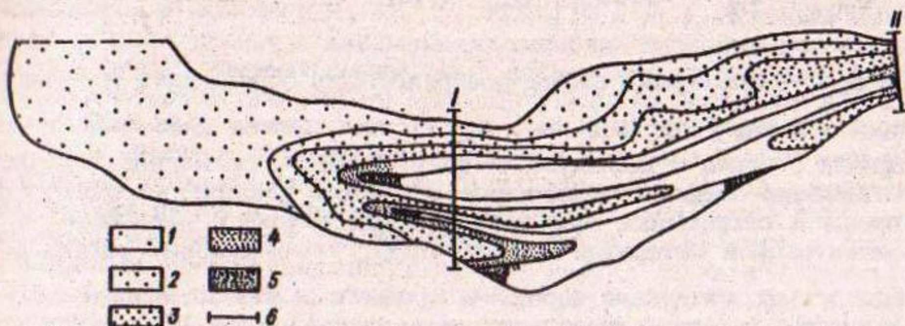
Рис. 6.5. Фрагмент карты моренного покрова на левой боковой гряде в языковой части ледника.
