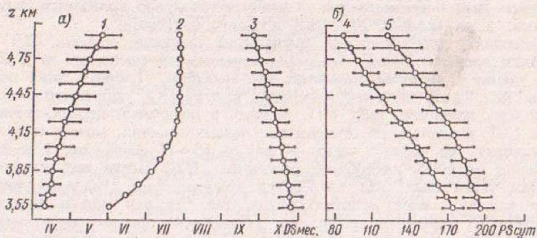
Рис. 4.13 Изменение с высотой ( z ) средних многолетних характеристик сезона таяния на неледниковых склонах дат DS (а) начала таяния снежного покрова (1), снежников (2), конца таяния (3) и числа дней PS (б) с таянием (4) и продолжительности периода таяния (5).
