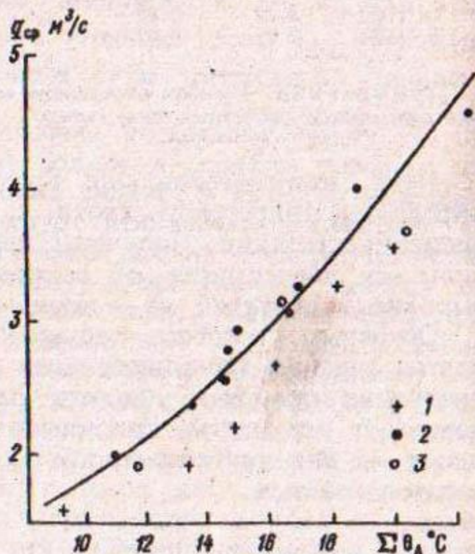
Рис. 4.24. Связь среднегодового расхода воды q_{\text{ср}} р. Коксу с суммой среднемесячных летних температур воздуха \Sigma\theta_A на станции Ледник Абрамова.
