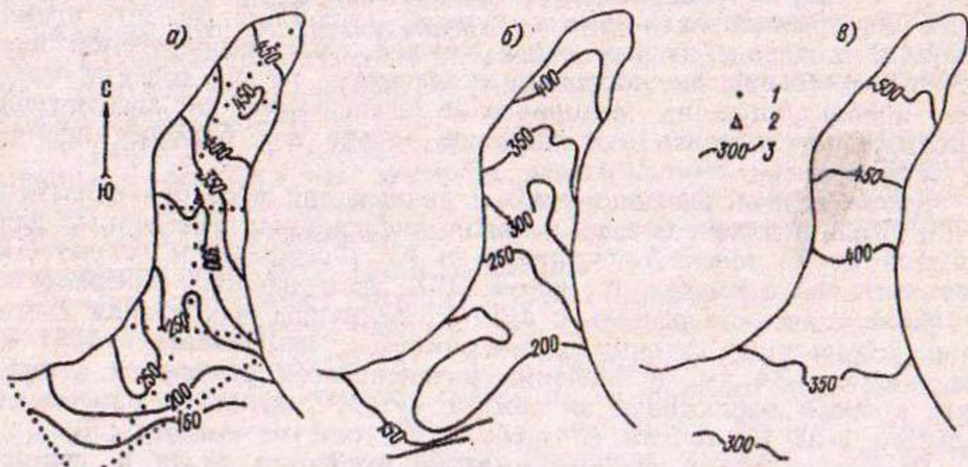
Рис. 4.6. Распределение годового удельного таяния ( \text{г/см}^2 ) на языке ледника Абрамова.
