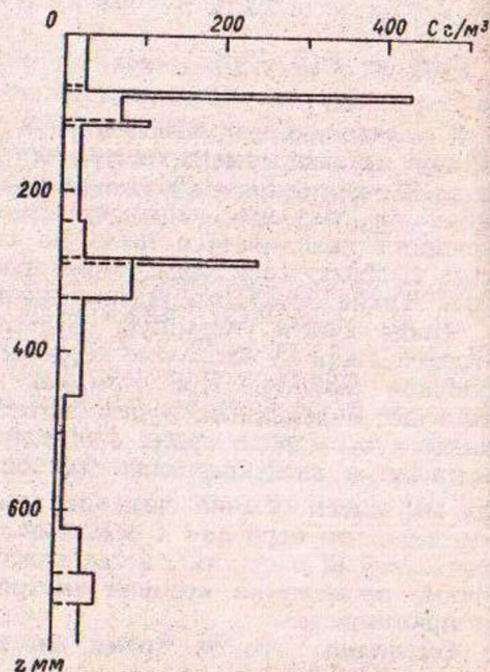
Рис. 6.1. Рассчитанный профиль концентрации пыли C в сезонном снегу.
