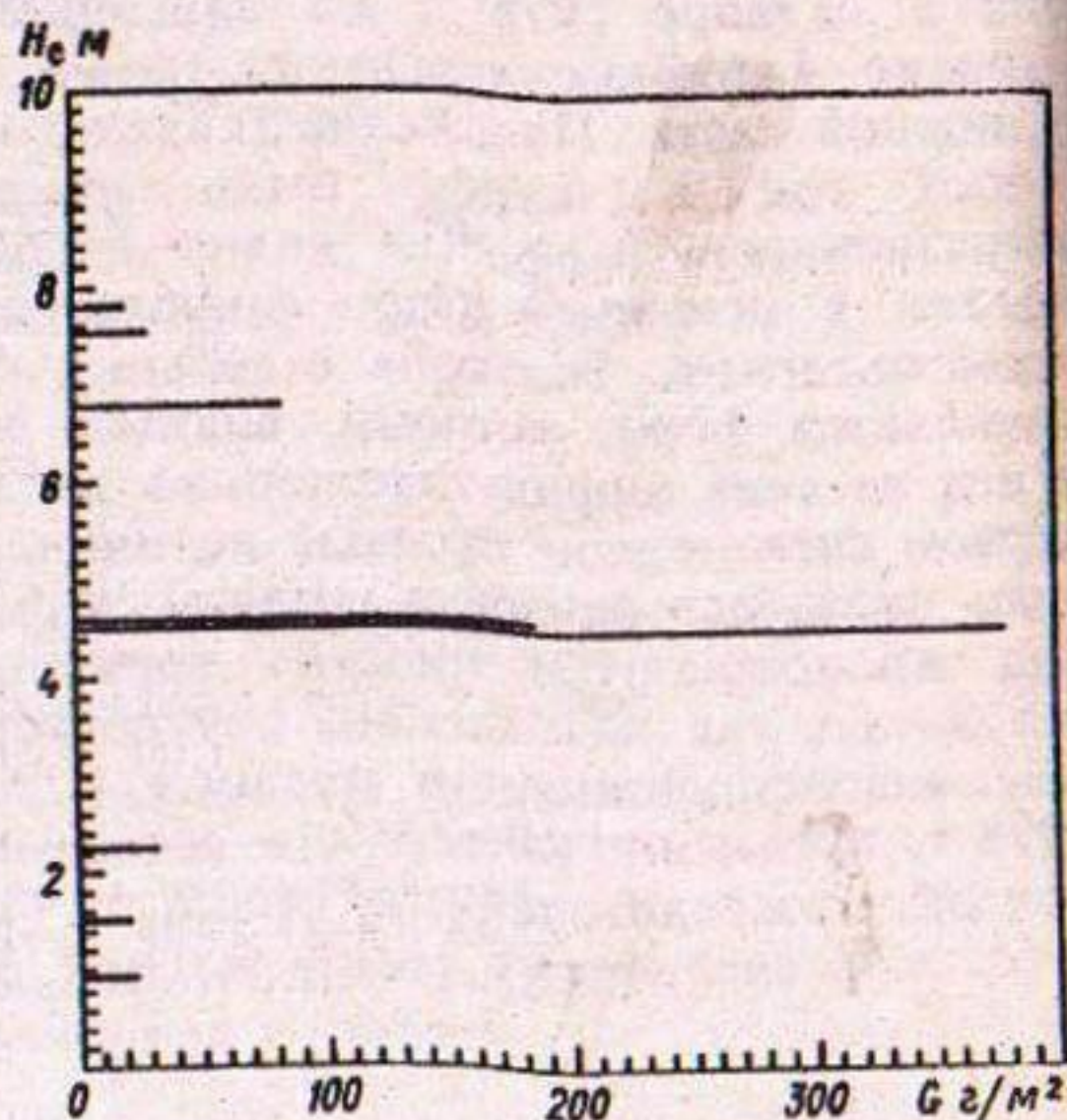
Рис. 7.12. Распределение загрязненности льда G по глубине шурфа
