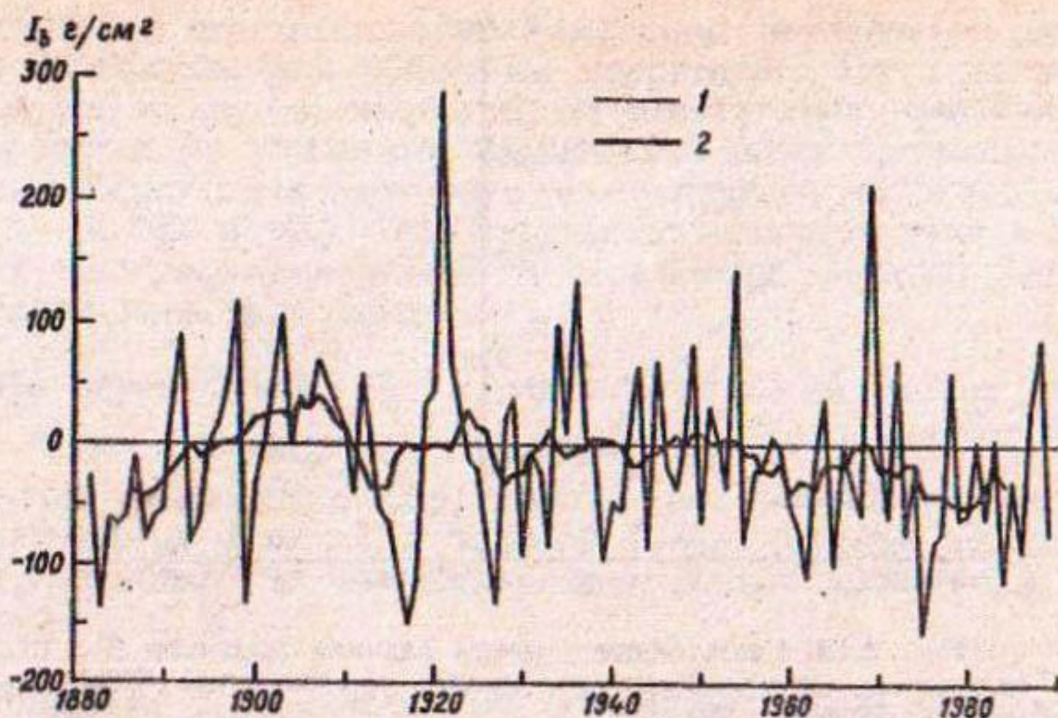
Рис. 3.14. Хронологический ход индекса баланса массы ледника Абрамова I_b , рассчитанный по данным ст. Фергана. 1 — ежегодные, 2 — сглаженные значения.
