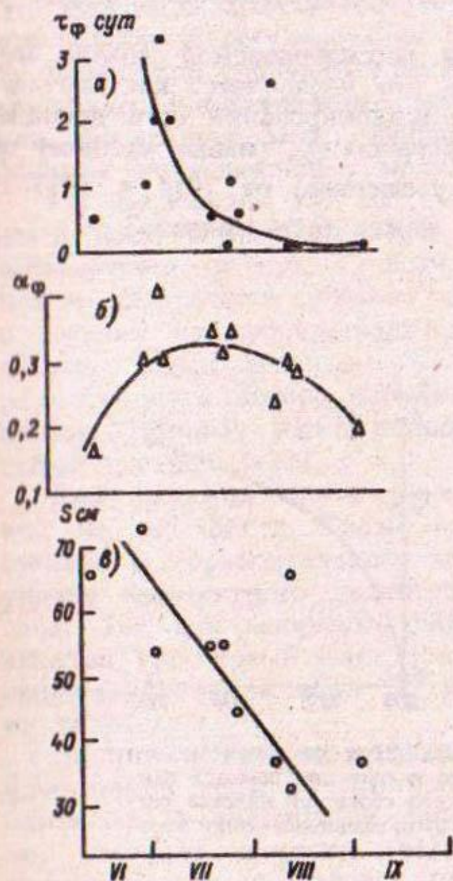
Рис. 4.15. Изменение с течением времени t внутри года времени просачивания талых вод \tau_{\phi} с поверхности до горизонта внутрифирновых вод (а), индекса развития дренажной сети \alpha_{\phi} (б) и стандартной ошибки расчета уровней S (в).
