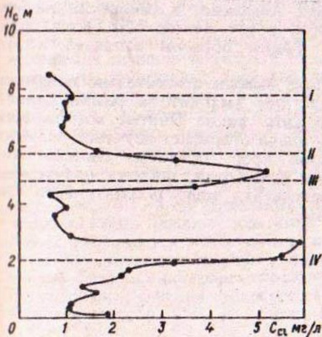
Рис. 7.15. Распределение по глубине шурфа в снежнике H_c концентрации ионов хлора во льду C_{cl} .
