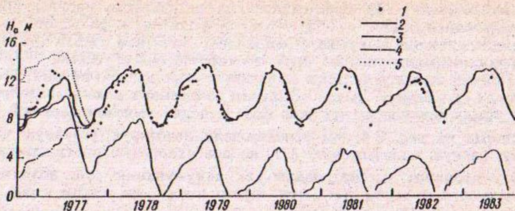
Рис. 7.7. Хронологический ход измеренной и вычисленной мощностей снежника H_c .
