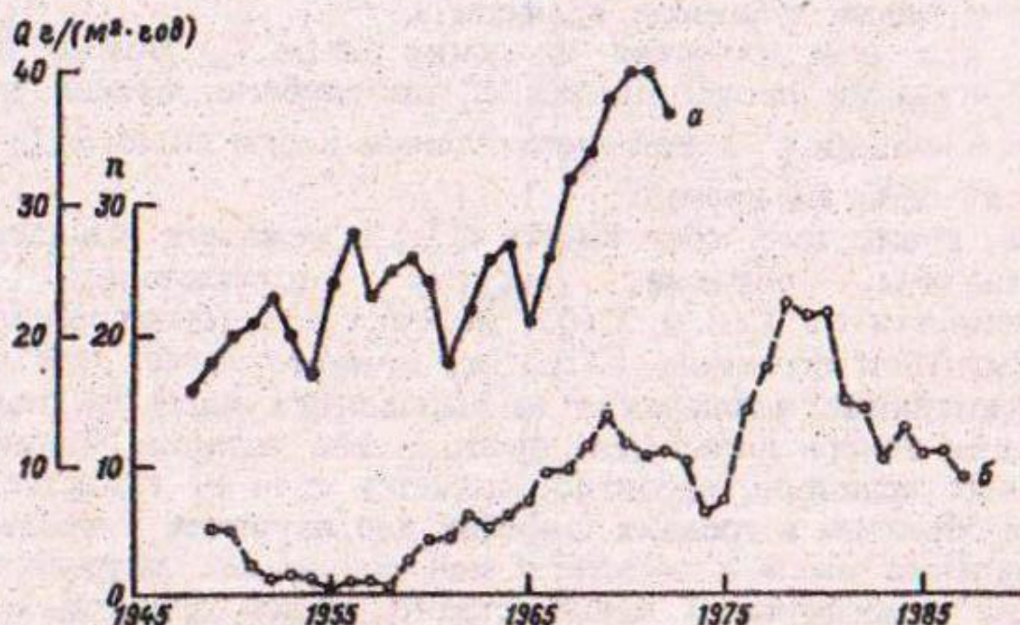
Рис. 6.2. Хронологические графики выпавших в фирновой области ледника годовых количеств пыли Q (а) и числа дней n с пыльной мглой за год на станции Дараут-Курган (б).
