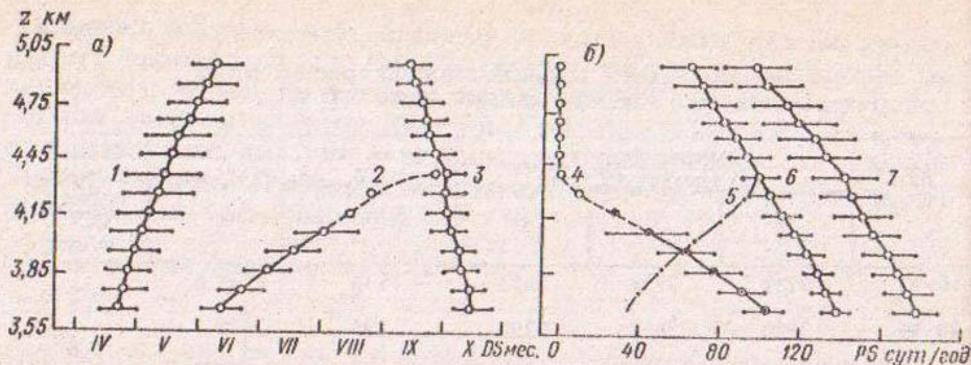
Рис. 4.12 Изменение с высотой z средних многолетних характеристик сезона таяния на ледниках дат DS (а) начала таяния снега (1), льда (2), конца таяния (3) и числа дней PS (б) с таянием льда (4), снега (5), их суммы (6) и продолжительности периода таяния (7).
