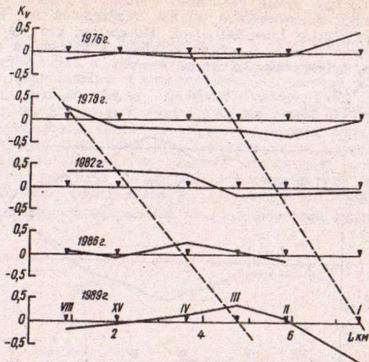
Рис. 5.5. Изменение скорости движения K_v по длине ледника L от перевала к языку.
