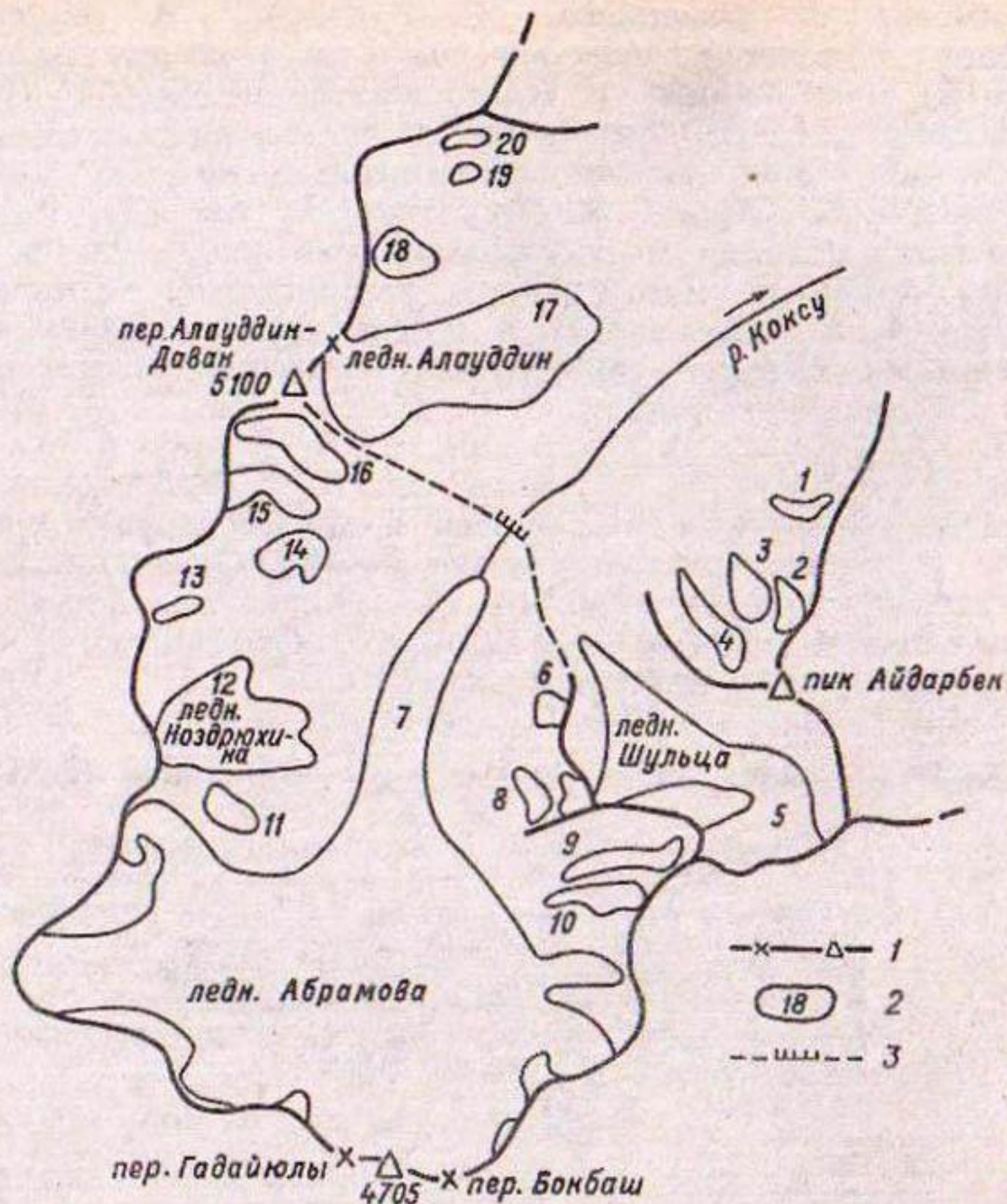
Рис. 1. 1. Схема оледенения верховьев р. Коксу.
