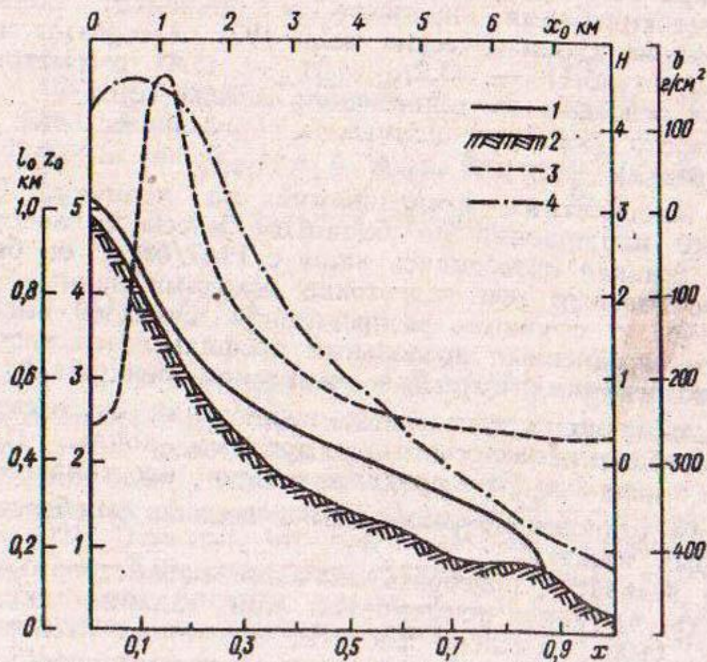
Рис. 5.7. Исходные данные для моделирования динамики ледника Абрамова.
