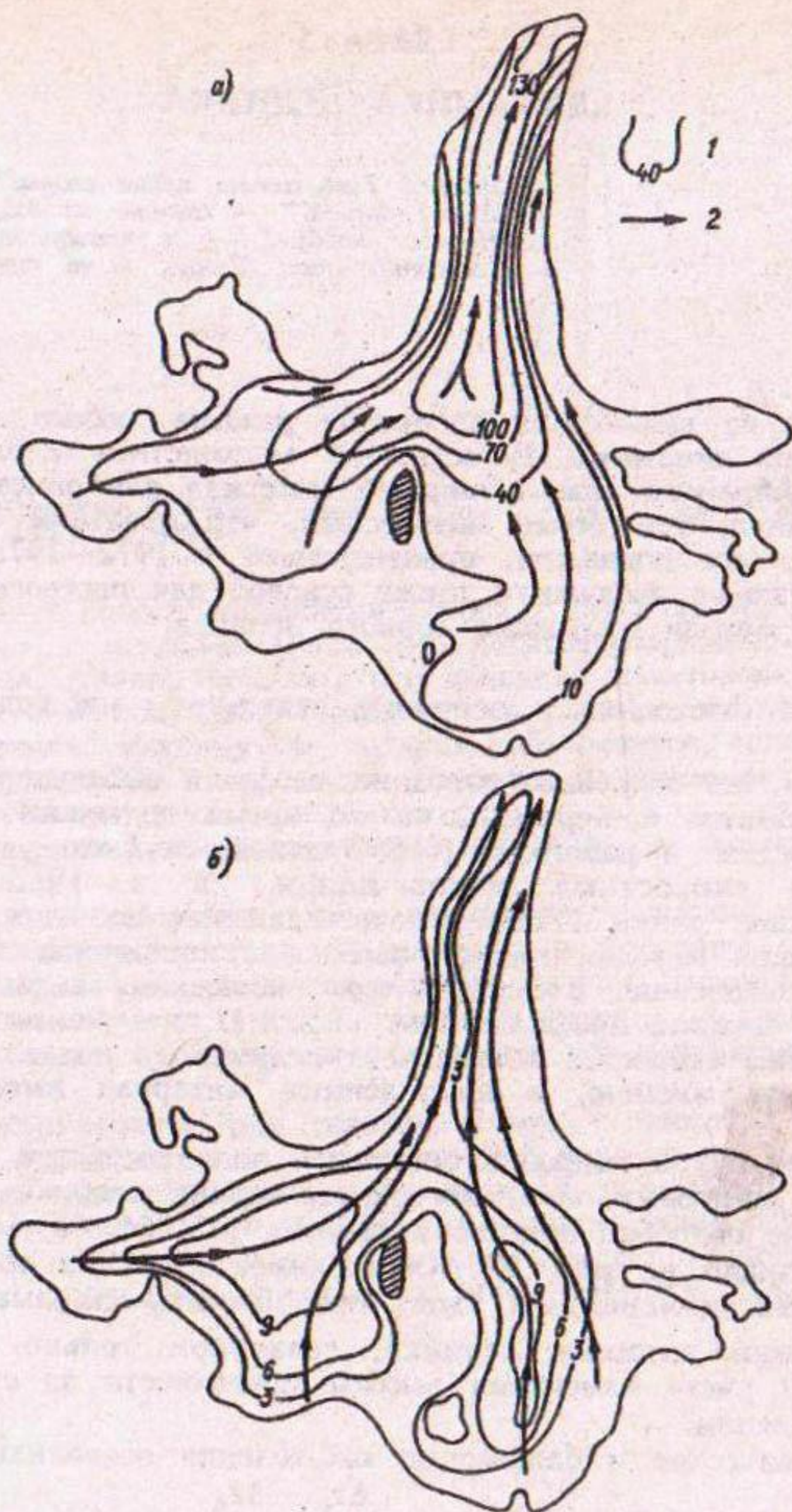
Рис. 5.1. Карта-схема поверхностных скоростей движения льда в период подвижки в 1973 г. (а) и в спокойный период в 1976 г. (б). 1 — изотакхи, см/сут; 2 — линии тока.
