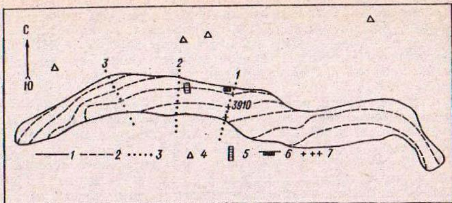
Рис. 7.3. Схема навейного снежника и расположение пунктов измерений на нем.
