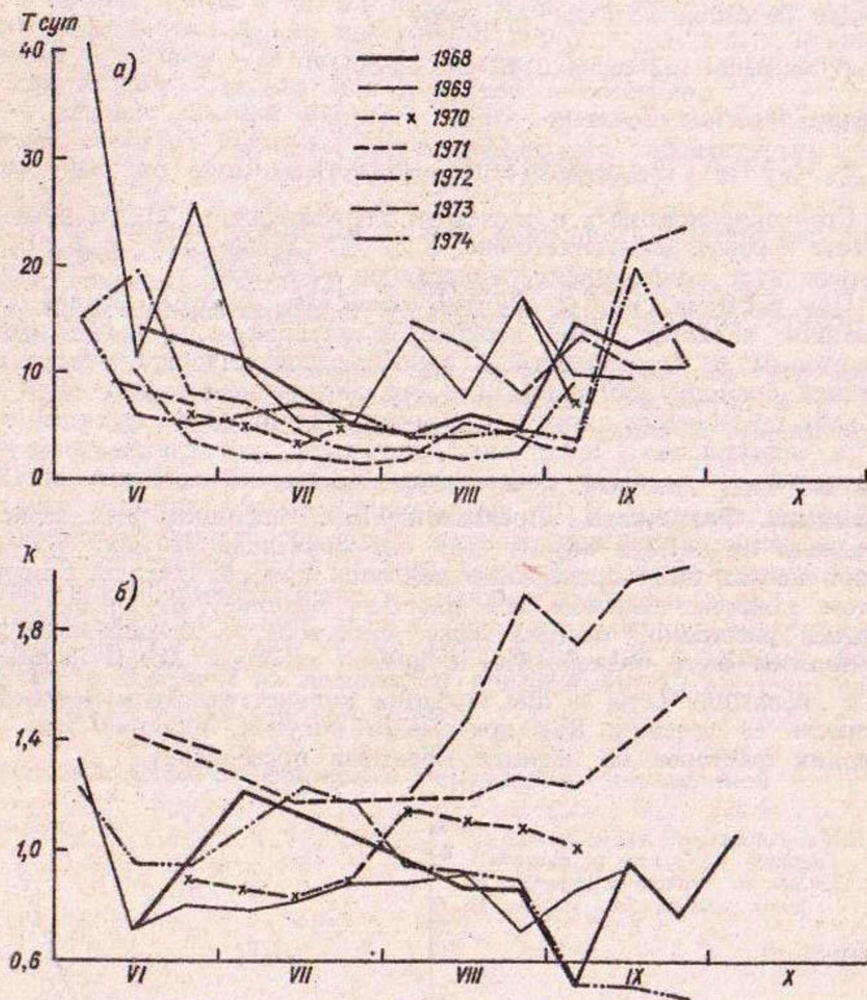
Рис. 4.2. Изменения во времени параметров T_{сут} (а) и k (б) однообъемной линейной модели трансформации для бассейна ледника Абрамова.
