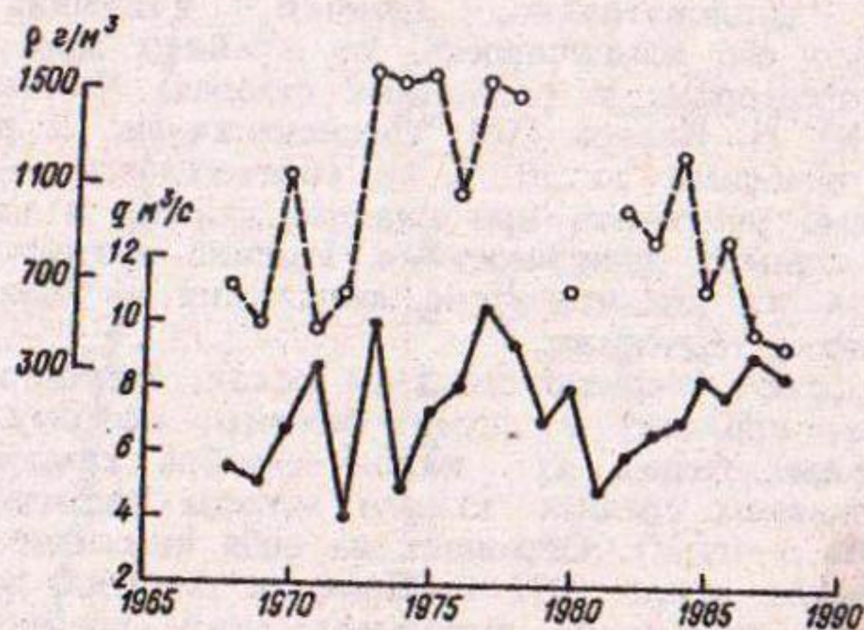
Рис. 4.28. Многолетний ход средних за июнь — сентябрь расходов воды q и мутности воды \rho р. Коксу у ледника Абрамова.
