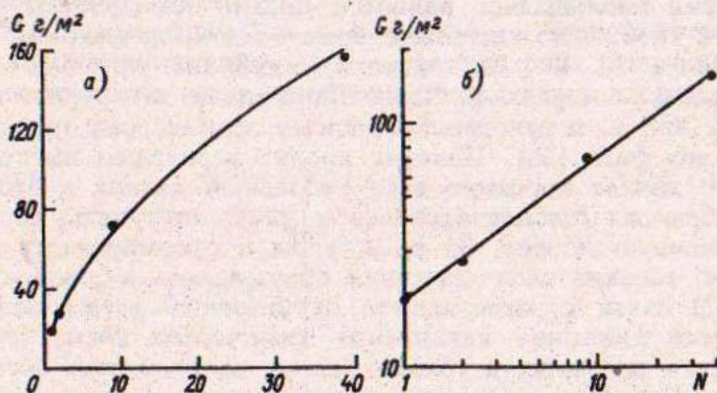
Рис. 7.14. Зависимость загрязненности слоя G от числа лет, за которые он сформировался N .
