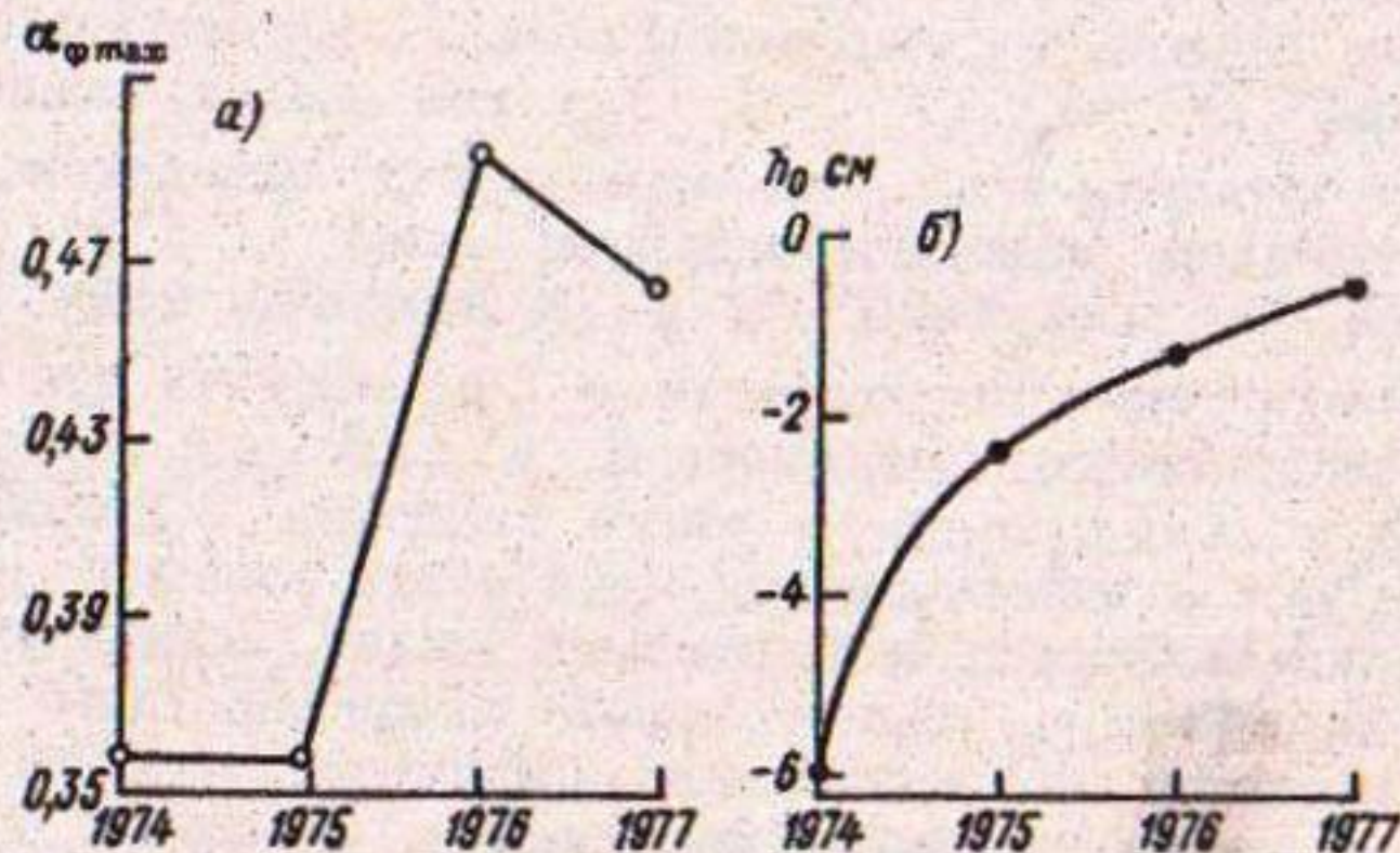
Рис. 4.16. Изменение параметров линейной модели режима уровней воды от года к году для периода наилучшего функционирования сети стока: а) индекса развития дренажной сети \alpha_{f \max} ; б) превышения рейки уровня над краем „водослива“ h_0 .
