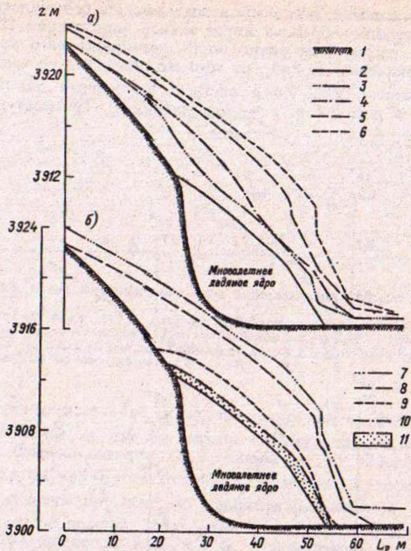
Рис. 7.5. Поперечные разрезы снежника по одному из снегомерных профилей на различные даты в течение периода накопления (а) и периода таяния (б) 1977—1978 гидрологического года.
