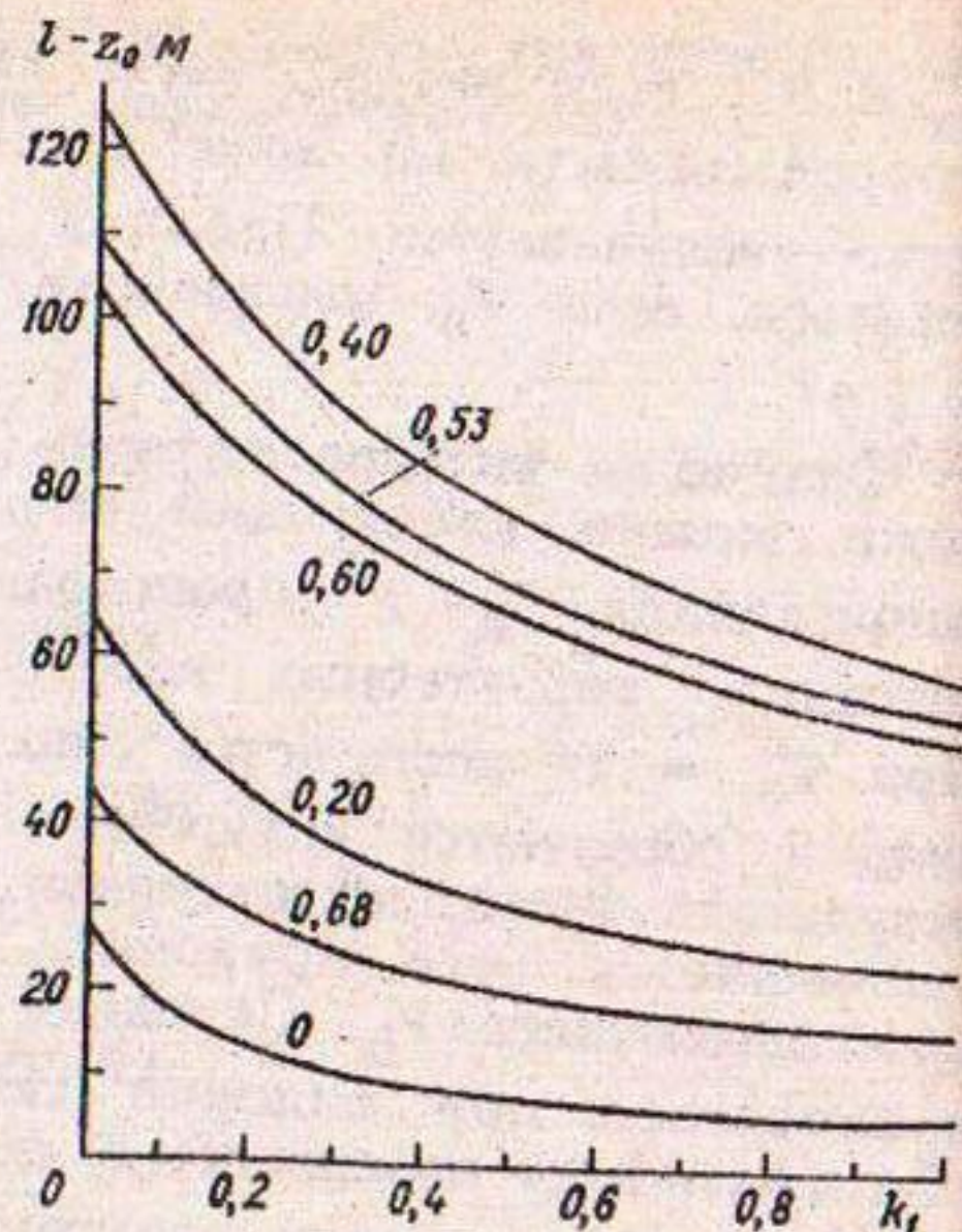
Рис. 5.6. Влияние коэффициента донного скольжения k_1 на толщину ледника ( l - z_0 ).
