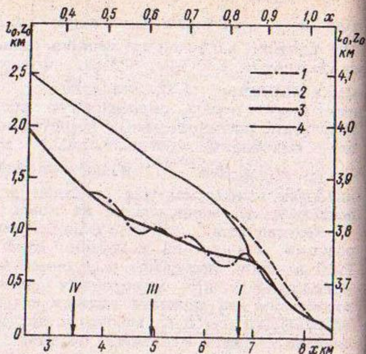
Рис. 5.8. Форма языка ледника Абрамова.
