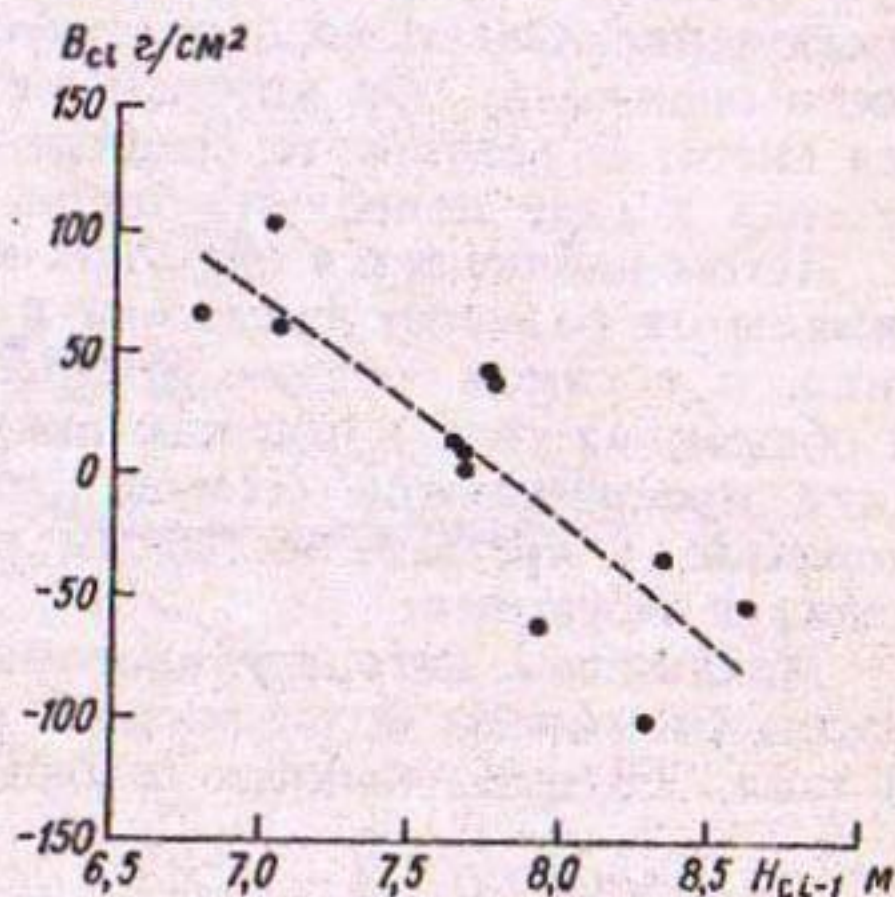
Рис. 7.6. Зависимость удельного годового баланса массы B_{cl} навешанного снежника от его средней мощности к началу гидрологического года H_{cl-1} .
