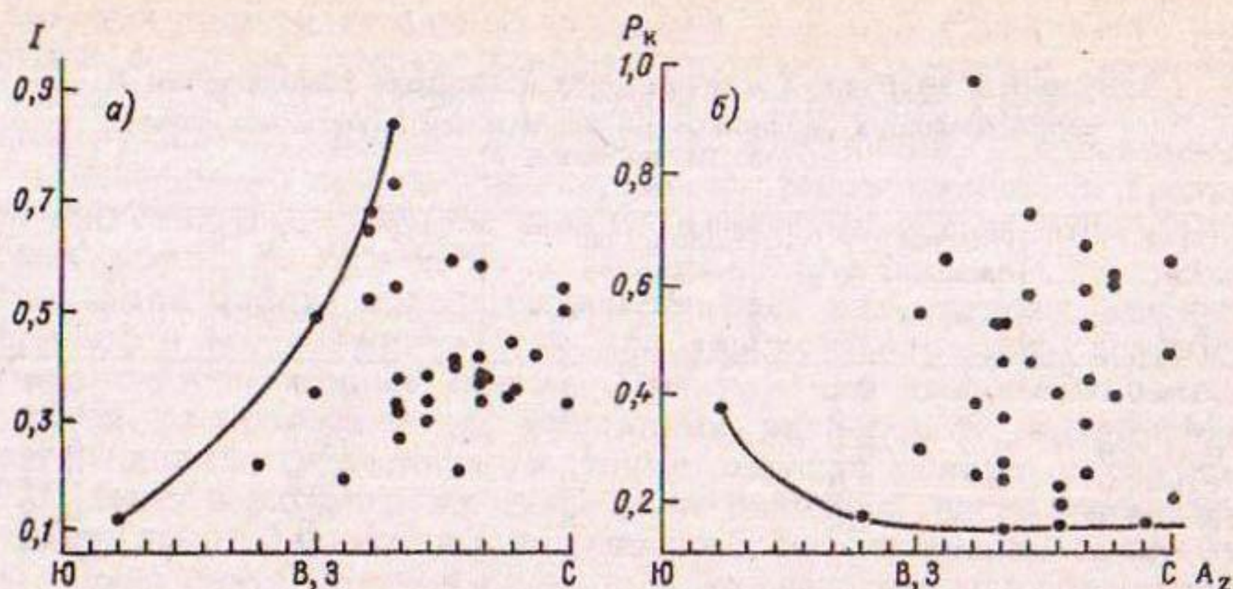
Рис. 7.1. Зависимости уклона I (а) и показателя компактности P_k (б) снежников от экспозиции A_z . Кривыми показаны огибающие.
