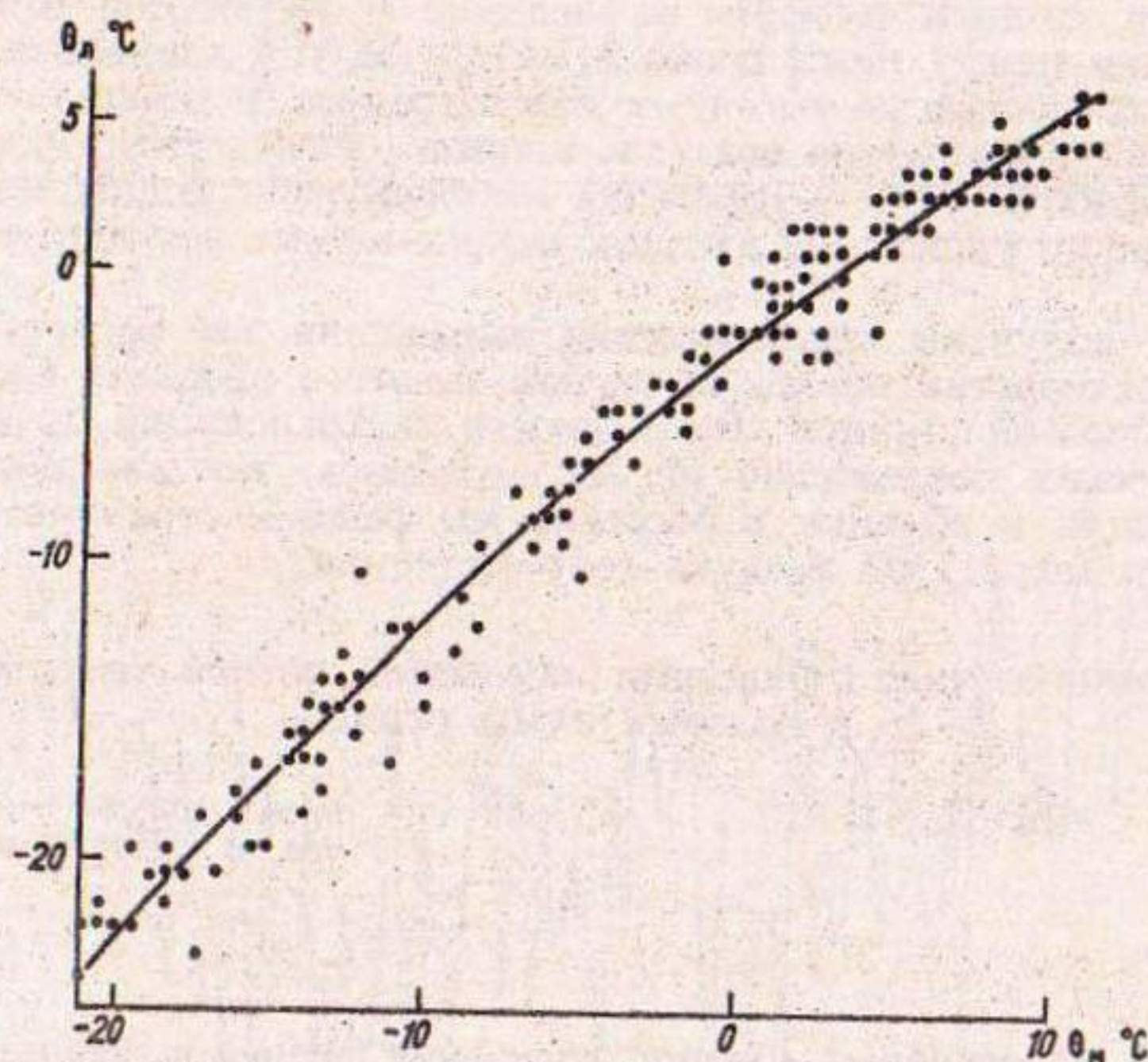
Рис. 2.3. Связь среднесуточных температур воздуха на леднике ( \theta_{\text{л}} ) и на морене ( \theta_{\text{м}} )
