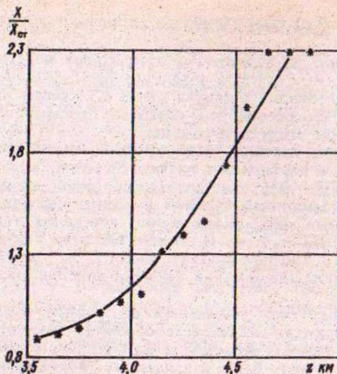
Рис. 2.2. Изменение с высотой z средней многолетней суммы осадков X за теплый период (VI—IX), нормированной по сумме осадков X_{ст} за тот же период на ст. Ледник Абрамова, морена.
