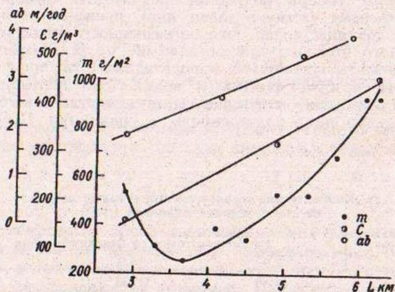
Рис. 6.3. Связь загрязненности поверхности льда m , концентрации твердых частиц C и средней многолетней интенсивности абляции только льда ab с расстоянием точек L от среднего многолетнего положения снеговой границы.
