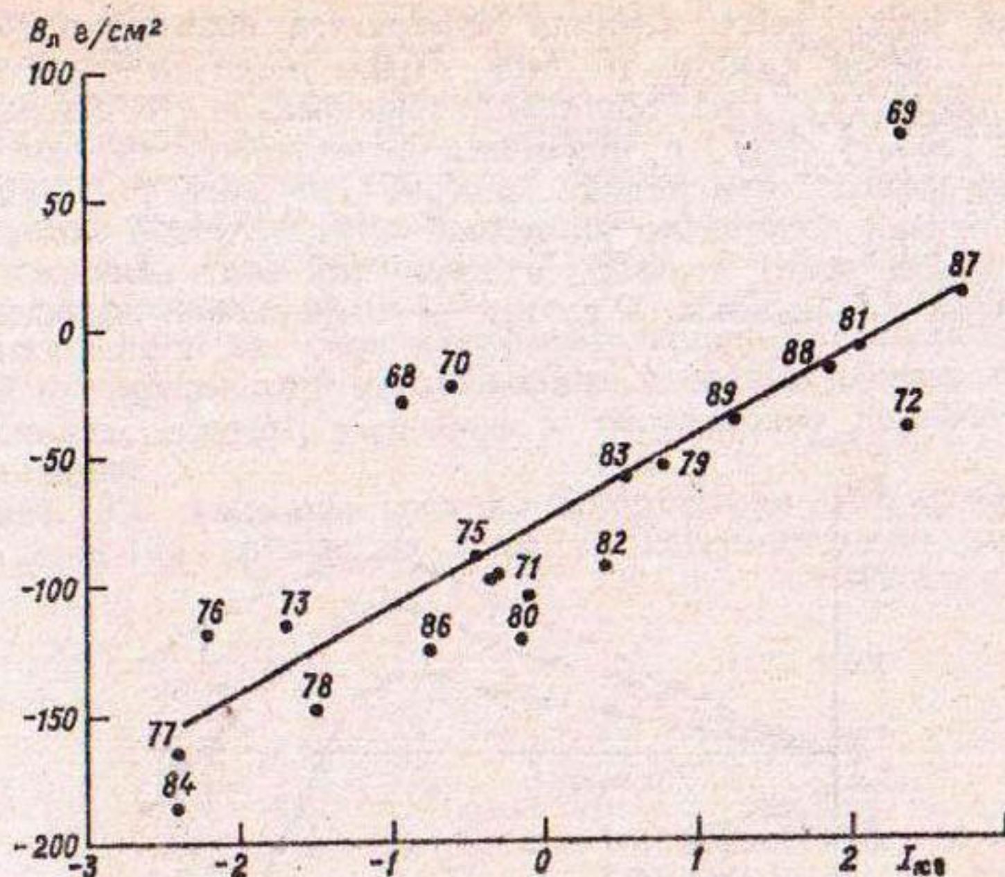
Рис. 3.1. Зависимость годового баланса массы ледника Абрамова B_{\text{л}} от индекса погодных условий I_{x\theta} .
