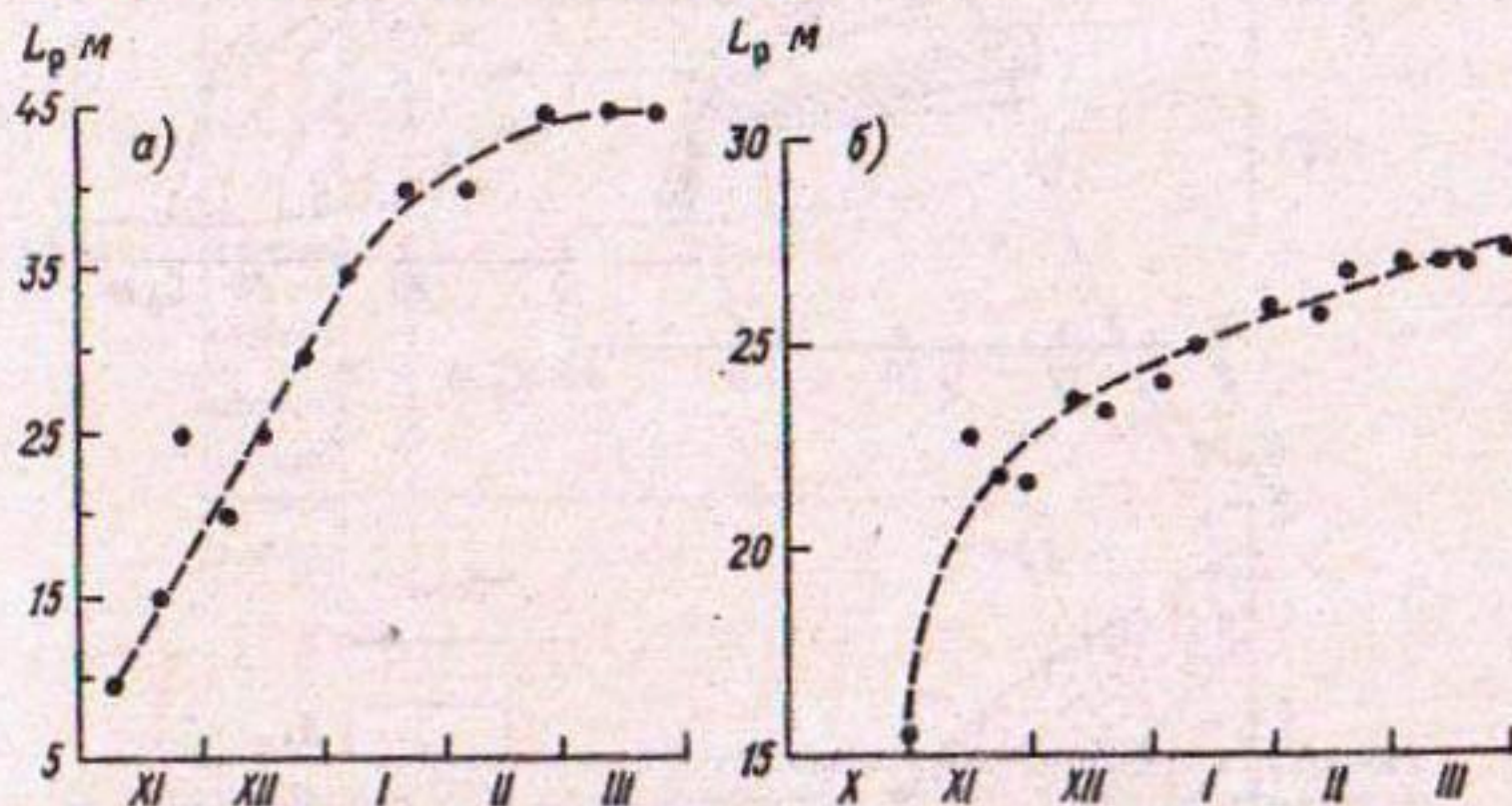
Рис. 7.9. Смещение с течением времени по длине поперечного профиля L_p точки с максимальным накоплением снега (а) и центра тяжести эпюры снега (б).
