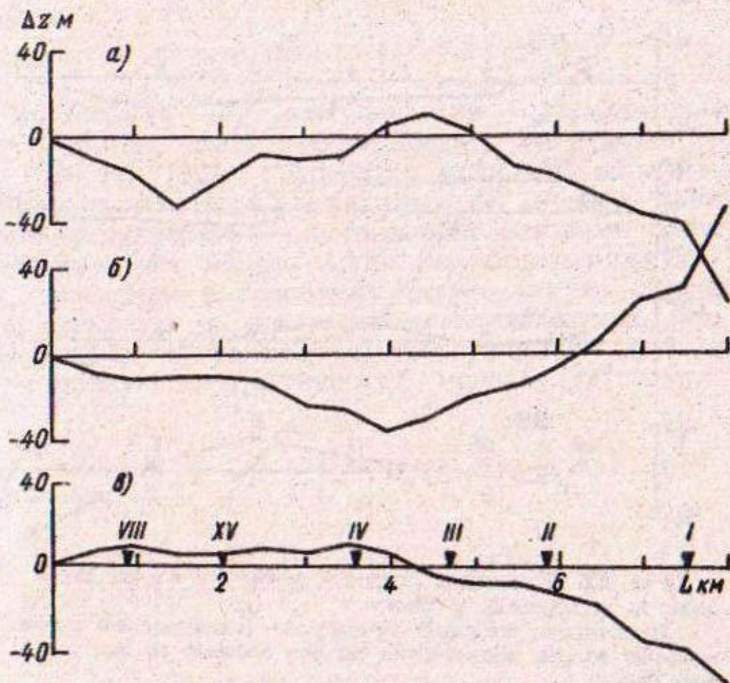
Рис. 5.4. Изменение высоты поверхности ледника \Delta z по его длине L от перевала к языку.
