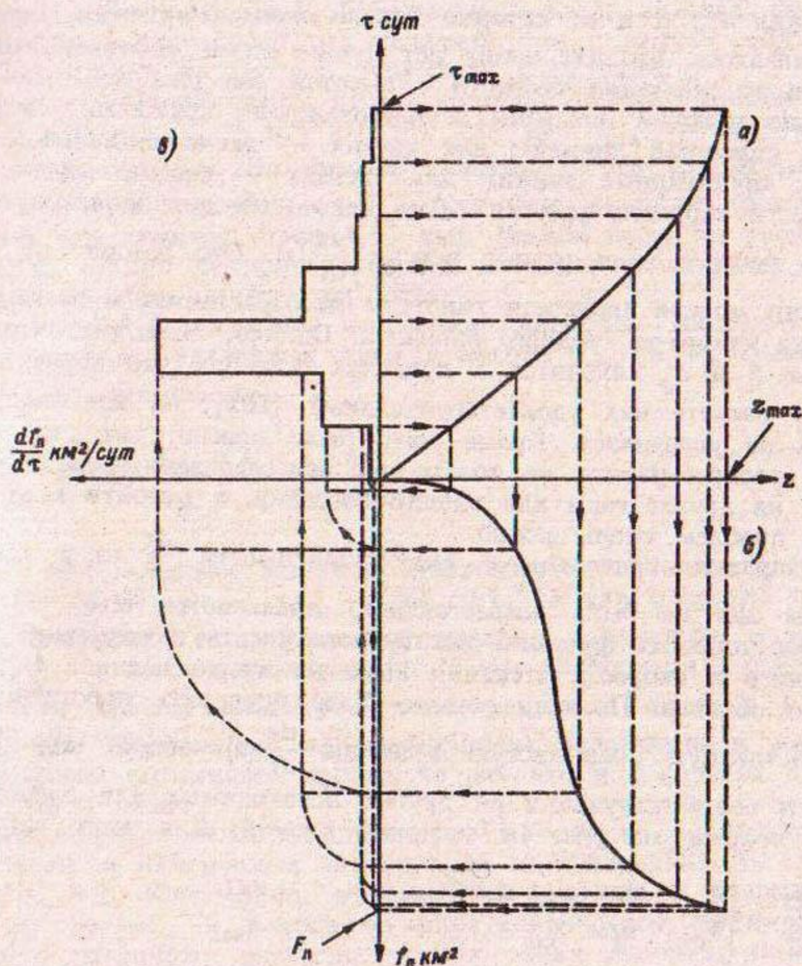
Рис. 4.18. Схема определения кривой добегания.
