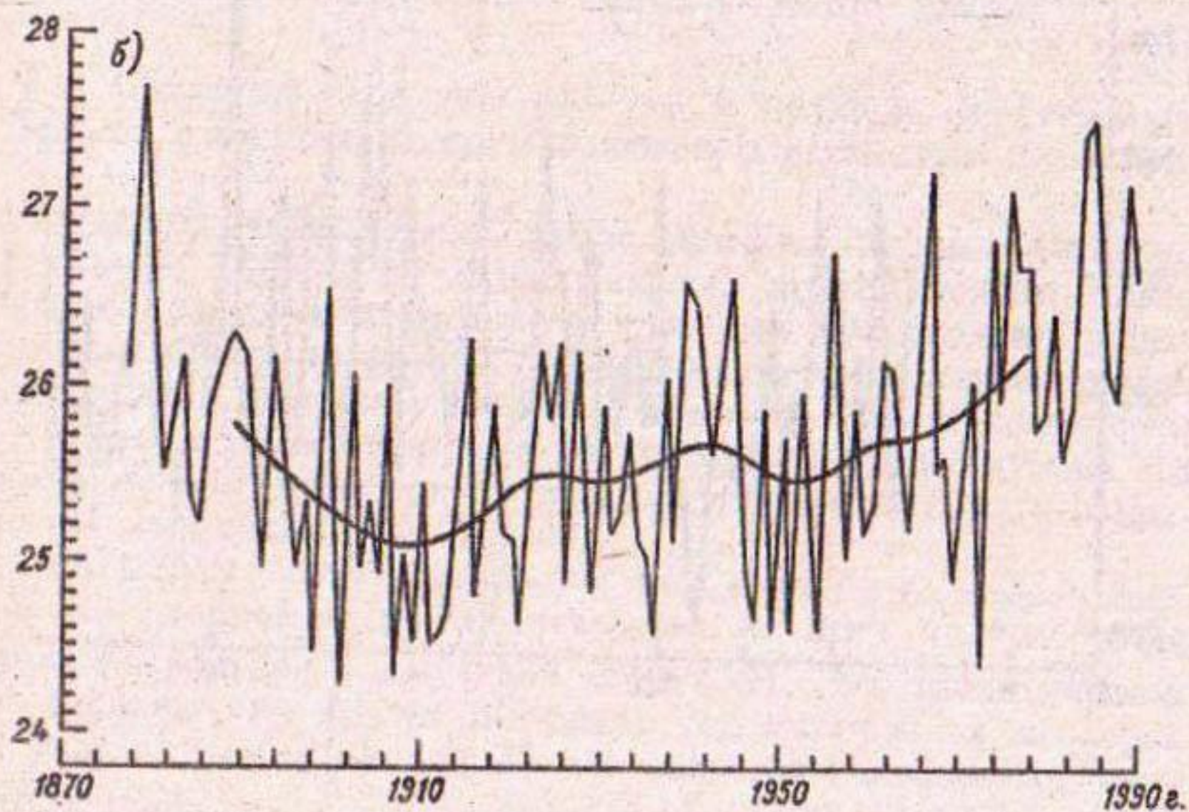
Рис. 2.4. Хронологический ход средней летней температуры воздуха \theta_{\text{л}} в Фергане (а) и Ташкенте (б). 1 — измеренные значения, 2 — сглаженные.
