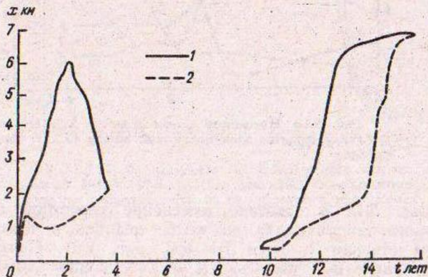
Рис. 5.9. Распространение зон интенсивного скольжения при установившихся автоколебаниях.
