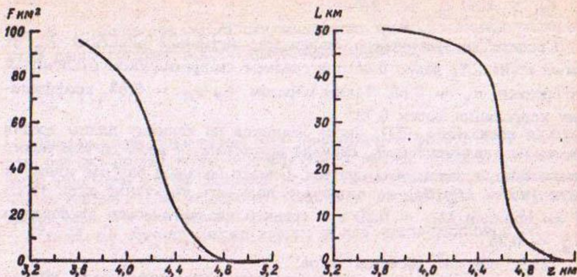
Рис. 8.3. Площадь верхней части бассейна р. Коксу F и длина окаймляющего его гребня L , расположенные выше горизонтали z .
