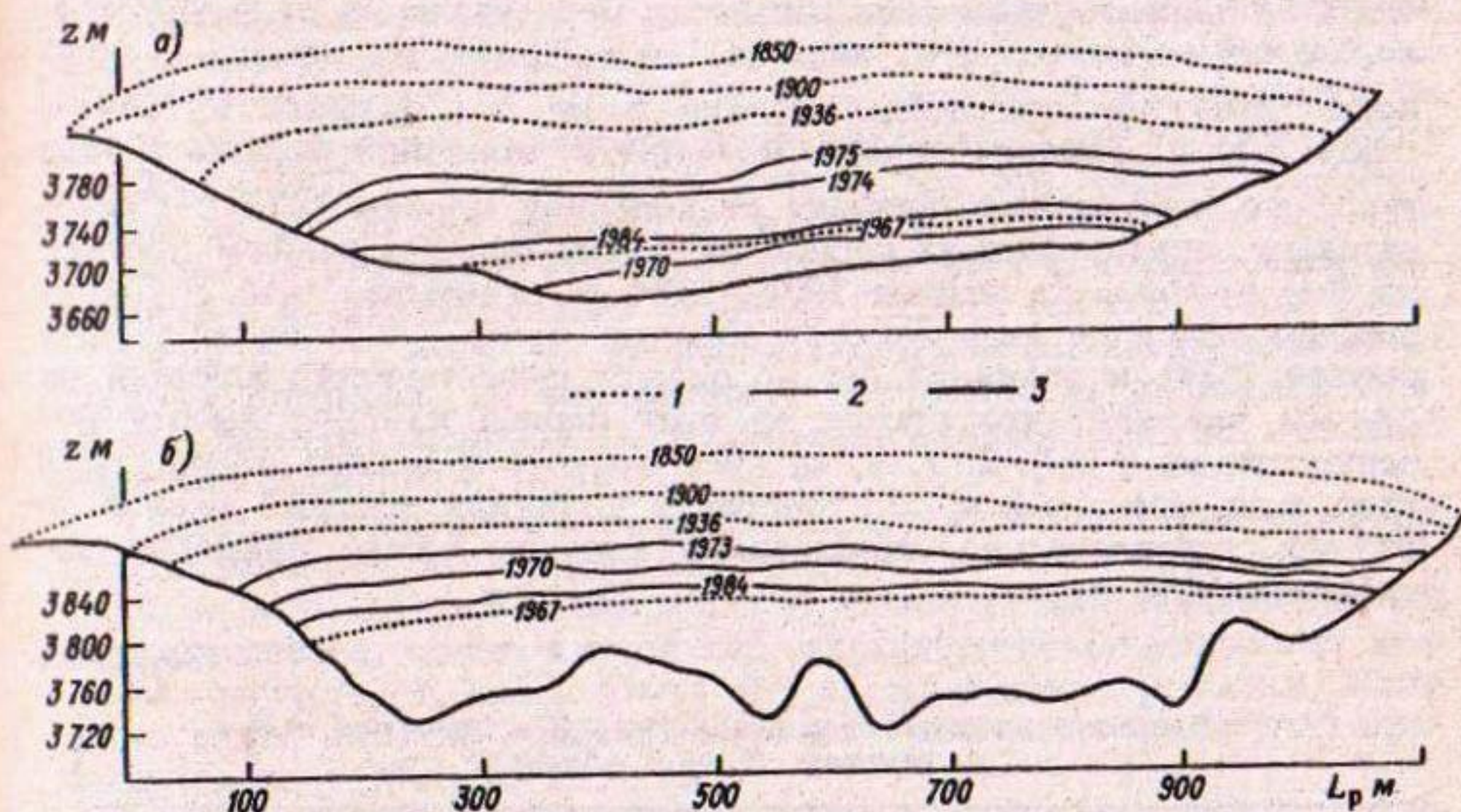
Рис. 8.2. Реконструированные (1) и фактические (2) сечения ледника в различные годы по первому (а) и второму (б) поперечным профилям. z — абсолютная высота, L_p — горизонтальное проложение, 3 — профиль ложа.
