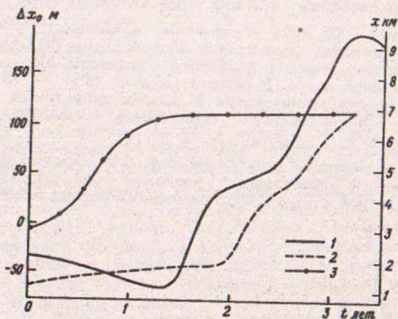
Рис. 5.10. Изменение длины ледника \Delta x_0 (1) и движение фронтов кинематической волны (2, 3) при сдвиге.
