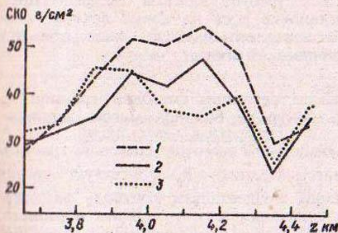
Рис. 3.10. Изменение среднего квадратического отклонения (СКО) годового удельного баланса массы ледника с высотой z . 1, 2 и 3 — в 1985, 1986 и 1987 гг. соответственно.
