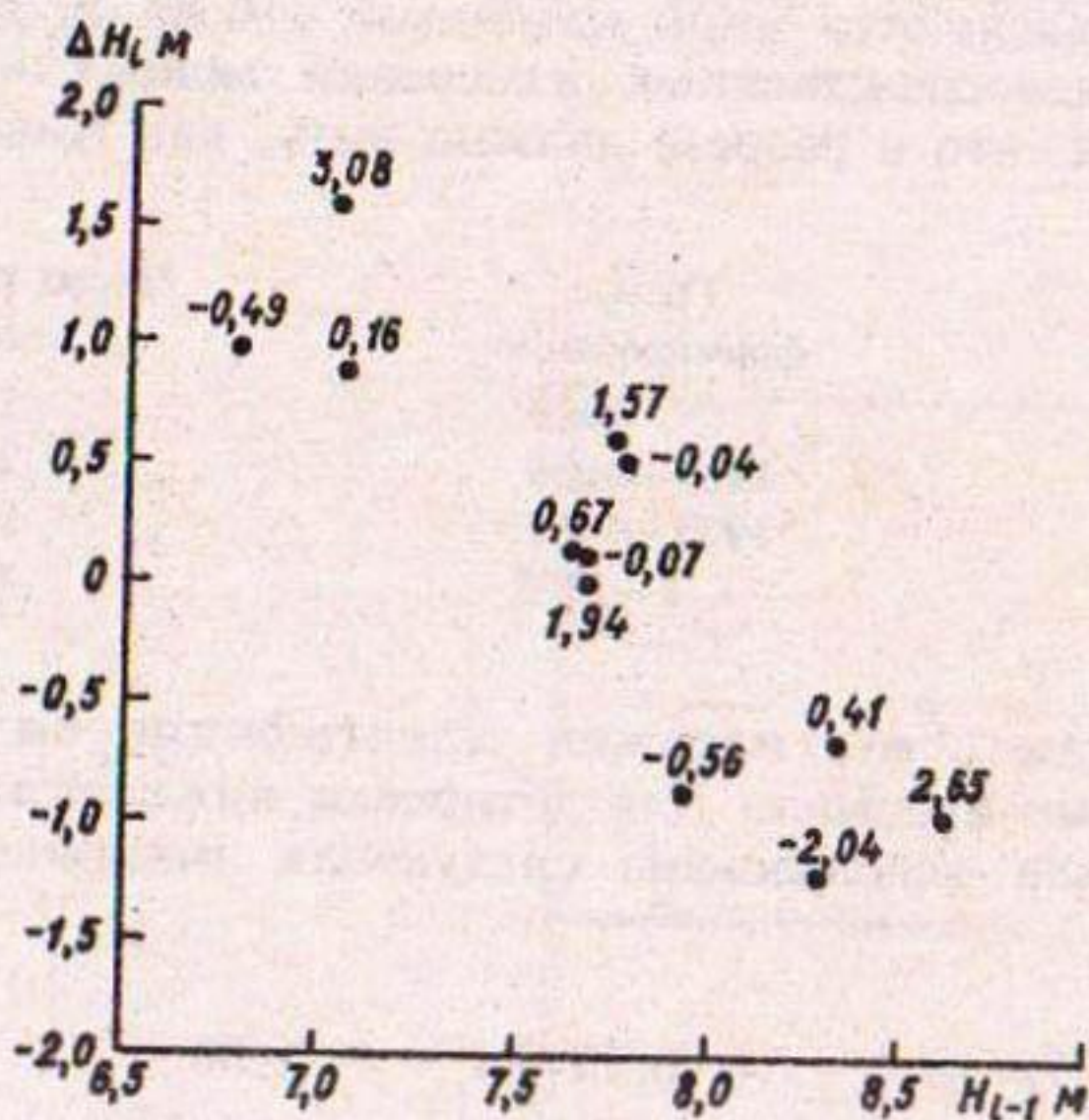
Рис. 7.13. Зависимость годового изменения мощности снежника \Delta H_i от его средней мощности на начало гидрологического года H_{i-1} .
