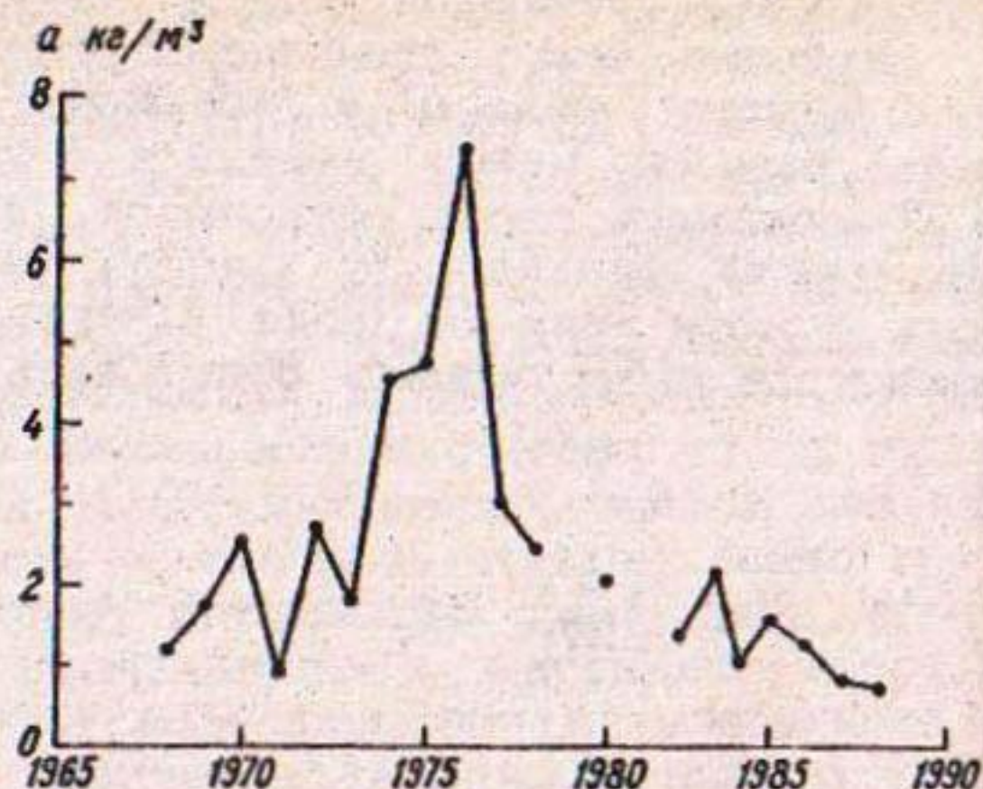
Рис. 4.30. Изменение параметра a в зависимости (4.22) по годам.
