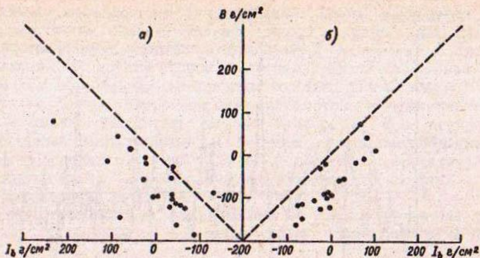
Рис. 3.13. Связь баланса массы ледника Абрамова B с индексом баланса I_b , рассчитанным по данным метеостанций Фергана (а) и Ледник Абрамова (б).
