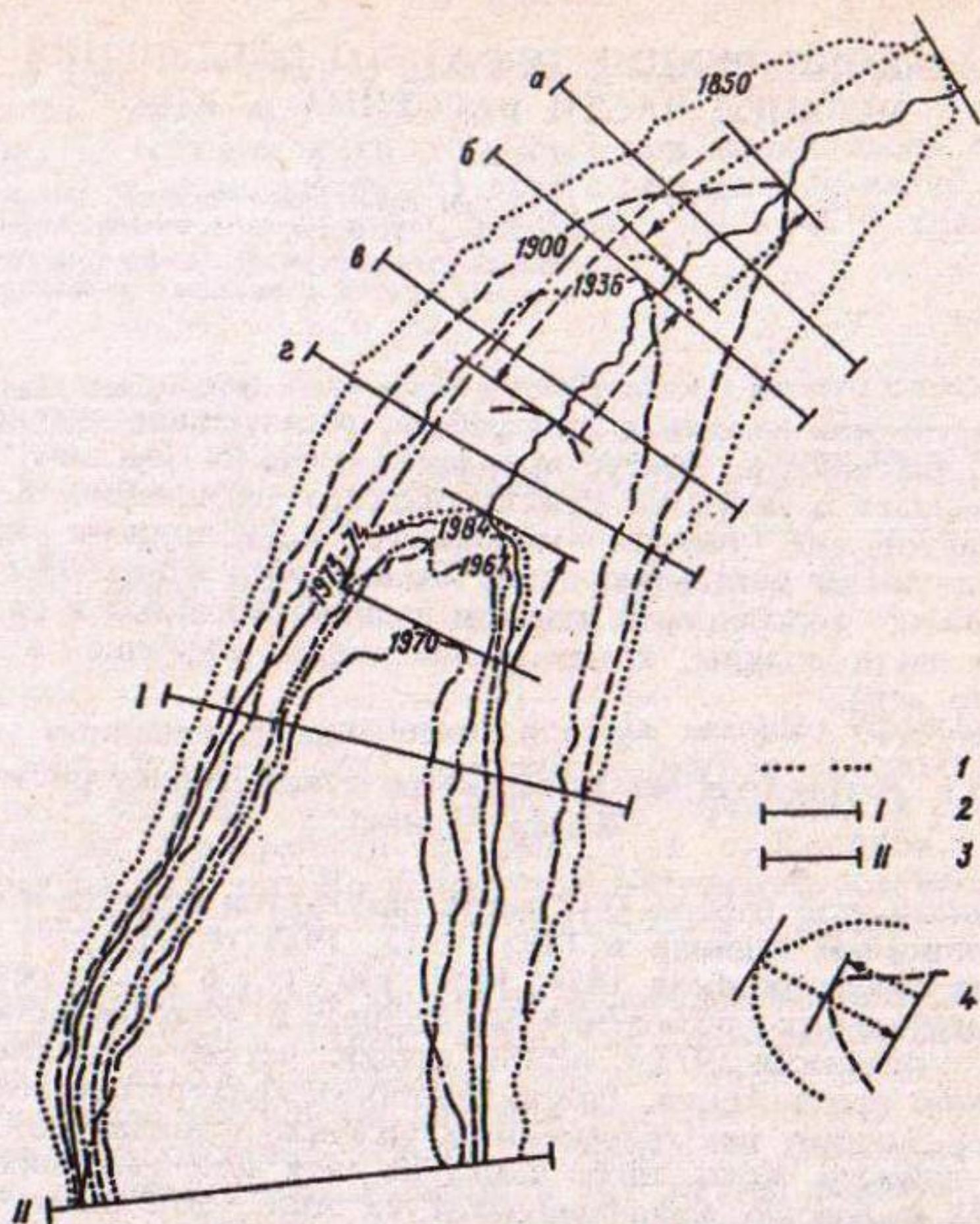
Рис. 8.1. Современные и прежние границы языка ледника. 1 — фактические границы, измеренные инструментально и определенные по аэрофотоснимкам; 2 — поперечный профиль; 3 — профиль, на котором проводится нивелировка; 4 — расчетная и фактическая амплитуда колебаний конца ледника.
