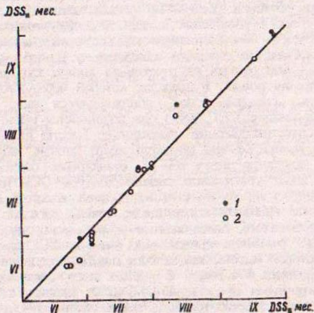
Рис. 4.11. Сравнение дат начала таяния льда в высотных зонах ледника Абрамова в 1985 и 1986 гг., рассчитанных ( DSS_м ) с помощью формулы (4.7) и определенных по высоте снеговой границы ( DSS_г ).
