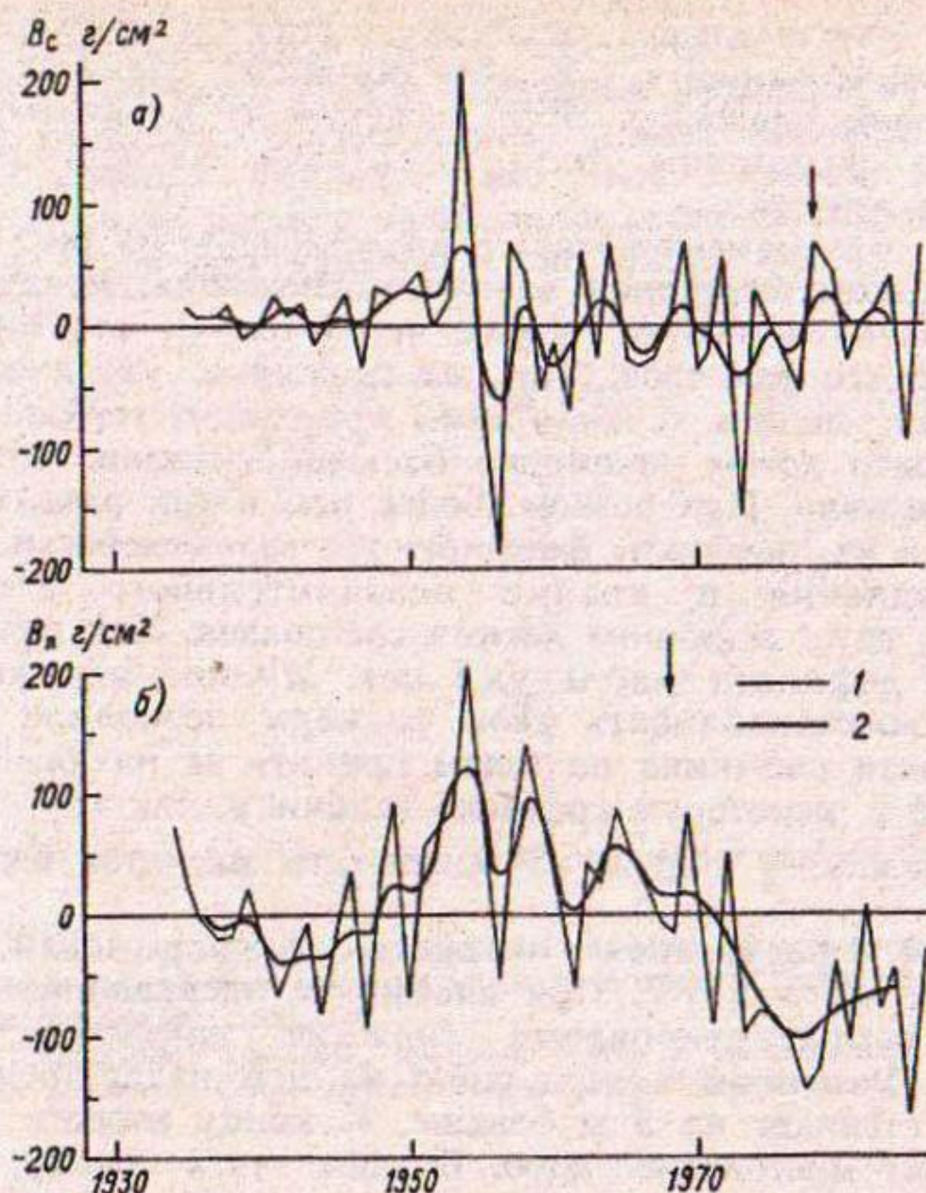
Рис. 7.8. Хронологический ход годового удельного баланса масс навейного снежника B_c (а) и ледника Абрамова B_A (б).
