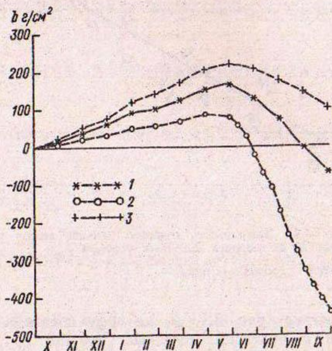
Рис. 3.2. Внутригодовой ход удельного баланса массы ледника b в 1990 г. 1 — весь ледник, 2 и 3 — высотные зоны 3,6—3,7 и 4,4—4,5 км соответственно.
