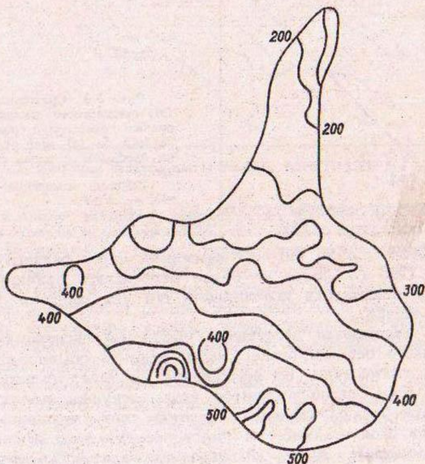
Рис. 3.9. Изолинии максимальной высоты снега (см) на леднике Абрамова в 1979 г.
