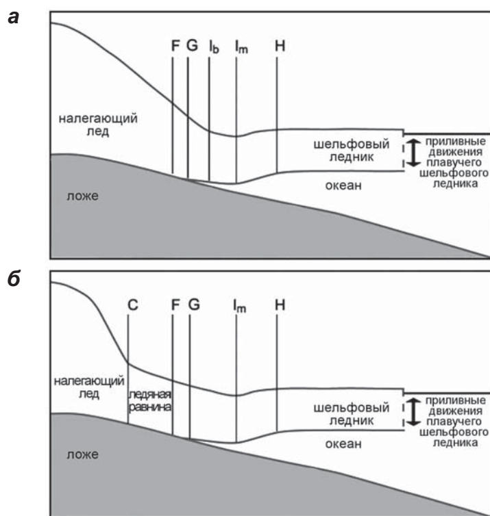
◀ Рис. 2.141. Схематический разрез шельфового ледника, показывающий характерные точки в зоне его налегания при отсутствии (а) и наличии (б) «ледяной равнины». Дальнейшие объяснения см. в тексте (Brunt et al., 2010)
