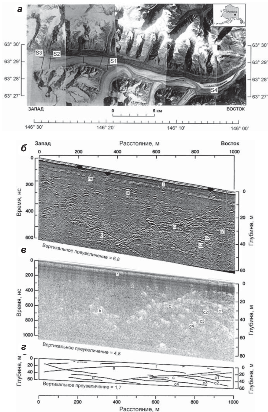
▲ Рис. 2.57. Профили радиозондирования на теплом леднике Блек-Репидз на Аляске на частоте 100 МГц (а); внутриледниковые каналы по данным аэрорадиозондирования на частотах 1,4 ГГц (б) и 100 МГц (в), г – отражение от поверхности, м – переотражение между поверхностью и вертолетом, а, б, с – протяженные внутренние горизонты, с1–с4 – отдельные горизонты вблизи поверхности; г) глубинный разрез по данным измерений на частоте 1,4 ГГц (Arcone, Yankielum, 2000)
