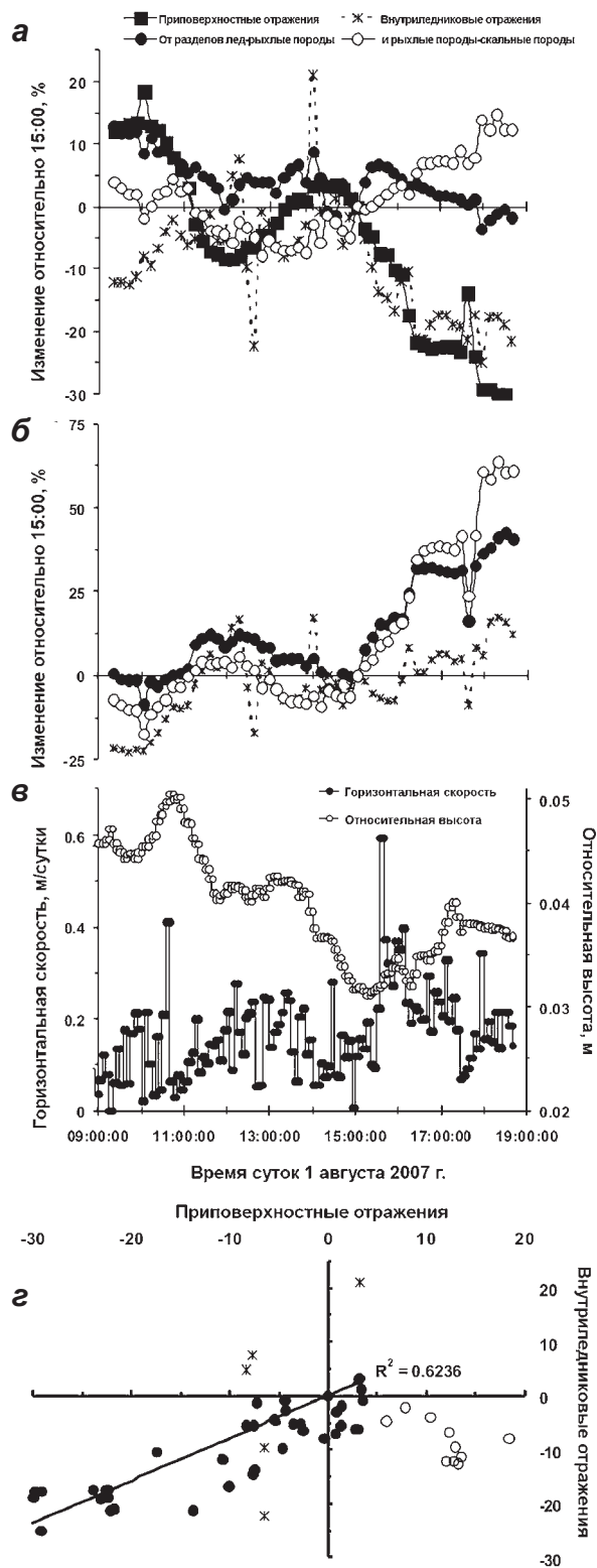
◀ Рис. 4.7. Изменение амплитуды отражений на леднике Грубен в Альпах: а) из поверхностной толщи (во временном окне 160 нс), от внутрiledниковых и подледниковых отражателей; б) то же, но нормированное по амплитудам сигналов из поверхностной толщи; в) изменения горизонтальной скорости и относительной высоты поверхности ледника; г) связь относительных изменений во времени амплитуд сигналов от внутрiledниковых отражателей по отношению к 15:00. Черные и белые кружки обозначают время после и до 11:00, звездочки показывают время начала ускорения движения ледника. Сплошная линия обозначает линейную регрессию для данных после 11:00 (черные кружки) (Kullessa et al., 2008)
