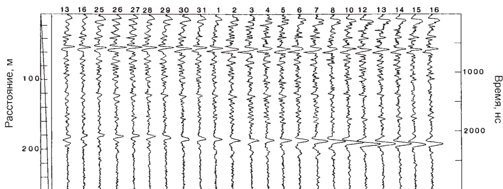
▲ Рис. 2.56. Изменение амплитуды и фазы отраженных сигналов от внутриледниковых скоплений воды на дальностях около 700, 1400 и 2200 нс при зондировании ледника Вариегейтед на Аляске в период с 13 мая по 16 июня 1983 г. на частоте 8 МГц (Jacobel, Anderson, 1987)
