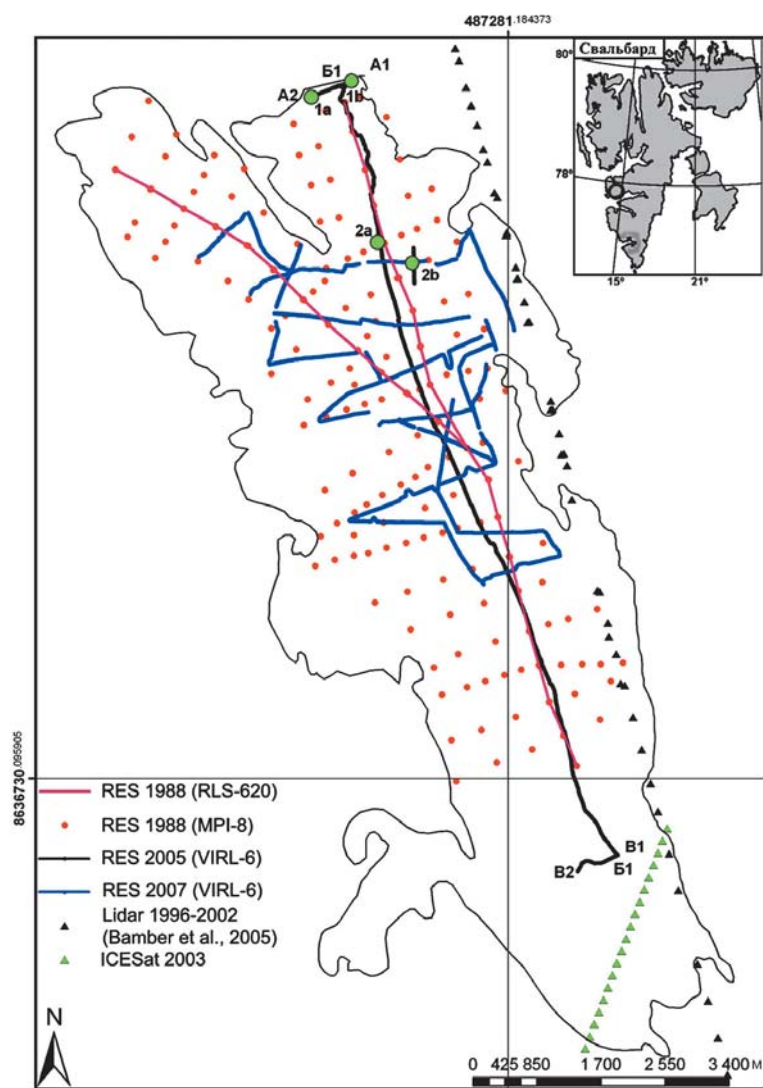
▲ Рис. 3.12. Радиолокационные и радиофизические исследования на леднике Фритьоф до (1977–1988 гг.) и после (2005 г.) его подвижки в 1990-х годах (Василенко и др., 2006)
