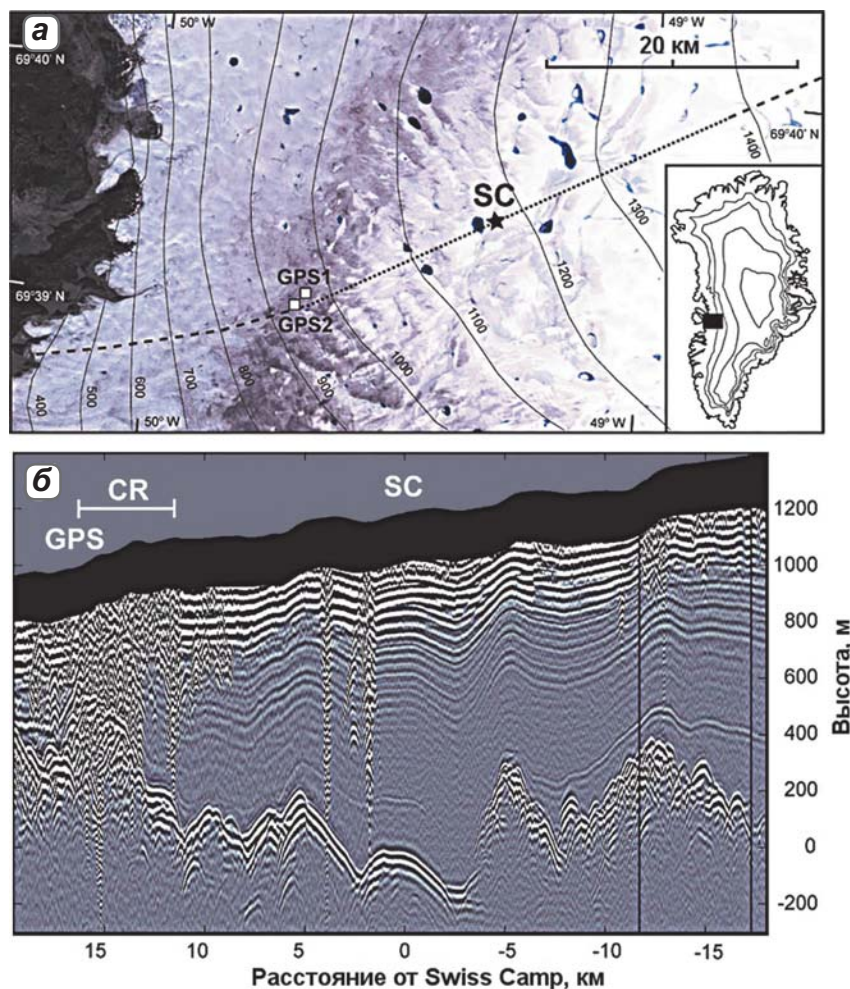
▲ Рис. 2.27. Радарный профиль и линия тока через станцию Swiss Camp (SC) (обозначены пунктирной и штриховой линиями), проходящие через зону сильной трещиноватости (а); радарная запись на частоте 2 МГц (б); на расстоянии около 1 км ниже зоны трещин SC предполагается существование вертикального канала, соединенного с подледниковой дренажной системой (Price et al., 2008)
