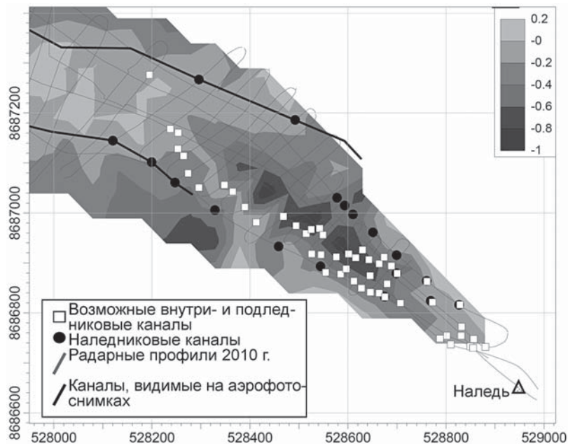
▲ Рис. 2.75. Относительный коэффициент r отражения от ложа ледника Телл на Шпицбергене по данным радиозондирования 2010 г. с применением моноимпульсного лоатора с центральной частотой 50 МГц. В областях с r < -0,5 предполагается присутствие воды на границе лед–подстилающие породы (Bælum, Benn, 2010)
