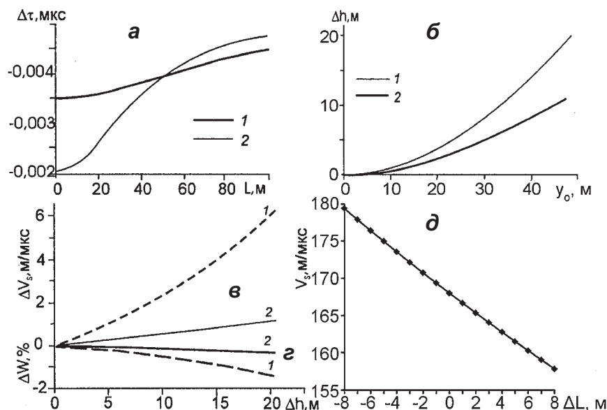
▲ Рис. 2.48. Ошибки определения параметров ледника по гиперболическим отражениям: а) разнице в двукратном времени распространения \Delta\tau отраженной волны от точечного отражателя, находящегося на глубине h = 50 м (1) и 100 м (2) во льду для одно- и двухпозиционного зондирования (с совмещенными и разнесенными на 10 м антеннами); б) ошибки \Delta h определения глубины h точечного отражателя по линейным годографам Y = f(X) отраженной волны от точечного отражателя во льду как функция расстояния y_0 между проекцией отражателя на поверхность ледника и профилем измерений при глубине отражателя h = 50 м (1) и h = 100 м (2); в, г) ошибки определения скорости радиоволн \Delta V_s (в) и содержания воды \Delta W (г) в теплом льду политермического ледника, которые возникают, если не учитывать удаление y_0 точечного отражателя от профиля радиолокационных измерений, для следующих параметров ледника (см рис. 2.14): h_d = 50 м, V_d = 170 м/мкс, h = 100 м, V = 164,8 м (1); h_d = 100 м, V_d = 170 м/мкс, h = 200 м, V = 164,8 м/мкс (2); д) ошибки в оценке скорости радиоволн V из-за неточного определения смещения \Delta L отражателя вдоль профиля радиозондирования. При расчетах принято, что точечный отражатель расположен на глубине h = 50 м непосредственно под профилем измерений, V = 168 м/мкс (Мачерет, 2000)
