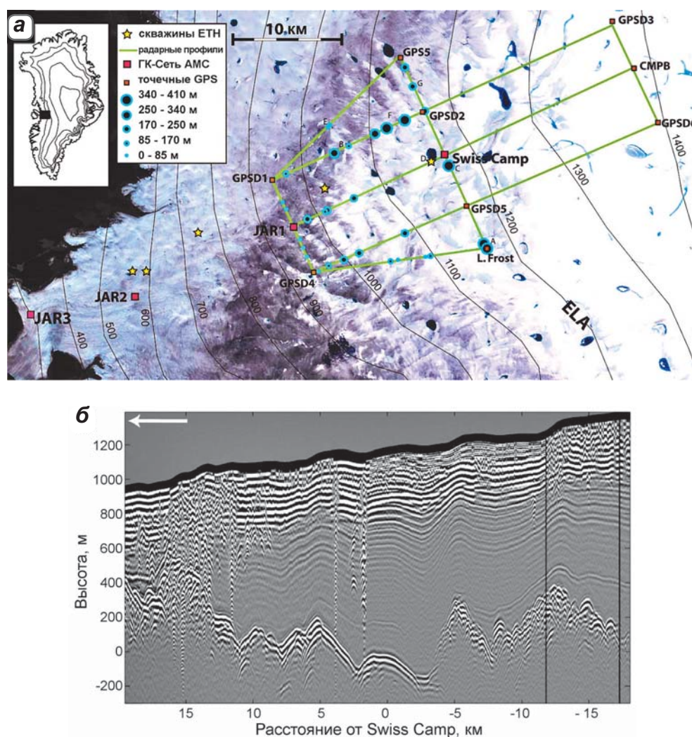
▲ Рис. 2.66. Наземные радиолокационные измерения весной 2006 г. (зеленые линии) на частоте 1 МГц в районе станции Swiss Camp на западе Гренландии (а); изогипсы (черные линии) проведены по данным (Bamber et al., 2001), расстояние от профиля до колодцев показано кружками разных размеров, красными квадратами – метеостанции, звездочками – скважины; радарный профиль через станцию Swiss Camp ( x = 0 ) от JAR1 (слева) до CMPB (справа) (б) (Catania et al., 2008)
