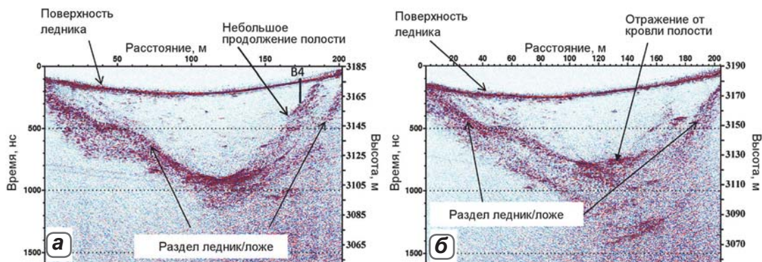
▲ Рис. 2.72. Данные радиозондирования на частоте 100 МГц, показывающие отражения от поверхности и ложа ледника Tête Rousse на профиле 10 (а), а также от свода подледниковой полости на профиле 9 (б). Положение профилей показано на рис. 2.71, а (Vincent et al., 2012)
