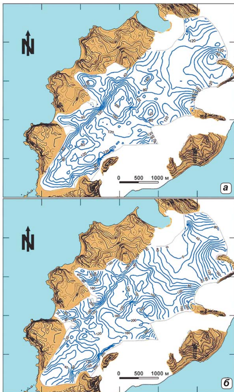
▲ Рис. 3.33. Толщина льда (а) и подледный рельеф (б) ледников Джонсонс и Хард по данным радиозондирования 1999–2003 гг. (Navarro et al., 2009)
