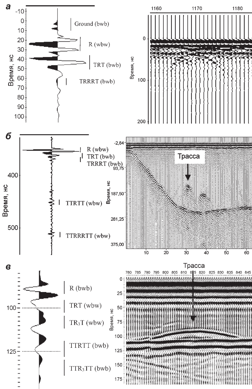
▲ Рис. 2.63. Отражения от внутриледниковых и подледниковых каналов на леднике Телл по данным радиозондирования на частоте 100 МГц: канал на глубине 2–4 м, заполненный снегом (а); внутриледниковый канал диаметром 2,3 м, на 2/3 заполненный водой (б); подледниковый канал высотой около 2 м с 0,5 м воды вблизи языка ледника (в). Кривизна гиперболы для случая (а) соответствует скорости радиоволн 22 нс/м, характерной для снега. Обозначения отражений от верхней и нижней стенок каналов те же, что и на рис. 2.59 и 2.61 (Bælum, Benn, 2010)
