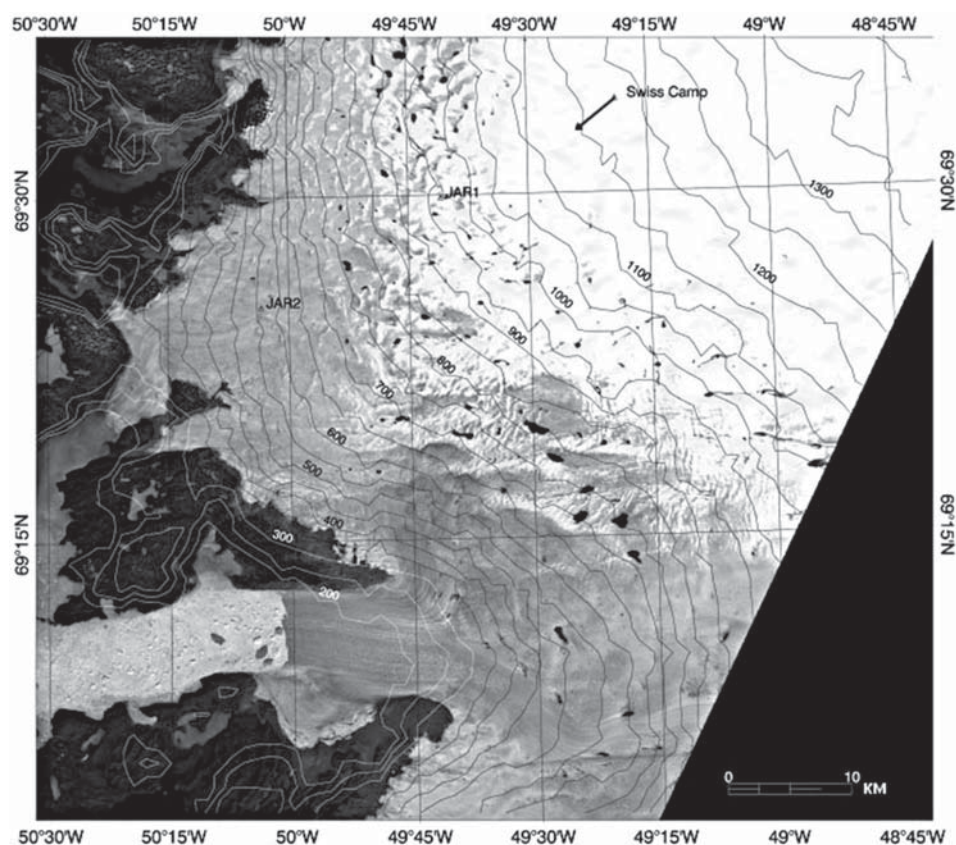
▲ Рис. 2.1. Изображение Landsat TM (канал 3, 0,63–0,69 мкм, разрешение 30 м) западной части Гренландского ледникового покрова в районе станции Swiss Camp, полученное в безоблачных условиях 22 июня 1990 г. Более темный участок соответствует области поверхностного таяния, темные пятна – наледниковым озерам, темные линии – втекающим в них потокам талой воды (Zwally et al., 2002)
