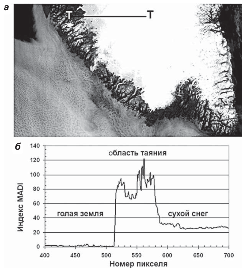
▲ Рис. 2.6. Изображение MODIS юга Гренландии 17 июня 2003 г (а) и индекс MADI вдоль профиля T-T (б) (Chilek et al., 2007)
