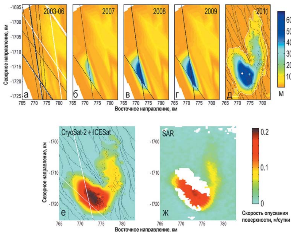
▲ Рис. 4.105. Изменение высоты ледниковой поверхности (цветная шкала, м) над подледниковым озером Кука по измерениям ICESat (а–г) и CryoSat-2 (д). Черными линиями показаны треки лазерной альтиметрии, белыми линиями на (а) – треки ICESat 2003 г., белым пунктиром на (д) показаны границы депрессии; скорости изменений по данным (е) ICESat и CryoSat-2, (ж) SAR (McMillan et al., 2013)
