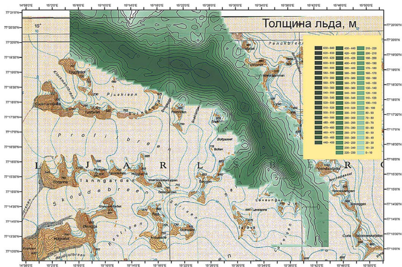
▲ Рис. 3.26. Строение ледникового плато Амундсена по данным наземного радиозондирования и DGPS-измерений 2004–2006 гг.: в) толщина льда (Гловацкий и др., 2008)
