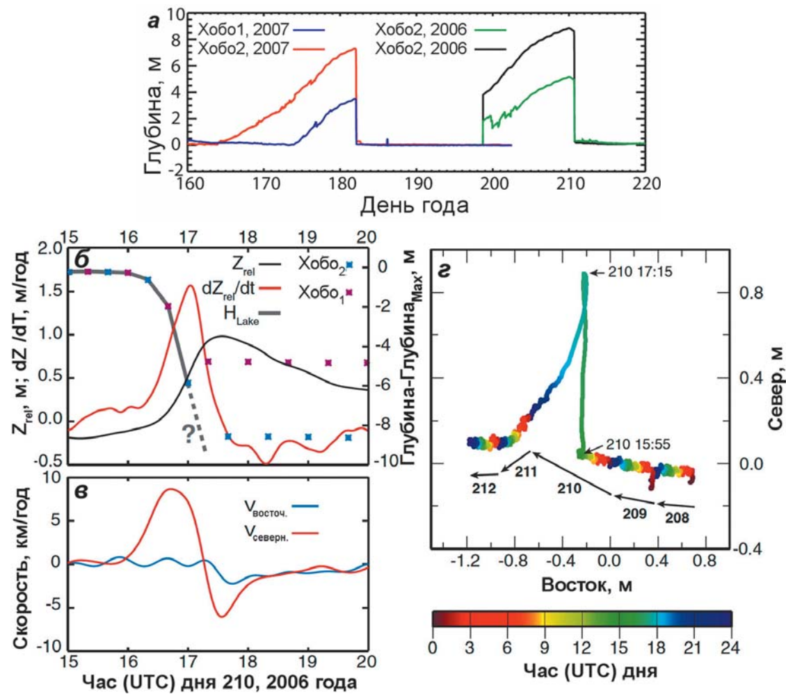
◀ Рис. 2.24. Изменение уровня озера (а) в 2006 г. (зеленая линия) и 2007 г. (красная линия); опорожнение озера в 2006 г.: (б) относительная скорость изменения высоты поверхности ледника Z_{rel} , м/ч, в двух точках на берегу озера по данным GPS измерений (голубые и фиолетовые звездочки) и глубина озера H_{Lake} , м (пунктиром показана экстраполяция); северная и восточная компоненты скорости движения льда (в) (красная и синяя линии) по данным GPS измерений; смещение GPS станции в течение 5 дней (г) (до, во время и после опорожнения озера); цветными точками показаны смещения за час, черными стрелками – суммарные смещения (Das et al., 2008)
