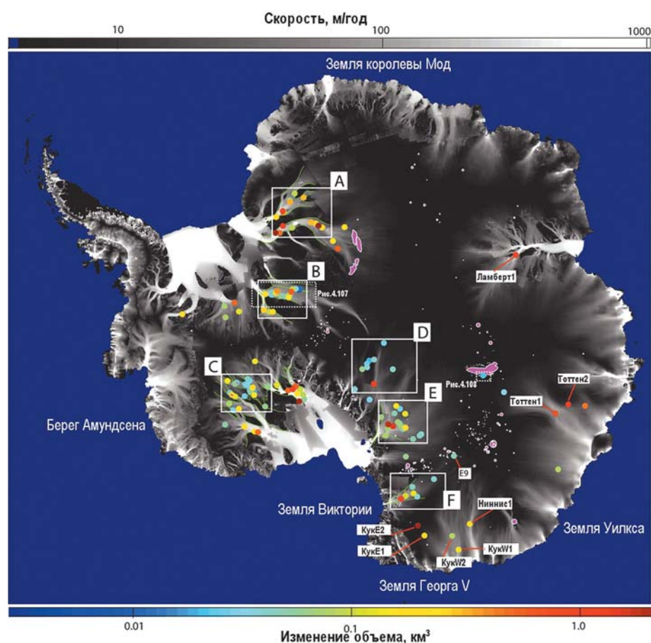
▲ Рис. 4.112. Положение 124 активных подледниковых озер в Антарктиде по данным съемок со спутника ICESat в 2003–2008 гг. Белым и фиолетовым цветом указаны ранее известные подледниковые озера; кружками – подледниковые озера, идентифицированные по данным радиолокации, их диаметр пропорционален длине озер (Siegert et al., 2005; Carter et al., 2007; Popov, Masolov, 2007). Белыми прямоугольниками отмечены места, показанные на рис. 4.113 (Smith et al., 2009)
