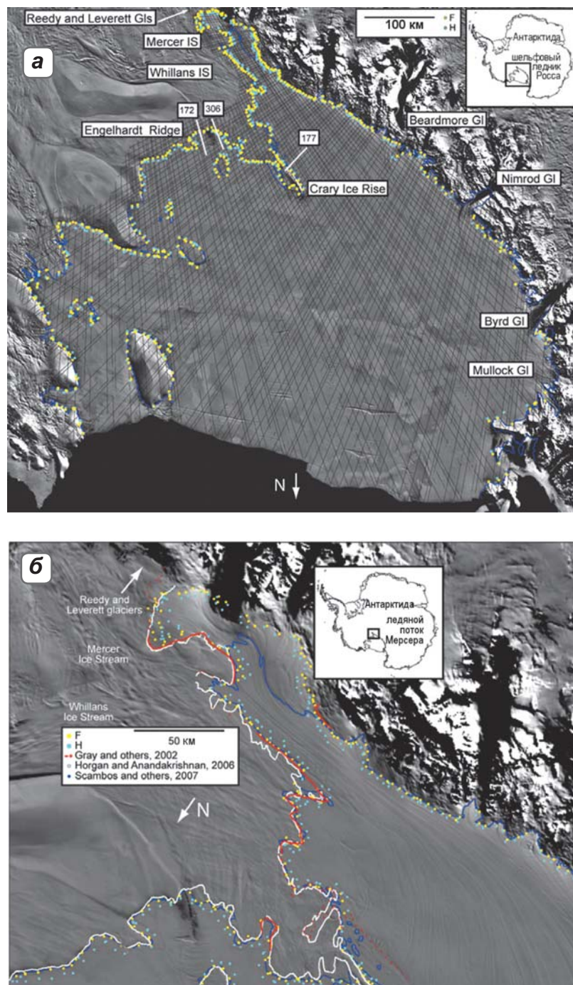
▲ Рис. 2.143. Положение линии налегания всего шельфового ледника Росса (а) и его южной части (б). Ее положение оценено по точкам F (желтые точки), H (голубые точки), по данным ICESat 2003 г. (черные линии) и точкам I_b (синие линии по данным MOA (Scambos et al., 2007). Дополнительно на (б) показано положение линии налегания по данным (Horgan, Anandakrishnan, 2006) (белая линия) и по данным (Gray et al., 2002) (красная линия) (Brunt et al., 2010)
