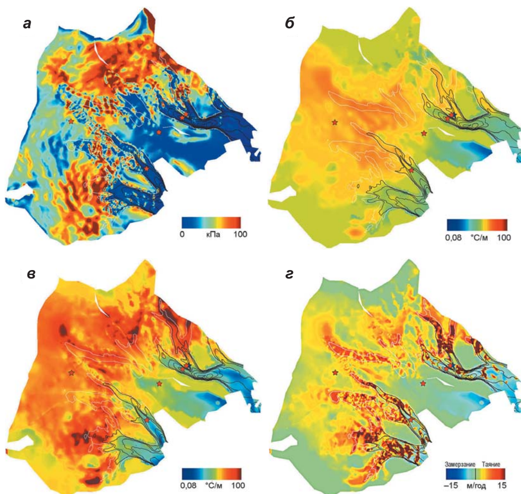
▲ Рис. 4.55. Условия на ложе ледяных потоков Росса по данным численного моделирования: напряжение сдвига на ложе (а), градиент температуры льда у ложа без учета (б) и с учетом (в) горизонтальной адвекции; скорость донного таяния–намерзания (г) (Joughin et al., 2004)
