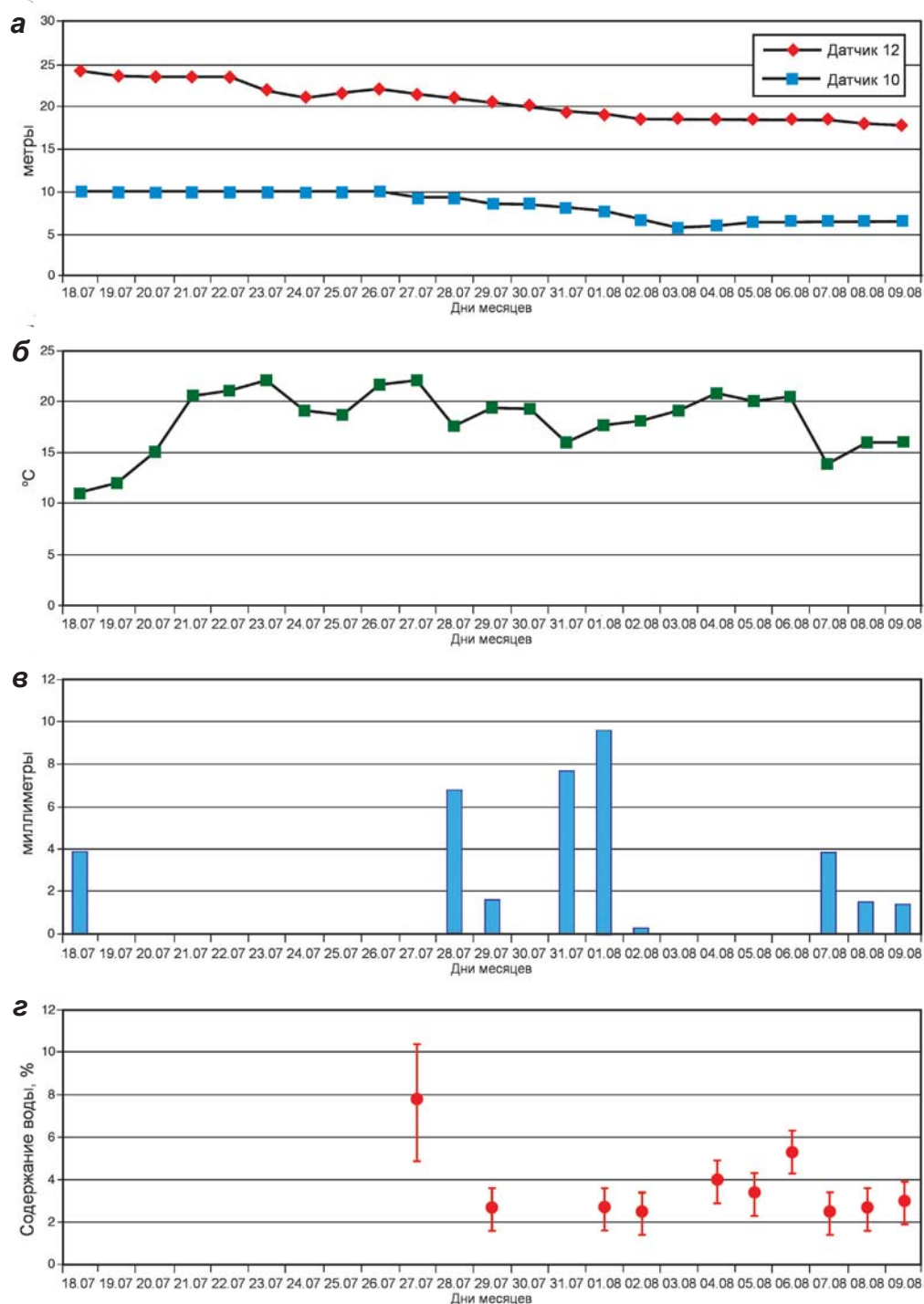
▲ Рис. 4.9. Давление воды (в метрах водного эквивалента) по данным измерений датчиками 10 и 12 (а); средняя суточная температура (б); средние суточные осадки (в); содержание воды во льду (г) (см. табл. 4.2) (Hart et al., 2011)
