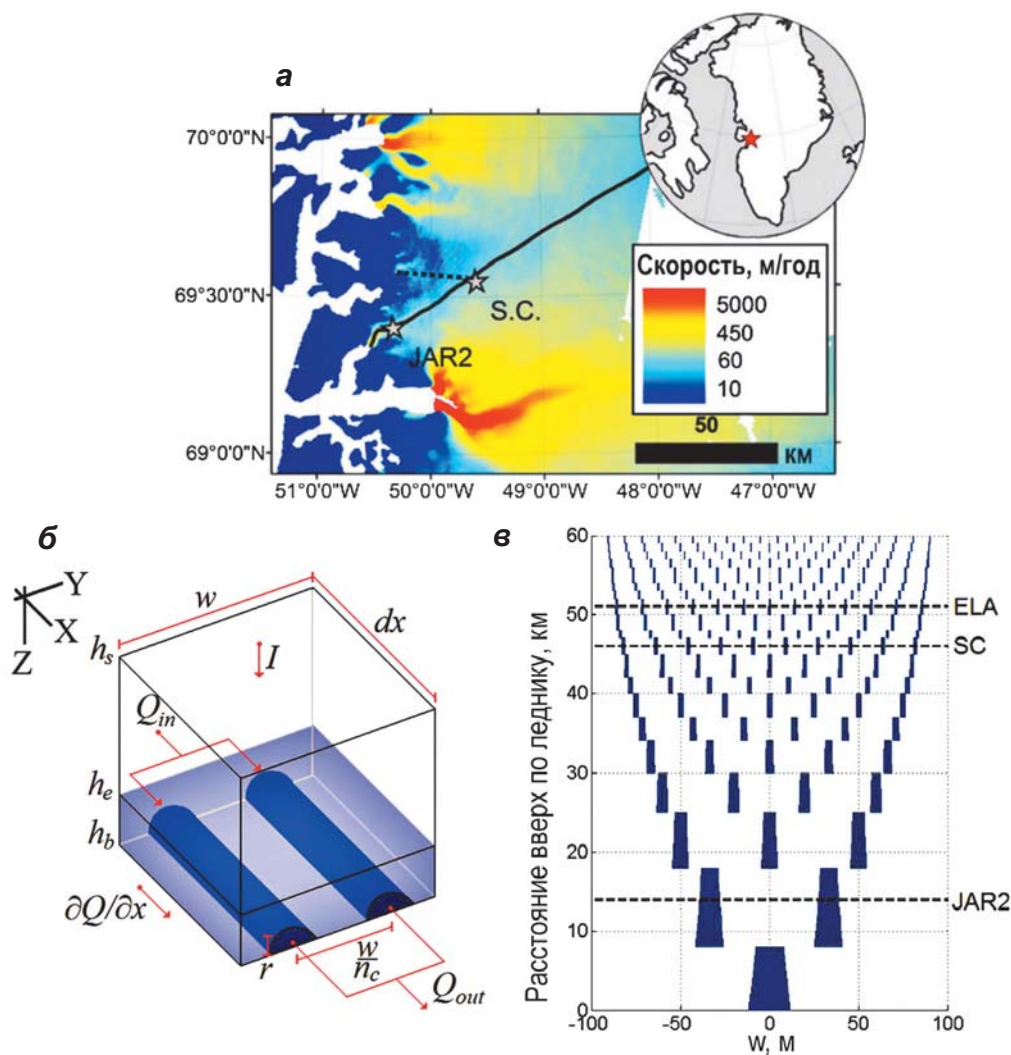
▲ Рис. 4.68. Расчетная линия тока на леднике Сермек Аваннарлек, проходящая через станции JAR2 и Swiss (обозначены звездочками) (а); пунктирная линия показывает кратчайший путь от станции Swiss Camp до края ледникового покрова; схематическая модель гидравлического напора h_e (уровня вод) в разветвленной сети каналов при поступлении Q_{in} со скоростью I , стоке Q_{out} и расходе Q воды в подледниковых каналах радиусом r , расположенных на ложе на высоте h_b на расстоянии w друг от друга (б); схема древовидной гидрологической сети (в): количество каналов и максимальный диаметр канала (с 5-кратным увеличением) в зависимости от гидрологической длины a вдоль линии тока, когда a = 20 км. Горизонтальные пунктирные линии обозначают положение станций JAR2 и Swiss Camp и положение границы питания (Colgan et al., 2011)
