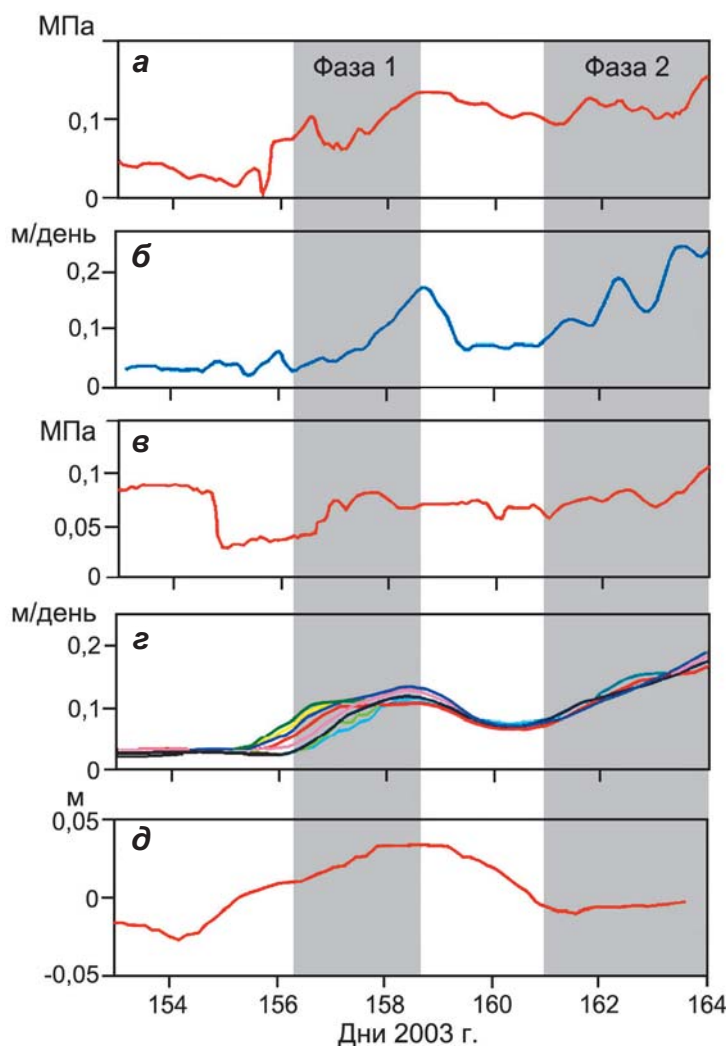
▲ Рис. 1.11. Поверхностная скорость и эффективное давление на ложе ледника Бенч по данным измерений 2003 г.: а) локальное эффективное давление, осредненное по 17 скважинам на площади 60 \times 100 м; б) поверхностная скорость; в) среднее эффективное давление по 29 скважинам на площади 500 \times 300 м; г) региональная скорость по 29 скважинам; д) отделение ложа на единицу площади, вычисленное по формуле (1.17) для района детальных исследований. Серым выделены две фазы усиления скольжения (Harper et al., 2007)
