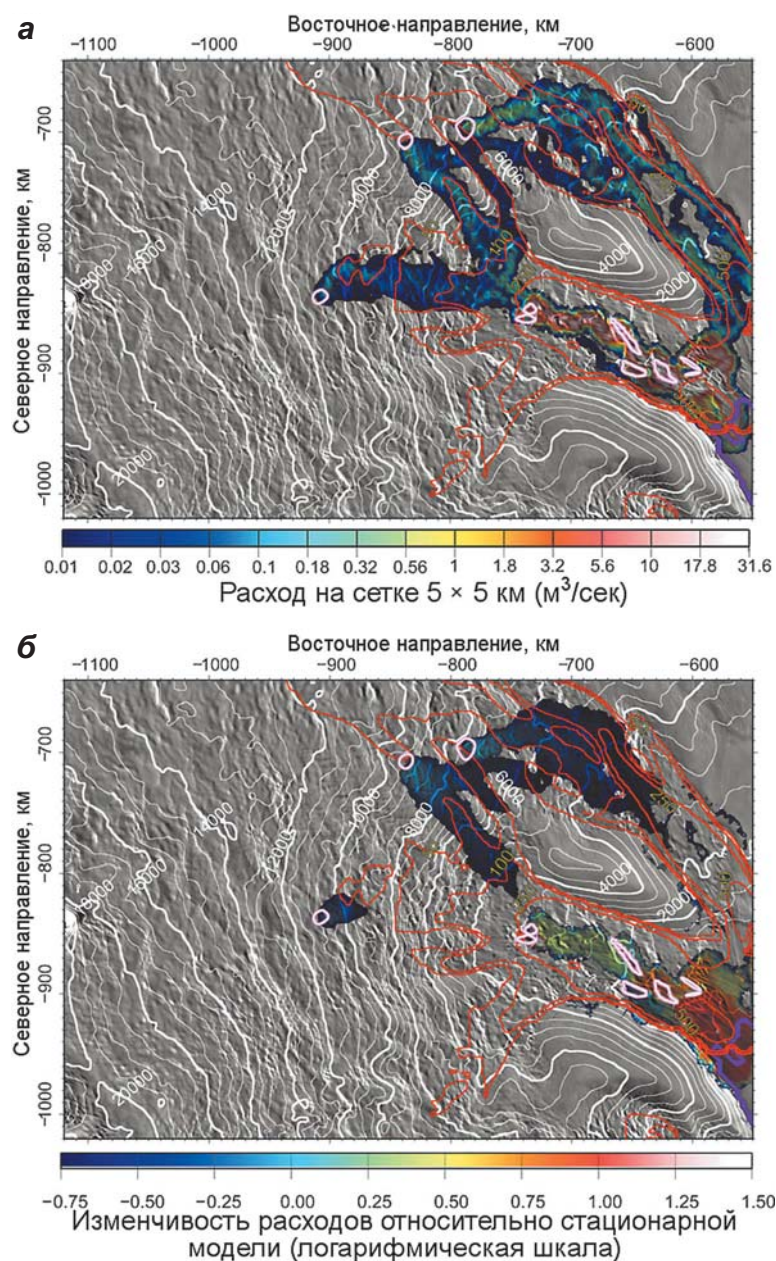
▲ Рис. 4.102. Диапазон расходов воды (цветная шкала, \text{м}^3/\text{с} ) по модели с сеткой 5 \times 5 \text{ км} (максимум–минимум) (а) и отклонения величин расхода по отношению к стационарному случаю (цветная логарифмическая шкала) (б) (Carter et al., 2011)
