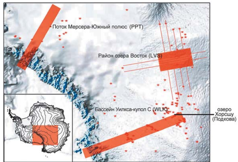
► Рис. 4.78. Районы радиозондирования в Антарктиде, где подледниковые озера были классифицированы по характеру и интенсивности радиолокационных отражений: бассейн озера Восток (LVS), ледяной поток Мерсера–Южный полюс (PPT), бассейн Уилкса–купол С (WLK) (Carter et al., 2007)
