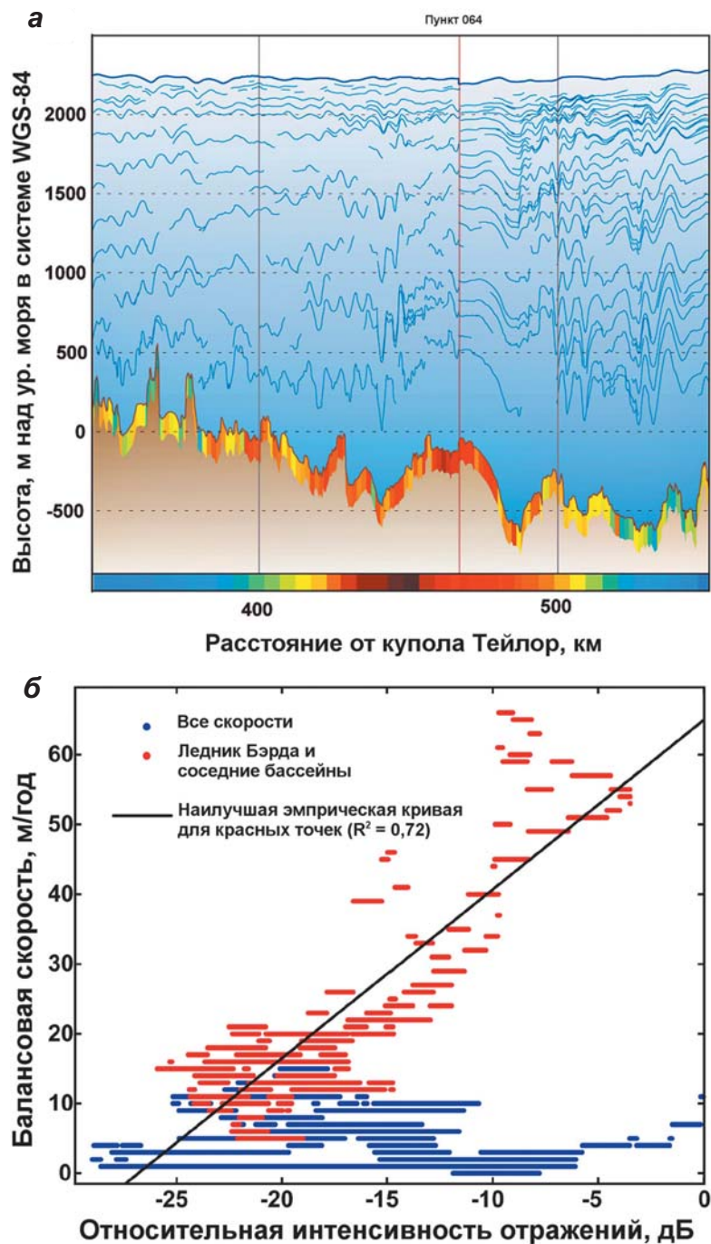
▲ Рис. 2.94. Интенсивность отражений от ложа (см. цветную шкалу на рис. 2.92, а) в северной части бассейна ледника Бэрд (а); для сравнения показаны балансовые скорости (нижняя цветная шкала от 0 до 70 м/год); связь между интенсивностью отражений от ложа на частоте 3 МГц и балансовыми скоростями (б). Красным выделены те данные, которые относятся к леднику Бэрд и прилегающим бассейнам; черной линией показана их линейная аппроксимация с коэффициентом детерминации R^2 = 0,72 (Jacobel et al, 2010)
