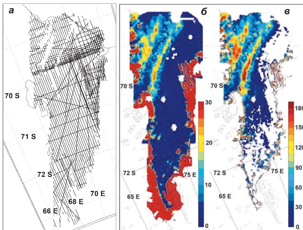
▲ Рис. 2.139. Шельфовый ледник Эймери: а) профили радиозондирования 1986–1995 гг. на частоте 60 МГц; б) распределение гидростатической аномалии \delta h' (цветная шкала); в) вычисленная толщина морского льда на подошве ледника (цветная шкала); серые линии – базовая карта района (береговая линия, фронт по данным ледника в 1997 г. и выходы горных пород) (Fricker et al., 2001; Wen et al., 2010)
