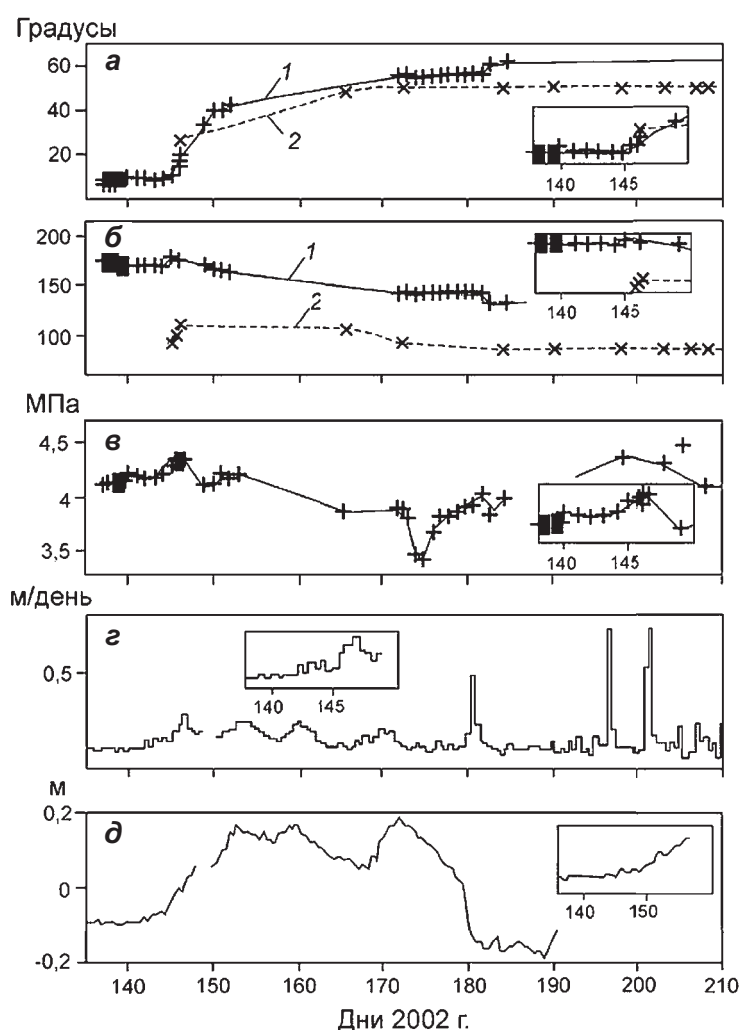
▲ Рис. 1.15. Результаты исследований 2002 г. на леднике Блэк-Репидс на Аляске (а, б); угловое смещение в слое тилла первого (1) и второго (2) датчиков соответственно; в – поровое давление воды по первому датчику; г – поверхностная скорость GPS-измерений; д – смещение поверхности поперек основного направления течения ледника (Truffer et al., 2006)
