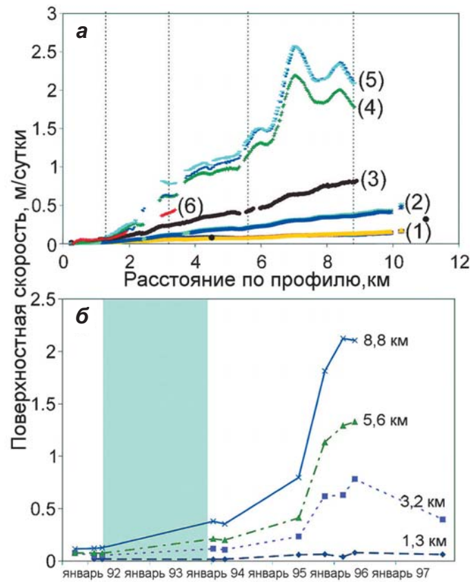
▲ ► Рис. 3.23. Изменение поверхностной скорости вдоль профиля от верховьев северо-западной ветви ледника Фридьоф до его нижней части (в): по данным спутниковой радиоинтерферометрии (Murray et al., 2003) (цветные линии) (а) в октябре 1991 г., феврале и марте 1992 г. (1), феврале и марте 1992 г. (2), январе и марте 1994 г. (3), июне 1995 г. (4), ноябре 1995 г. (5), феврале и мае 1996 г. (6) и октябре 1997 г.; на разных расстояниях от начала профиля по данным спутниковой радиоинтерферометрии (б) в период с января 1992 г. по январь 1997 г. (Murray et al., 2003) (цветные линии) и полевых измерений 1987 г. (Зингер и др., 1997) (черные кружки); голубой полосой показан интервал времени, когда скорости не могли быть определены из-за некогерентности радиоинтерферометрических изображений (Murray et al., 2003)
