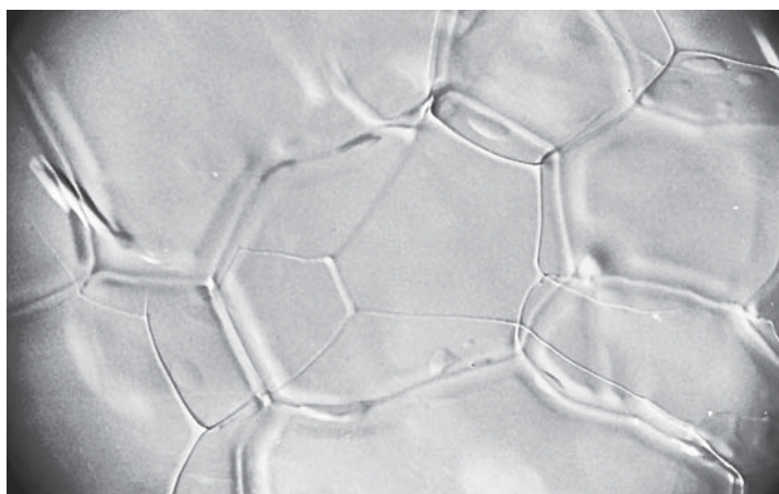
▲ Рис. 1.4. Канальцы воды в теплом льду на стыке трех зерен. Размер зерна в центре снимка около 1 мм (Fountain, Walder, 1998)
