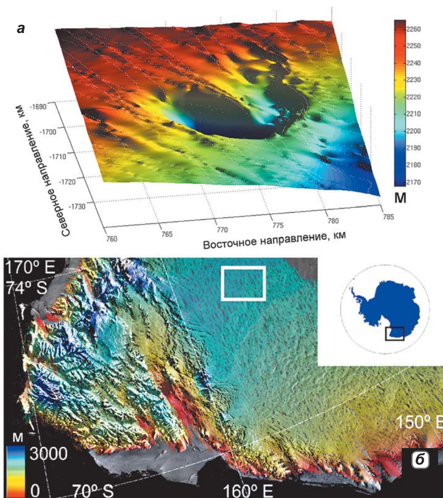
▲ Рис. 4.104. Подледниковое озеро Кука: а) область просадки поверхности ледника над опорожнившемся озером (цветная шкала в м над ур. моря), устанавливаемая по интерферометрическим измерениям (белые точки) со спутника CryoSat-2 в период между январем и ноябрем 2011 г.; б) местоположение района озера в Восточной Антарктиде выделено белым прямоугольником, высота поверхности по данным CryoSat-2 показана цветом (McMillan et al., 2013)
