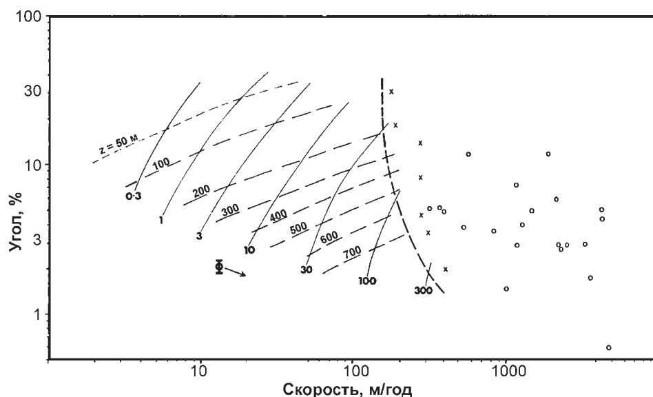
▲ Рис. 1.16. Связь средней толщины Z ледников, м (штриховые линии) с поверхностной скоростью V , м/год и наклоном \alpha поверхности, % вдоль их осевой линии. Расходы льда \Phi = VZ , 10^3 \text{ м}^3/\text{год} показаны сплошными линиями. Кружки и кресты – значения \Phi для быстро движущихся полярных ледников и ледников пульсирующего типа. Толстой штриховой линией показана кривая \alpha\Phi , которая может определять переход от нормальных к быстро движущимся ледникам, включая пульсирующие (Budd, 1975)
