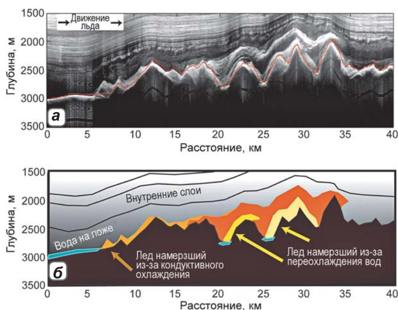
▲ Рис. 4.121. Процессы намерзания: а) радарная запись – стрелкой обозначено направление движения ледника, красной линией – отражение от ложа; б) интерпретация радарной записи в виде схемы процессов намерзания, голубым цветом показаны скопления воды на ложе, коричневой стрелкой – область намерзания за счет кондуктивного охлаждения, желтыми стрелками – области намерзания переохлажденной воды. Положение профиля показано на рис. 4.121, а (Bell et al., 2011)
