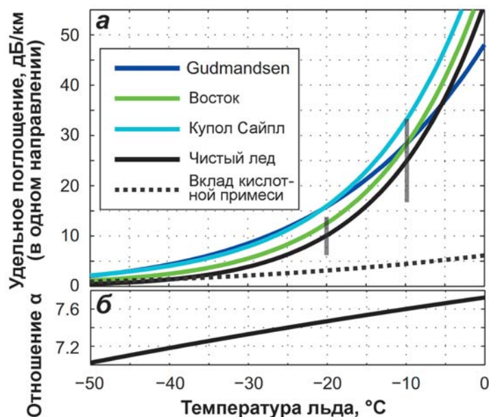
▲ Рис. 2.83. Зависимости ослабления радиоволн во льду от его температуры и содержания примесей кислот ( C_1 ) и солей ( C_2 ). (а) Чистый лед (черная кривая), влияние кислотных примесей (черный пунктир) при C_1 = 1 мкМ (микромоль на литр). Показаны также расчетные региональные зависимости для льда атмосферного происхождения (синяя кривая – по данным Gudmandsen, 1971), для льда на куполе Сайпл в Западной Антарктиде (голубая кривая) с осредненными по глубине значениями C_1 = 1,2 мкМ и C_2 = 4,1 мкМ (MacGregor et al., 2007); для льда со станции Восток (зеленая кривая) в Восточной Антарктиде со средними значениями C_1 = 0,5 мкМ и C_2 = 2,0 мкМ (MacGregor et al., 2009). Две серые линии показывают интервалы неопределенности для чистого льда, оцененные с учетом средних квадратичных отклонений диэлектрических измерений (MacGregor et al., 2007); (б) \alpha (%) показывает соотношение вклада кислотных примесей и солей (при одинаковой молярности) в ослабление радиоволн в зависимости от температуры льда (Matsuoka et al. 2012)
