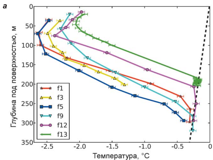
▲ ► Рис. 4.5. Вертикальные профили температуры (относительно точки плавления) в леднике Гренч: (а) в скважинах f1, f3, f5, f9, f12, f13, расположенных вдоль центральной линии тока, пунктирная линия показывает температуру таяния льда при соответствующем давлении; (б) красная линия – поверхность раздела холодного и теплого льда CTS); (в) радарный профиль;
