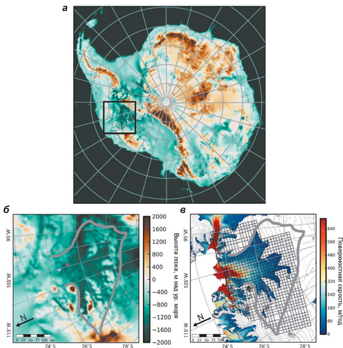
▲ Рис. 4.52. Ледник Туейтс: а) положение ледника в Западной Антарктиде (черный квадрат); б) высота ложа в бассейне ледника; в) радарные профили по сети 15×15 км и поверхностные скорости более 35 м/год (цветная шкала справа), светлые и темные фиолетовые точки показывают положение радарограмм на рис. 4.53, б (Schroeder et al., 2013)
