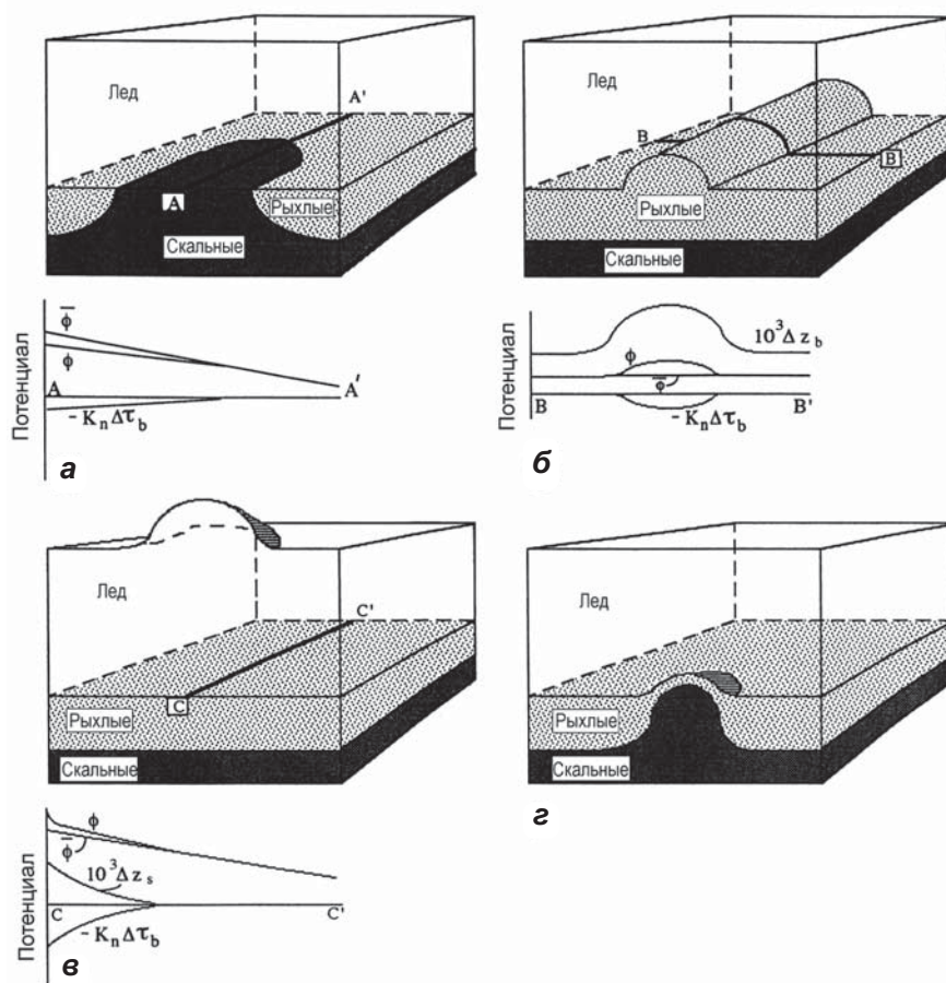
▲ Рис. 4.62. Пятна прилипания на ложе и их влияние на подледниковый гидравлический потенциал \phi = \phi_0 + 10^4 \Delta z_s + 10^3 \Delta z_b - K_n \Delta \tau_b , где \phi_0 отражает региональный тренд \phi , \Delta z_s и \Delta z_b – пертурбации высот поверхности и ложа относительно региональных значений; \Delta \tau_b – напряжение сдвига на ложе, K_n – безразмерная константа, равная 0 или 1. Пятно прилипания, связанное с неоднородностью поверхности ложа, без пертурбации верхнего или нижнего слоев льда (а); пятно прилипания, связанное с длинной складкой однородного ложа, без изменений верхней поверхности (б); выступ поверхности над ненарушенным ложем, приводящий к локальному возмущению поля гидравлического потенциала (в); пятно прилипания, связанное с выступом на ложе, покрытого или нет слоем тилла, играющего роль смазки (г) (Alley, 1993)
