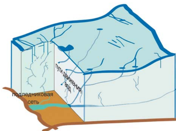
◀ Рис. 2.22. Поступление талых вод из поверхностных водотоков и наледниковых озер в толщу и к ложу ледникового покрова через трещины, ледниковые колодцы и зоны дробления льда (Phillips et al., 2010)
