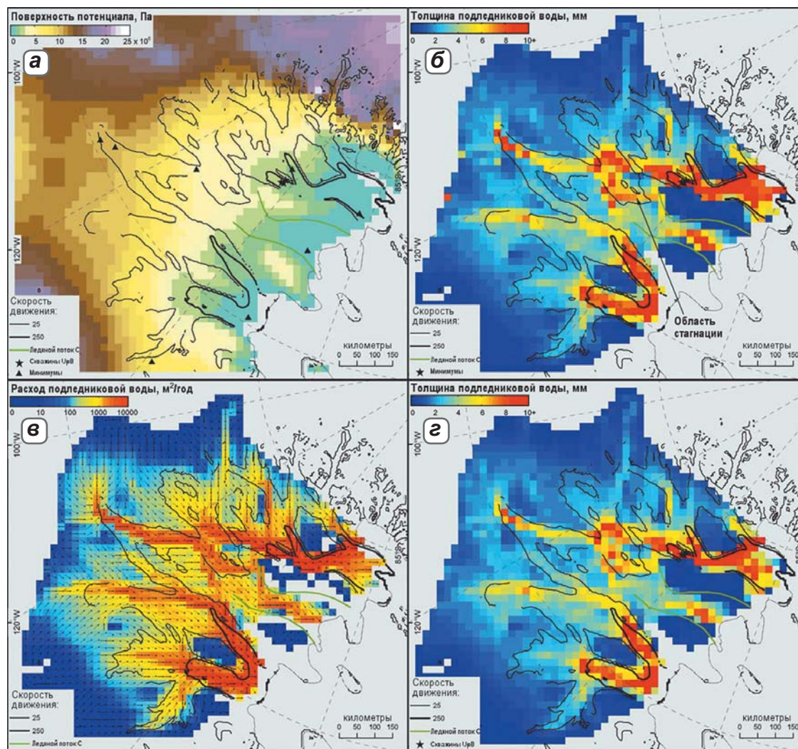
◀ Рис. 4.58. Ледяные потоки в секторе моря Росса: а) поверхность гидравлического потенциала (замкнутые минимумы в поле потенциала обозначены треугольниками); б) рассчитанная толщина воды под ледником для нестационарного случая; в) расход подледниковой воды на единицу ширины для нестационарного случая; г) рассчитанная толщина воды под ледником для стационарного случая. На всех рисунках изолинии черного цвета показывают измеренные скорости на поверхности ледника. Разрешение модели 20 км (LeBrocq et al., 2009)
