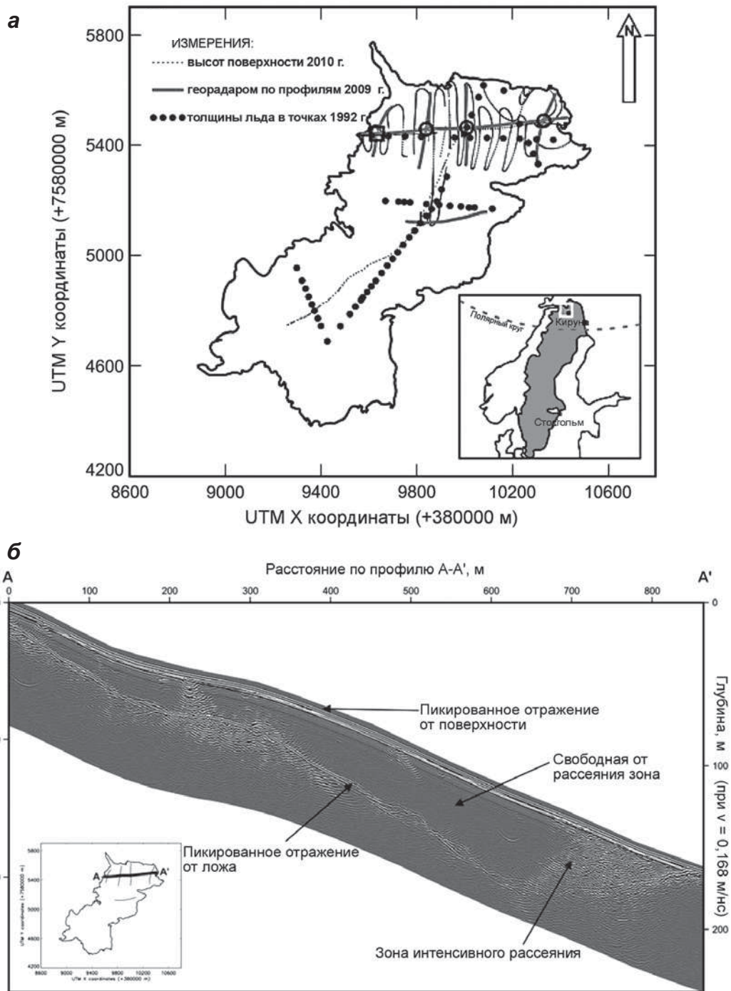
▲ Рис. 4.24. Радиолокационные измерения в 2009 г. на леднике Карса в северной Швеции на частоте 50 МГц (а); радарные отражения на продольном профиле (б): внизу – от ложа, справа – интенсивное внутренне рассеяние вблизи языка ледника, вверху – свободная от рассеяния зона (Rippin et al., 2011)
