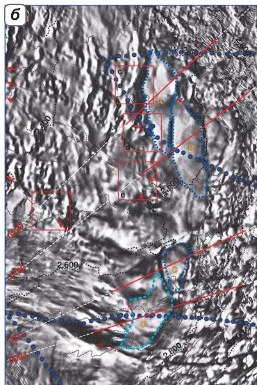
▼ Рис. 4.81. Подледниковые озеро на 90° в.д. в Восточной Антарктиде (а) и озера в верховьях ледяного потока Рекавери в Западной Антарктиде (б), выявленные по данным космических съемок. На рис. (а) треугольники показывают положение других озер в этом районе по данным (Sieger et al., 2005). Сплошная и точечная линии указывают положение радарного профиля, цветные точки – аномалии силы тяжести в мГал по измерениям 1958 г.; на рис. (б) показаны четыре подледниковых озера (А, В, С, D) в верховьях ледяного потока Рекавери по данным лазерной альтиметрии со спутника ICESat (Bell et al., 2006, 2007)
