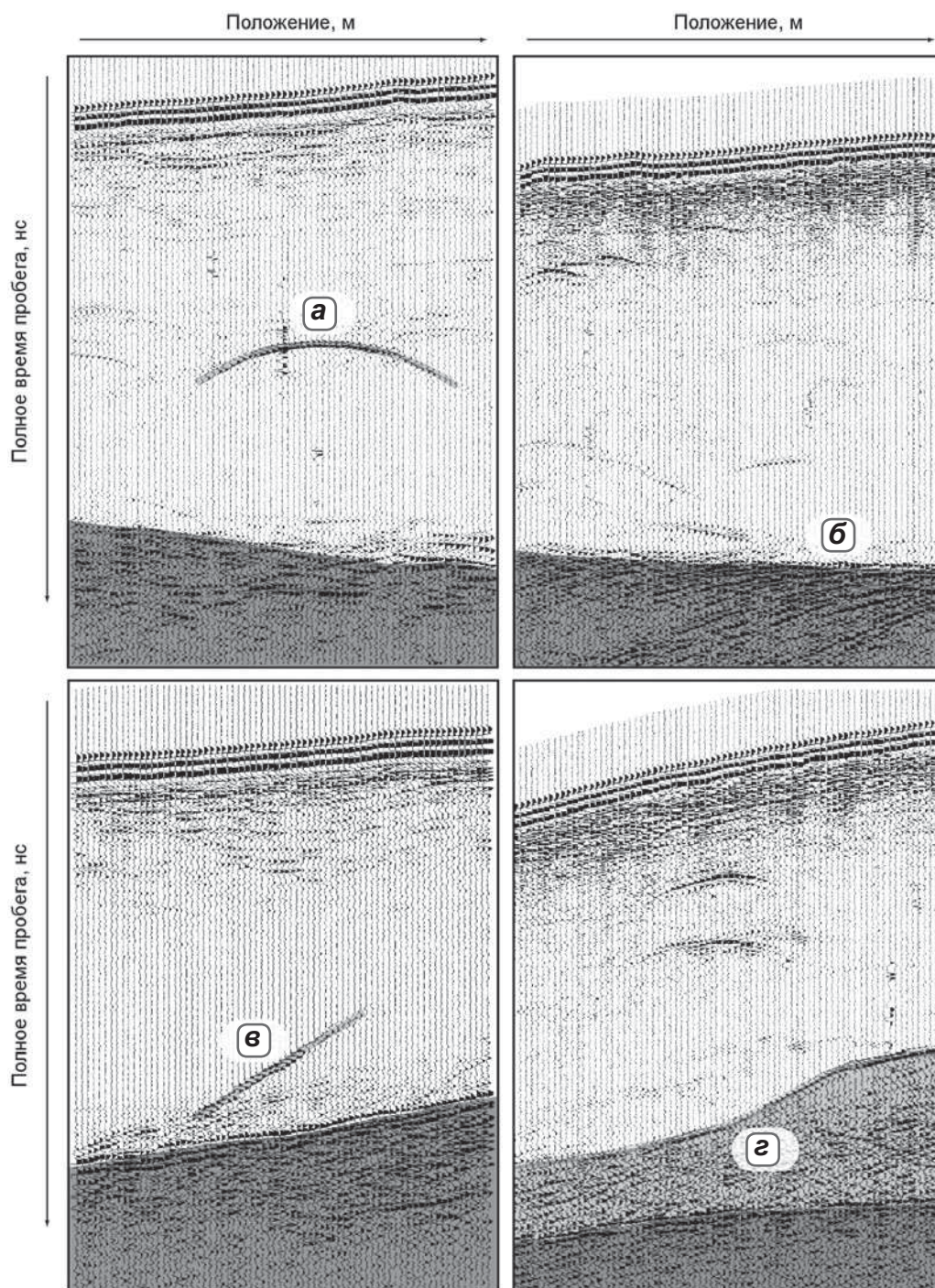
▲ Рис. 4.12. Типичные отражения на леднике Стагнейшн: а) гиперболические отражения А от точечного внутриледникового отражателя; б) отражения от наклонного ложа В; в) линейное внутриледниковое отражение С; г) хаотические отражения из придонного слоя теплого льда D (Irvine-Fynn et al., 2006)
