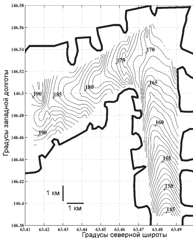
▲ Рис. 4.36. Распределение гидравлического потенциала на теплом леднике Блэк Рэпидс (Gades, 1998)
