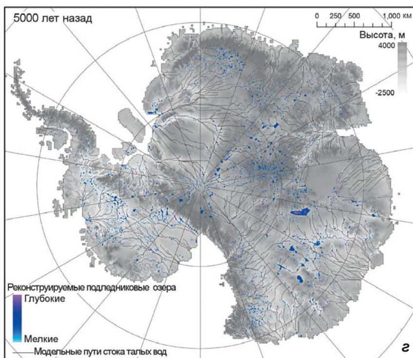
20, 15, 10 и 5 тыс. лет назад (а-г) (Livingstone et al., 2013) ▲
