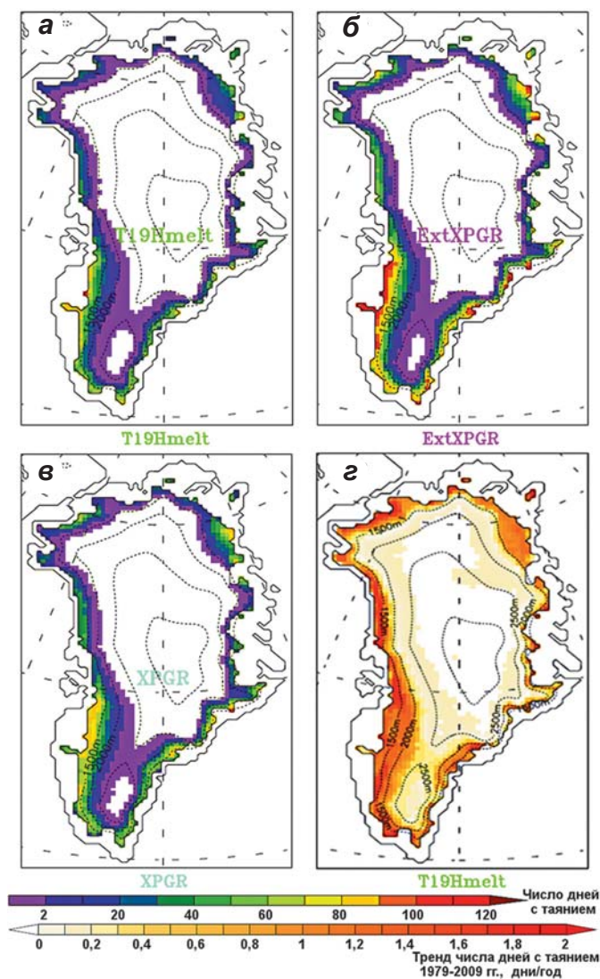
▲ Рис. 2.8. Среднее годовое количество дней с таянием за период 1979–2009 гг. на ледниковом покрове Гренландии по данным микроволновых измерений, оцененное тремя описанными выше методами: T19H melt (а), ExtXPGR (б) и XPGR (в); тренд количества дней с таянием в году за тот же период по данным TP19 melt (г). Верхняя цветная шкала относится к (а–в), нижняя – к (г) (Fettweis et al., 2011)
