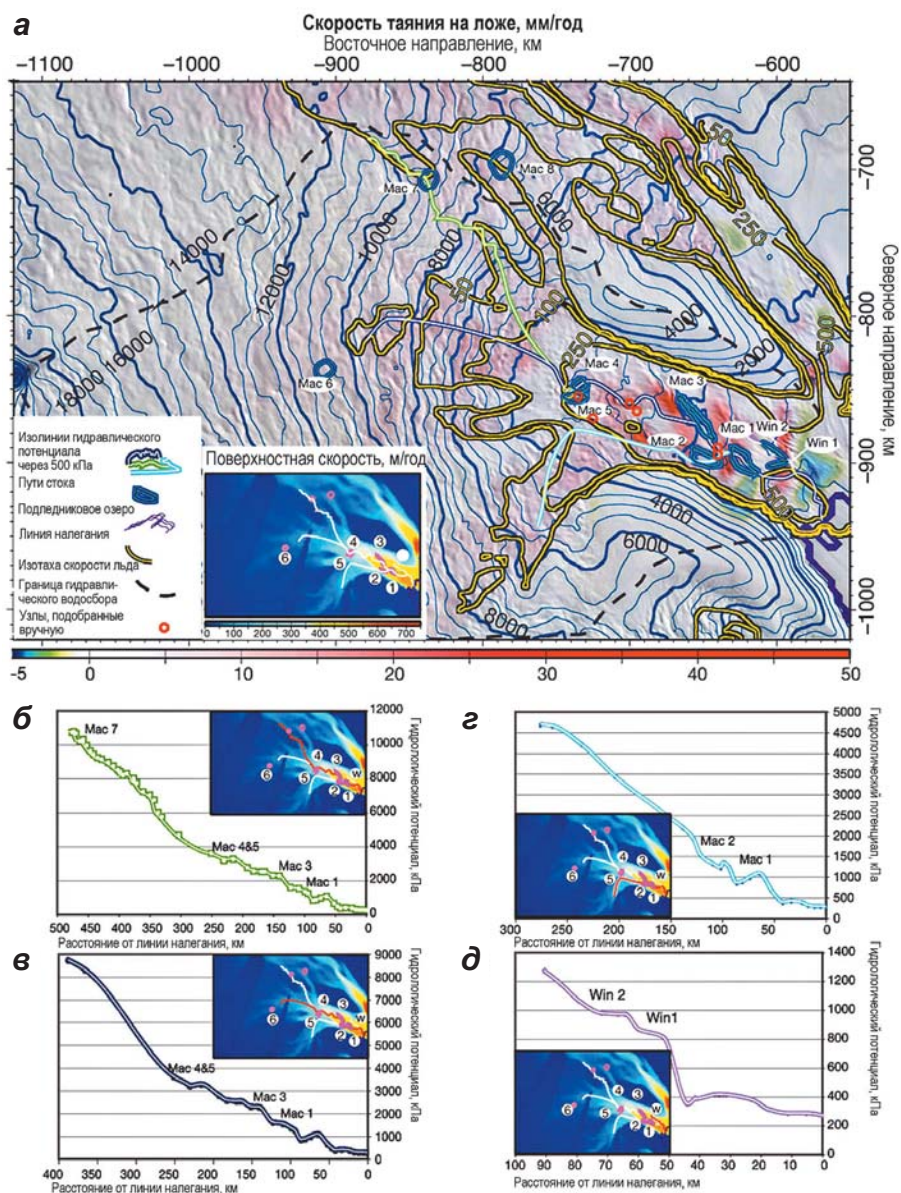
▲ Рис. 4.100. Подледниковые озера в бассейне ледяного потока Мак-Эйла (Е): а) скорость донного таяния (цветная шкала внизу), изолинии гидравлического потенциала (синие линии) и поверхностной скорости, желтым цветом показаны контуры 50, 100, 250 и 500 м/год по данным (Joughin et al., 2004); б–д) гидравлический потенциал по профилям через локальные минимумы (показаны красными линиями на врезках) (Carter et al., 2011)
