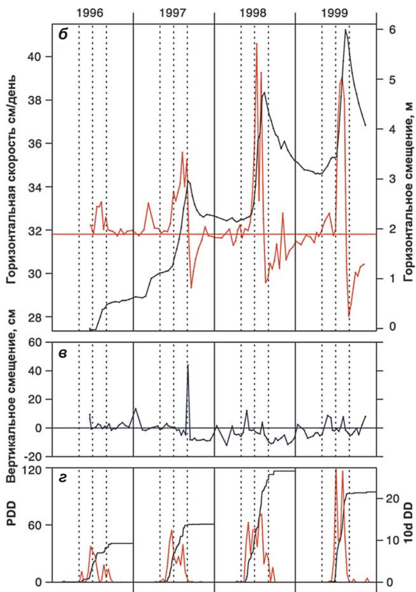
▲▲ Рис. 2.26. Область таяния и наледниковые озера в области абляции ледникового покрова Гренландии в районе станции Swiss Camp на Landsat TM (канал 13) от 22 июня 1990 г. (а); горизонтальная скорость (красная кривая) вдоль сглаженной линии тока, показывающая ускорения льда во время летних сезонов таяния и резкие переходы к замедлению при прекращении таяния (б); кумулятивное дополнительное смещение (черная линия) относительно средней зимней скорости 31,33 см/день, равное 6,0 м на время максимальной скорости в 1999 г.; вертикальное смещение (синяя линия), показывающее подъем на 50 см во время перехода в 1997 г. от ускоренного к замедленному течению льда (в); кумулятивные положительные дневные температуры воздуха (PDD, градусо-дни), демонстрирующие корреляцию для 10-дневных интервалов (красные линии) с интенсивностью и временем ускорений и замедлений (г); вертикальные пунктирные линии обозначают дни 1 мая, 1 июля и 1 сентября каждого года (Zwally et al., 2002)
