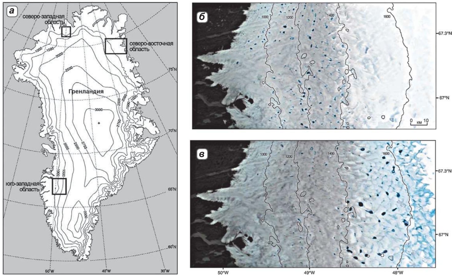
► ▼ Рис. 2.18. Изменение положения и размеров наледниковых озер на юге юго-западной области Гренландии (а) в сезон таяния 2003 г. Показано состояние озер на 162 день (б) и 169 день (в) этого года на изображениях MODIS (Sundal et al., 2009)
