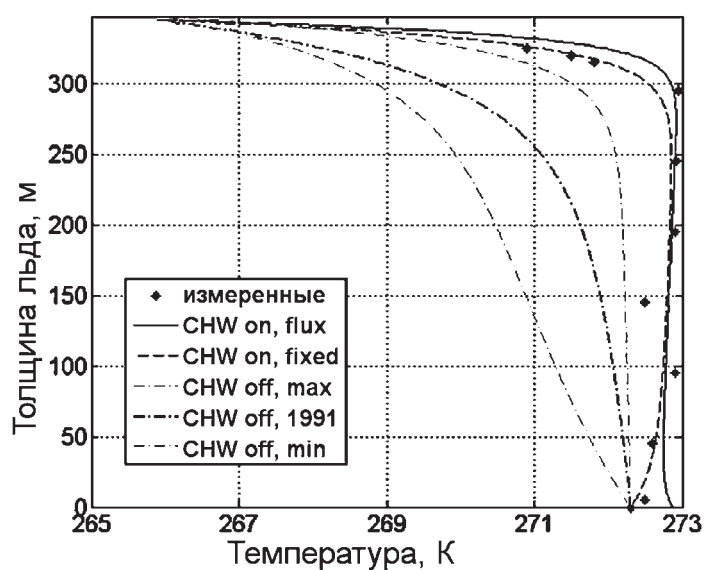
▲ Рис. 4.27. Измеренные (точки) и рассчитанные (линии) температуры для скважины TD3 на выводном леднике Сермек Аваннарлек; в расчетах с криогидрологическим отоплением (CHW on) использовали градиент температуры 0,0227 К/м или измеренную температуру ("fixed") на ложе; в расчетах без криогидрологического отопления (CHW off) использовали измеренную температуру на ложе; кривые "min" и "max" получены при скоростях адвекции льда в 2 раза больше и в 4 раза меньше средней скорости (80 м/год на поверхности и 6 м/год у ложа) (Phillips et al., 2011)
