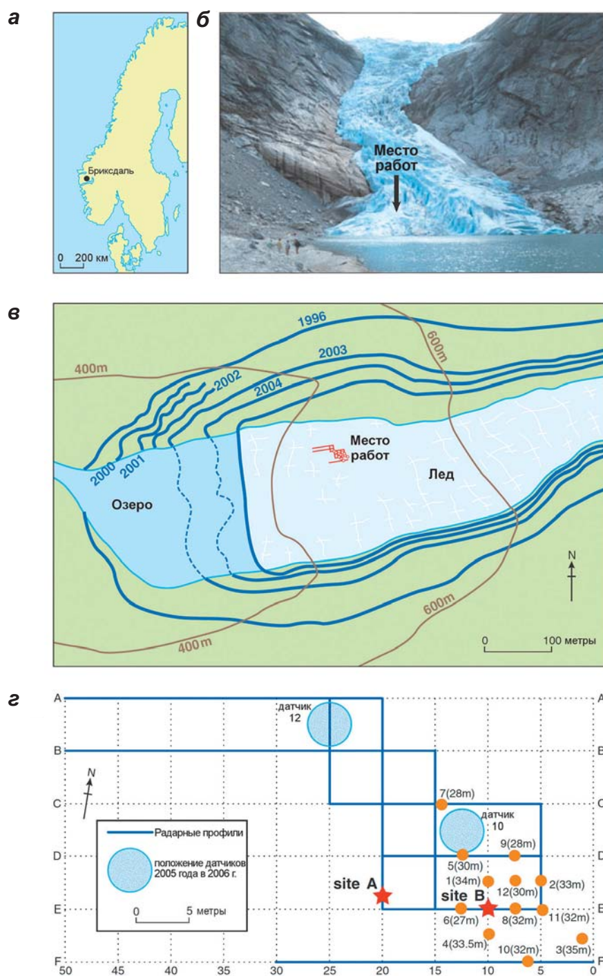
▲ Рис. 4.8. Ледник Бриксдаль (а) и участок эксперимента (б); в) положение радарных измерений по профилям (толстые синие линии) и г) в фиксированных точках А и В (красные звездочки), места скважин (желтые кружки) и положения беспроводных датчиков давления (большие синие кружки) (Hart et al., 2011)
