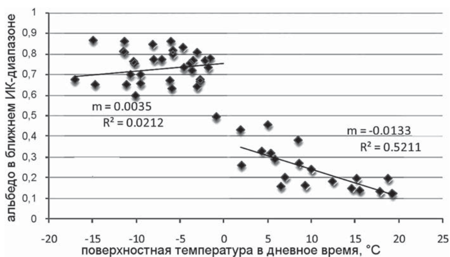
▲ Рис. 2.3. Альbedo снега в ближнем инфракрасном диапазоне в зависимости от поверхностной температуры (Malik, 2009)
