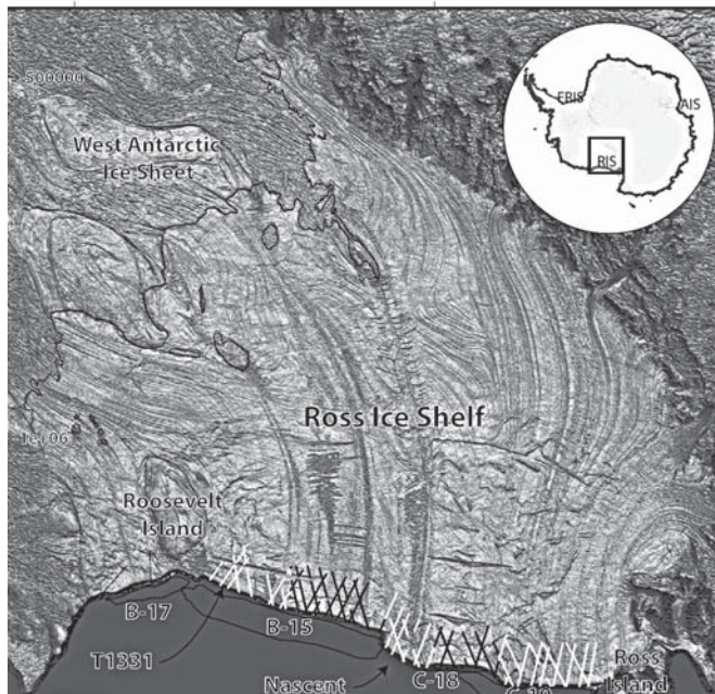
◀ Рис. 2.152. Треки измерений со спутника ICESat высоты поверхности у фронта шельфового ледника Росса. Толстой черной линией показано положение линии налегания. Тонкие черные линии и стрелки обозначают отдельные события откола айсбергов с января 2000 г. (Horgan et al., 2011)
