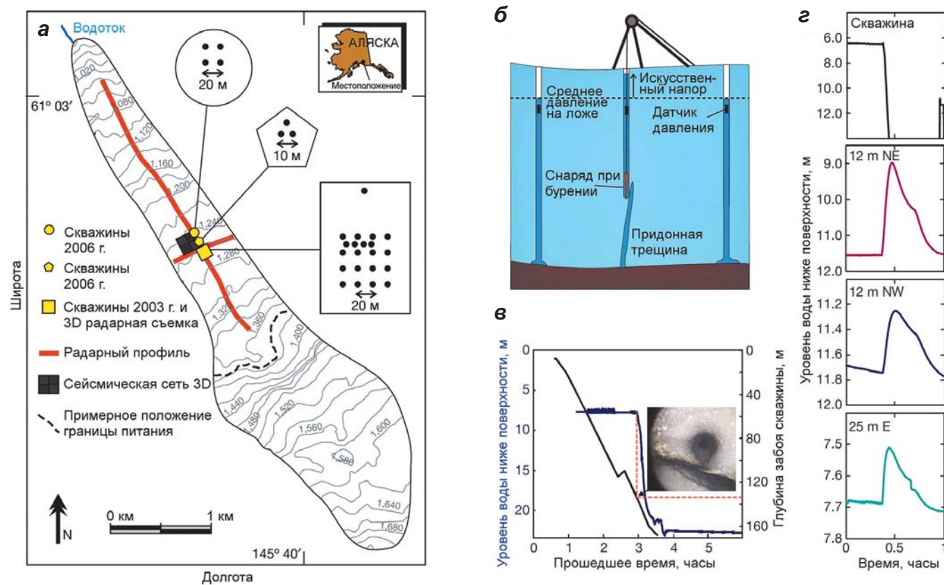
▲ Рис. 2.69. Положение скважин на леднике Бенч на Аляске и участков сейсмических, радиолокационных и DGPS измерений (а); измерение уровня и давления воды в скважине, пересекшей придонную трещину, и в соседней скважине (б); падение уровня воды в скважине, пересекшей придонную трещину на глубине 133 м (в 32 м выше ложа) (в); график проходки скважины – черная линия, уровень воды в скважине – голубая линия; уровни воды в четырех скважинах (г): когда одна из скважин достигла трещины на глубине 106 м, уровень воды в ней упал более чем на 10 м, а в трех соседних скважинах на расстоянии до 25 м он одновременно поднялся (Harper et al., 2010)
