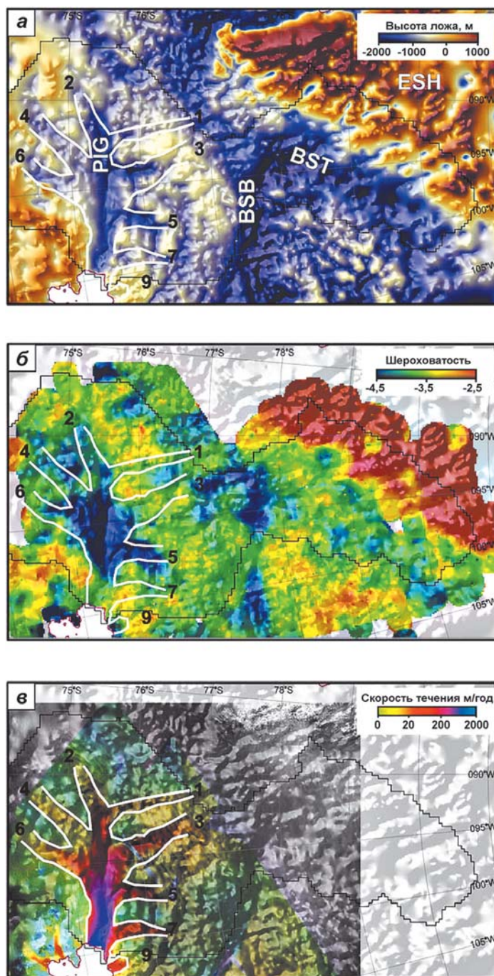
▲ Рис. 2.109. Топография ложа всего района ледника Пайн Айленд по данным (Vaughan et al., 2006) и из многих источников (а); буквами обозначены: PIG – ледник Пайн Айленд, BSB – подледниковый бассейн Берда, BST – подледниковый трог Бенгли, ESH – подледниковая горная страна Элсуорта; цифрами (как на рис. 2.106) – притоки ледника Пайн Айленд; шероховатость ложа в этом районе в логарифмическом масштабе (б); InSAR скорости по данным (Rignot et al., 2004) (в) (Rippin et al., 2011)
