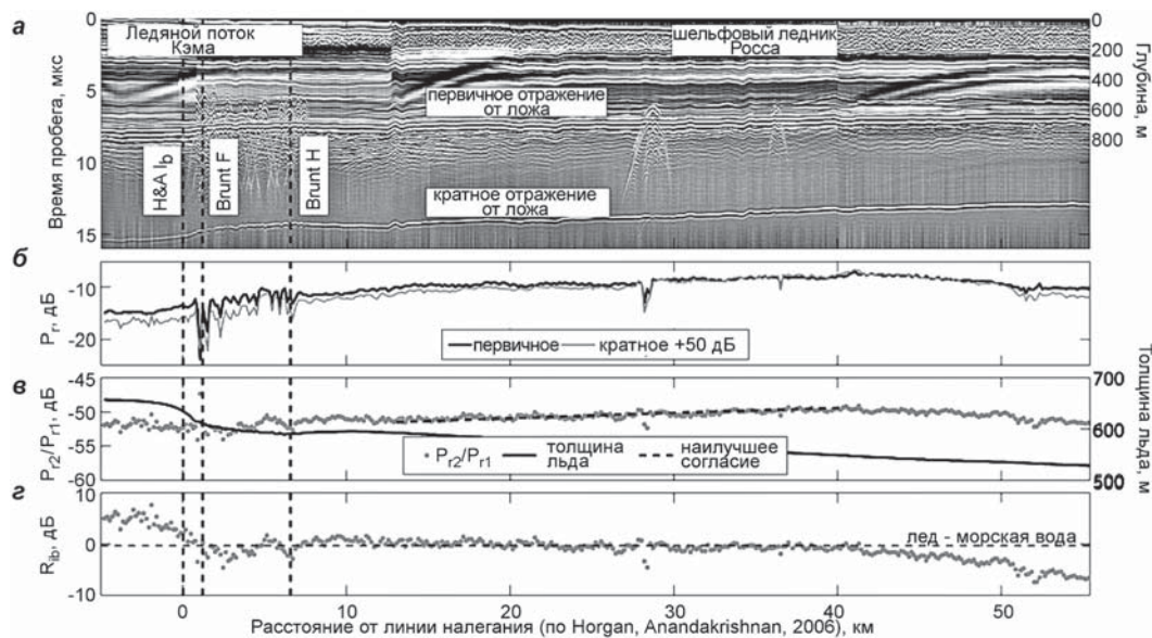
▲ Рис. 2.89. Радарная запись вдоль профиля K4 (а); мощность, дБ, однократных ( P_{r1} ) и двукратных ( P_{r2} ) отражений от ложа (б) (темная и светлая линии); для отражений P_{r2} шкала интенсивности увеличена на 50 дБ; отношение P_{r2}/P_{r1} (в); толщина льда (черная и пунктирная линии) найдена методом наименьших квадратов из уравнения (2.75); коэффициент отражения от ложа R_{ib} выше и ниже линии налегания, оцененной по точкам I_b (Hogan, Anandakrishnan, 2006) и F и H (Brunt et al., 2010) (г) (вертикальные пунктирные линии) (McGregor, 2011)
