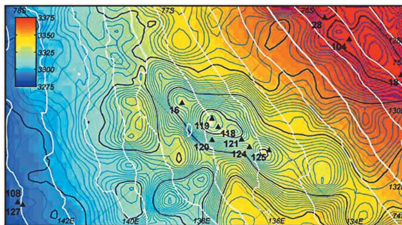
▲ Рис. 4.127. Вычисленное потенциальное гидравлическое давление, м льда (цветная шкала) в районе подледникового трога Адвенчер. Высота поверхности показана белыми линиями с интервалом 50 м, высота ложа – голубыми и более толстыми линиями с интервалом 50 и 500 м, подледниковые озера – черными треугольниками (Wright et al., 2008)
