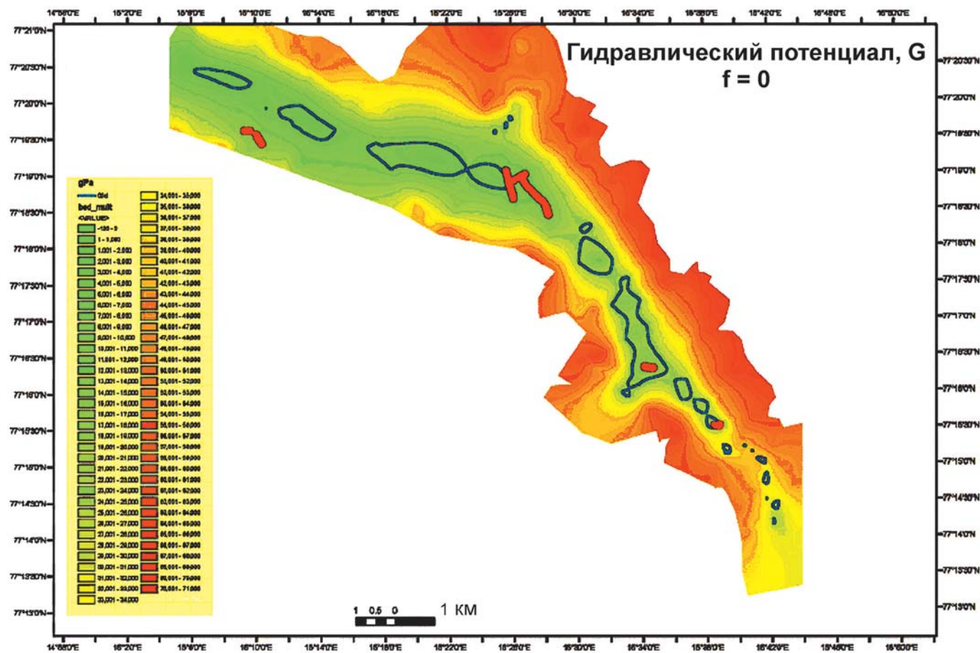
▲ Рис. 3.26. Строение ледникового плато Амундсена по данным наземного радиозондирования и DGPS-измерений 2004–2006 гг.: д) распределение гидравлического потенциала (Гловацкий и др., 2008)
