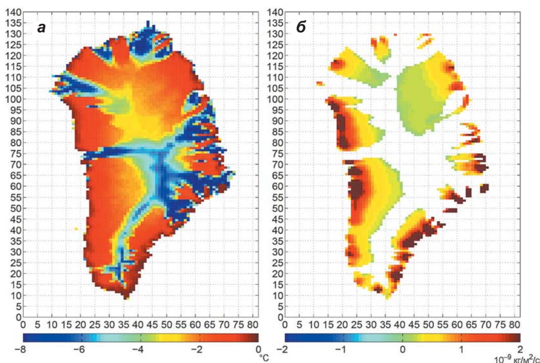
▲ Рис. 4.45. Температура (а) и скорость донного таяния (б) в Гренландии по данным моделирования (Heimbach, Bougnion, 2009)
