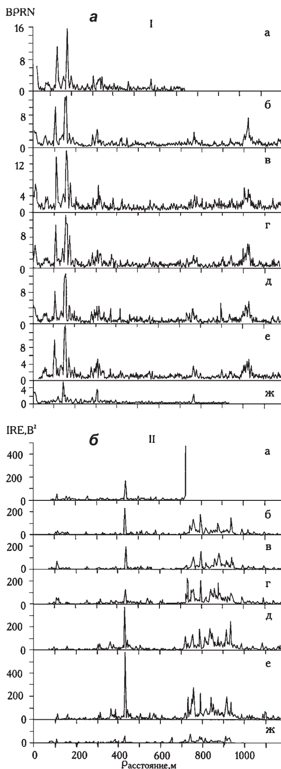
◀ Рис. 3.5. Изменение мощности отраженных сигналов от ложа BPRN (а) и из толщи теплого льда IRE (б) вдоль поперечного профиля ледника Ханс в период таяния 2003 г. (а – 17 июля, б – 19 июля, в – 20 июля, г – 23 июля, д – 25 июля, е – 26 июля, ж – 4 августа) (Яниа и др., 2005)
