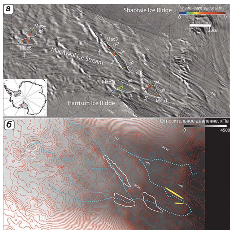
▲ Рис. 4.97. Ледяной поток Мак-Эйла (Е) (а), где по данным ICESat 2003–2009 гг. (тонкие серые линии) обнаружены (б) пять районов со значительными (до 9 м) изменениями высоты поверхности ледника. Границы озер показаны белыми сплошными линиями. Гидрологический потенциал (кПа) рассчитан по отношению к давлению на линии налегания. Голубым пунктиром намечены пути стока воды. Желтым выделены области, где в 2005/06 г. были зафиксированы сейсмические всплески (Winberry et al., 2009; Fricker et al., 2010)
