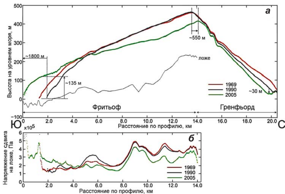
▲ Рис. 3.19. Изменение высоты поверхности ледников Фритьюф и Восточный Гренфьорд и положение ложа на леднике Фритьюф (синяя линия) вдоль их центральной линии, показанной на рис. 3.17, а), до подвижки ледника Фритьюф в 1969 и 1990 гг. (черная и зеленая линии) и после его подвижки в 2005 г. (красная линия) (а); вычисленное по ЦМР поверхности и ложа напряжение сдвига на ложе ледника Фритьюф до его подвижки в 1969 г. (черная линия) и в 1990 г. (зеленая линия) и после его подвижки в 2005 г. (красная линия) (б) (Murray et al., 2012)
