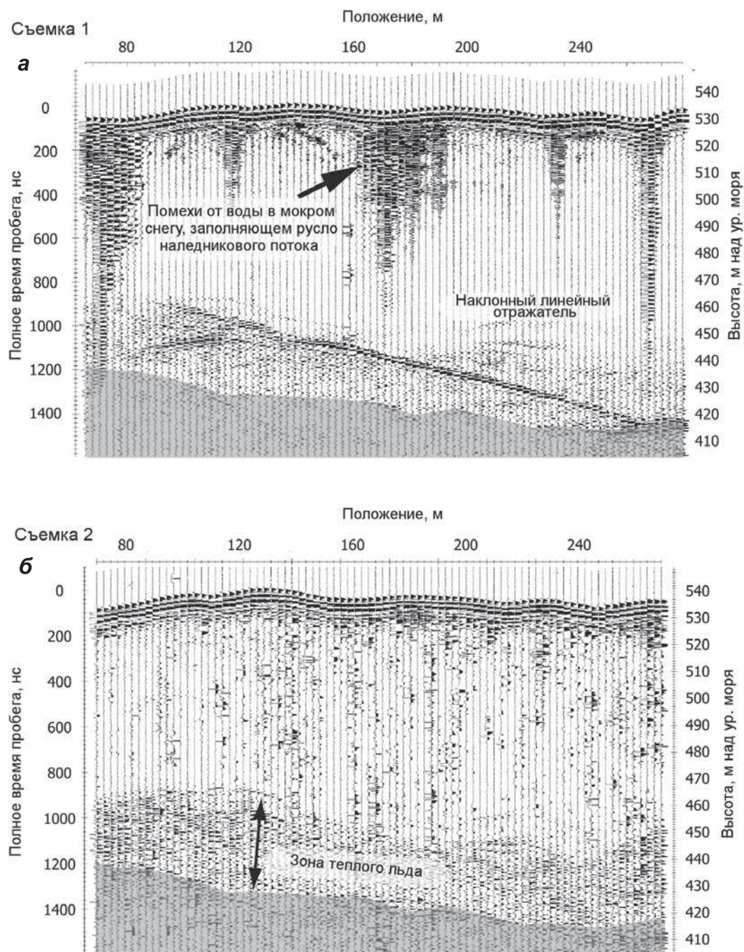
▲ Рис. 4.13. Изменение гидротермической структуры ледника Стагнейшн в июне–августе 2002 г. между радарными съемками 1 (а) и 2 (б) на частоте 50 МГц на профиле N17 (см. рис. 4.11). Стрелкой показаны отражения от воды в зоне снежной слякоти. В нижнем слое теплого льда толщиной около 100 м на (а) видно сильное линейное отражение, которое отсутствует на (б) (Irvine-Fynn et al., 2006)
