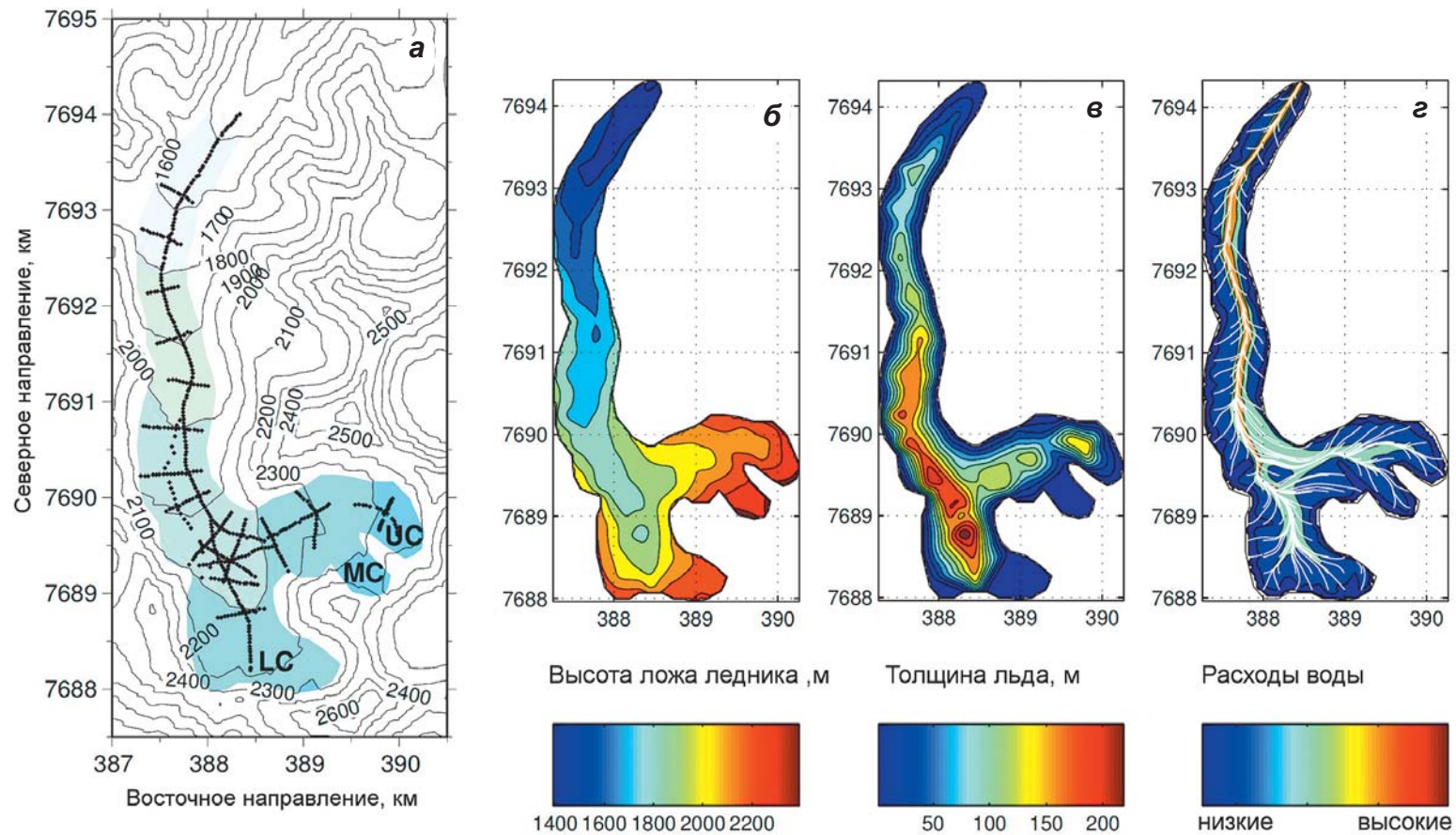
▲ Рис. 4.35. Политермический ледник Мак-Ком на Аляске: а) радиолокационные профили; б) высота ледниковой поверхности и радиолокационные профили; в) толщина льда, г) подледниковая гидрологическая сеть (Pattyn et al., 2009)
