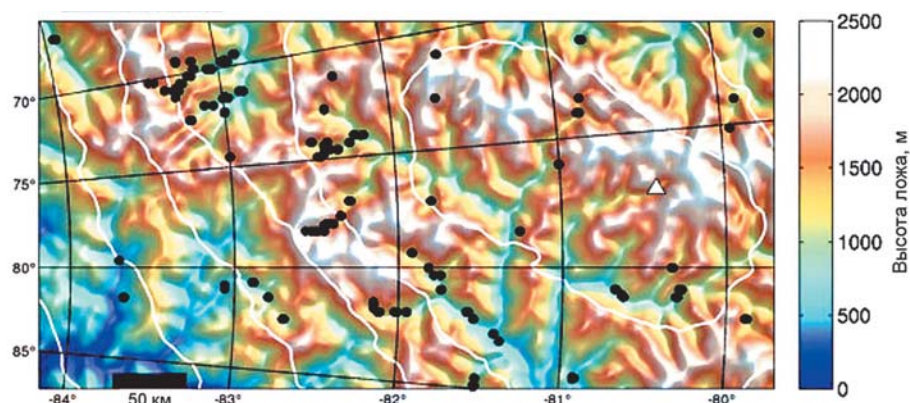
▲ Рис. 4.123. Рельеф ложа, где черными точками показано положение скоплений воды, которые с высокой степенью достоверности идентифицированы на радарных записях с использованием комплекса критериев (Wolovick et al., 2013)
