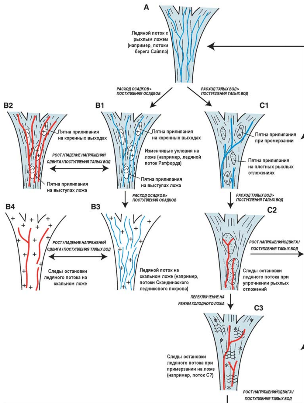
▲ Рис. 4.65. Влияние пятен прилипания на эволюцию ледяных потоков с мягким ложем при сценариях, когда накопление подледниковых отложений (сценарии В1–В4) и накопление талой воды (сценарии С1–С3) становятся ограничивающими факторами. Серым цветом показаны мелкозернистые деформируемые отложения, черными крестами – твердые кристаллические породы ложа, тонкими голубыми линиями – распределенная система мелких каналов, более толстыми голубыми линиями – система более крупных R-каналов. Заполнение этих каналов водой продуцирует эскеры (показаны толстыми красными линиями) (Stokes et al., 2007)
