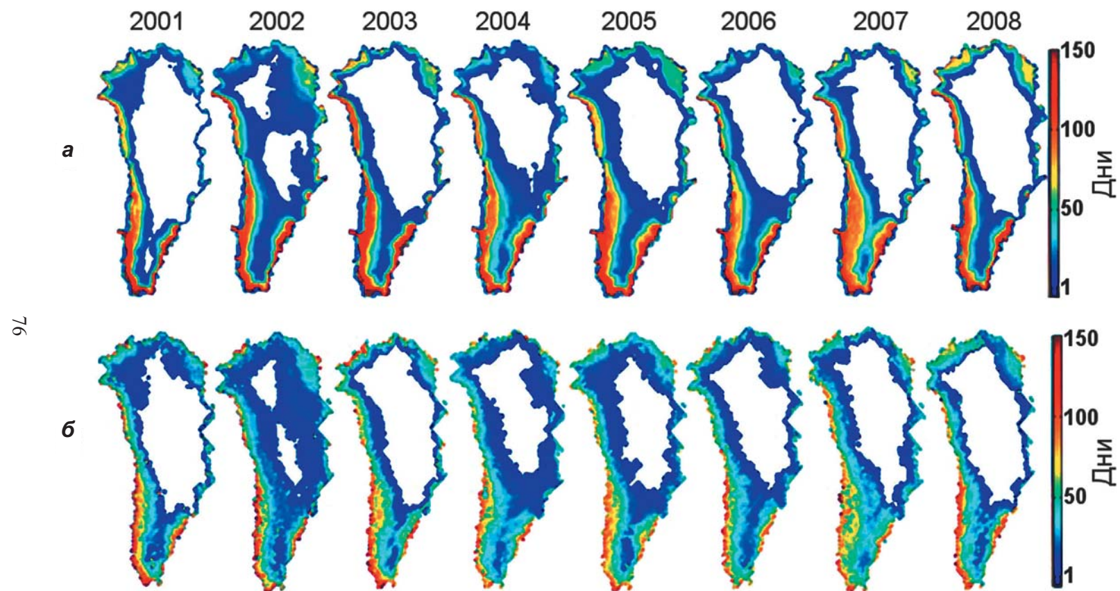
▲ Рис. 2.13. Продолжительность сезона таяния в 2001–2008 гг. по данным QuikSCAT (а) и SSM/I (б) (Bhattacharya et al., 2009)
