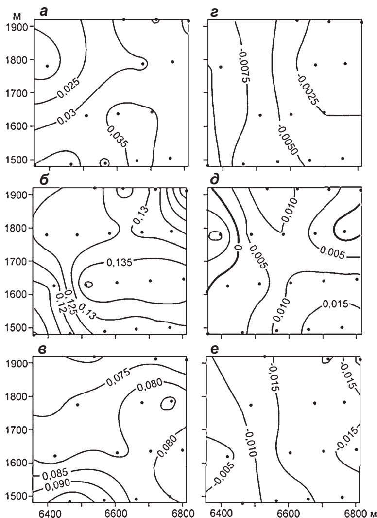
▲ Рис. 1.12. Продольные (а–в) скорости: (а) до события повышения скорости (дни 169–173 с начала 1994 г.), (б) во время этого события (дни 173–176) и (в) после него (дни 176–180) и вертикальные скорости (г–е) для соответствующих событий. Положение точек измерения скорости показано точками (Mair et al., 2002)
