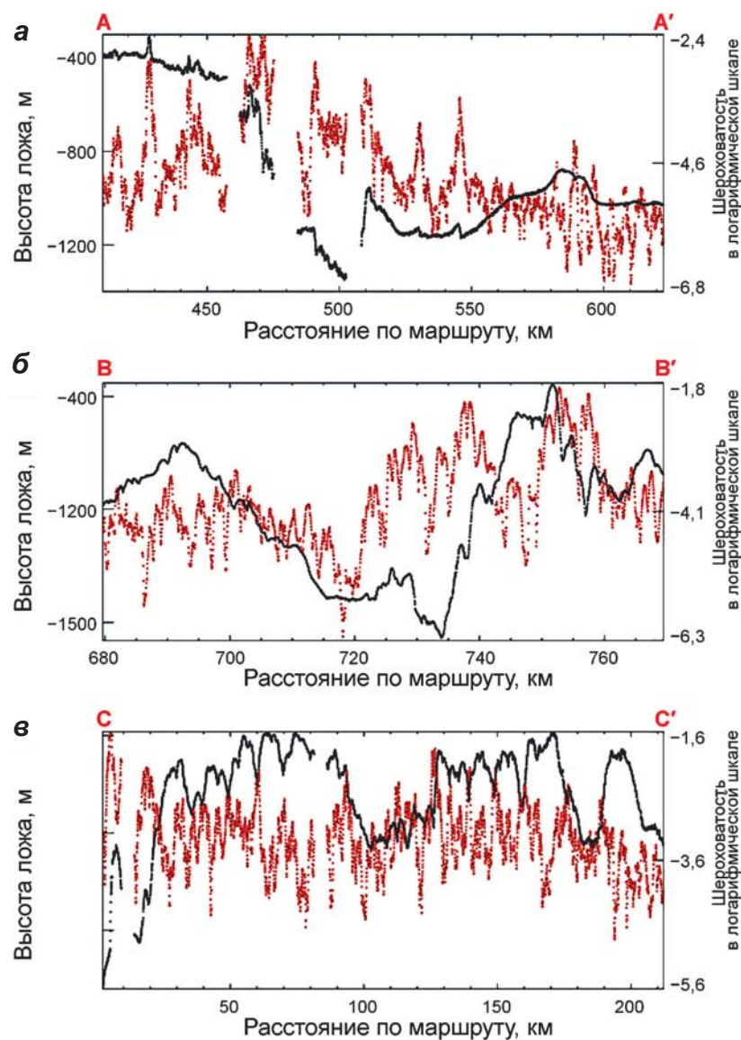
▲ Рис. 2.108. Высота ложа (черные линии) и его шероховатость в логарифмической шкале (красные линии) вдоль профилей A–A' (а), B–B' (б) и C–C' (в) на рис. 2.107 (Rippin et al., 2011)
