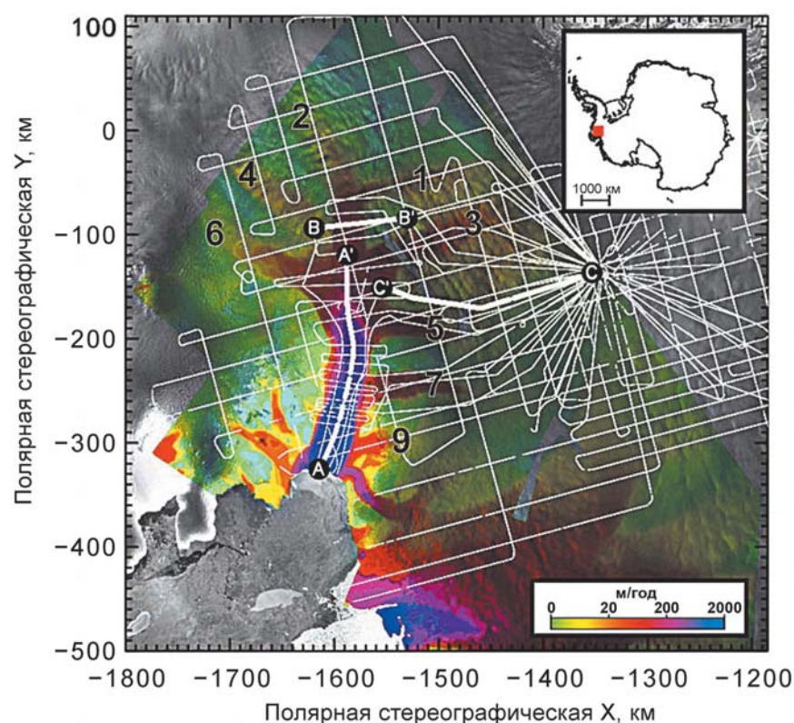
▲ Рис. 2.107. Маршруты полетов (тонкие белые линии) над ледником Пайн Айленд и его притоками (обозначены цифрами) со скоростями течения до 2000 м/год (цветная шкала); толстыми белыми линиями показаны участки полетов вдоль основного ствола ледника (A–A'), части притока 2 (B–B') и в районе медленного течения льда вне притоков C–C') (Rippin et al., 2011)
