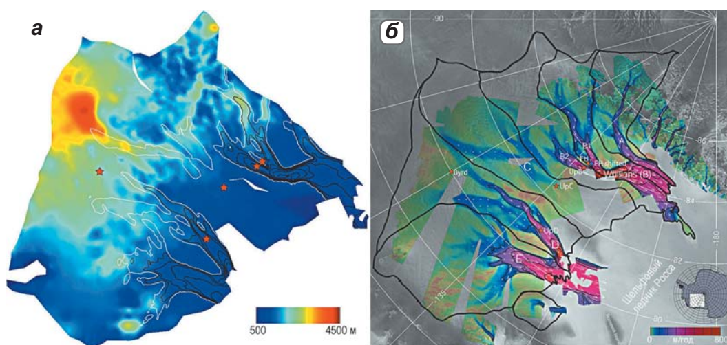
▲ Рис. 4.54. Толщина льда (а) и скорость течения (б) ледяных потоков Росса (Joughin et al., 2002). Белые стрелки показывают векторы скорости в быстро движущихся областях. Границы бассейнов ледяных потоков А, В, С и D и Е обозначены черными линиями, красными звездочками показано положение глубоких скважин, в которых измерена температура льда на ложе (Joughin et al., 2004).
