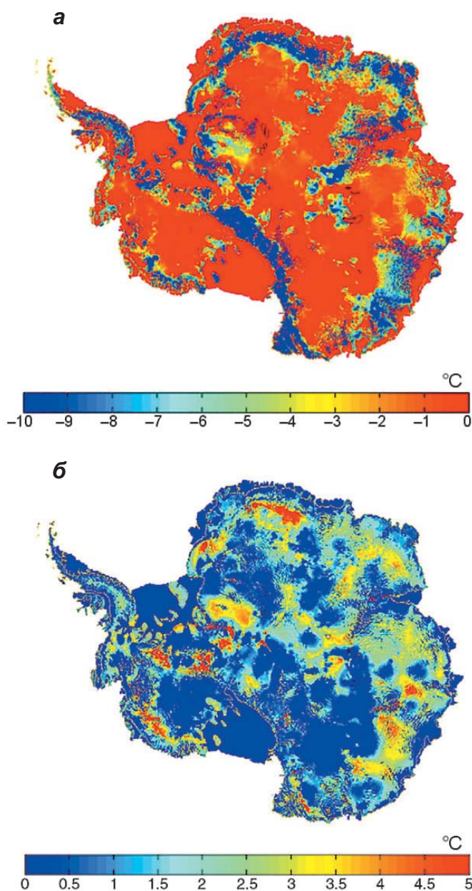
◀ Рис. 4.43. Средняя температура на ложе в °C с поправкой на давление (а); показаны только температуры выше -10 °C. Стандартное отклонение в °C для 24 тестов на чувствительность модели к ошибкам задания входных данных (б). Правдоподобие оценок наличия холодного и теплого ложа: градации шкалы – от синего (холодное ложе во всех тестах) до красного (теплое ложе во всех тестах) (Pattyn, 2010)
