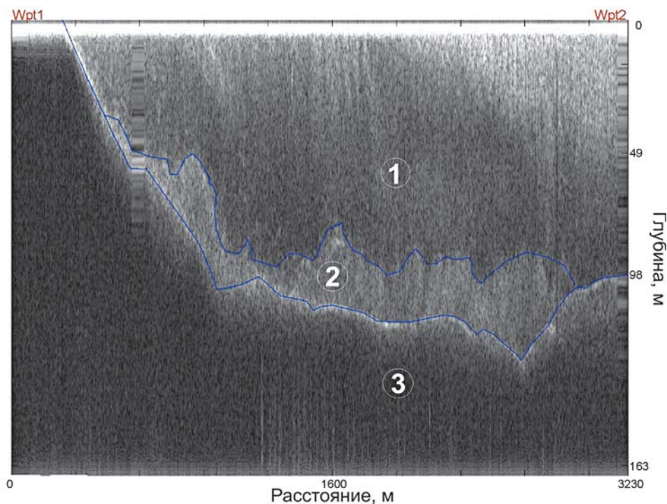
▲ Рис. 3.29. Пример радарной записи, полученной на леднике Тавле с применением шведского лоатора с синтезированной частотой 350 МГц. 1 – слой холодного льда, 2 – слой теплого льда, 3 – отражения от ложа (Лаврентьев и др., 2011)
