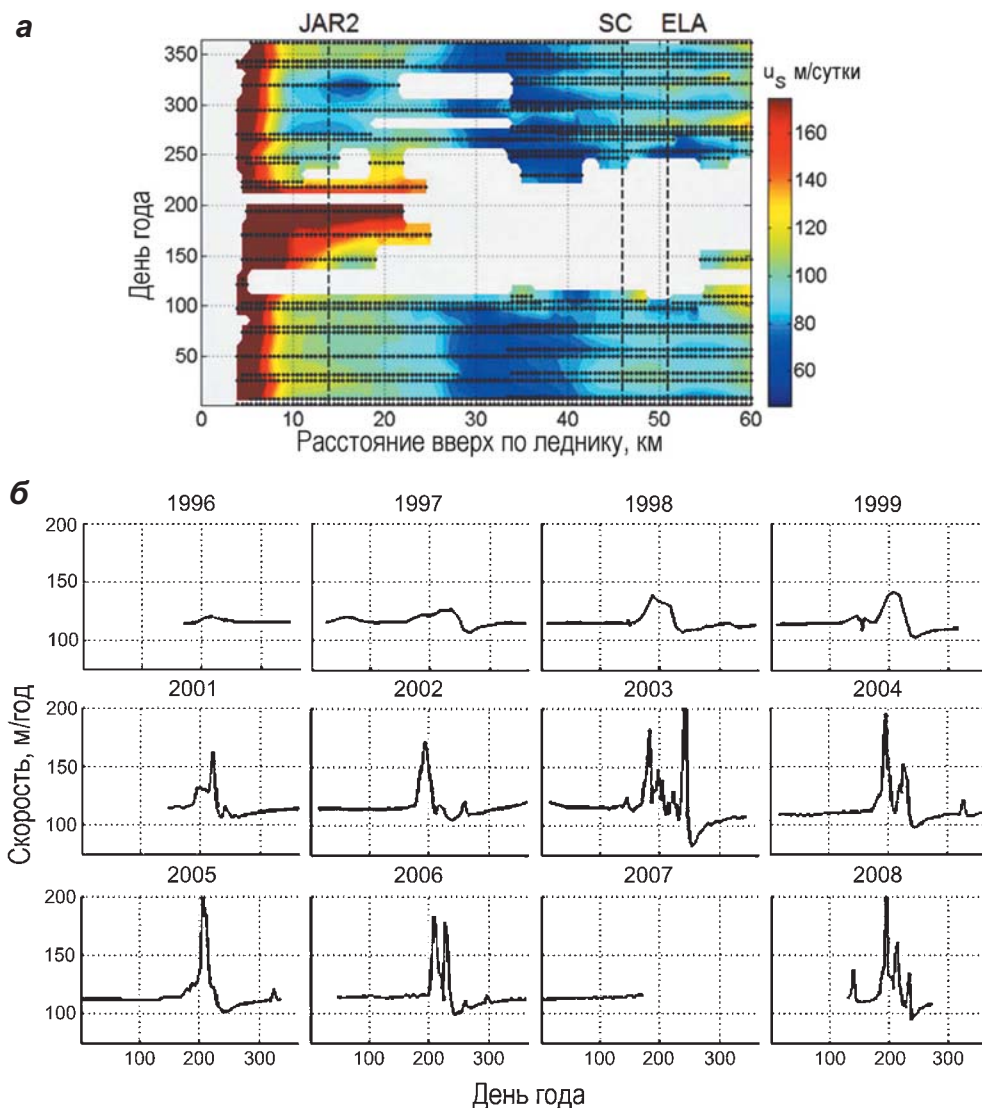
▲ Рис. 4.72. Поверхностные скорости движения (м/год) нижних 60 км ледника Сермек Аван-нарлек в течение года (а); пунктирными линиями отмечены конкретные даты измерения скоростей по данным inSAR, показано также положение станций JAR2, Swiss Camp и границы питания ELA. Скорость движения ледника в районе станции Swiss Camp в 1996–2008 гг. (б) (Colgan et al., 2011)
