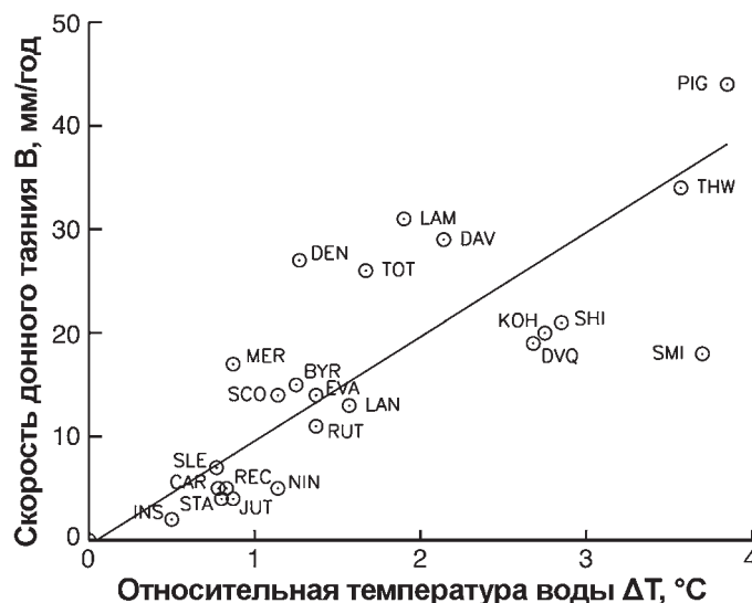
▲ Рис. 2.151. Скорость донного таяния B (мм/год) ниже линии налегания шельфовых и выводных ледников в Антарктиде как функция температуры океанских вод относительно точки замерзания \Delta T на глубине, равной 0,88 от толщины льда на линии налегания (Rignot, Jacobs, 2002)
