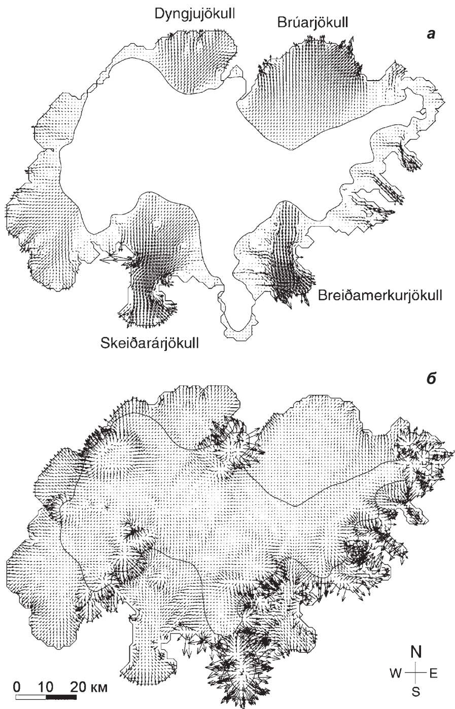
▲ Рис. 4.37. Структура подледникового дренажа ледниковых куполов Dyngjujökull, Brúarjökull, Skeiðarárjökull и Breiðamerkurjökull в Исландии: а) динамическая стационарная модель, б) статическая модель. Векторы параллельны и пропорциональны градиенту потенциала. Тонкой линией показано положение границы питания (Flowers et al., 2003)
