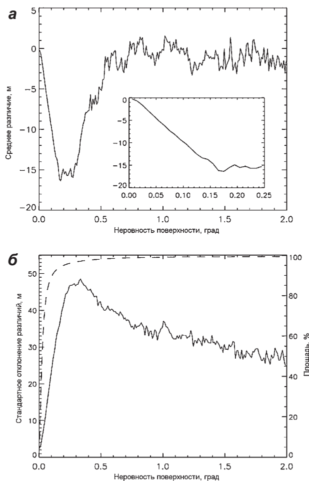
► Рис. 2.125. Среднее различие между высотами поверхности ледникового покрова Антарктиды по данным измерений со спутников ICESat и ERS-1 как функция угла наклона поверхности (а). На врезке показана левая часть графика для углов наклона до 0,25°. Стандартное отклонение от средних значений (сплошная линия) и кумулятивный процент площади ледникового покрова как функция наклона поверхности (пунктирная линия) (б) (Bamber et al., 2009)
