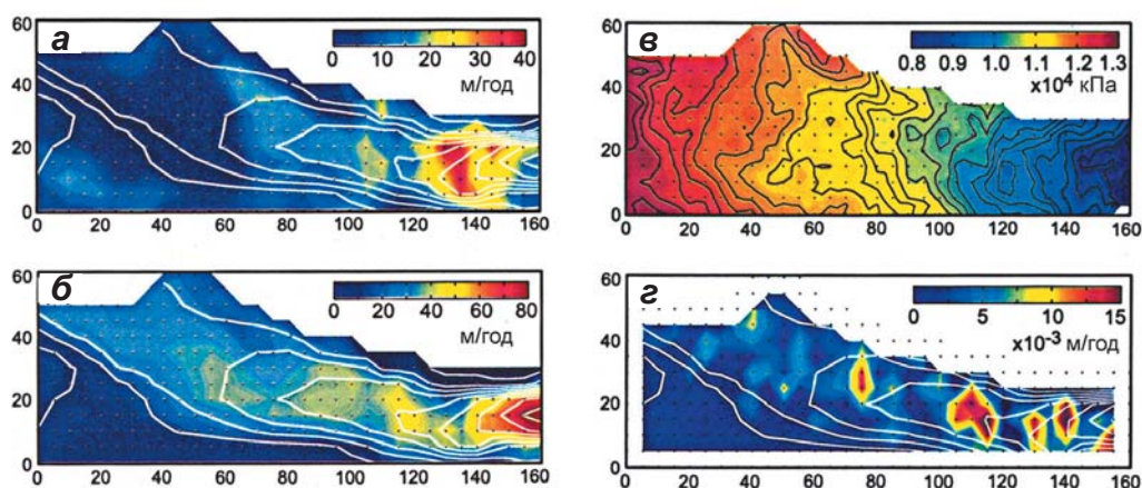
▲ Рис. 4.57. Рассчитанные характеристики ледяного потока D: а) скорость движения за счет деформации льда, м/год; б) скорость донного скольжения, м/год; в) гидравлический потенциал с шагом 20 кПа; г) скорость донного таяния из-за трения на границе лед–ложе (Price et al., 2002)
