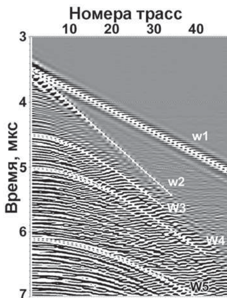
▲ Рис. 3.9. Пример радарных записей, полученных при ОГТ-измерениях на леднике Ханс летом 2003 г. Типы волн: W1 – прямая воздушная волна, W2 – волна, распространяющаяся вдоль поверхности ледника, W3 и W4 – отраженные волны от скопленной воды в слое теплого льда, W5 – отраженная волна от ложа ледника (Яния и др., 2005; Jania et al., 2005)
