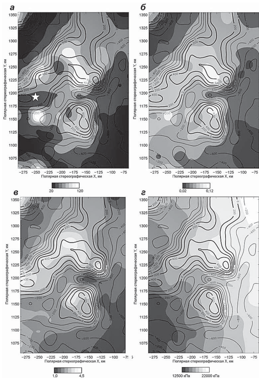
▲ Рис. 2.105. Шероховатость ложа в районе ледника Слессор, оцененная тремя методами: а) по среднеквадратическим (SD) вариациям высоты ложа с разрешением около 60–75 м, путем осреднения по сети 5×5 км; б) по SD вариациям BRP сорт осредненным по сети 5×5 км; в) по длине импульса около 1,12 м, без осреднения. На всех картах шероховатость ложа оконтурена и показана оттенками серого цвета: более светлыми – сглаженные области, более темными – более шероховатые области, топография ложа – изолиниями высот в метрах выше (толстые линии) и ниже (тонкие линии) эллипсоида WGS 84; на (а) звездочка показывает пример района с уменьшенной шероховатостью ложа на отметке – 260 м ниже ур. моря внутри медленно движущейся области между притоками; г) распределение гидравлического потенциала при давлении воды P_w равно давлению P_i вышележащего льда (Rippin et al., 2006)
