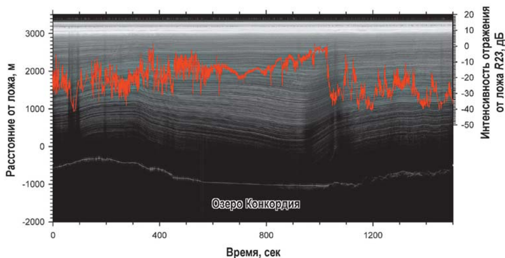
▲ Рис. 4.115. Внутренние отражающие и свободная от радиоэха зона в Восточной Антарктиде в районе озера Конкордия (красной линией показана интенсивность отражения от ложа) (Wright et al., 2012)
