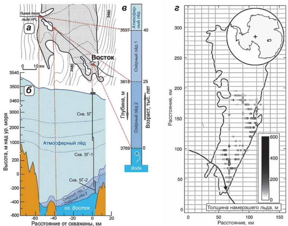
▲ ► Рис. 4.116. Слои озерного льда над южной частью подледникового озера Восток: а) область формирования озерного льда вдоль линии тока VFL, проходящей через скважину 5Г; береговая линия (Masolov et al., 2006); б) разрез по линии тока с указанием положения скважины 5Г и ее боковых стволов 5Г-1 и 5Г-2; в) озерный лёд в скважинах 5Г-1 и 5Г-2, указаны глубина и возраст границ (Salamat et al., 2009); г) толщина слоя намерзшего льда над озером Восток (Tikku et al., 2004); черной линией показана линия тока через станцию Восток; д) содержание \text{Cl}^- и \text{H}^+ во льду (Angelis et al., 2004); е) интенсивность отражений из слоя намерзшего озерного льда 1, оцененная по ориентировке с-осей кристаллов. Из работ (Липенков и др., 2012) (а-в), (MacGregor et al., 2009) (г-е)
