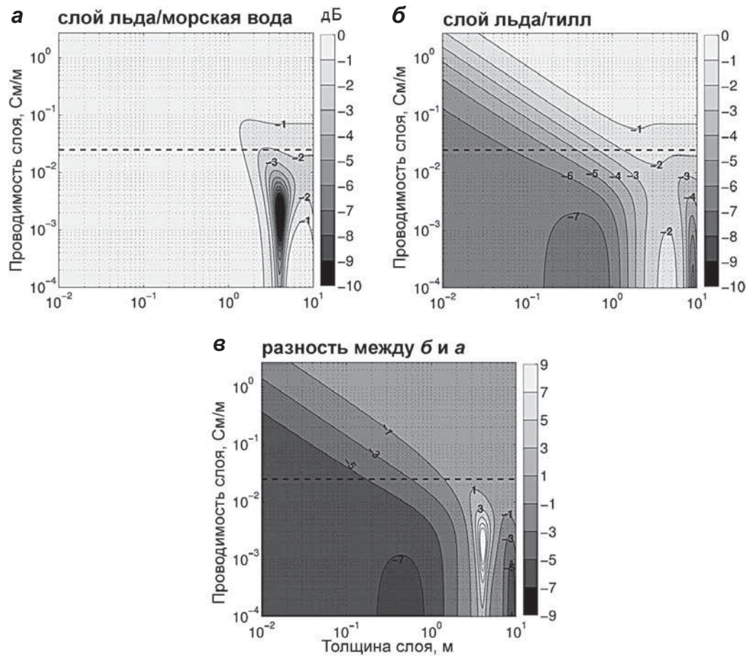
▲ Рис. 2.82. Коэффициент отражения, дБ (изолинии и черно-белая шкала) от границы раздела лед-морская вода (а) и лед-тилл (б) как функция толщины слоя, м (нижняя шкала) и проводимости, См/м (левая шкала); в) разность между (б) и (а). Горизонтальная пунктирная линия – проводимость воды под ледяным потоком В по данным (Engelhardt et al., 1990) (McGregor et al., 2011)
