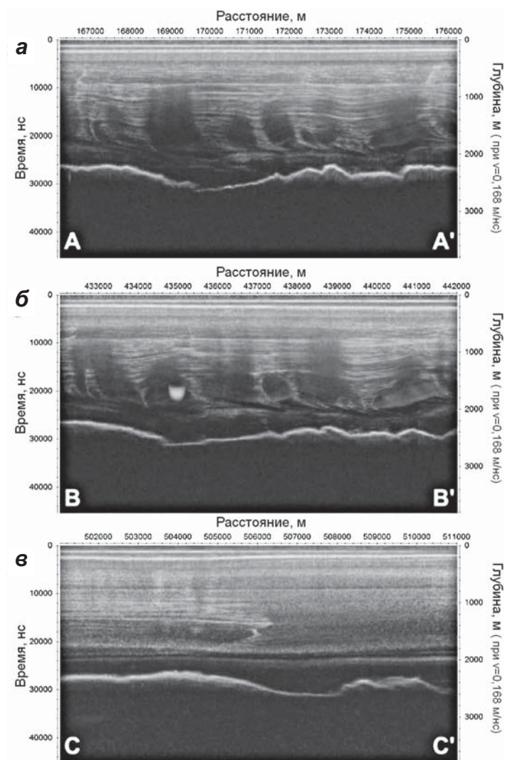
► ▼ Рис. 4.110. (а-в) Радарные отражения от подледникового озера Институт Е2 вдоль профилей (см. рис. 4.109); (г) интенсивность отражений от ложа, дБ вдоль этих же профилей (цветная шкала) и гидравлический потенциал (цветная шкала) в районе озера (его границы показаны белой пунктирной линией) (Siegert et al., 2013)
