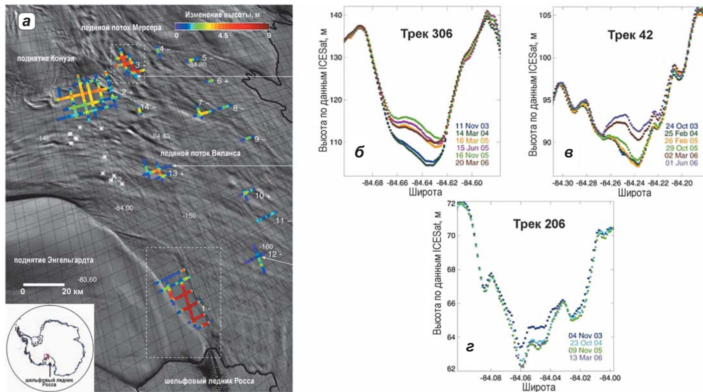
▲ Рис. 4.91. Участки на ледяных потоках Виланса (В) и Мерсера (А), на которых по данным съемки со спутника ICESat с интервалом 91 день в период с 2003 по 2006 г. обнаружены изменения высоты поверхности (а). Черными линиями показаны треки альтиметрии ICESat, цветом – диапазон изменений высоты поверхности. Знаки (+), (–) и (~) обозначают подъем, опускание и осцилляции высоты поверхности. Общее движение ледника направлено слева направо в сторону линии налегания, отмеченной толстой черной линией. Белые звездочки показывают места небольших проседаний поверхности на ледяном потоке Виланса в 1987–1988 гг. Изменение высоты поверхности вдоль треков ICESat: 306 (б), 42 (в) и 206 (г) (Fricker et al., 2007)
