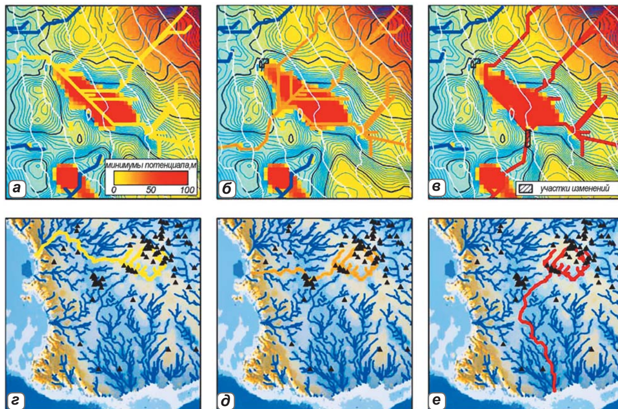
◀ Рис. 4.128. Крупномасштабные перестройки пути стока воды из подледникового трога Адвенчер, которые возникают при малых изменениях ( \pm 10 м) высоты поверхности ледникового покрова на локальных участках (отмечены штриховкой на б и в): а–в) поле гидравлического потенциала, м (цветная шкала) у южной оконечности трога Адвенчер и пути стока подледниковой воды. Красно-желтым цветом выделены локальные минимумы потенциала, где должна скапливаться вода. За их пределы вода начинает перетекать, только достигнув их порога; г–е) общая схема дренажной системы Восточной Антарктиды, где цветом выделены изменения пути стока из трога Адвенчер (Wright et al., 2008)
