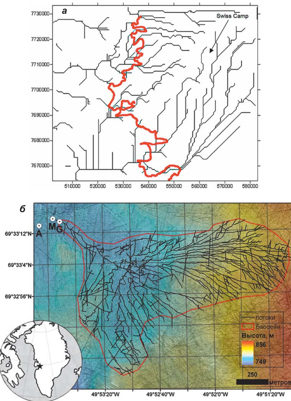
▲ Рис. 2.16. Поверхностная (красная линия) и подледниковая (серые линии) дренажная сеть в районе Паакитсок у западного побережья Гренландии по данным воздушных радио- и DGPS-измерений, позволяющих определить пути течения воды в понижениях поверхности и ложа (а) (Motttram et al., 2009) и сеть поверхностных водотоков в дренажном бассейне в 6 км от края ледникового покрова на западе Гренландии, определенная по снимку ASTER от 15 июля 2009 г. (б) (McGrath et al., 2011)
