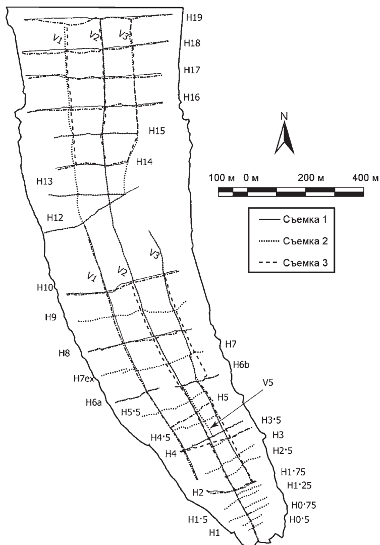
▲ Рис. 4.11. Повторные радарные съемки с 50 МГц локатором на политермическом леднике Стагнейшн (о. Байлот, Канада) в июне–августе 2002 г. (Irvine-Fynn et al., 2006)
