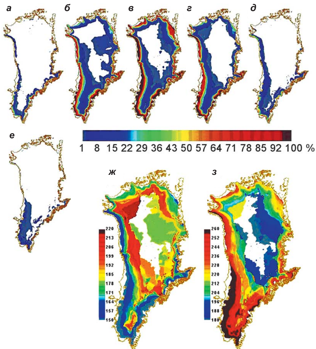
▲ Рис. 2.12. Среднее месячное распространение таяния и его вероятность (%) в мае (а), июне (б), июле (в), августе (г), сентябре (д) и октябре (е); средние даты начала таяния (ж) и даты замерзания (з) (дни года в период с 2000 по 2004 гг.). Белым цветом показаны области, не испытывавшие таяния в эти месяцы и годы (Wang et al., 2007)
