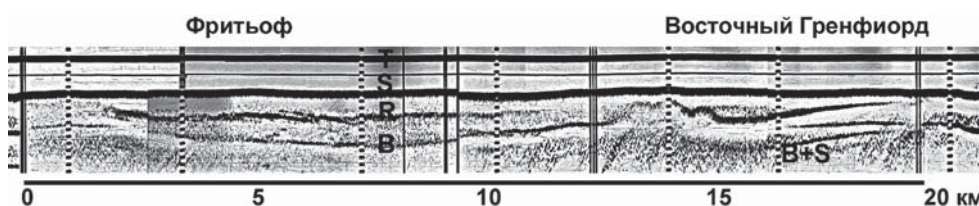
▲ Рис. 2.30. Отражения от внутреннего отражающего горизонта (R) и от ложа (B) ледника Фритьоф по данным аэрорадиозондирования на частоте 620 МГц. Т – зондирующий импульс, S – отражения от поверхности, B – отражения от ложа, B + S – двукратные отражения от ложа (Мачерет и др., 1992)
