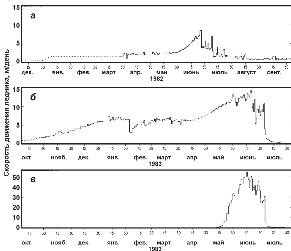
▲ Рис. 1.19. Скорость движения ледника Вариегейтед на Аляске до, во время и после его подвижки в 1982–1983 гг.: в верхних 8 км ледника (а, б), в 15 км от верховьев или в 4–5 км от фронта (в) (Kamb et al., 1985)
