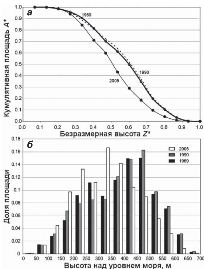
► Рис. 3.20. Гипсометрические кривые ледника Фритьоф в разные периоды времени (1969, 1990 и 2005 гг.) как функция A^* и Z^* – безразмерной площади и высоты поверхности (см. Furbish, Andrews, 1984), где A^* – кумулятивная площадь выше определенной высоты Z^* (равна нулю на краю и единице на самых больших высотах ледника) (а); доля площади в те же годы в разных высотных зонах (б) (Murray et al., 2012)
