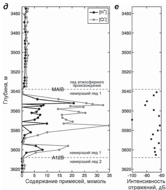
▲ ► Рис. 4.116. Слои озерного льда над южной частью подледникового озера Восток: а) область формирования озерного льда вдоль линии тока VFL, проходящей через скважину 5Г; береговая линия (Masolov et al., 2006); б) разрез по линии тока с указанием положения скважины 5Г и ее боковых стволов 5Г-1 и 5Г-2; в) озерный лёд в скважинах 5Г-1 и 5Г-2, указаны глубина и возраст границ (Salamat et al., 2009); г) толщина слоя намерзшего льда над озером Восток (Tikku et al., 2004); черной линией показана линия тока через станцию Восток; д) содержание \text{Cl}^- и \text{H}^+ во льду (Angelis et al., 2004); е) интенсивность отражений из слоя намерзшего озерного льда 1, оцененная по ориентировке с-осей кристаллов. Из работ (Липенков и др., 2012) (а-в), (MacGregor et al., 2009) (г-е)
