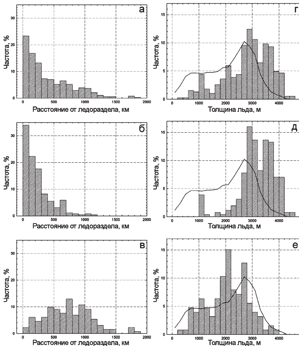
▲ Рис. 4.87. Гистограммы распределения подледниковых озер в Антарктиде в зависимости от расстояния вдоль линии тока от основного ледораздела (левый столбец) и в зависимости от толщины перекрывающего льда (правый столбец): для всех известных подледниковых озер (а, г), для озер, идентифицированных по данным радиозондирования (б, д), для озер, идентифицированных по спутниковым измерениям вертикального движения поверхности ледникового покрова (в, е). Для сравнения черной линией показано распределение толщины льда для всего ледникового покрова Антарктиды (Wright, Siegert, 2010)
