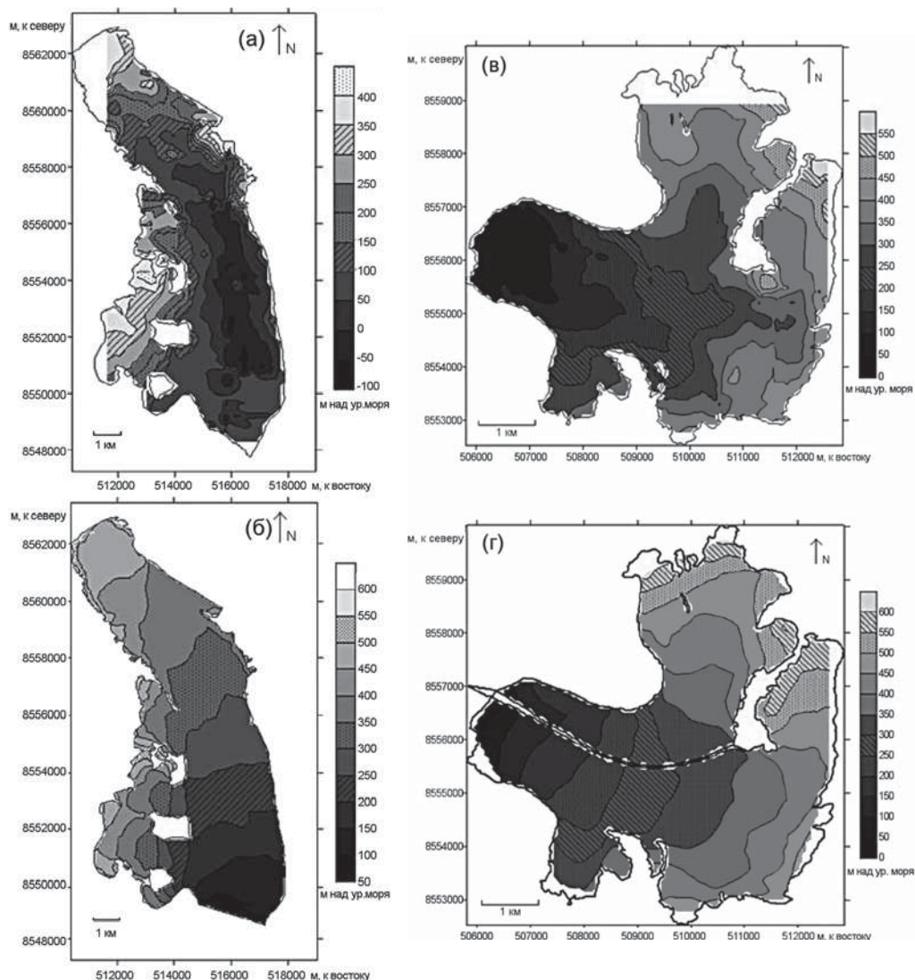
▲ Рис. 4.29. Ледник Ханс: а) ЦМР ложа, б) ЦМР поверхности; ледник Вереншельд: в) ЦМР ложа, г) ЦМР поверхности, где показана моренная гряда между ледником Вереншельд на юге и ледником Скилриг на севере (Pälli et al., 2003)
