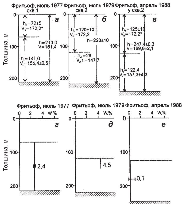
▲ Рис. 3.15. Сезонные и годовые изменения скорости V распространения радиоволн (а–в) и содержания воды W (г–е) в леднике Фритьоф в 1977–1988 гг. (Глазовский, Мачерет, 2007)
