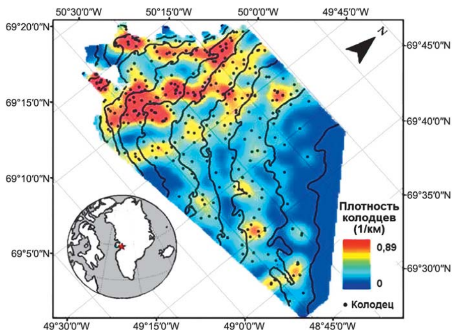
▲ Рис. 2.17. Плотность ледниковых колодцев в интервале высот от уровня моря на западе до 1100 м на востоке в районе ледника Якобсхавн (Colgan, Steffen, 2009)
