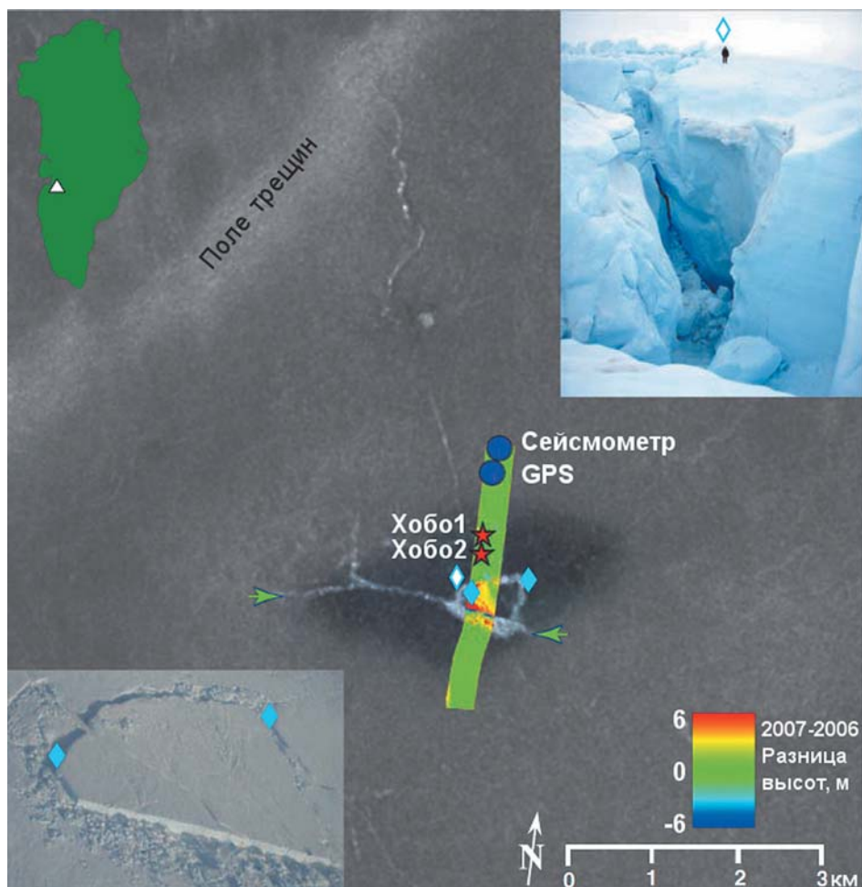
▲ Рис. 2.23. Положение озера (обозначено голубым цветом) 29 июля 2006 г. Красные звездочки и синие кружки показывают места измерений уровня воды в озере и GPS и сейсмометрических измерений. Поднятие блока льда (слева внизу), которое было обнаружено по разнице высот (цветная шкала) при лазерной альтиметрии с самолета (ATM) в мае 2006 и 2007 гг. Крупное нарушение, видимое на SAR снимке, выглядит как длинная полоса (отмечено зелеными стрелками). Сплошные голубые ромбы обозначают места, где ATM измерения показали крупные отверстия на дне озера в 2006 г. Вверху справа показано отверстие после дренирования озера в 2007 г. (Das et al., 2008)
