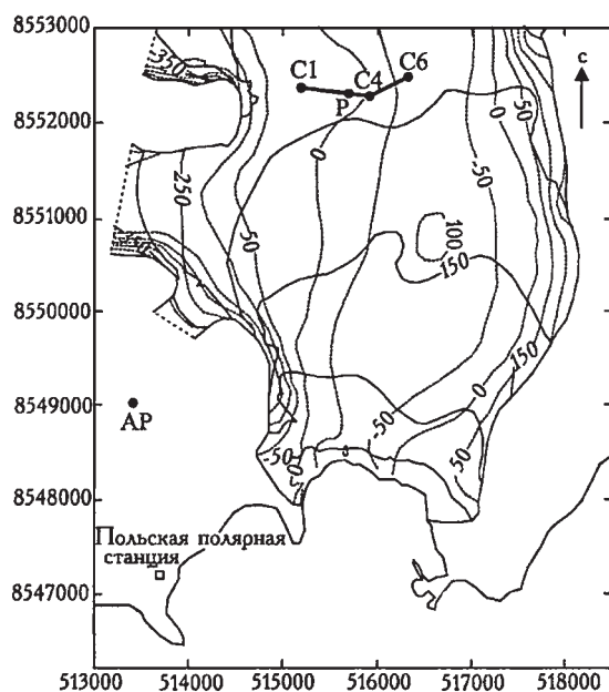
◀ Рис. 3.3. Радиолокационные и радиофизические исследования на леднике Ханс в 2003 и 2004 гг. С1–С6 – поперечный профиль, где в период таяния с 17 июля по 4 августа 2003 г. проводились повторные измерения, С4 – центральная точка ОГТ-измерений, Р – положение автоматической метеостанции, DGPS-приемника и радарных измерений в фиксированной точке в период таяния с 25 июля по 1 августа 2003 г. (Яния и др., 2005; Jania et al., 2005)
