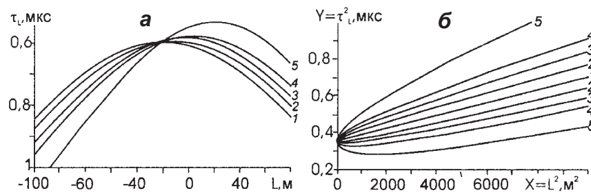
▲ Рис. 2.47. Квадратические (а) и линейные (б) годографы отраженной волны от наклонного линейного отражателя, рассчитанные по формуле (2.57) как функция расстояния L от точки перенесения профиля зондирования с проекцией отражателя на поверхность ледника (вершины гиперболы) для разных углов \beta наклона отражателя: ( h_o = 50 м, V = 168 м/мкс, \beta = 0^\circ ): \beta = 0^\circ (1), \beta = 5^\circ (2), \beta = 10^\circ (3), \beta = 15^\circ (4), \beta = 30^\circ (5) (Мачерет, 2000)
