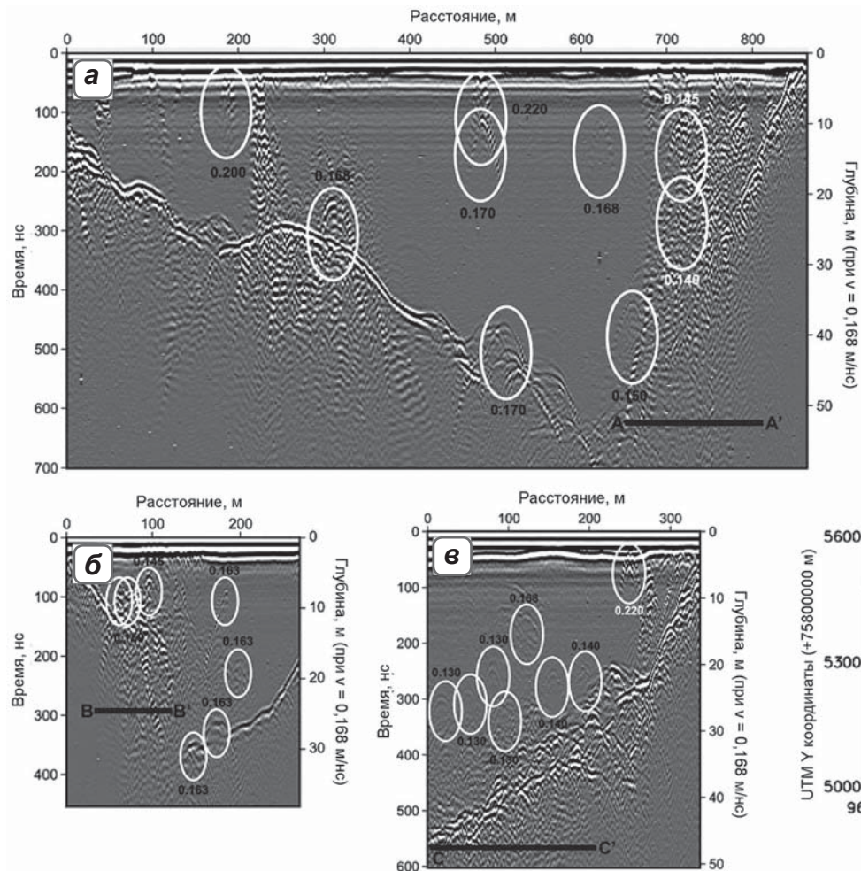
◀ ▼ Рис. 4.25. Внутреннее строение ледника Карса в северной Швеции по данным радиозондирования 2009 г. на частоте 50 МГц; радарные записи с интенсивным внутренним рассеянием: а) профиль А–А'; б) профиль В–В'; в) профиль С–С'; г) положение этих профилей на леднике; белыми эллипсами на (а–в) выделены гиперболические отражения, по которым оценена скорость распространения радиоволн в леднике, м/нс (черные цифры) (Rippin et al., 2011)
