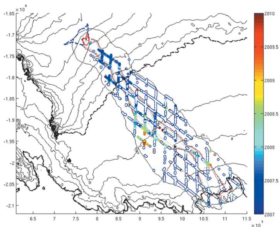
▲ Рис. 2.133. Даты начала заполнения подледниковых емкостей в гидрологически связанной области по пути стока озера Кука Е2. Изогипсами (через 400 м до 2000 м и через 50 м выше) показана высота поверхности ледникового покрова Голубым пунктирным контуром показан водосбор подледникового озера, красным – края самого озера (Flament et al., 2011)
