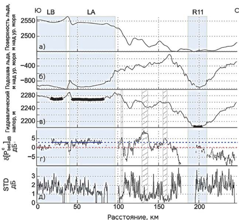
▲ Рис. 2.131. Высота поверхности (а) и ложа (б), м; в) гидравлический напор, м; радарные характеристики трех подледниковых озер LA, LB и R11 вдоль профилей зондирования, показанных черной линией на рис. 2.130, а: отклонение мощностей отражений от ложа ( P_{bed}^c ), дБ от регионально предсказанных величин (г), их средние квадратические изменения (STD), дБ (д); серые области показывают ранее предполагавшиеся по данным лазерной альтиметрии со спутника ICESat границы озер (Bell et al., 2007; Smith et al., 2009); в) участки, пересекающие однородные локальные минимумы (+3 м) гидравлического напора h (подчеркнуты черной линией); г) красные и синие сплошные и пунктирные линии показывают мощности отражения, осредненные по участкам над озером R11, над западным краем озера LB и центральной областью озера LA; заштрихованные столбики показывают внутриозерные участки с мощными отражениями с низким STD (Flament et al., 2013)
