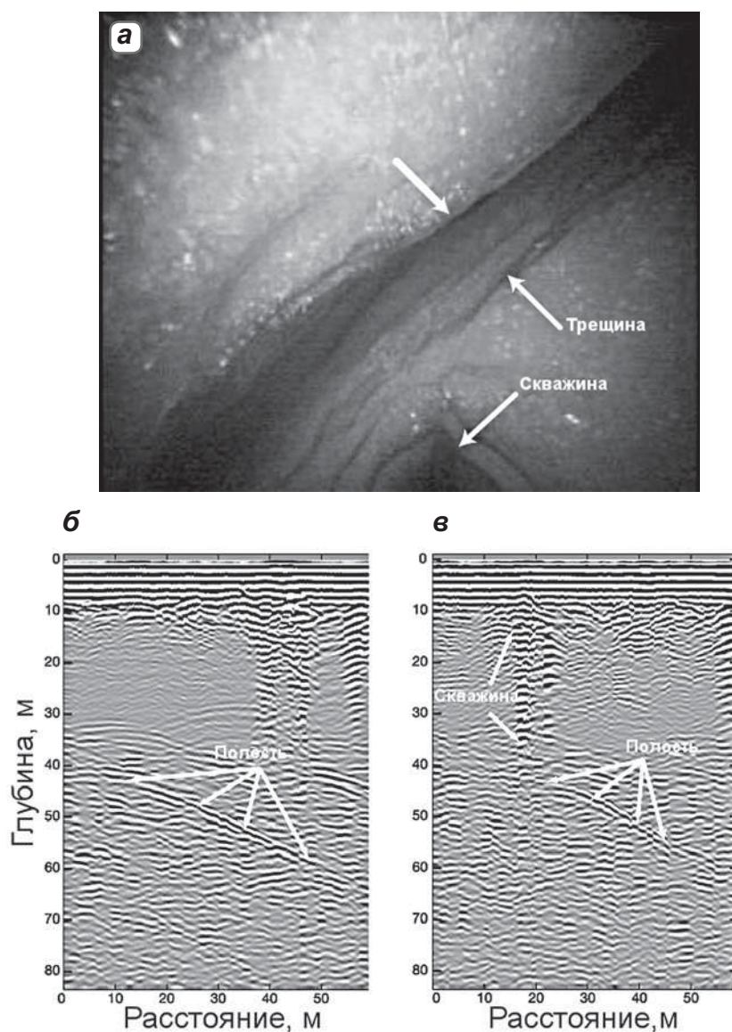
▲ Рис. 2.54. Видеоизображение зоны дробления льда шириной 4 см в одной из скважин, пробуренных в политермическом леднике Стур (Швеция) (а); отражения от внутриледниковой каверны на глубине около 40–50 м по данным радиозондирования на частоте 50 МГц: до бурения скважины горячей водой (б), после пересечения каверны скважиной на глубине 38 м в зоне дробления льда (в) (Fountain et al., 2005)
