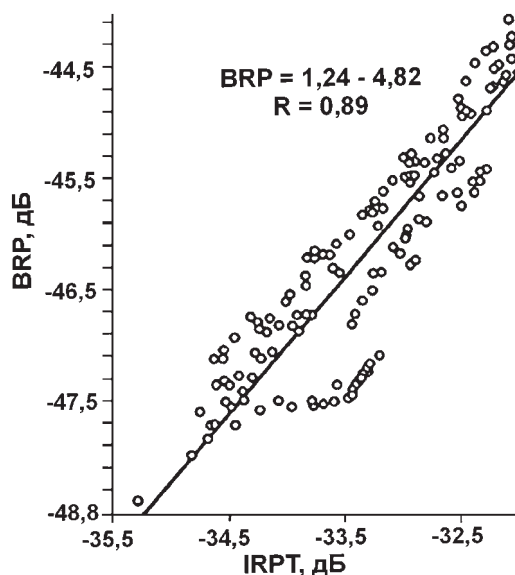
▲ Рис. 3.8. Связь мощности отражений из слоя теплого льда (IRPT) и от ложа (BRP) (Яния и др., 2005)
