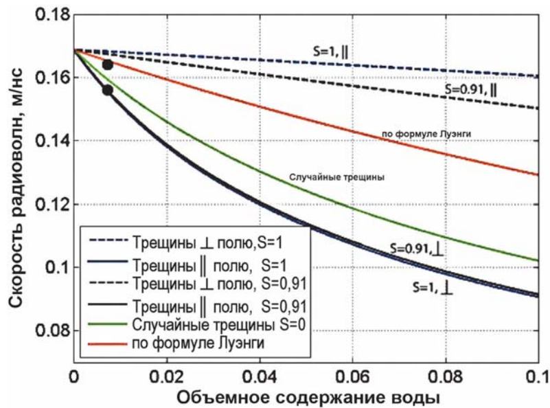
▲ Рис. 2.40. Скорости распространения радиоволн во льду с анизотропным и случайным распределением включений воды, рассчитанные по формулам (2.37)–(2.39) при разной преимущественной ориентации включений относительно направления электромагнитного поля и разных значениях фактора деполяризации S , а также по формуле Луэнги (2.32). Величина S = 0,91 вычислена на основе видеонаблюдений в скважинах на леднике Бенч (Bradford et al., 2013)
