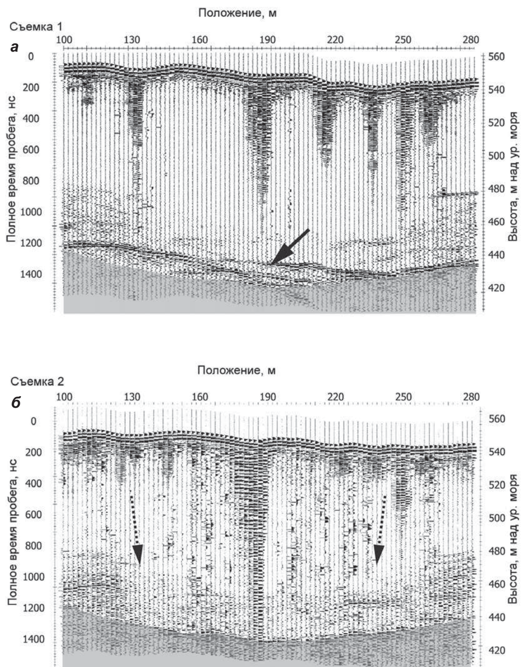
▲ Рис. 4.16. Профиль N19 (см. рис. 4.11). На (а) отражение вблизи ложа (отмечено стрелкой), которое отсутствует на (б); видно также изменение интенсивности отражений (показаны пунктирными стрелками), возможно, из-за начала дренирования теплого льда вблизи центральной линии ледника (Irvine-Fynn et al., 2006)
