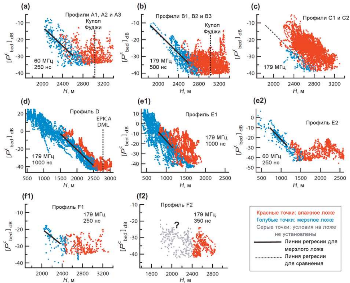
◀ Рис. 2.97. Оцененные по графикам Н-Р влажные (красные точки) и мерзлые (синие точки) условия на ложе на разных участках профилей A1, A2, A3 (a), B1, B2, B3 (b), C1, C2 (c), D (d), E3 (e1), E2 (e2), F1 (f1), F2 (f2); для профиля F2 достоверная оценка не получена (серые точки). Положение профилей показано на рис. 2.96 (Fujita et al., 2012)
