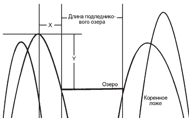
◀ Рис. 4.83. Оценка радарной длины L , подледникового озера и наклона его берегов по гиперболическим отражениям на краях озера. Крутизна берегов Y/X определяется как отношение превышения Y ближайшей гиперболы над озером к расстоянию между ними X (Dowdeswell, Siegert, 1999)
