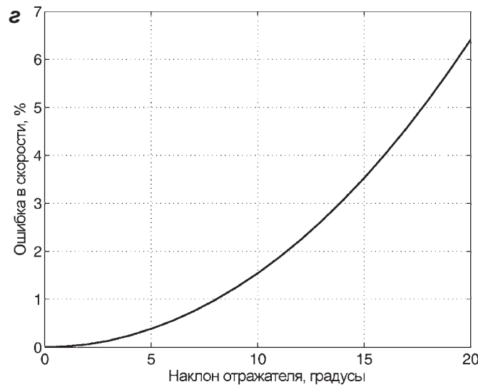
▲ ▲ Рис. 2.53. Ошибки, влияющие на определение скорости распространения радиоволн в ледниках по данным двухпозиционных ОП-измерений: а) форма квадратичного годографа f^2 = f(x^2) при точном определении времени начала зондирующего импульса (толстая линия) и при статической ошибке 10 нс (пунктирная линия) и 100 нс (штриховая линия); б) ошибки в скорости (толстые линии), возникающие из-за неточного определения начала зондирующего импульса (в % по отношению ко времени t_0 ), в зависимости от отношения R ; в) ошибка в скорости, вычисленной по уравнению Дикса (2.55) для модели ледника, состоящего из слоев холодного и теплого льда толщиной по 50 м по отношению к истинной скорости, вычисленной с учетом преломления на границе слоев для той же модели; г) ошибка в скорости за счет наклона отражающей границы (Barrett et al., 2007)
