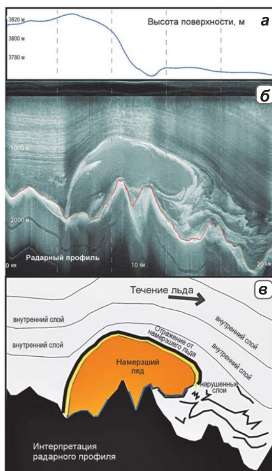
▲ Рис. 4.122. Профиль высоты поверхности ледника в области над пластом намерзшего льда (по данным лазерной альтиметрии) (а); картина радиолокационных отражений на частоте 150 МГц над пластом намерзшего льда толщиной 1100 м (б); на схеме (в) показан изгиб вверх на 410 м внутренних слоев над пластом намерзшего льда (Bell et al., 2011)
