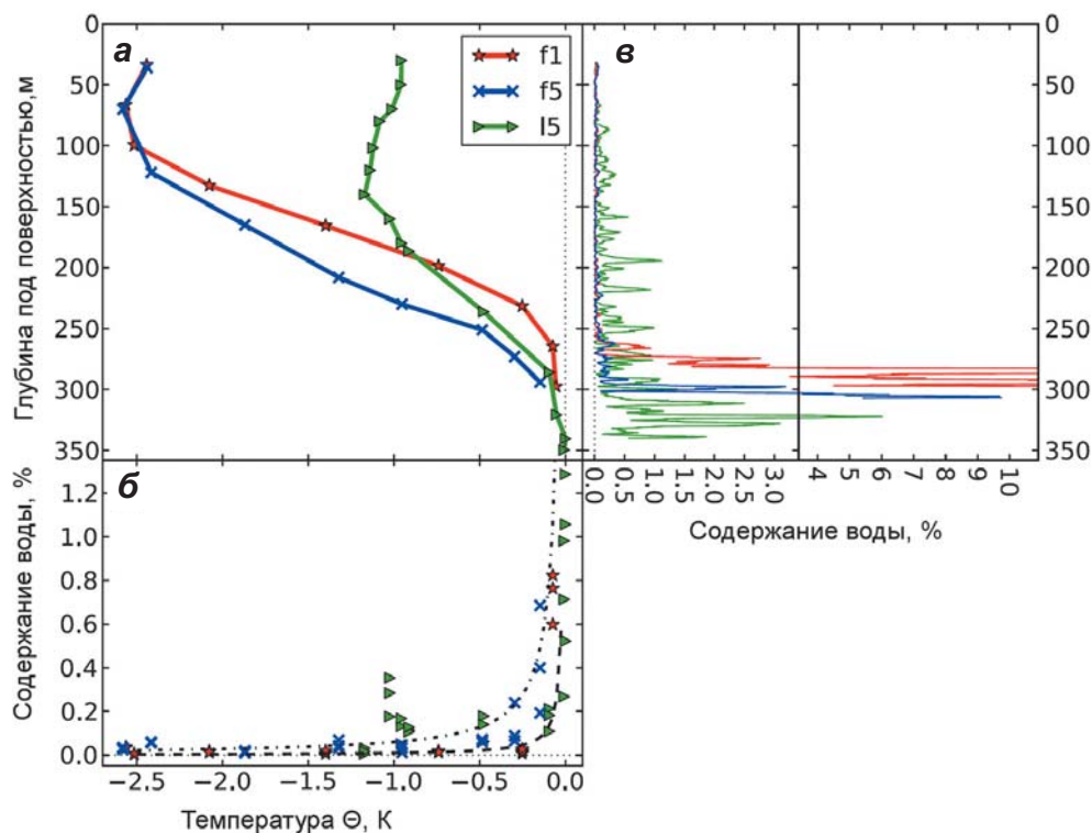
▲ Рис. 4.6. Температура (относительно точки плавления) в леднике по датчикам, установленным в скважинах f1, f3, f5 вблизи радарных профилей D и E (а); содержание воды во льду по радарным данным (б). Оценки сделаны для тех глубин, где измеряли температуру льда. Пунктирные кривые показывают теоретически возможное содержание воды во льду (см. формулу (4.1)) в зависимости от температуры и константы C' (от 0,01 до 0,05). Рассчитанное распределение воды с глубиной вблизи скважин (в) (Ryser et al., 2013)
