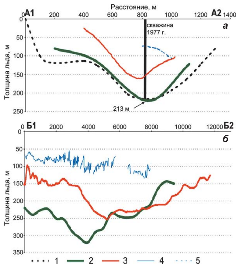
▲ Рис. 3.14. Изменение толщины и гидротермической структуры ледника Фрит'оф на поперечном профиле в районе ледораздела (а) и на продольном профиле (б) с 1977 по 2005 г. (Василенко и др., 2006)
