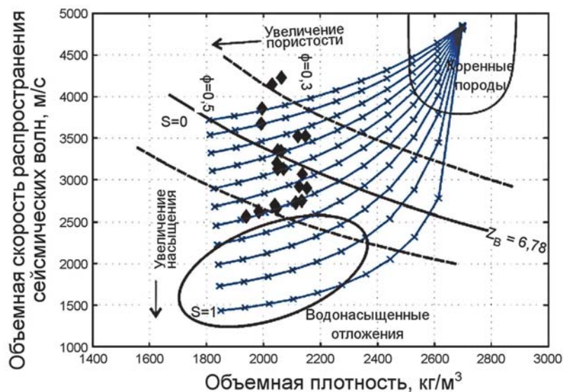
▲ Рис. 2.122. Акустический импеданс ложа Z_b ( 10^6 \text{ кг·м}^{-2}\text{·с}^{-1} ) ледника Ловен Средний как функция скорости (м/с) и плотности ( \text{кг/м}^3 ) для пород ложа и водонасыщенных отложений. Сплошная линия вычислена по сейсмическим данным вдоль профиля LONG с Z = 6,78 \cdot 10^6 \text{ кг·м}^{-2}\text{·с}^{-1} , пунктирные линии показывают диапазон неопределенности \pm 1,53 \cdot 10^6 \text{ кг·м}^{-2}\text{·с}^{-1} ; показаны также типичные соотношения скорости и плотности для ложа, мерзлоты (ромбы) и насыщенного водой тилла по данным разных авторов; синие линии показывают рассчитанные значения скорости и плотности для трехкомпонентной смеси изо льда, воды и пород (Zimmerman, King, 1986) при постоянном насыщении S с шагом 0,1; точки пресечения показывают пористость \phi с шагом 0,05 в диапазоне от 0 до 0,5 (King et al., 2008)
