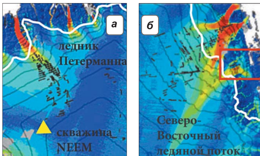
▲ Рис. 4.46. Поверхностная скорость по данным спутниковой радиоинтерферометрии в районе ледника Петерманн (а) и ледяного потока Северо-Восточный (б) на севере Гренландии, где по данным радизондирования 2010 г. на частоте 150 МГц обнаружены участки с признаками намерзания льда вблизи ложа (обозначены черными линиями и точками). Из презентации (Abdi et al., 2011)
