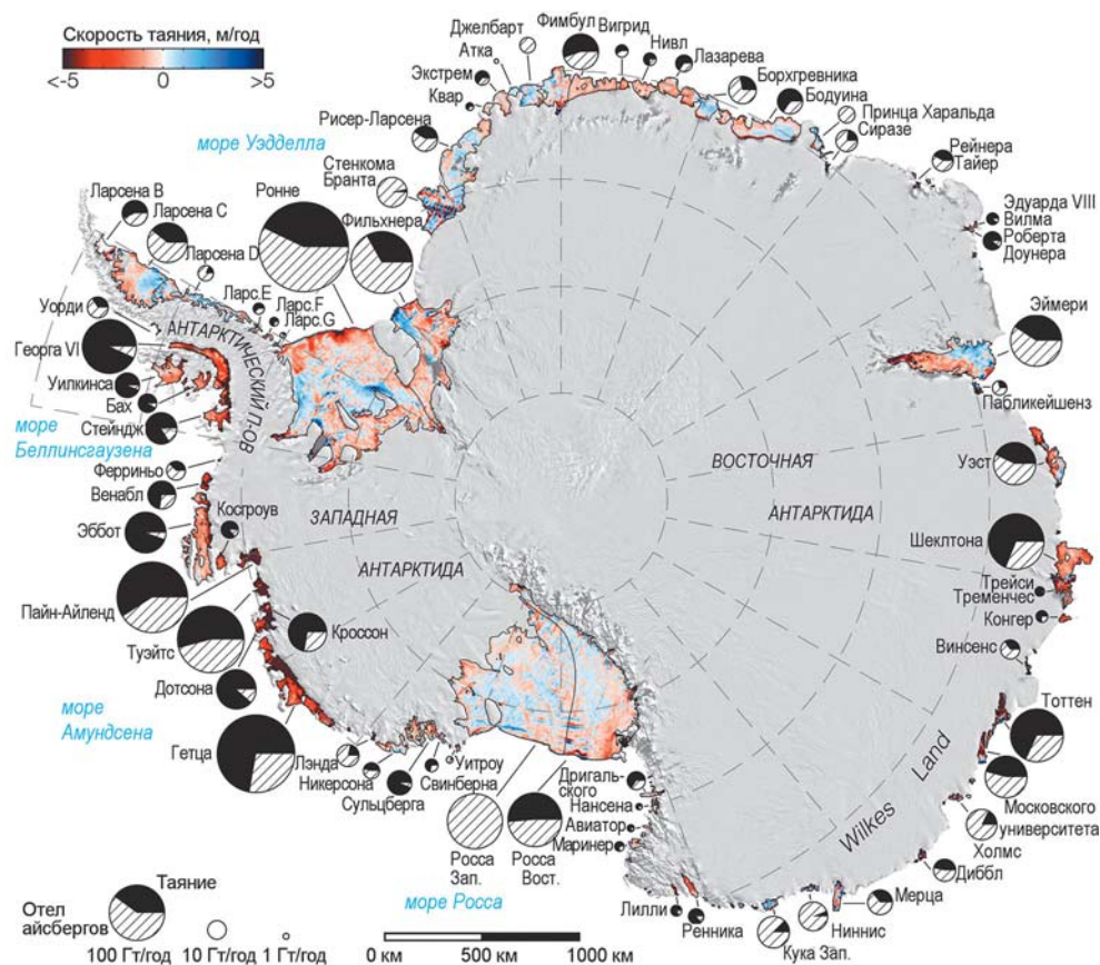
▲ Рис. 4.47. Скорости донного таяния-намерзания (цветная шкала, от -5 до +5 м/год) шельфовых ледников Антарктиды. Круговые диаграммы показывают общие потери для каждого шельфового ледника (Гт/год) и долю в них откола айсбергов (заштрихована) и донного таяния (показана черным цветом). Периметр шельфовых ледников в 2007–2008 гг. обозначен тонкими черными линиями, за исключением ледяных поднятий и островов (Rignot et al., 2013)
