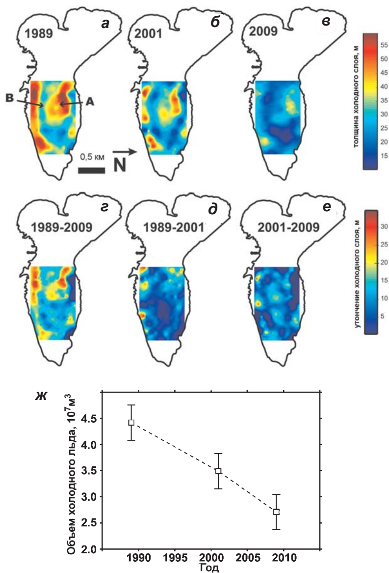
▲ Рис. 4.22. Сокращение толщины слоя холодного льда в области абляции ледника Стур в 1989 (а), 2001 (б), 2009 (в), 1989–2009 (г), 1989–2001 (д), 2001–2009 гг. (е); изменение объема слоя холодного льда с 1989 по 2010 г. (ж); вертикальные линии показывают ошибки вычисления объема льда в предположении, что толщина льда измерена с ошибкой \pm 3 м, включающей ошибки привязки профилей радарных измерений и обнаружения поверхности раздела холодного и теплого льда (CTS) (Gusmeroli et al., 2012)
