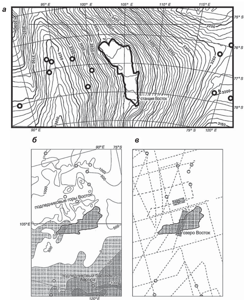
▲ Рис. 4.89. Топография поверхности и ложа и положение подледниковых озёр (показаны кружками) в районе поднятия В: а) топография поверхности по данным спутниковой радиоальтиметрии (Siegert, Ridley, 1998); б) топография подледного ложа с изолиниями через 500 м; в) профили аэрорадиозондирования, использованные для картирования положения подледниковых озёр (Dowdeswell, Siegert, 2002)
