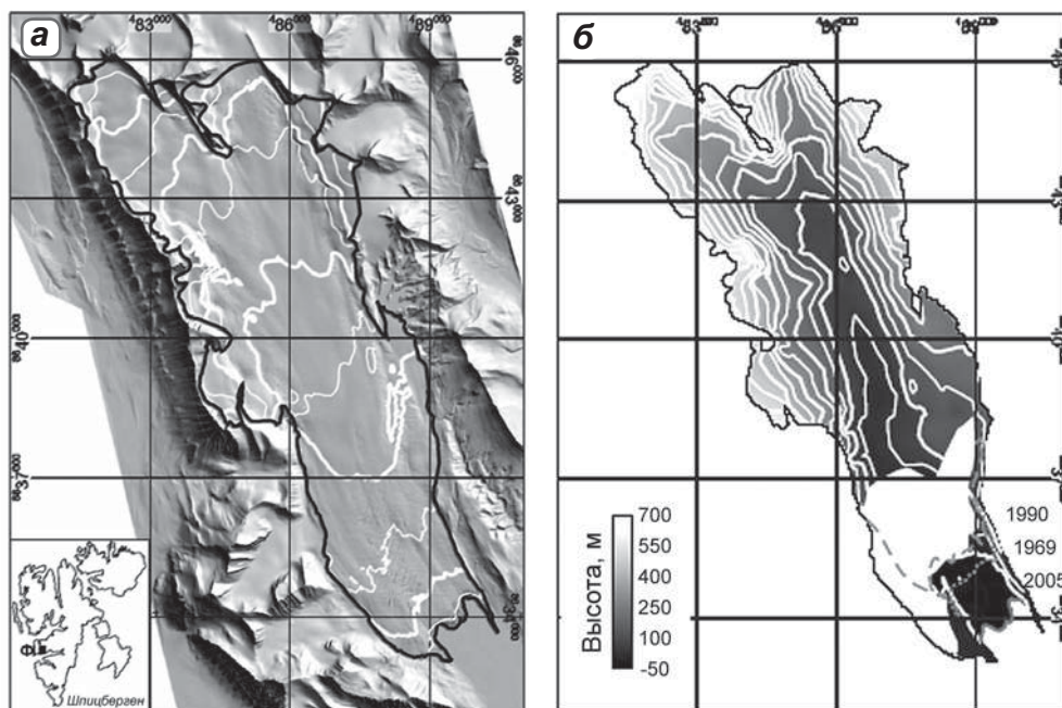
▲ Рис. 3.17. Цифровая модель рельефа (ЦМР) поверхности ледников Фритьоф (FJ), Грёнфьорд Западный и Восточный (G) в границах 2005 г. (а) (показаны черной линией) по данным воздушных лидарных измерений 2005 г.; пунктиром показано положение радарного профиля (см. рис. 3.19), черными линиями – край ледника Фритьоф в 1936, 1969, 1990 и 1998/1999 гг. по топографическим картам и аэроснимкам, в 1860–1861 гг. – по реконструированным картам (Lønne, 2006). ЦМР ложа ледника Фритьоф по данным наземного радиозондирования 1988 г. (б), изогипсы проведены через 50 м (Глазовский, Москалевский, 1989; Глазовский и др., 1991; Лаврентьев, 2008; Glazovsky et al., 1991). В нижней части толщина ледника не была измерена (белый участок). Показано положение края ледника в 1990, 1969 и 2005 гг. (зеленая, синяя и красная линии) (Murray et al., 2012)
