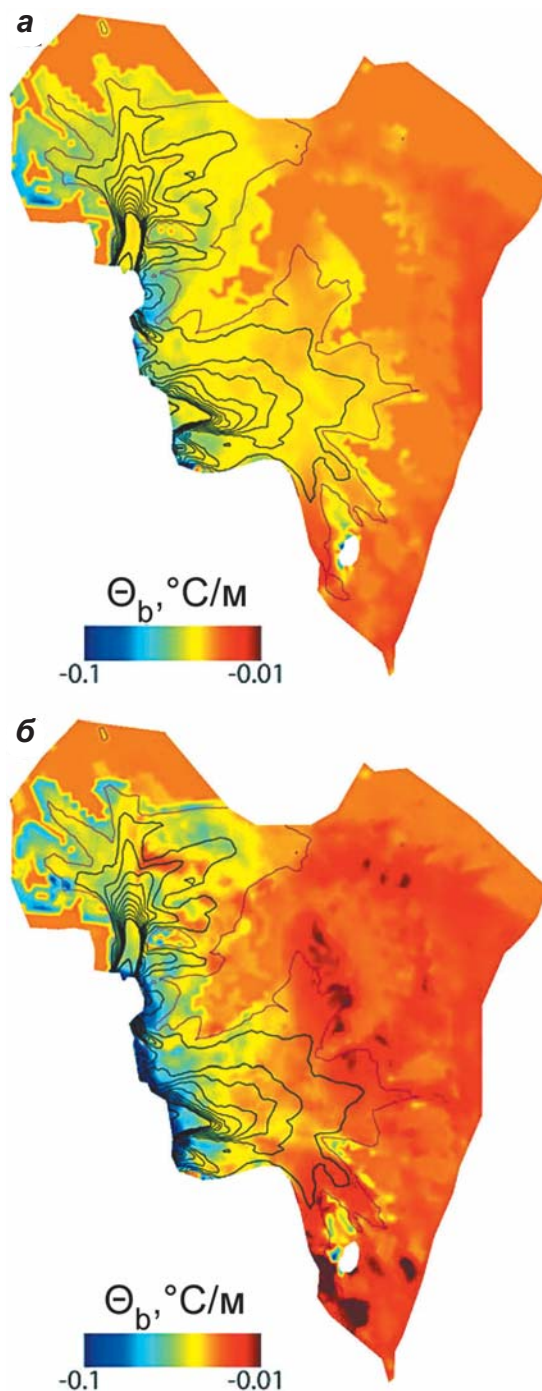
▲ Рис. 4.51. Модельный градиент температуры у ложа ледников Пайн Айленд и Туейтс с пренебрежением малой горизонтальной адвекцией (а) и включая горизонтальную адвекцию (б). Показаны изолинии скорости от 50 до 1000 м/год (Joughin et al., 2009)
