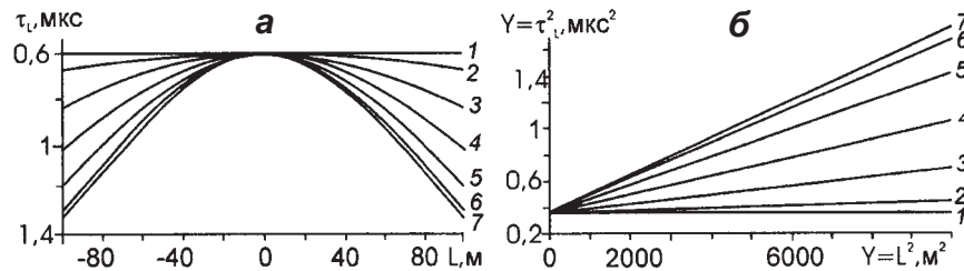
▲ Рис. 2.46. Квадратические (а) и линейные (б) годографы отраженной волны от линейного горизонтального отражателя на глубине h во льду, рассчитанные по формуле (2.56) как функция расстояния L от точки перенесения профиля зондирования с проекцией отражателя на поверхность ледника (вершины гиперболы) для разных углов \alpha между профилем измерений и отражателем ( h = 50 м, V = 168 м/мкс): \alpha = 0^\circ (1), \alpha = 15^\circ (2), \alpha = 30^\circ (3), \alpha = 45^\circ (4), \alpha = 60^\circ (5), \alpha = 75^\circ (6), \alpha = 90^\circ (7) (Мачерет, 2000)
