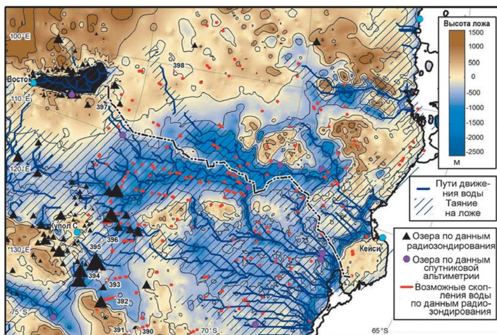
▲ Рис. 4.111. Современные представления о подледниковой гидрологии области бассейна Аврора (топография ложа отображена градациями цвета). Показаны все идентифицированные подледниковые озера (треугольники) и все места, где были зафиксированы изменения высоты поверхности, вероятно, связанные с перемещением подледниковых вод. Красным цветом обозначены места скопления подледниковых вод, установленные по данным радиолокации, но не полностью соответствующие критериям идентификации их как озер. В областях таяния на ложе (штриховка) показана гидрологическая сеть (синие линии) (Wright et al., 2012)
