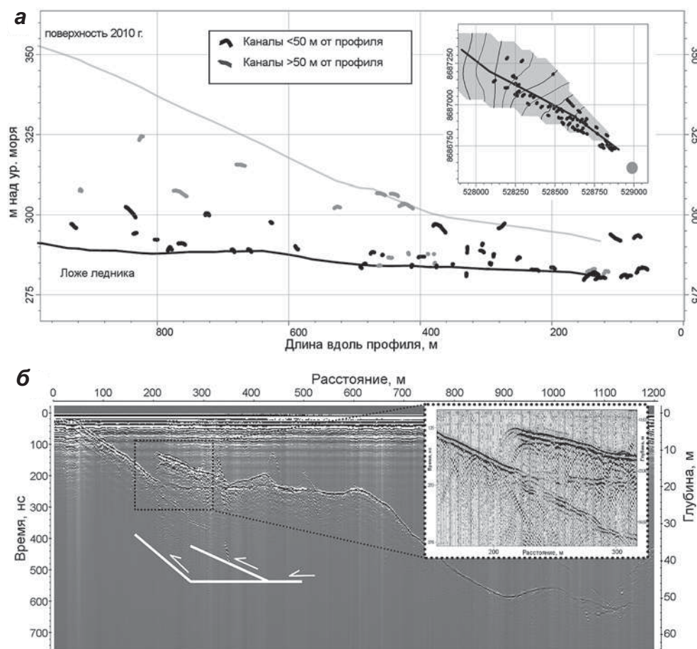
▲ Рис. 2.64. Внутриледниковые и подледниковые каналы в нижней части ледника Телл на Шпицбергене, идентифицированные по данным радиозондирования на частоте 100 МГц на расстоянии <50 м и >50 м от профилей измерений; положение профилей и каналов показано на врезке (а). Строение ледника Телл по данным радиозондирования на частоте 100 МГц вдоль продольного профиля (б). Получены также отражения от надвиговых дислокаций или слоя мореносодержащего льда (Vælum, Benn, 2010)
