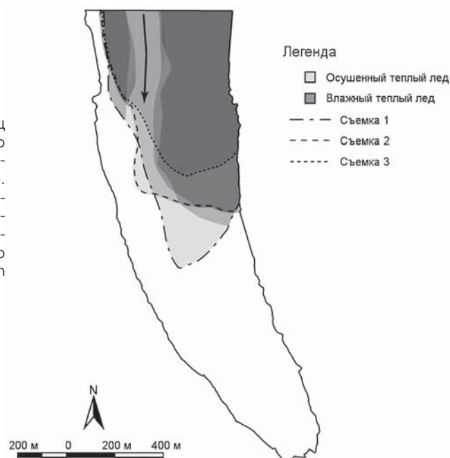
► Рис. 4.17. Изменения границ (пунктирная линия) зоны теплого льда за период между съемками 1, 2 и 3 (июнь–август 2002 г.). Относительно устойчивая область «дренируемого теплого льда» показана светлым тоном, области «влажного теплого льда» – более темным (Irvine-Fynn et al., 2006)
