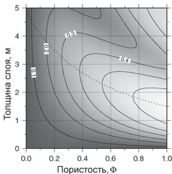
► Рис. 2.80. Интенсивность отражений R от придонного слоя водосодержащего льда как функция его пористости \Phi (содержания воды W во льду) и толщины этого слоя h , м. Точечная линия показывает максимумы интенсивности отражения R_{\max} (Pattyn et al., 2003)
