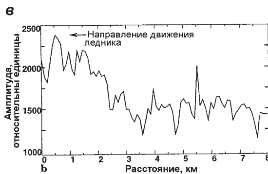
► Рис. 2.142. Линия налегания в районе слияния ледяных потоков D и E вдоль профиля В (а); (б) высота поверхности и глубина ложа (сплошные линии) по данным наземного радиозондирования на частоте 2 МГц и гидростатическая поверхность (штриховая линия), соответствующая условию всплывания ниже линии налегания (0,9 толщины льда); (в) амплитуда отраженных от ложа сигналов вдоль этого профиля (Jacobel et al., 1994)
