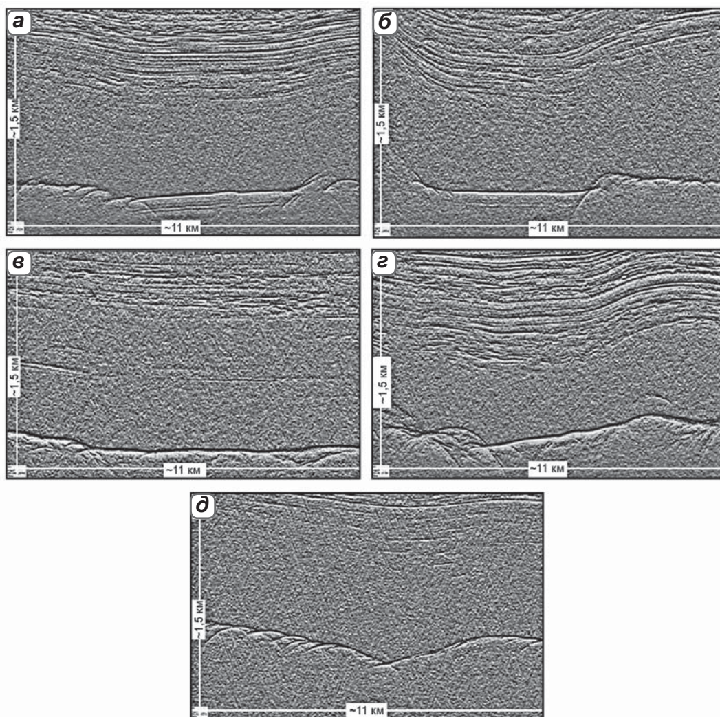
▲ Рис. 4.77. Примеры радарных записей, иллюстрирующие классификацию подледниковых озер Антарктиды по характеру и интенсивности радарных отражений: а) озеро 103 в бассейне Уилкса по каталогу (Siegert et al., 2005) как пример озера категории (1); б) озеро категории (2) в том же бассейне похоже на озеро категории (1), но коэффициент отражения приблизительно на 10 дБ меньше расчетного значения; в, г) два озера категории (3) в окрестности подледникового желоба Адвенчер отдаленно напоминают озера категории (1), высокий коэффициент отражения показывает, что на ложе есть вода, но в виде не большого бассейна, а, вероятно, множества небольших водоемов; д) озеро категории (4) к северу от желоба Адвенчер (расположено в центре записи) находится в небольшой выемке между окружающими участками ложа и мало отличается от них (Carter et al., 2007)
