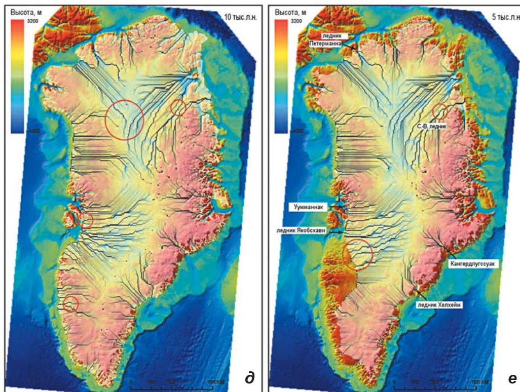
◀▲ Рис. 4.135. Реконструированные подледниковые дренажные сети (голубые линии) и озера (синие области) для шести временных срезов: 19, 16, 13, 12, 10 и 5 тыс. лет назад (а–е). Прежний ледниковый покров показан полупрозрачным фоном поверх гипсографической карты ложа и прилегающих областей. Красными окружностями помечены места перестройки дренажной сети (Livingstone et al., 2013)
