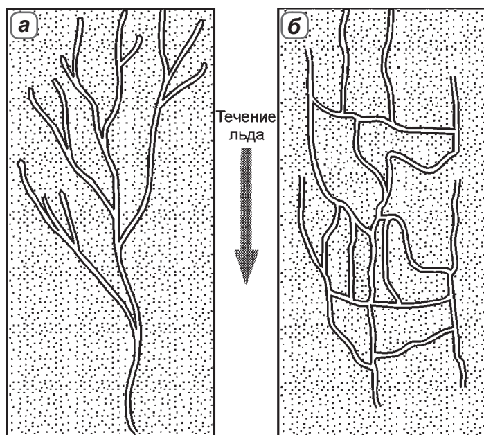
▲ Рис. 1.5. Древовидная (а) и распределенная (б) системы подледниковых каналов (Kamb, 1987; Fountain, Walder, 1998)
