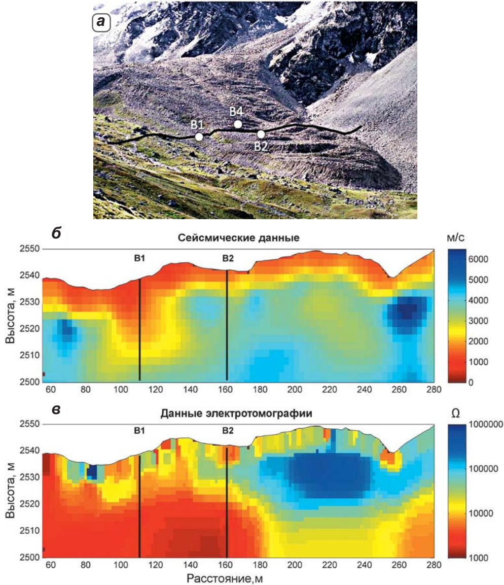
▲ Рис 2.42. Профиль сейсмических и геоэлектрических измерений (черные линии) на каменном глетчере Мюраг в Швейцарских Альпах (а). Белыми кружками показаны скважины, в которых измерялась температура льда и в кернах определялось содержание пород во льду; скорость распространения Р-волн (м/с) по данным сейсмозондирования (б), электрическое сопротивление (Ом) по данным электротомографии (в) (Hauck et al., 2011)
