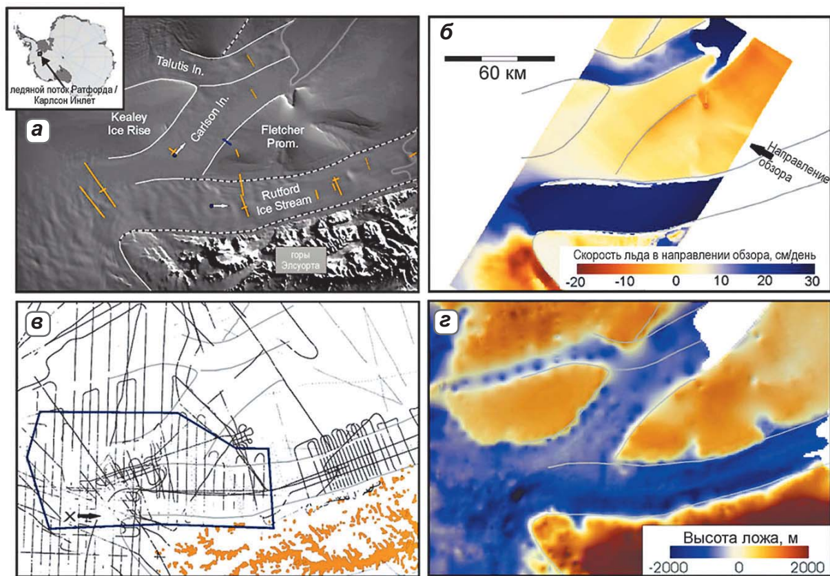
◀ Рис. 4.59. Исследования на ледяном потоке Ратфорд и выводящем леднике Карлсон Инлет в Западной Антарктиде (а). Направления течения льда показаны белыми стрелками, точечной белой линией – трещиноватые края ледяного потока, синими кружками – места определения напряжения сдвига на ложе, оранжевыми линиями – сейсмические профили, где были сделаны измерения акустического импеданса ложа, синими линиями – профили радиозондирования, линии налегания ледников – серыми линиями. Скорости течения льда (направление примерно параллельно горизонтальной оси) по данным радиоинтерферометрических съемок 12 и 13 ноября 1995 г. со спутников ERS-1 и ERS-2 (б). Измерения высоты поверхности и ложа (черные точки), использованные для построения цифровых моделей поверхности и ложа (в). Толстой черной линией выделен участок, для которого цифровые модели поверхности и ложа использованы для вычисления путей течения подледниковой воды (см. рис. 4.60, 4.61). Цифровая модель ложа (г) (Vaughan et al., 2008)
