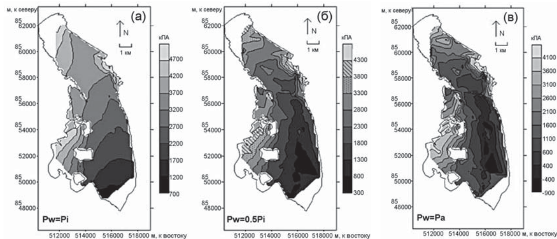
Рис. 4.30. Распределение гидравлического потенциала на леднике Ханс при разных отношениях давления воды P_w , льда P_i и воздуха P_a : а) P_w = P_i ; б) P_w = 0,5P_i ; в) P_w = P_a (Pälli et al., 2003)
