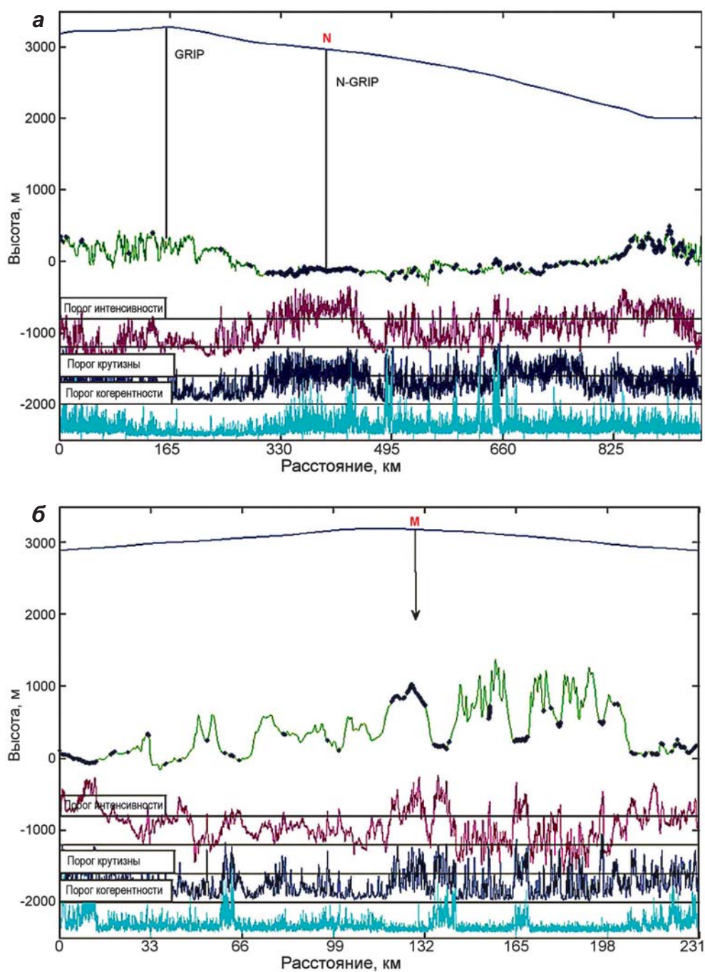
▲ Рис. 2.112. Результаты радиозондирования ледникового покрова Гренландии вдоль двух профилей, проходящих через места бурения GRP и N-GRP: точки (а) и М (б). Линиями разного цвета показаны: высота поверхности (синий), глубина ложа (зеленый), интенсивность отражений от ложа (фиолетовый), их крутизна (темно-синий), когерентность (голубой). Синими ромбами отмечены скопления воды на ложе, установленные по интенсивности и крутизне отражений. Положение точек N и М показано на рис. 2.115 (Oswald, Gogineni, 2008)
