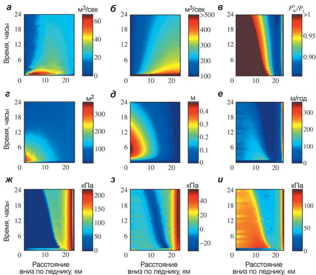
▲ Рис. 4.73. Графики изменений основных показателей динамики покровного ледника при прорыве наледникового озера (в координатах расстояние–время): а) пластовый расход воды, \text{м}^3/\text{с} ; б) расход воды в каналах, \text{м}^3/\text{с} ; в) относительное давление воды под ледником; г) поперечное сечение каналов, \text{м}^2 ; д) вертикальное поднятие, м; е) скорость на ложе, м/год; ж) напряжение сдвига на ложе, кПа; з) осредненное по вертикали продольное напряжение, кПа; и) осредненное по вертикали латеральное напряжение сдвига, кПа (Pimentel, Flowers, 2011)
