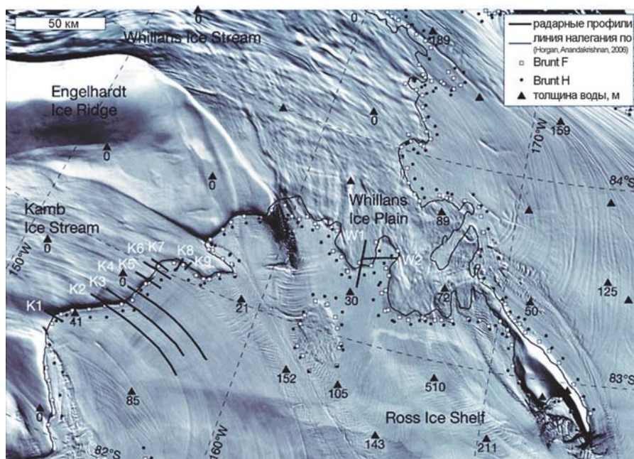
▲ Рис. 2.87. Положение линии налегания на шельфовом леднике Росса в районе впадения ледяных потоков Вилланса (В) и Кэма (С). Ее положение (тонкая черная линия) между шельфовым ледником и ледяными поднятиями определено по данным (Horgan, Anandakrishnan, 2006), а положение точек F (белые квадраты) и H (черные точки) – по данным ICESat (Brunt and et al., 2010); цифрами обозначены глубины моря по данным сейсмозондирования (Robertson, Bentley, 1990); буквами К1–К9 и W1–W2 – профили радиозондирования на частоте 2 МГц (MacGregor et al., 2011)
