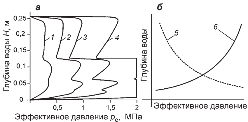
▲ Рис. 1.10. Стационарная толщина слоя воды H как функция эффективного давления p_e и постоянных величин градиента гидравлического потенциала d\Phi/dy , Па/м (а): 1 – 2,5; 2 – 5,0; 3 – 7,5; 4 – 12,5; плоские участки кривых со слабым наклоном вправо соответствуют стабильным состояниям, участки с наклоном влево – нестабильным состояниям. Для сравнения показано соотношение между быстрым (5) и медленным (6) типом подледниковых систем стока (Creyts, Schoof, 2009)
