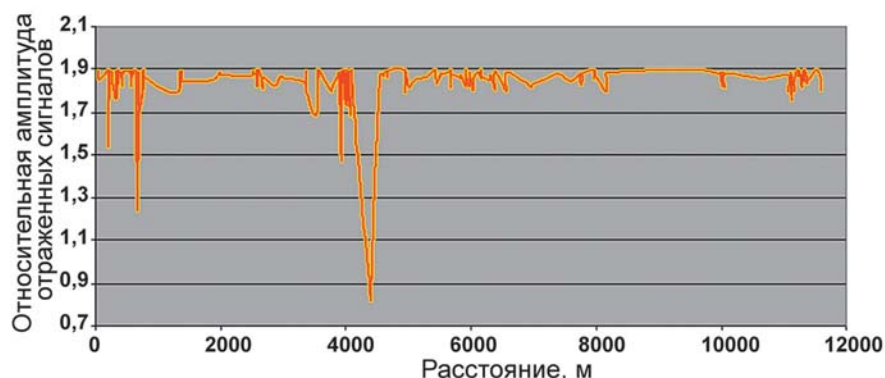
▲ Рис. 3.25. Изменение амплитуды отраженных от ложка сигналов вдоль продольного профиля 2005 г. Б1–Б2 (см. рис. 3.12) на леднике Фритьюф; положение пиков амплитуды показано на карте гидравлического потенциала (рис. 3.24)
