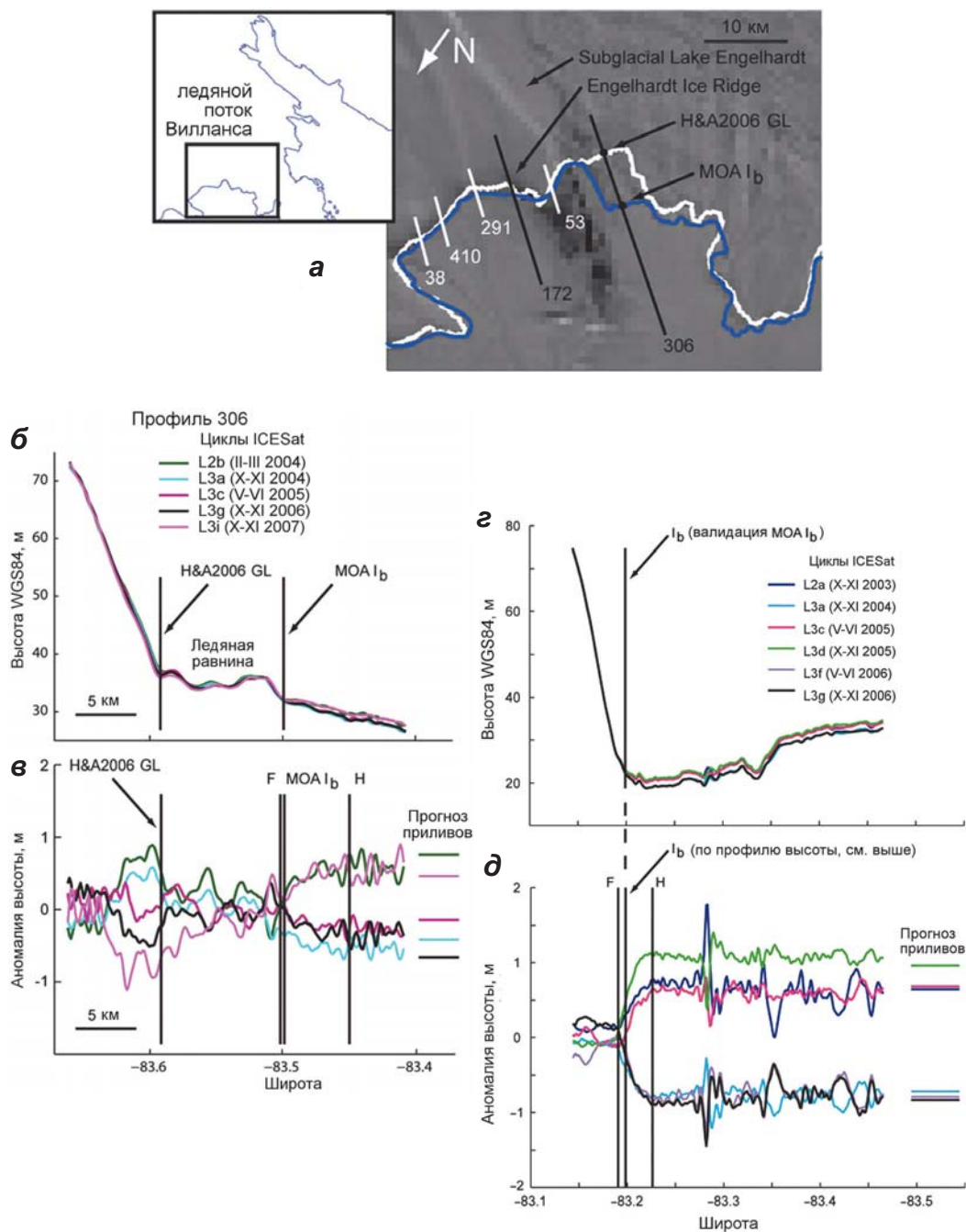
▲ Рис. 2.144. Положение линии налегания GL (белая линия) и точки I b (голубая линия) в окрестности подледникового озера Энгельгардт, оцененное по ЦМР по данным дифференциальной радиоинтерферометрии (Horgan, Anandakrishnan, 2006) (H&A2006) (а) и точек F и H по данным ICESat 2004–2007 гг. (б, в) в сравнении с предсказанными высотами приливов (справа); положение точек I b , F и H в районе ледяного поднятия Керри (рис. 2.144, а) по данным ICESat 2003–2008 гг. с учетом предсказанной высоты приливов (справа) (г, д) (Brunt et al., 2010)
