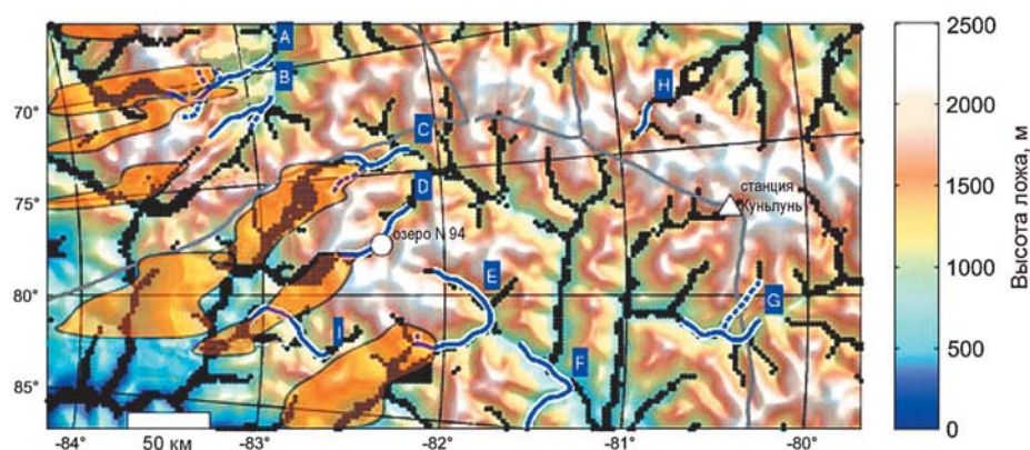
▲ Рис. 4.124. Рельеф ложа, где показаны основные тальвеги подледниковых долин (черные линии), гидрологические сети (голубые линии), области намерзшего льда (оранжевый фон), озеро № 94 (Popov, Masolov, 2007; Siegert et al., 2005), ледоразделы (серые линии) (Wolovick et al., 2013)
