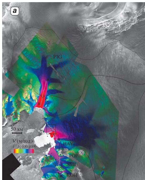
► ▼ Рис. 4.48. (а) Скорость ледников Пайн Айленд (PIG) и Туейтс по данным радиоинтерферометрии 1996 г. со спутников ERS-1 и ERS-2 (в логарифмическом масштабе). Линия налегания показана толстой черной линией; границы дренажных бассейнов, определенные по данным о толщине льда, – тонкой черной линией; (б) ускорение движения ледника Пайн Айленд за 1973–2005 гг. по данным со спутников ERS-1 и ERS-2 и Radarsat-1 вдоль профиля В от положения линии налегания в 1996 г. (Rignot, 2006).
