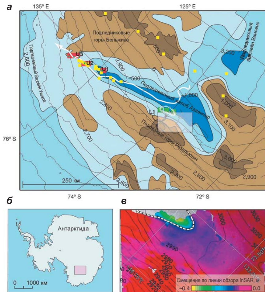
▲ Рис. 4.106. Активные озера в подледниковом трое Адвенчер в районе купола С в Восточной Антарктиде: а) высота поверхности ледникового покрова и положение подледниковых озер U1, U2, U3 (желтые квадраты) и L1 (его граница показана пунктирной белой линией); изолинии поверхности показаны тонкими линиями, другие небольшие подледниковые озера в этом районе – желтыми квадратами, участки понижения и повышения высоты поверхности на 1 м по данным альтиметрии со спутника ERS-2 – зеленым и красным цветом; направление течения воды, вычисленное по градиенту давления подледниковой воды – белой толстой линией со стрелкой; голубым и коричневым цветом показаны высоты ложа ниже и выше уровня моря; б) положение района исследований в Антарктиде; в) район, покрытый радиоинтерферометрической (InSAR) съемкой со спутника ERS-2. Для периода с 14 августа 1997 г. по 16 марта 1998 г. выделены также участки понижения поверхности, показанные на (а) (Wingham et al., 2006)
