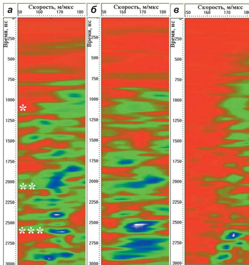
▲ Рис. 3.10. Скоростной профиль ледника Ханс по данным двухпозиционных ОГТ-измерений и итеративного скоростного сембланс-анализа: а) СМР-1, б) СМР-3 и в) СМР-4. Знак * показывает время распространения до отражателя 1, ** – до отражателя 2, *** – до ложа (Яния и др., 2005; Jania et al., 2005)
