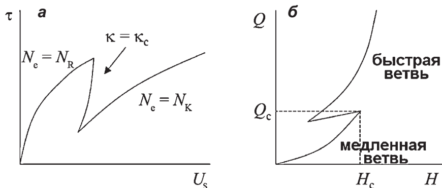
▲ Рис. 1.18. Связь между напряжением сдвига на ложе \tau и скоростью скольжения U_s (а); связь между расходом льда Q и толщиной льда H (б). N_e – эффективное давление воды, N_R – стабильное давление воды в каналах, N_K – давление воды, при котором система связанных полостей стабильна, K – параметр течения: при K = K_c происходит переход от дренажа в каналах к дренажу в системе связанных полостей. При критической толщине ледника H_c и соответствующем критическом потоке Q_c ледник скачком переходит с медленной ветви на быструю (Jiscoot, 1999)
