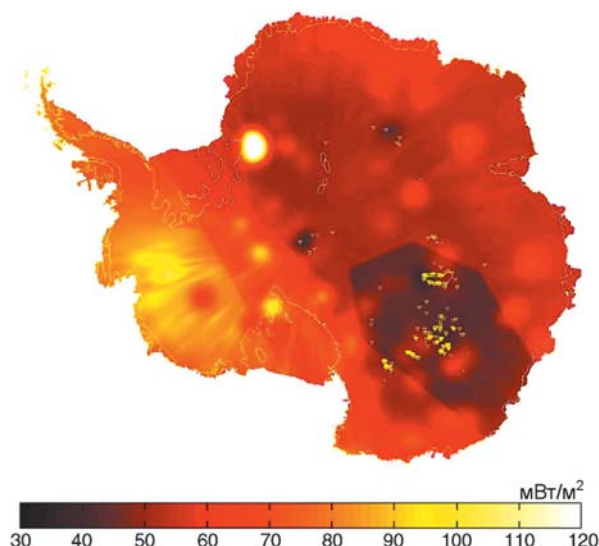
◀ Рис. 4.41. Распределение геотермического потока тепла в основании ледникового покрова Антарктиды, основанное на комбинации баз данных (Shapiro, Ritzwoller, 2004; Pollard et al., 2005) и исправленное с учетом данных термозондирования скважин, а также распределения подледниковых озер разных типов (Pattyn, 2010)
