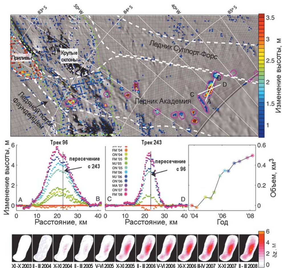
▲ Рис. 4.107. Вверху: изменение высоты поверхности ледника Академия и объема подледникового озера по данным ICESat в 2003–2008 гг. (тонкие темные линии). Изменения высоты поверхности вдоль треков более 0,5 м показаны цветной шкалой, границы бассейнов ледяных потоков – белым пунктиром; оранжевый пунктир – линия налегания шельфового ледника с большими приливными колебаниями. Графики посередине: смещения высоты поверхности в октябре–ноябре 2003 г. по трекам АВ (96) и CD (243), пересекающим подледниковое озеро и кривую заполнения подледникового озера с 2004 по 2008 г. Внизу: изменения высоты над подледниковым озером в 2003–2008 гг. (Smith et al., 2009)
