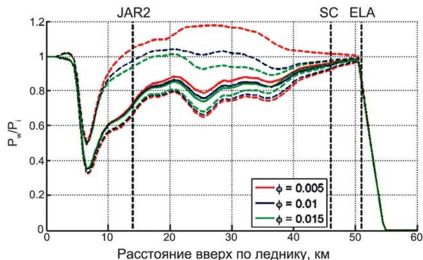
▲ Рис. 4.71. Изменение условий всплывания P_w/P_i вдоль линии тока ледника в зависимости от объемной пористости льда \phi = 0,005 ; 0,01 и 0,015 . Штриховыми линиями показаны максимальные и минимальные пределы в течение года. Показано положение станций JAR2, Swiss Camp и границы питания ELA (Colgan et al., 2011)
