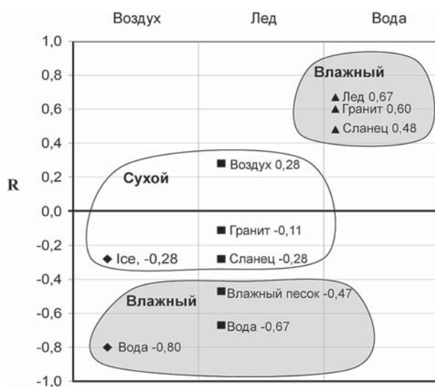
► Рис. 2.74. Относительный коэффициент отражения r от разных границ (Bælum, Benn, 2010)
