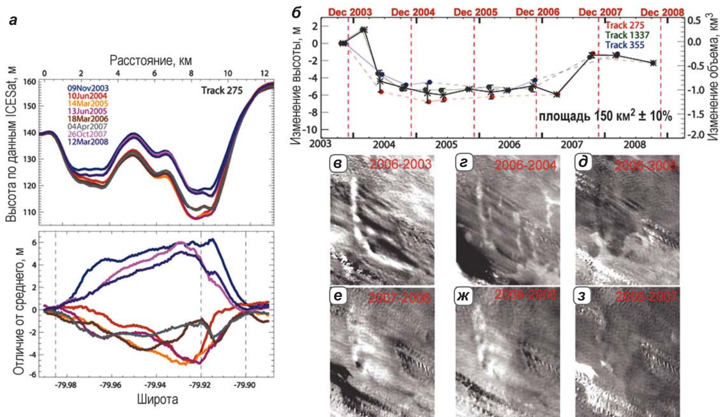
▲ Рис. 4.99. Подледниковое озеро Мас1 под ледяным потоком Мак-Эйела (Е): а) повторные ICESat профили и аномалии высоты поверхности по данным ICESat для трека 275; б) временные серии изменений высоты и объема по трем трекам ICESat, красные вертикальные линии показывают приблизительное время съемок в период с 2003 по 2008 г.; в–з) изображения, иллюстрирующие цикл заполнения–дренирования озера (Fricker et al., 2010)
