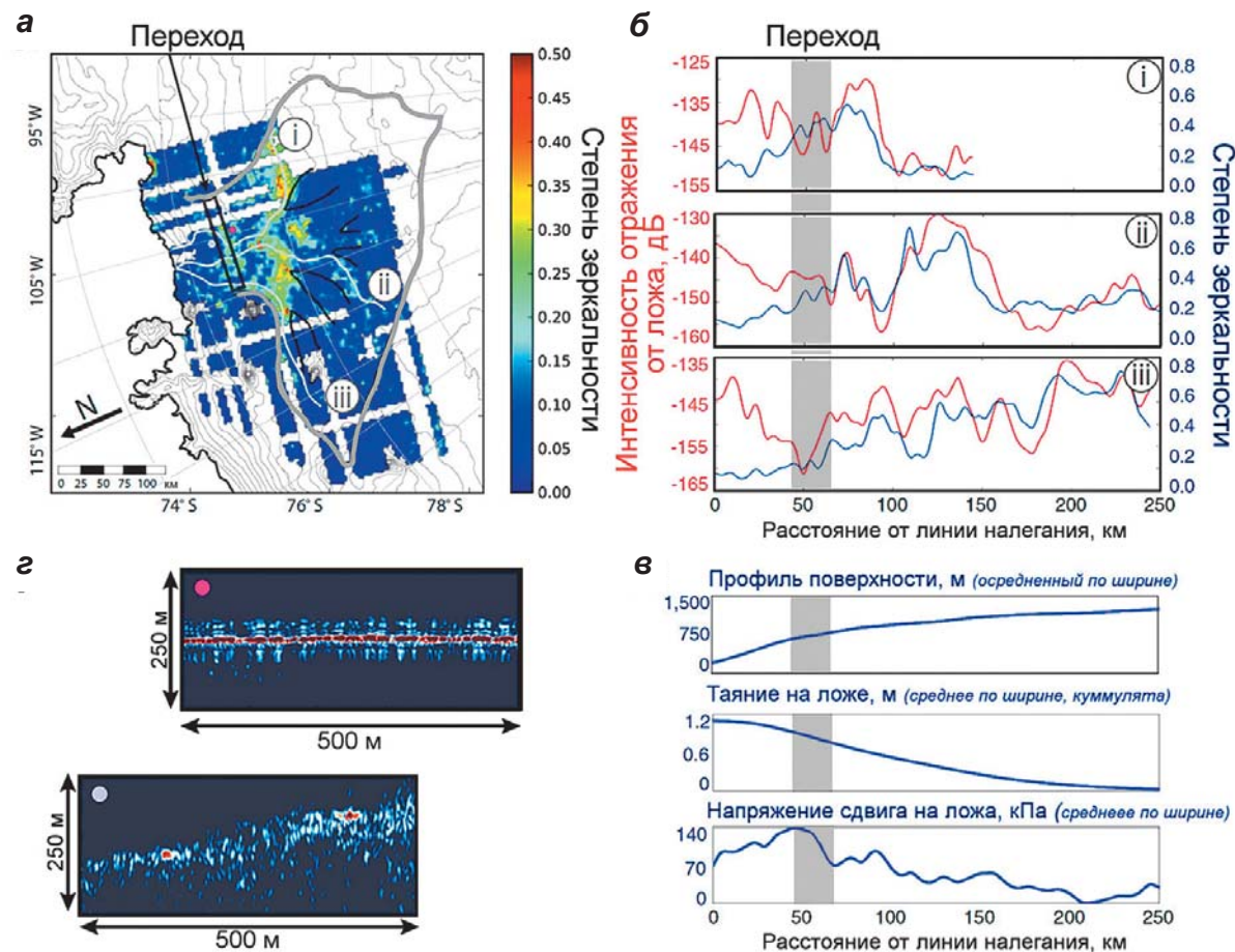
◀ Рис. 4.53. Переход от распределенной к концентрированной системе стока под ледником Ту-ейтс. а) Степень зеркальности радарных отражений от ложа (цветная шкала) в бассейне ледника (выделен толстой серой линией), поле гидравлического потенциала (изолинии) и модельные линии тока воды (черные линии), три основные линии (i, ii, iii) выделены светло-серым цветом. Зона перехода от распределенной к концентрированной системе выделена черным прямоугольником. б) Интенсивность отражения от ложа (левая шкала) и степень зеркальности (правая шкала) вдоль линий тока воды (i, ii, iii). Переходная зона от распределенной к концентрированной дренажной системе выделена серой полосой. в) Сверху вниз: профиль поверхности ледника, скорость донного таяния (накопленные значения вниз по леднику), напряжения сдвига на ложе. Все значения осреднены по ширине ледника. г) Радарограммы участков ложа, выполненные поперек предполагаемого движения воды. Они сделаны в области распределенных систем стока (помечена фиолетовым пунсоном) и в области концентрированных систем (светло-розовый пунсон) (Schroeder et al., 2013)
