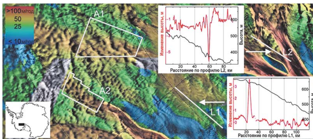
▲ Рис. 4.90. Области подъема и опускания поверхности на притоке ледяного потока Кема (участок A1) и на ледяном потоке Биндшадлера (участок A2) по данным радиоинтерферометрической съемки со спутника RADARSAT за период с 24–26 сентября по 20 октября 1997 г. Шкала скорости движения льда – сверху слева. На врезках – области измерений вертикального смещения, где черной и красной линиями показаны высота поверхности и ее изменения вдоль лидарных воздушных профилей L1 и L2 (белые линии) (Gray et al., 2005)
