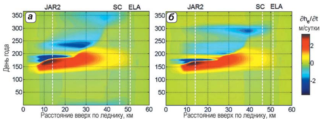
▲ Рис. 4.70. Изменения гидравлического напора в течение года при коэффициенте трения в каналах f = 0,05 (а) и 0,01 (б). Показано положение станций JAR2, Swiss Camp и границы питания ELA (Colgan et al., 2011)
