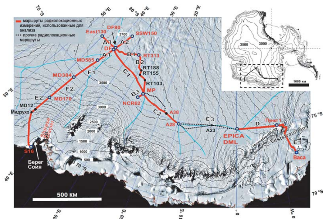
▲ Рис. 2.96. Наземные радиолокационные измерения (красные линии) на частотах 60 и 179 МГц на Земле Королевы Мод в Восточной Антарктиде от побережья у станций Сёва и Васа до купола Фуджи (DF) на профилях, проходящих через места глубокого бурения Dome Fuji и EPICA DML. Измерения около скважин использованы для определения скорости распространения радиоволн во льду (Fujita et al., 2012)
