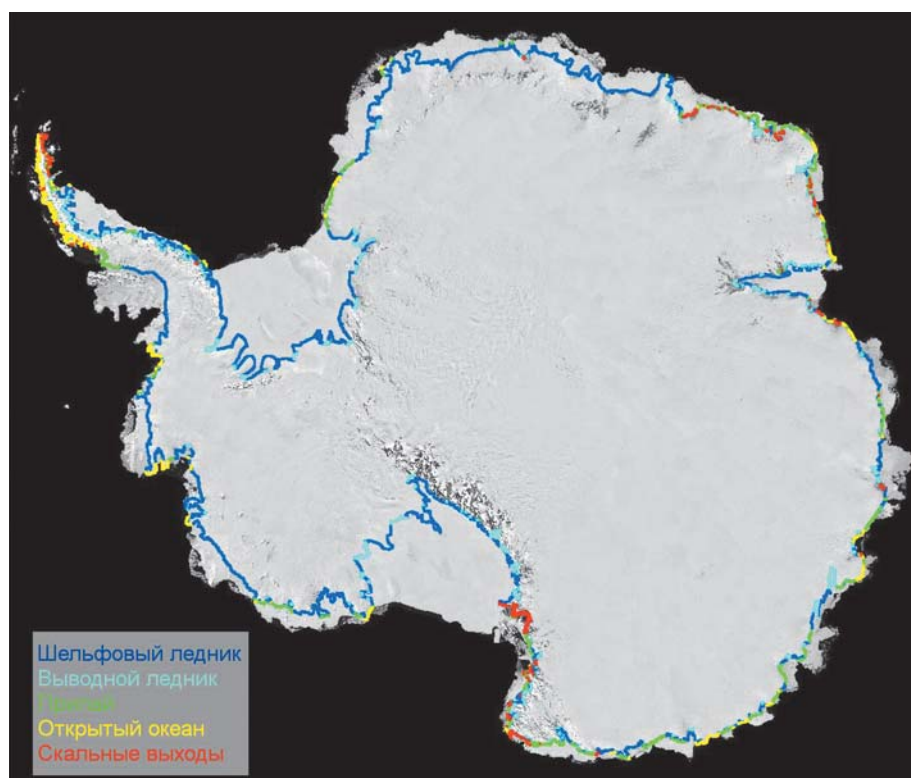
▲ Рис. 2.148. Границы наземного льда в Антарктиде, установленные на шельфовых ледниках (синие линии, 61 %), выводных ледниках (голубые линии, 13 %), быстро движущемуся льду (зеленые линии, 10 %), у открытого океана (желтые линии, 9 %) и у выходов горных пород (красные линии, 7 %) (Bindschadler et al., 2011)
