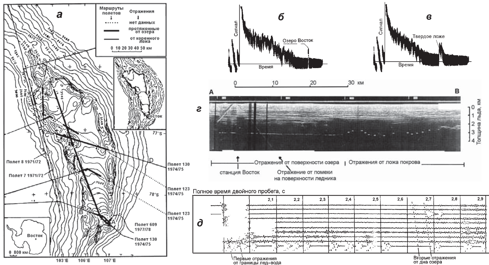
◀ ▼ Рис. 2.124. Изогипсы поверхности ледникового покрова в районе станции Восток (через 2 м над озером и через 10 м в остальной части) по данным радиоальтиметрии 1993 г. со спутника ERS-1 (Ridley et al., 1993) и профили аэрорадиозондирования 1974/75 и 1977/78 гг. (тонкие черные линии) с участками регистрации отражений от поверхности озера (толстые черные линии) (а); на врезке показаны границы озера по данным радиоальтиметрии и радиозондирования; отражения от поверхности озера (б) и ложа ледникового покрова (в) на дискретных А-записях (Зотиков, 2010) и на непрерывной Z-записи (г) (Kapitsa et al., 1996); д) данные сейсмозондирования 1964 г. с отражениями от поверхности и дна озера (выделены пунктирными линиями) (Kapitsa et al., 1996)
