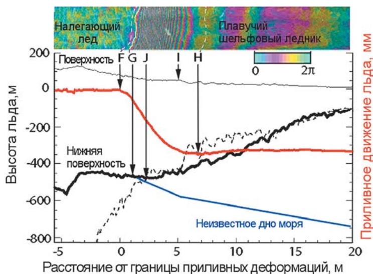
▲ Рис. 2.146. Зона налегания выводного ледника Петерманн в Гренландии. Буквами обозначены: предел влияния приливов (F), линия налегания (G), место, где ледник впервые достигает гидростатического равновесия (J), точка перегиба наклона поверхности (I), граница зоны приливных деформаций (H), тонкой черной линией показана высота поверхности льда над средним уровнем моря по данным лазерной альтиметрии, толстой черной линией – топография ложа по данным радиозондирования, пунктирной линией – глубина ложа, вычисленная из условия гидростатического равновесия, голубой линией – неизвестная глубина дна (вероятно, превышающая 800 м), красной линией – высота приливов в миллиметрах вертикального движения, измеренная по данным ERS-1 DInSAR. Цветная вставка сверху показывает интерферометрические полосы от 0 до 2\pi , по которым определено положение точек F, G и H (Rignot et al., 2011)
