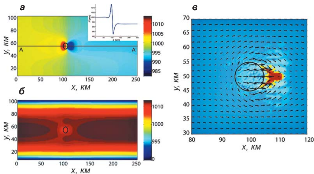
▲ Рис. 4.66. Стационарная модель течения ледяного потока над пятном прилипания (показано кружком): а) толщина льда, м; на врезке показана толщина льда вдоль поперечного сечения AA'; б) скорость течения, м/год; в) течение воды от пятна прилипания при напряжении сдвига на пятне прилипания 50 и 10 кПа вне нее; направление течения слева направо. Цветом показана концентрация талой воды, продуцируемой над пятном прилипания (показана черным кругом). Черные стрелки показывают скорости, пропорциональные скорости течения воды, отрицательный градиент гидравлического потенциала \phi указывает направление течения воды (Sergienko, Hulbe, 2011)
