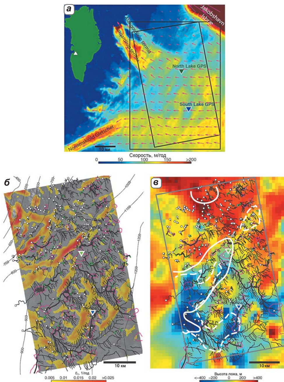
▲ Рис. 2.28. Направление (стрелки) и средняя скорость течения льда (м/год) в зимы 2007–2009 гг. (цветная шкала) по данным RADARSAT (а); треугольниками показаны места GPS-измерений; изображение Terra SAR-X, на котором изолиниями показана высота поверхности, поверхностные потоки и потоки между озерами, а цветом – напряжения сдвига (год -1 ), достаточные для образования трещин (б); высота ложа (м) по данным (Griggs et al., 2012) и гидрология поверхности: бассейны озер (красные контуры), скопления воды и ледниковые колодцы (белые кружки) (в); белыми линиями показаны области, где скорости движения увеличивались на 100 % (пунктиром – 15 июля 2009 г., сплошная линия – 10 июня 2010 г.) (Joughin et al., 2013)
