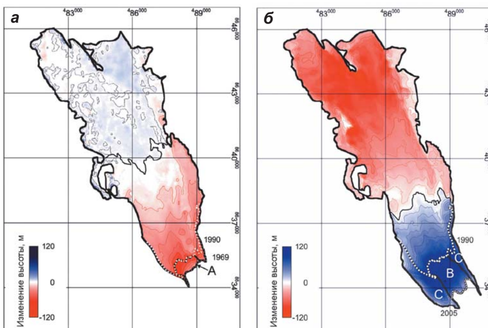
▲ Рис. 3.18. Изменение высоты поверхности ледника Фритьоф: а) до подвижки – с 1969 по 1990 г., б) после подвижки – с 1990 по 2005 г. (Murray et al., 2003). Изолинии проведены через 10 и 50 м; черной линией показана примерная граница между зонами накопления и убыли массы льда (синим и красным цветом). А и В – области, где ледник отступал и наступал в тех частях фьорда, для которых нет батиметрии; С – области, где ледник наступал по осадочным отложениям или захватывал свой западный приток Сарабреен (Murray et al., 2012)
