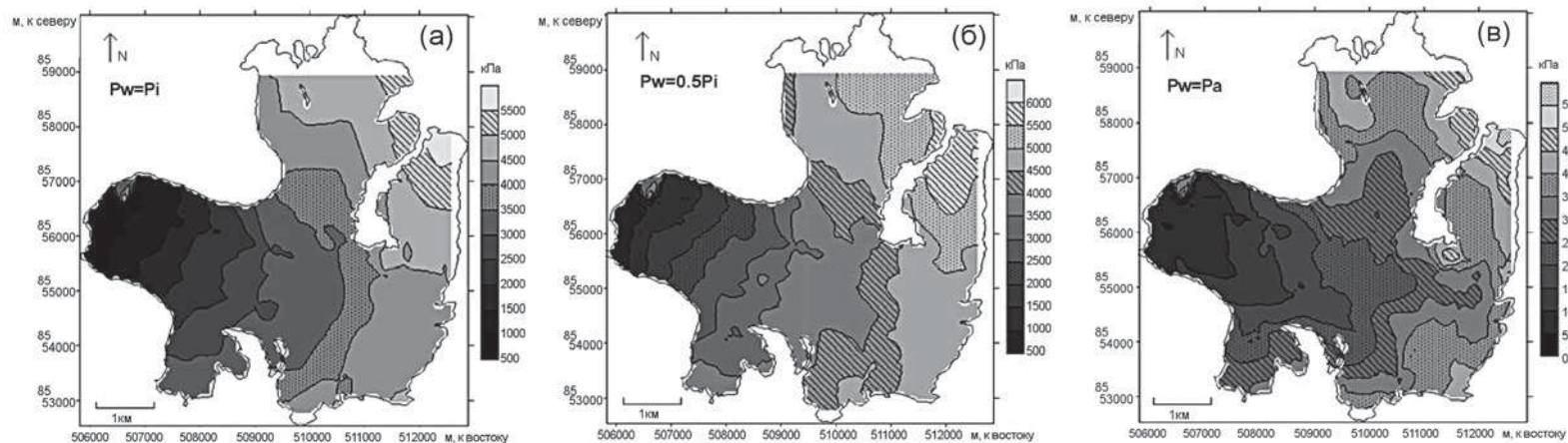
Рис. 4.31. Распределение гидравлического потенциала на леднике Вереншельд при разных отношениях давления воды P_w , льда P_i и воздуха P_a : а) P_w = P_i ; б) P_w = 0,5P_i ; в) P_w = P_a (Pälli et al., 2003)
