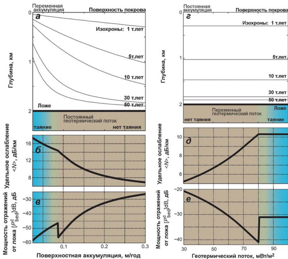
▲ Рис. 2.85. Влияние аккумуляции на поверхности (а–в) и потока геотермического тепла (г–е) на удельное ослабление \langle N \rangle (дБ/км) (б, д) и мощность отражений от ложа P^c_{bed} (дБ) (в, е). При расчетах принято: толщина льда H = 2 км, поверхностная температура -30^\circ\text{C} (Matsuoka, 2011)
