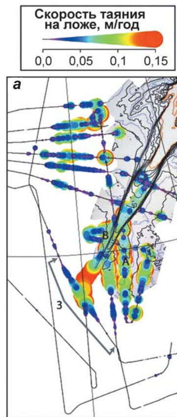
◀ ▲ Рис. 2.116. Скорость донного таяния, м/год, вдоль профилей радиозондирования в Северной Гренландии (а). Цифрой 3 и серыми стрелками обозначен участок радарного профиля (б), для которого на (в) показана оцененная скорость донного таяния, м/год (Fahnestock et al., 2001)
