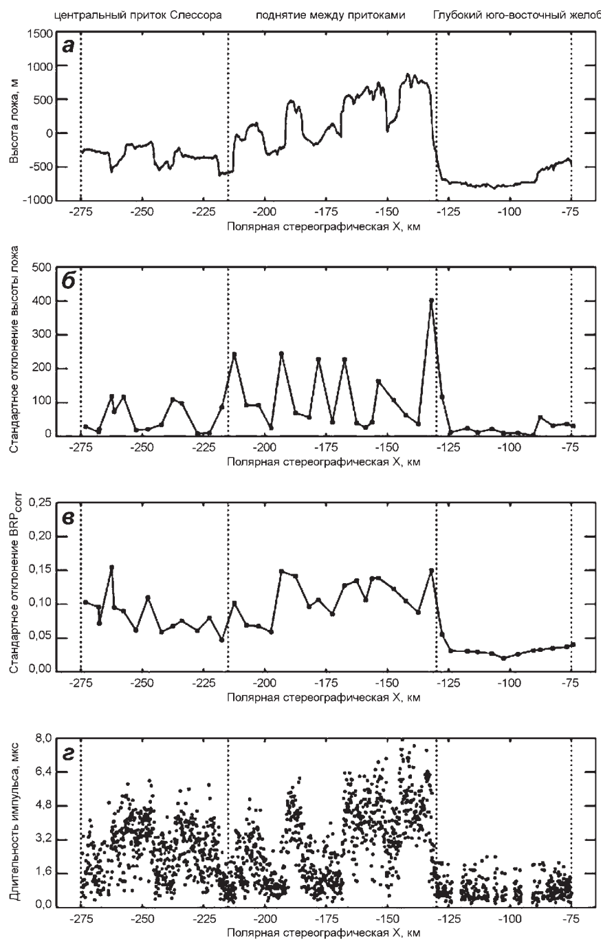
▲ Рис. 2.104. Пример использования трех методов для оценки степени шероховатости ложа вдоль части профиля, показанного на рис. 2.103, б: высота ложа (а); среднее квадратическое отклонение высоты ложа с разрешением ~60–75 м, осредненное по сети 5×5 км (б); среднее квадратическое отклонение мощности отражений от ложа с учетом поправки на толщину льда таким же разрешением и осреднением (в); длина отраженного импульса, мкс с разрешением 1,12 м (без осреднения) (г) (Rippin et al., 2006)
