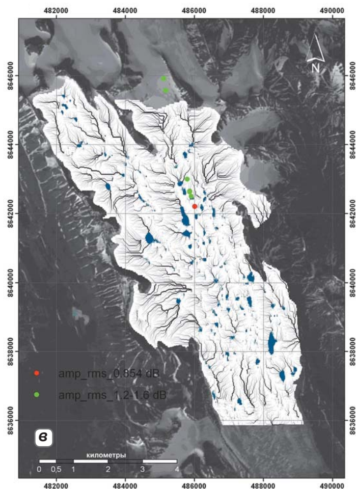
◀ ▲ Рис. 3.24. Подледниковая гидрологическая сеть ледника Фритьоф в 1936 (а), 1990 (б) и 2004 (в) гг.; на (в) красными и зелеными точками показано положение максимумов амплитуды отраженных от ложа сигналов
