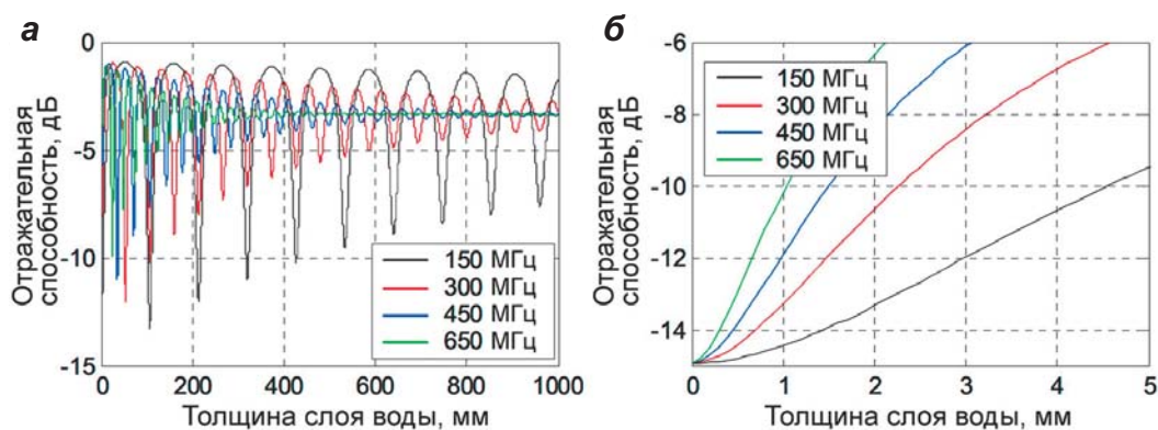
▲ Рис. 2.78. Зависимость интенсивности отражений (коэффициента отражения R ) от слоя воды толщиной от 0 до 1 м (а) и 0 до 5 мм (б) на ложе ледника на частотах 150, 300, 450 и 650 МГц (Paden, 2003)
