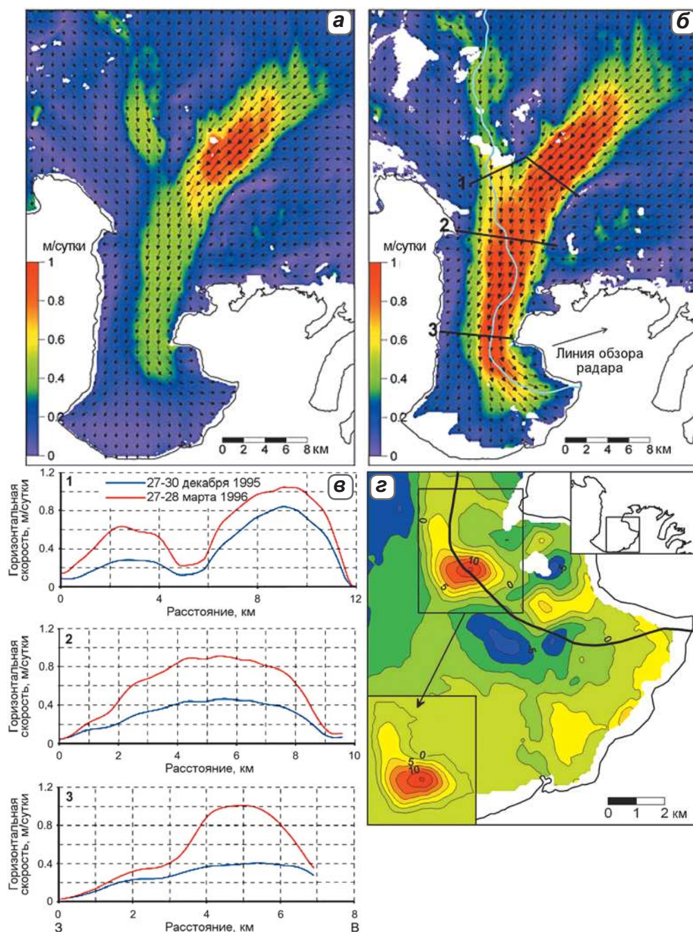
▲ Рис. 2.137. Горизонтальные поверхностные скорости, м/день, на леднике Скейдарарйёкюдль в Исландии по данным InSAR: а) 27–30 декабря 1995 г. до начала йокульлаупа, б) 27–28 марта 1996 г. в начале йокульлаупа. Голубой линией на (б) показано вычисленное направление подледникового прорыва под ледником Скейдарарйёкюдль; в) скорости в декабре 1995 г. и марте 1996 г. на трех поперечных профилях 1, 2 и 3, показанных на (б); г) оценка вздымания (см) поверхности ледника Скейдарарйёкюдль из-за накопления подледниковой воды 27–28 марта 1996 г. в начале йокульлаупа. На врезке показан подъем поверхности с учетом коррекции. Черная линия показывает путь сброса воды в р. Скейдара (Magnússon et al., 2007)
