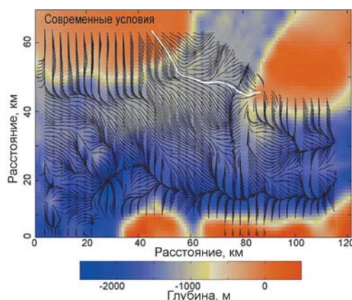
► Рис. 4.60. Градиенты подледникового гидравлического потенциала для системы ледяной поток Ратфорд – выводной ледник Карлсон Инлет, вычисленные по цифровым моделям поверхности и ложа (см. рис. 4.59) при современных условиях. Подледный водораздел между ледяным потоком и выводным ледником показан белой линией (Vaughan et al., 2008)
