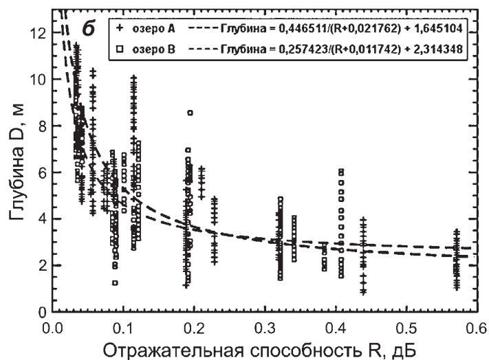
▲ Рис. 2.20. Наледниковые озера на юго-западе Гренландии на изображении MODIS с разрешением 250 м, полученном 26 августа 2003 г. (а) и связь между отражательной способностью R и измеренной глубиной D озер А и В в виде функции D = (\alpha_0/R + \alpha_1) + \alpha_2 (б); (Box, Ski, 2007)
