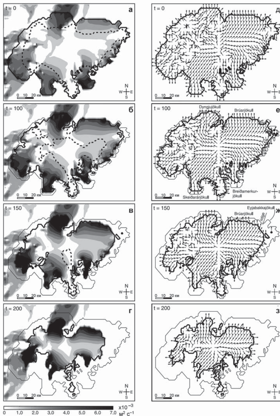
▲ Рис. 4.38. Модельная реакция подледниковой и поверхностной гидрологии ледникового купола Ватнайёкюдль в Исландии на потепление климата на 2 °C за столетие без изменения осадков для: исходного состояния (а, д), через 100 лет (б, е), 150 лет (в, ж) и 200 лет (е, з). Слева: сумма подледникового и поверхностного потока, вычисленных как среднее по сети 1,62×1,85 км; справа: вычисленные направления течения подледниковой воды. Начальные размеры ледникового купола показаны тонкой линией, область аккумуляции на рис. 4.38, а–в показана точечной линией и не показана на рис. 4.38, г (Flowers et al., 2005)
