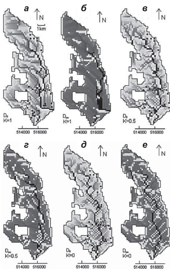
◀ Рис. 4.32. Схемы подледникового дренажа на леднике Ханс, полученные методами D_8 (а, в, д) и D_\infty (б, г, е) при разных отношениях давления воды P_w льда P_i и воздуха P_a : (а, б) P_w = P_i ; (в, г) P_w = 0,5 P_i ; (д, е) P_w = P_a . Черными квадратами с номерами обозначены ледниковые колодцы. Направление течения из колодца Кристал-Кейв обозначено черной стрелкой (Palli et al., 2003)
