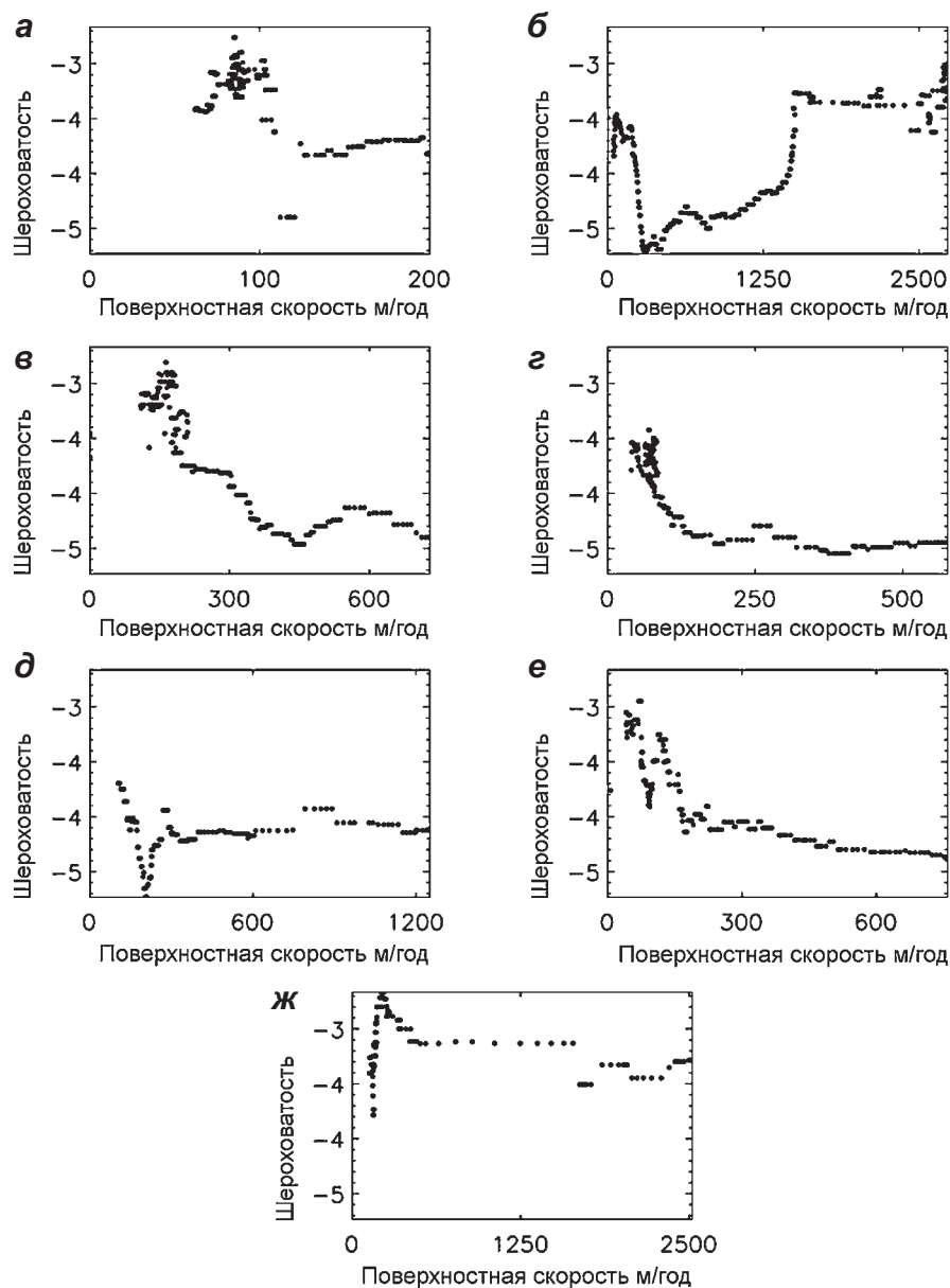
▲ Рис. 2.110. Вариации шероховатости ложа (в логарифмическом масштабе) в зависимости от скорости вдоль притоков (см. рис. 1.109, в): а) приток 1; б) приток 2 и основной ствол ледника Пайн Айленд; в) приток 3; г) приток 4; д) приток 5; е) приток 6; ж) приток 7 (Rippin et al., 2011)
