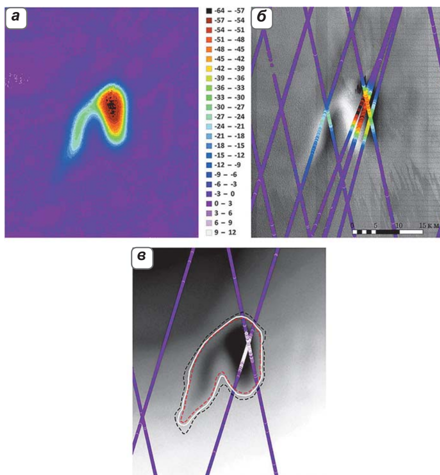
▲ Рис. 2.132. Изменения высоты (м) ледникового покрова над подледниковым озером Кука E2 по данным ЦМР на основе ICESat, SPOT5 и ASTER. Отрицательные значения соответствуют снижению поверхности; разница высот ЦМР до и после спуска озера (а); разница высот 9 февраля 2012 (SPOT5 DEM) и измерений ICESat, полученных до спуска озера (б); разница высот 9 февраля 2012 (SPOT5 DEM) и измерений ICESat, полученных в марте 2009 г. после спуска озера (в). На последнем рисунке черная, белая и красные линии оконтуривают депрессию с шагом -1,5 , -3 и -5,5 м. Им соответствует «площадь озера» 267, 219 и 192 км 2 (Flament et al., 2011)
