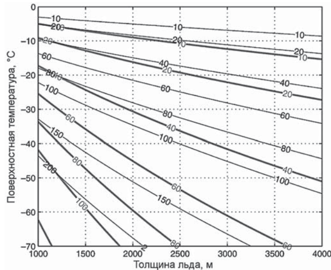
▲ Рис. 4.42. Минимум геотермического потока тепла, необходимый для достижения точки таяния при соответствующем давлении как функция толщины льда и поверхностной температуры. Высокая (0,5 м/год) и низкая (0,05 м/год) скорости вертикальной адвекции показаны толстой и тонкими линиями (Pattyn, 2010)
