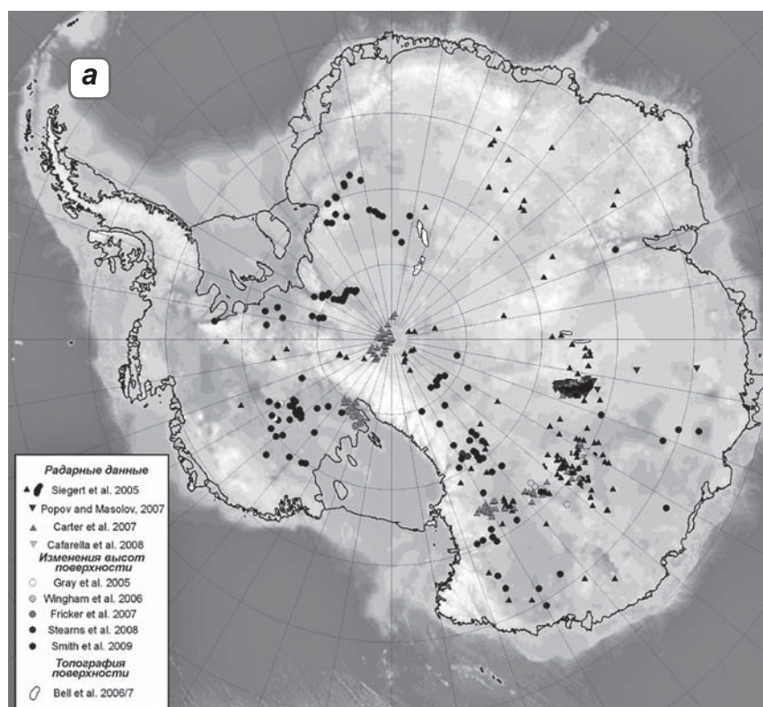
▲ ► Рис. 4.82. Положение всех подледниковых озер в Антарктиде, известных на июль 2010 г. (а). Показаны границы более крупных озер, более мелкие озера и озера с неизвестной площадью по данным радиозондирования и спутниковых съемок обозначены соответственно треугольниками и кружками. Озера по инвентаризации 2005 г. (Siegert et al., 2005) показаны черным цветом; озера, открытые позднее, обозначены разными значками, которые соответствуют первым публикациям о них (Wright, Siegert, 2010). Карта высоты ледникового покрова
