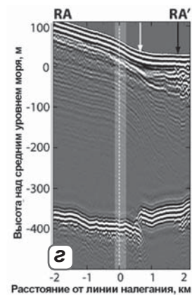
◀▶ Рис. 2.150. Радарные записи вдоль профилей NA-NA' (а), NB-NB' (б), NC-NC' (в), RA-RA' (г), SA'-SA (д), SB'-SB (е), SC'-SC (ж) на куполе Сайпл и о. Рузвельт. Положение профилей показано на рис. 2.149. Черная и белая стрелки показывают положение стратиграфического погружения верхних слоев и перегиб склона поверхности; область гидростатического равновесия находится в районе линии налегания на 0 км (зона ее возможного положения выделена прозрачным белым цветом) (Catania et al., 2010)
