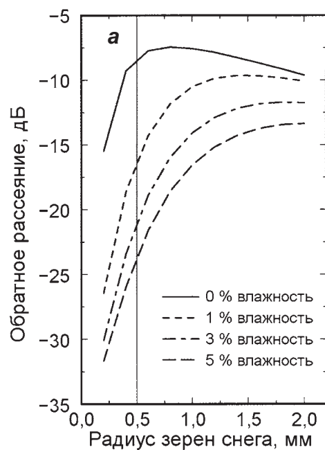
▲ ▼ Рис. 2.10. Обратное рассеяние (дБ) в снежном покрове влажностью от 0 до 5 % и размером зерен снега от 0,2 до 2,0 мм в Ku-диапазоне при угле падения 54^\circ (а) (Ngheim et al., 2001); радиус зерен снега в зависимости от глубины снежно-фирновой толщи (м) и скорости аккумуляции (см/год в.э.) (б) (Jordan, 1991)
