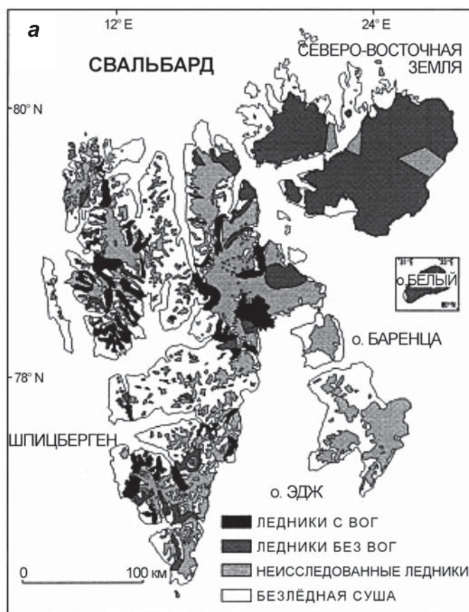
► Рис. 4.28. Распространение политермических (а) и пульсирующих (б) ледников на архипелаге Шпицберген (Jiskoot et al., 2000)
