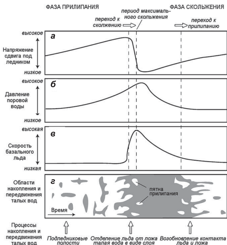
▲ Рис. 4.64. Связь изменений напряжения сдвига на ложе (а), давления поровой воды (б) и базальной скорости (в) во время цикла скольжения с пространственной и временной эволюцией пятен прилипания (г) (Knight et al., 2002)
