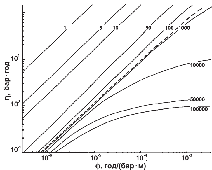
▲ Рис. 1.17. Вариации максимальной скорости скольжения, м/год (сплошные линии) для идеализированной модели ледника Бруарйокуль в Исландии в зависимости от «фактора смазки» ( \Phi ), год/(бар·м), и вязкости льда ( \eta ), бар·год. Штриховая линия – раздел между стационарными (слева) и пульсирующими (справа) ледниками. Максимальные скорости скольжения стационарного ледника достигаются тогда, когда они намного превышают 100 м/год, что ведет к возникновению его подвижки (Budd, 1975)
