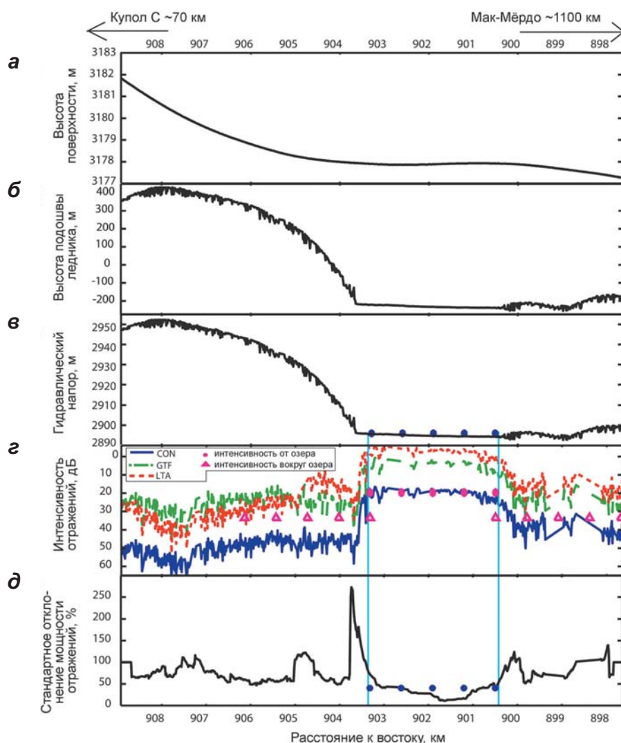
▲ Рис. 4.79. Подледниковое озеро Хорсшу (Подкова) (положение озера см. на рис. 4.78): а) высота поверхности ледникового покрова; б) высота основания льда; в) гидравлический напор, м; г) интенсивность отражений от поверхности озера (розовые точки) и вокруг озера (розовые треугольники); д) локальное стандартное отклонение мощности отражений, % (Carfer et al., 2007)
