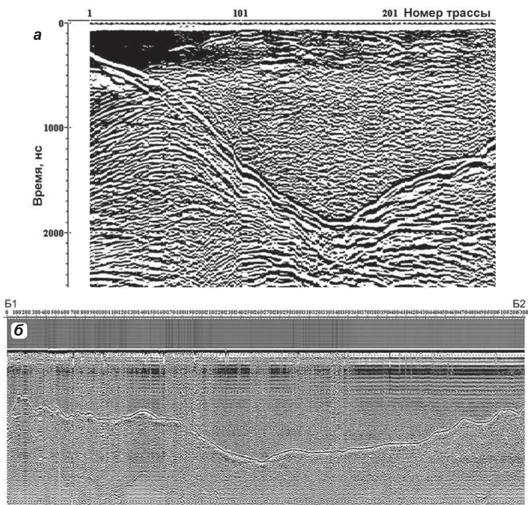
▲ Рис. 3.13. Строение ледника Фритьоф по данным радиозондирования 2005 г. с лоатором ВИРЛ-6 с центральной частотой 20 МГц на поперечном профиле А1–А2 в районе ледораздела (а) и на продольном профиле Б1–Б2 (б). Положение профилей показано на рис. 3.12 (Василенко и др., 2006)
