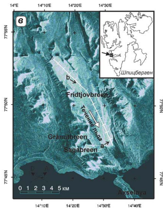
▲ ► Рис. 3.23. Изменение поверхностной скорости вдоль профиля от верховьев северо-западной ветви ледника Фридьоф до его нижней части (в): по данным спутниковой радиоинтерферометрии (Murray et al., 2003) (цветные линии) (а) в октябре 1991 г., феврале и марте 1992 г. (1), феврале и марте 1992 г. (2), январе и марте 1994 г. (3), июне 1995 г. (4), ноябре 1995 г. (5), феврале и мае 1996 г. (6) и октябре 1997 г.; на разных расстояниях от начала профиля по данным спутниковой радиоинтерферометрии (б) в период с января 1992 г. по январь 1997 г. (Murray et al., 2003) (цветные линии) и полевых измерений 1987 г. (Зингер и др., 1997) (черные кружки); голубой полосой показан интервал времени, когда скорости не могли быть определены из-за некогерентности радиоинтерферометрических изображений (Murray et al., 2003)
