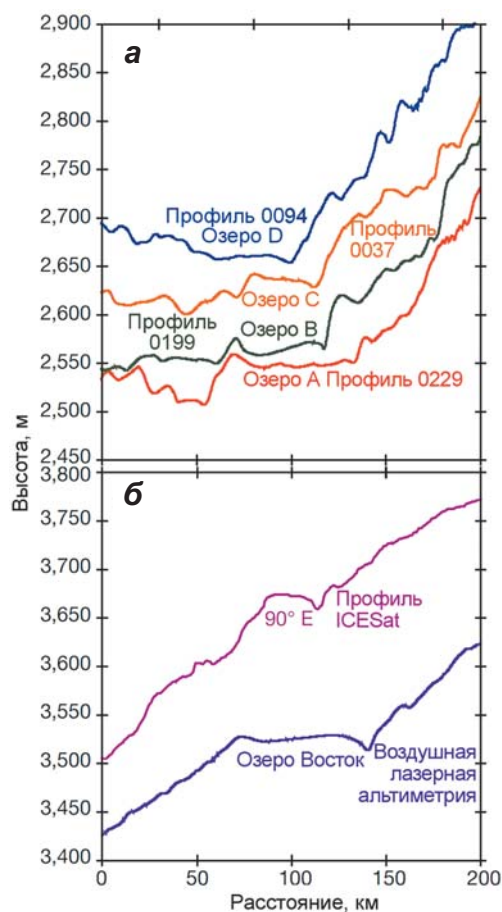
◀ Рис. 4.80. Высота поверхности над участками А, В, С и D в верховьях ледяного потока Рекавери (а) и подледниковыми озерами Восток и на 90° в.д. (б) (Bell et al., 2007)
