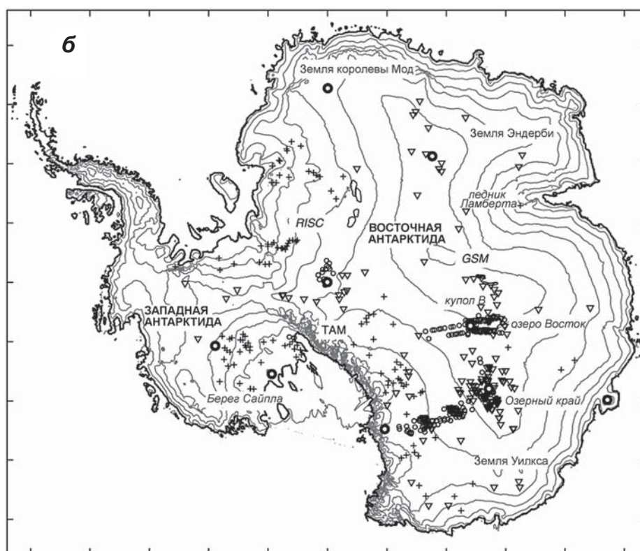
Антарктиды, где показаны следующие подледниковые озера (б): крупные (черными контурами), надежно различимые (треугольниками), малоконтрастные (кружками), активные (крестами). Черными точками показаны места измерений температуры льда в скважинах, черной линией – современное положение линии налегания. Буквами обозначены: TAM – Трансантарктические горы; RISC – бассейн ледяного потока Рекавери; GSM – подледные горы Гамбурцева (Pattyn, 2010) ▲
