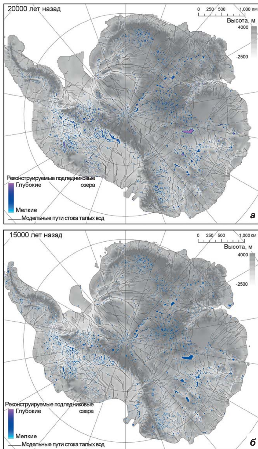
▲ ► Рис. 4.130. Реконструированные пути стока и подледниковые озера Антарктиды ➡
