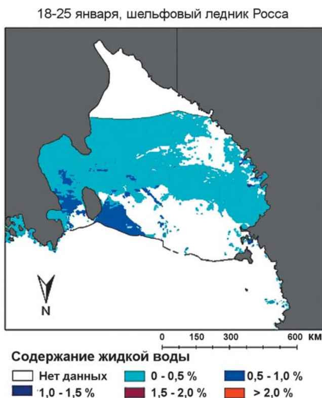
▲ Рис. 2.4. Содержание жидкой воды в снежном покрове шельфового ледника Росса 2–9 января 2003 г. по данным MODIS (Lampkin, Karmosky, 2009)
