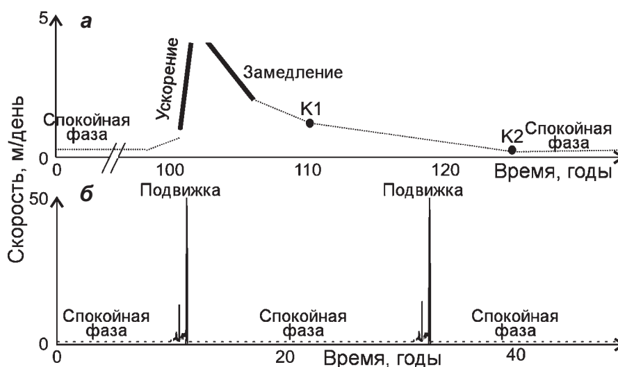
▲ Рис. 1.21. Схема динамики подвижки ледника Монако и других ледников Свальбарда (а). Жирные линии – данные по леднику Монако (Murray et al., 2003b), пунктирная линия – ранняя медленная часть фазы ускорения ледника (Murray et al., 2003a), точки K1 и K2 соответствуют изменениям скорости примерно через 20 и 45 лет после начала подвижки ледника Конгсвеген (Melvold, Hagen, 1998). Подвижка ледника Вариегейтед по данным (Kamb et al., 1985) (б). Спокойная фаза характеризуется сезонными циклами скорости с более быстрым течением летом, чем зимой (Raymond, Harrison, 1988), и минисёрджками (Kamb, Engelhardt, 1987) (на рисунке не показаны). Инициация подвижки ледника была менее резкой, чем ее прекращение, в противоположность леднику Монако (Murray et al., 2003)
