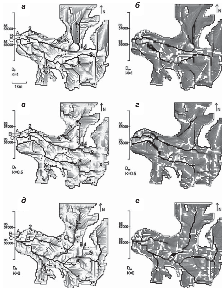
▲ Рис. 4.33. Схемы подледникового дренажа на леднике Вереншельд, полученные методами D_8 (а, в, д) и D_\infty (б, г, е) при разных отношениях давления воды P_w , льда P_i и воздуха P_a : P_w = P_i (а, б); P_w = 0,5P_i (в, г); P_w = P_a (д, е). Черными квадратами с цифрами показаны ледниковые колодцы. Криокарстовые депрессии обозначены кружками, выходы вод в верхней части ледника – знаком X; центральный выход воды на языке с тремя отдельными ветвями – буквами А, В и С; ледниковый ручей Kvisla I, образующийся в случаях (а) и (б) – черными стрелками (Pälli et al., 2003)
