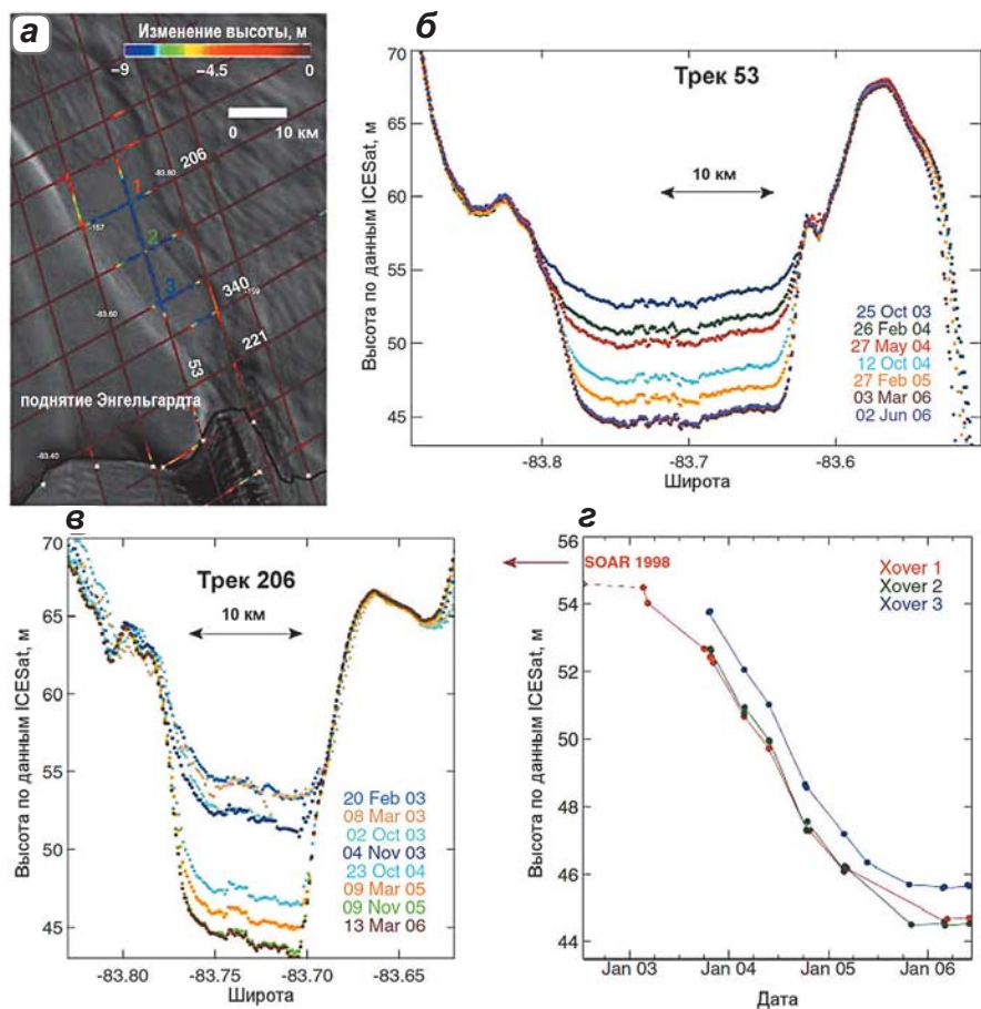
▲ Рис. 4.93. Изменение высоты поверхности над подледниковым озером Энгельгардта с октября 2003 г. по ноябрь 2005 г. по данным лазерной альтиметрии ICESat (а) и над тем же озером на поперечных профилях 53 и 206 с интервалами 91 день (б, в); изменения высоты поверхности ледника в трех точках над центральной частью озера (г) (Fricker et al., 2007)
