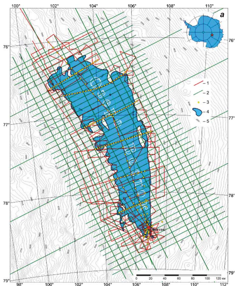
▲ ► Рис. 4.85. Границы и глубина подледникового озера Восток по данным радиозондирования и сейсмозондирования: а) геофизические исследования 1998–2008 гг. 1) профили радиозондирования 44–53 РАЭ (1998–2008 гг.); 2) маршруты американской аэрогеофизической съемки 2000–2001 гг.; 3) пункты зондирования МОВ 41–53 РАЭ (1995–2008 гг.);
