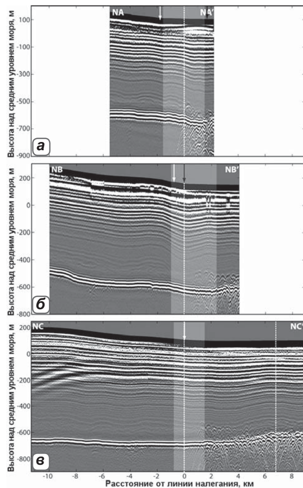
◀▶ Рис. 2.150. Радарные записи вдоль профилей NA-NA' (а), NB-NB' (б), NC-NC' (в), RA-RA' (г), SA'-SA (д), SB'-SB (е), SC'-SC (ж) на куполе Сайпл и о. Рузвельт. Положение профилей показано на рис. 2.149. Черная и белая стрелки показывают положение стратиграфического погружения верхних слоев и перегиб склона поверхности; область гидростатического равновесия находится в районе линии налегания на 0 км (зона ее возможного положения выделена прозрачным белым цветом) (Catania et al., 2010)
