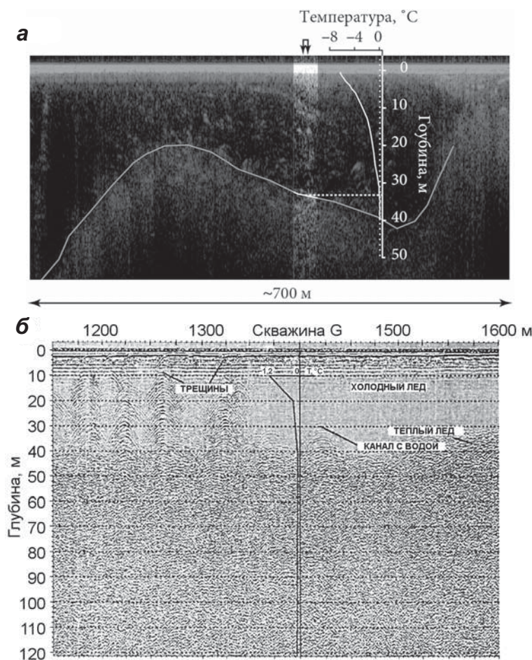
▲ Рис. 2.31. Глубина внутреннего отражающего горизонта на ледниках Стур (Pettersson et al., 2004) (а) и Ханс (Moore et al., 1999) (б) по данным радиозондирования на частотах 800 МГц (а) и 50 МГц (б) и измерений температуры льда в скважинах. Характер внутренних отражений изменяется на глубинах около 33 м (а) и 40 м (б), где температура льда достигает 0 °С
