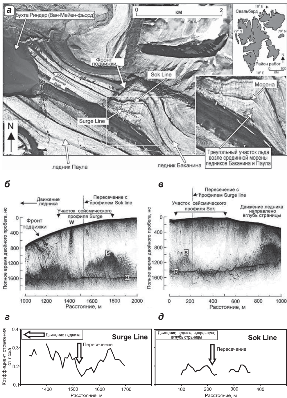
▲ Рис. 2.119. Профили сейсмических и радиолокационных измерений на леднике Баканина (а); радарные отражения вдоль профилей, частично перекрывающих сейсмические профили MOB Sok Line и Surge Line (б, в), буквами S и B обозначены отражения от придонного теплого льда и ложа; коэффициент отражения вдоль профилей Sok Line и Surge Line (г, д) (Smith et al., 2002)
