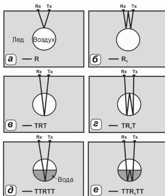
► Рис. 2.59. Пути распространения радиоволн через внутриледниковый канал круглого сечения: а, б) однократное ( R ) и двукратное ( R_3 ) отражение от крыши воздушного канала; в, г) однократное (TRT) и двукратное ( TR_3T ) отражение от дна канала, заполненного воздухом; д) отражение (TTRT) от дна канала, частично заполненного водой; е) двукратное отражение ( TTR_3TT ) от поверхности воды и дна канала, частично заполненного воздухом и водой (Stuart et al., 2003)
