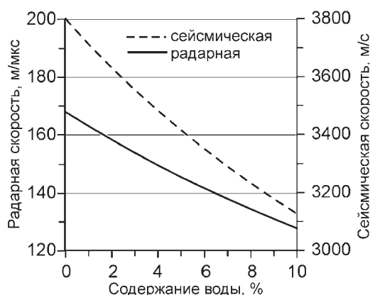
◀ Рис. 2.41. Зависимость скорости распространения сейсмических Р-волн и радиоволн от содержания воды в теплом льду (Benjumea et al., 2003)
