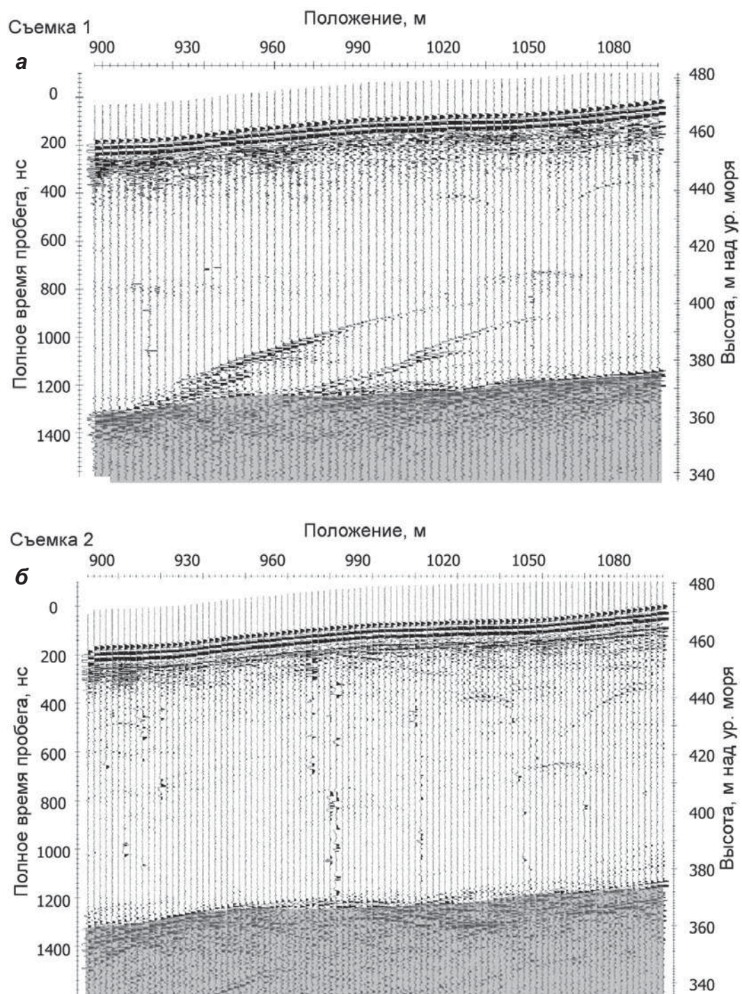
▲ Рис. 4.14. Профиль V17 (см. рис. 4.11). На (а) видны квазилинейные отражения, которые отсутствуют на (б) (Irvine-Fynn et al., 2006)
