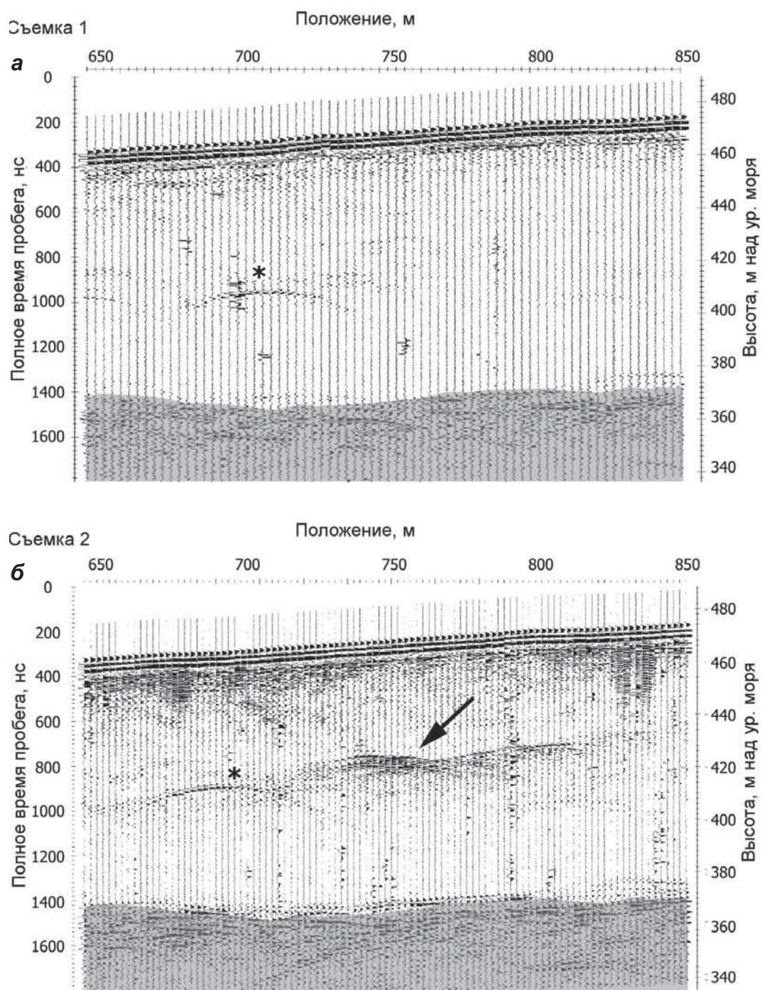
▲ Рис. 4.15. Профиль V1 (см. рис. 4.11). На (а) видно гиперболическое отражение (отмечено звездочкой), которое также видно на (б), но исчезло во время третьей съемки. Увеличение интенсивности близповерхностных отражений, вероятно, связано с ростом содержания воды у поверхности (Irvine-Fynn et al., 2006)
