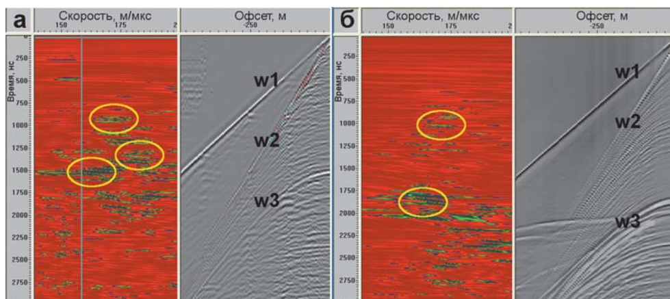
▲ Рис. 3.16. Профиль скорость–глубина (дальность), полученный с применением итеративного скоростного сембланс-анализа данных ОГТ-измерений на леднике Фритьоф в 2005 г. Типы волн: W1 – прямая воздушная волна, W2 – волна вдоль поверхности ледника, W3 – отражение от ложа. Кружками показаны отражения от скоплений воды в леднике (Василенко и др., 2006)
