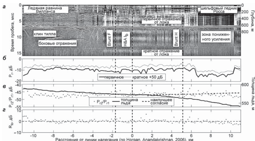
▲ Рис. 2.88. Радарная запись на частоте 2 МГц вдоль профиля W1; положение линии налегания 'H&A lb' (по Horgan, Anandakrishnan, 2006) и точек F и H по данным (Brunt et al., 2010) взято из рис. 2.87 и показано вертикальными пунктирными линиями (а); мощность, дБ, однократных ( P_1 ) и двукратных ( P_2 ) отражений от ложа (тонкая и толстая линии), осредненная по среднему радиусу первой зоны Френеля (160 м); для отражений P_2 шкала интенсивности увеличена на 50 дБ (б); отношение интенсивностей отражений P_2/P_1 (точки), толщина льда (сплошная линия) определена методом наименьших квадратов из уравнения (2.83) (в); коэффициент отражения от ложа R_{lb} ; горизонтальная пунктирная линия – коэффициент отражения от гладкой границы лед–морская вода (–0,16 дБ) (г) (McGregor, 2011)
