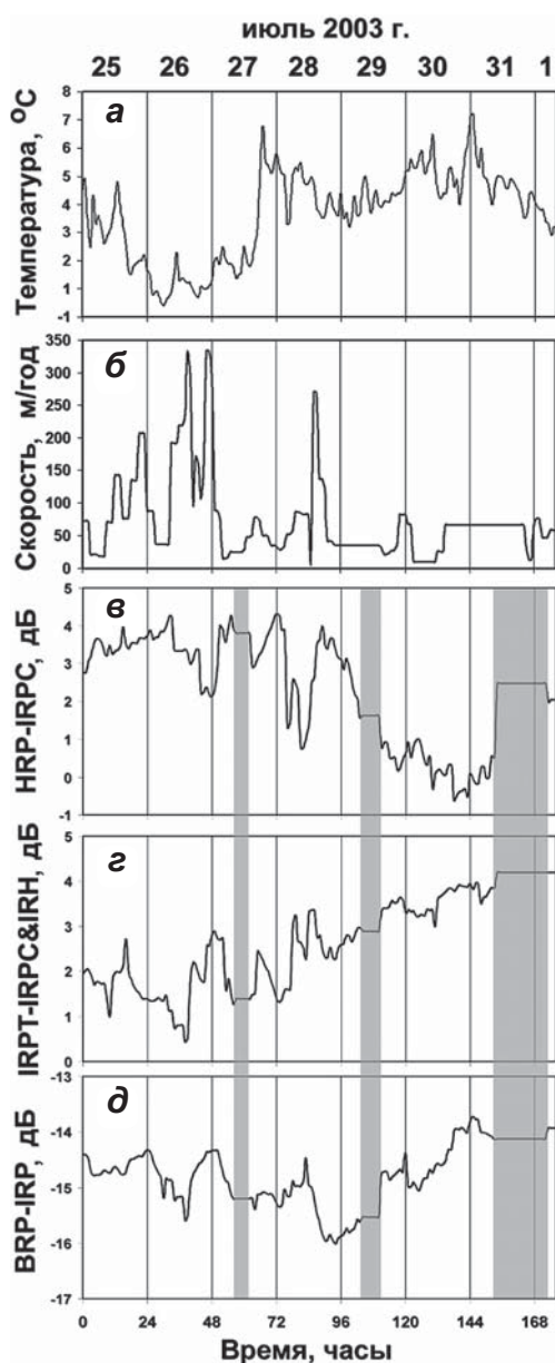
▲ Рис. 3.7. Изменение температуры воздуха (а), поверхностной скорости (б), мощности отражений из слоя холодного льда и от границы раздела холодного и теплого льда HRP–IRPC (в), из слоя холодного и теплого льда IRPT–IRPC–IRH (г), из слоя теплого и льда и от ложа BRP–IRP (д) период таяния с 27 июля по 1 августа 2003 г. (Jania et al., 2005; Яния и др., 2005)
