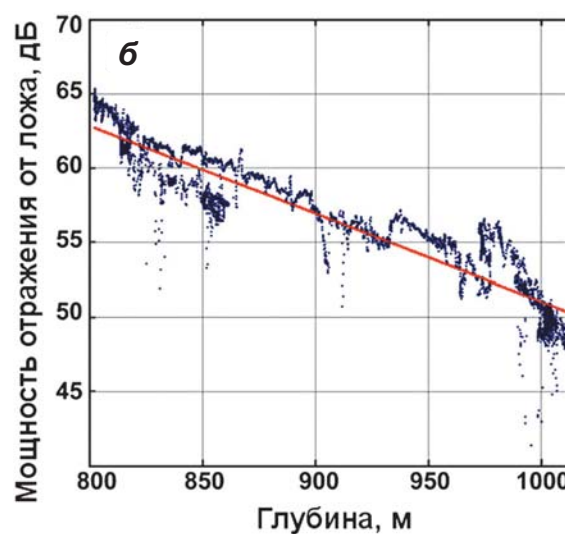
▲ ► Рис. 2.84. Профили радиозондирования на частоте 3 МГц на ледяном потоке Кэма (С) и куполе Сайпл и в районе «точки прилипания» с почти нулевыми скоростями течения льда (на вкладки) (а); мощность отражения от ложа, дБ, вдоль профиля А–А' как функция толщины льда, м (б); линейная регрессия (красная линия с коэффициентом корреляции r^2 = 0,89 соответствует удельному поглощению A = 29,5 \pm 0,3 дБ/км (Jacobel et al., 2009)
