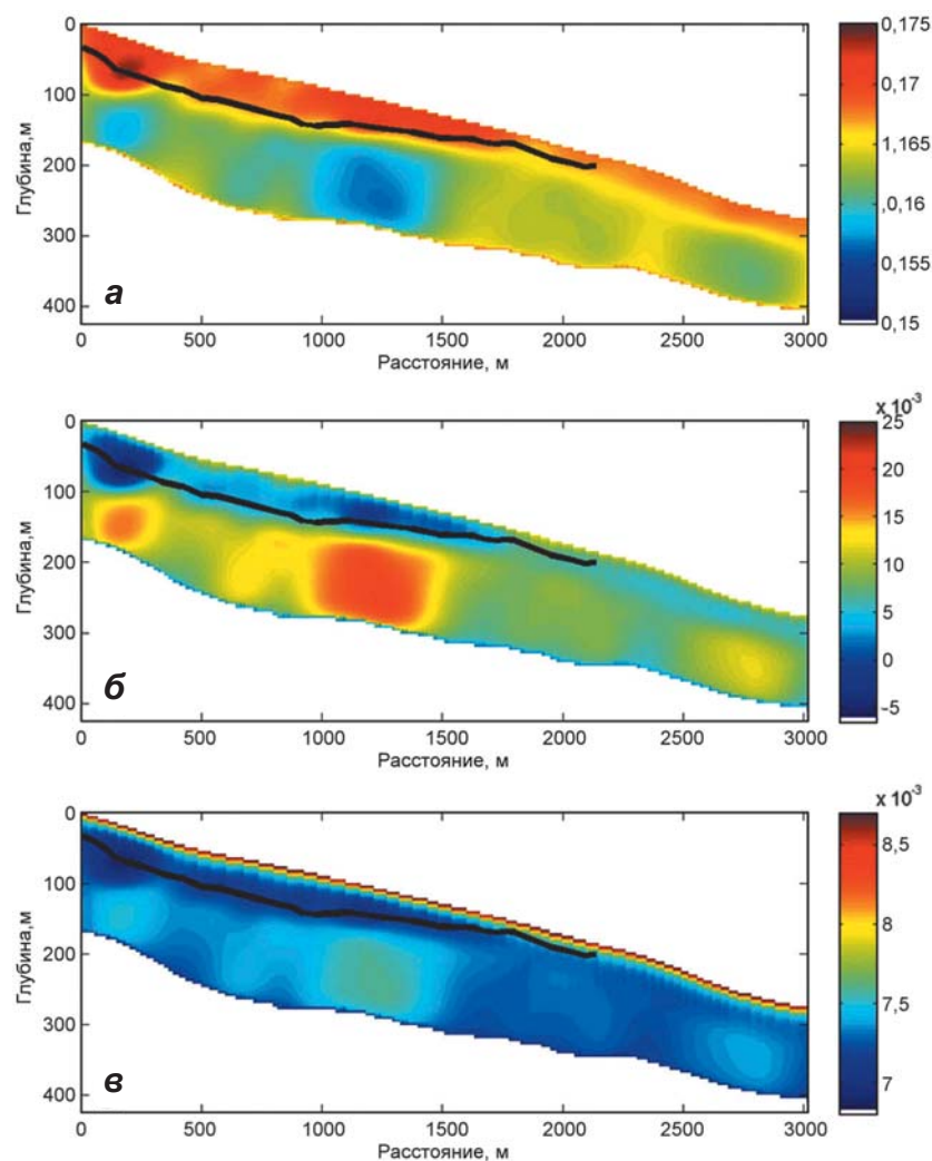
▲ Рис. 2.52. Результаты радиолокационных исследований на частоте 25 МГц вдоль продольного профиля ледника Бенч на Аляске (см. рис. 2.51, а): а) скоростная томографическая модель ледника по отраженным волнам; б) объемное содержание воды q_w в толще ледника, оцененное по формуле CRIM (2.35); в) неопределенность оценки q_w (Bradford et al., 2009)
