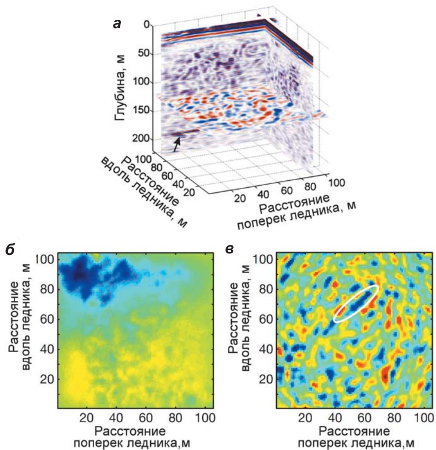
▲ Рис. 2.70. Трехмерное отображение амплитуд радарных отражений в толще ледника Бенч на Аляске по данным радиозондирования на частоте 50 МГц (теплые тона – положительные значения, холодные – отрицательные): три ортогональных сечения блока льда объемом 1,93 \cdot 10^6 \text{ м}^3 (а), стрелкой показано отражение от ложа на глубине около 175 м; горизонтальный срез на глубине 16 м, где практически отсутствуют сильные отражающие объекты (б), горизонтальный срез на глубине 137 м (примерно в 38 м от ложа) с многочисленными отражателями, некоторые из них протягиваются на десятки метров (например, участок, выделенный эллипсом) (в) (Harper et al., 2010)
