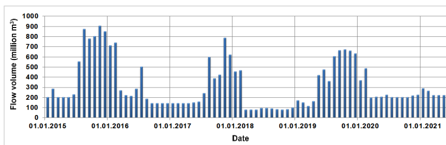
Рисунок 2-27 Динамика среднемесячных объемов потока в Русловом водохранилище в 2015-2021 годах
