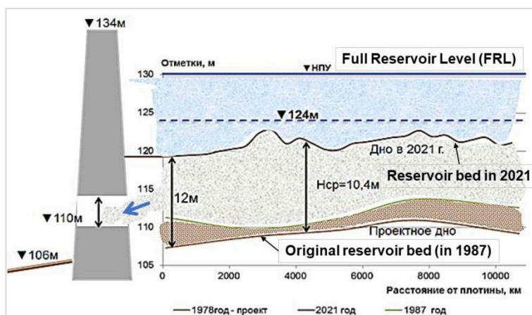
Рисунок 2-28 Схематическое изображение заиливания возле головных сооружений (М. Икрамова, 2021)
