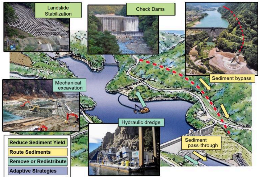
Рисунок 5-2 Варианты и стратегии решения проблем заиления в водохранилищах (Рэндл и др., 2019)
