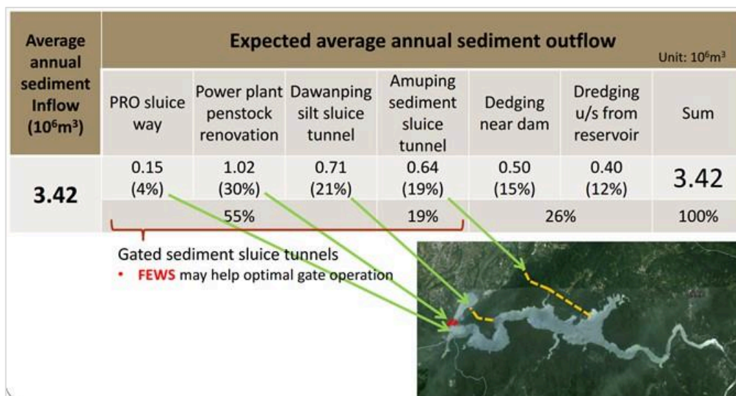
Рисунок 5-6 Существующие и предлагаемые меры управления наносами в водохранилище Шимэнь и ожидаемые результаты реализации (предоставлено: Джинн Чанг Янг)
