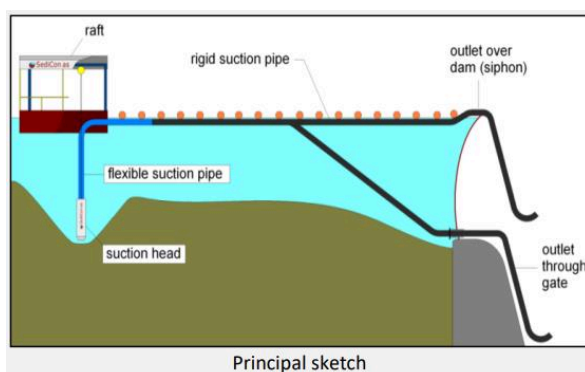
Рисунок 3-16 SediCon Dredge – гидровсасывающая система, использующая имеющийся напор между водохранилищем и выпуском отводной трубы для откачки воды и наносов (таким образом, не требует энергии). Типичная средняя мощность варьируется от 50 м³ вязких наносов в час с 200 мм снарядами до 1000 м³ в час песчаных материалов с 500 мм снарядами ( www.sedicon.no ).
