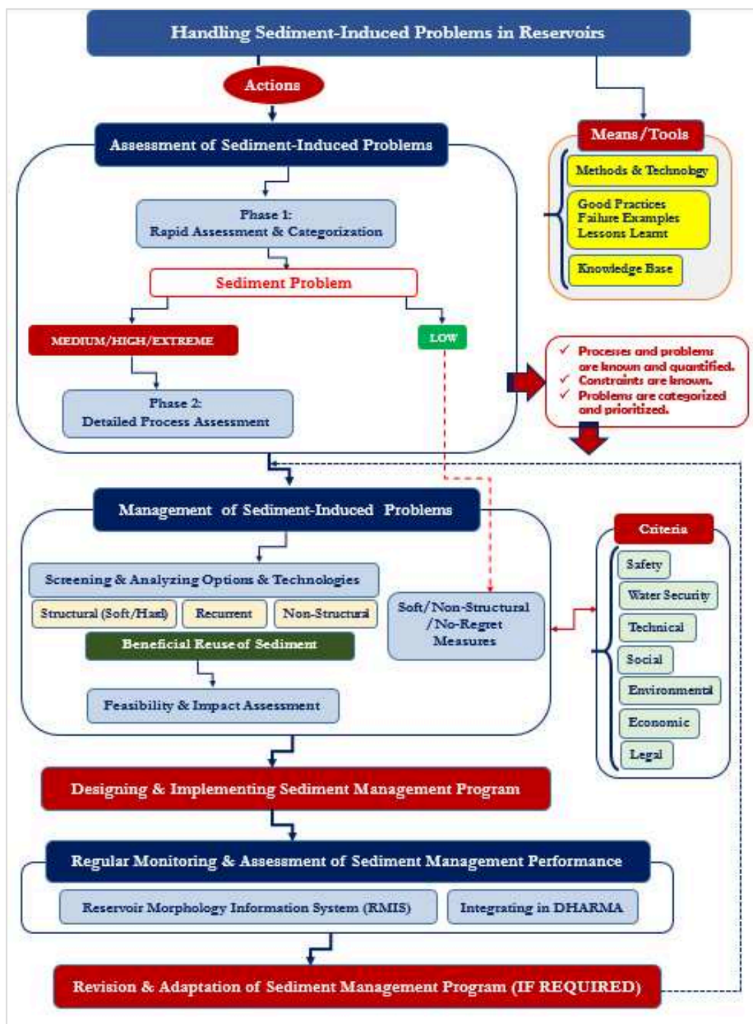
Рисунок 5-1 Схематическое изображение мер и инструментов для решения проблем заиления в водохранилищах (Гури и др., 2019)
