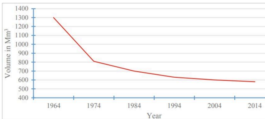
Рисунок 5-11 Динамика потери объема водохранилища Хашм Эль Гирба во времени
