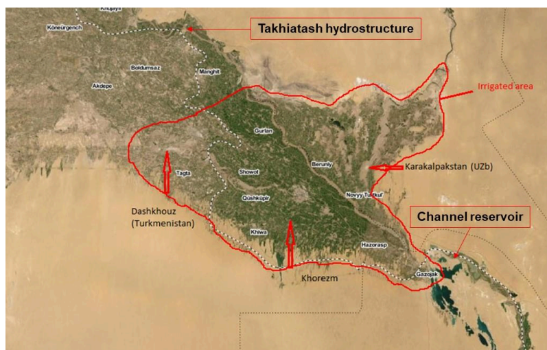
Рисунок 2-10 Зона, орошаемая ТМГУ, в Узбекистане и Туркменистане
