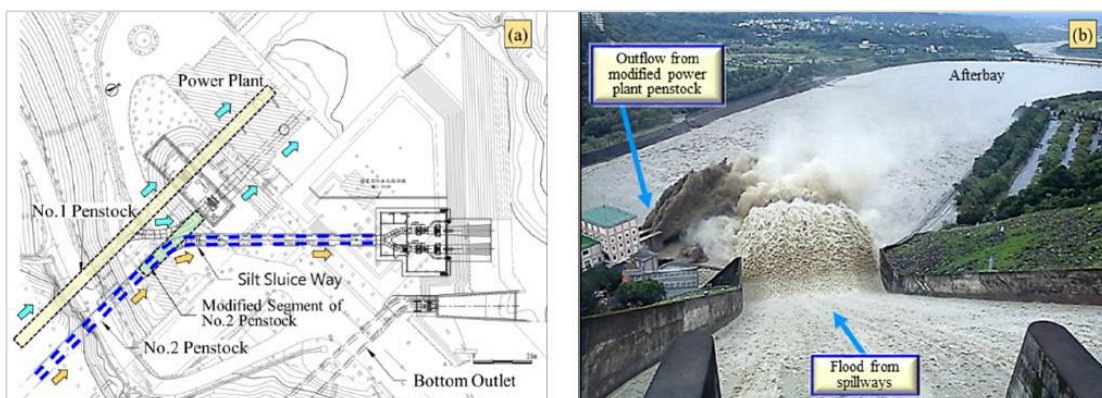
Рисунок 5-4 Измененный участок второго напорного водовода, используемого для промывания наносов (чертеж слева, и промывание наносов через измененный напорный водовод и водосброс (изображение справа) во время первой операции в 2013 году, когда произошел тайфун (Ли и др., 2022)
