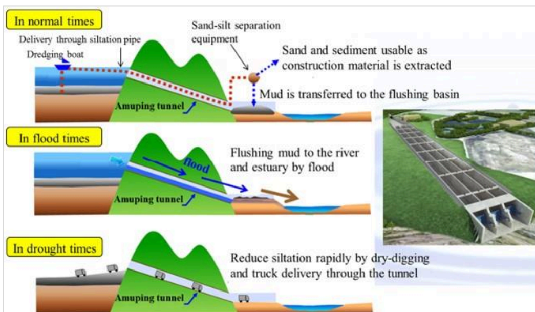
Рисунок 5-5 Функции и работа спроектированного обходного тоннеля (Лай, 2017)
