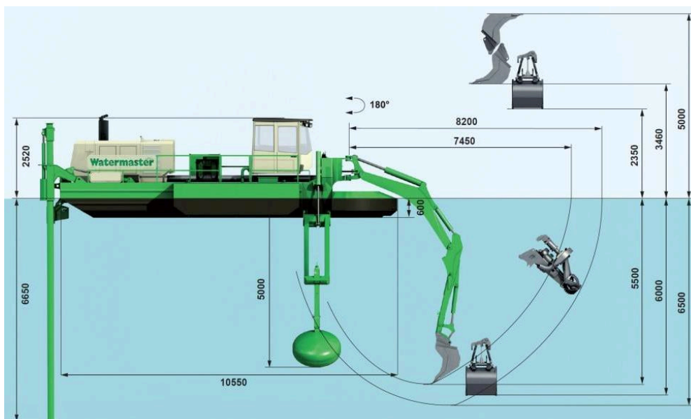
Рисунок 3-15 Водоходный многофункциональный Watermaster – подходит для сухих участков глубиной до 6,5 м; скорость откачки – 600-900 м³/час (при 10-30% твердых веществ) с максимальной дальностью откачки до 1,5 км. Коэффициент производства очень сильно зависит от разных условий, например, от состояния почвы, высоты и дальности откачки, наличия обломков или камней, опыта операторов, т.д. ( https://watermaster.fi ).
