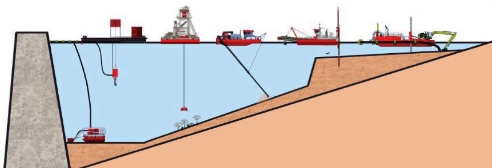
Рисунок 3-14 Различные дноуглубительные технологии для удаления наносов из водохранилища в зависимости от гидравлических и морфологических условий (предоставлено Royal IHC)
