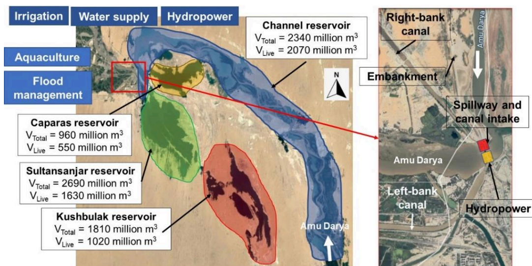
Рисунок 2-4 Комплекс водохранилищ (слева) и головные сооружения (справа)
