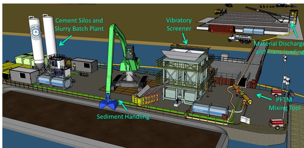
Рисунок 3-26 Плавучая система PFTM: мобильная операционная инженерная система переработки наносов (MOSES)
