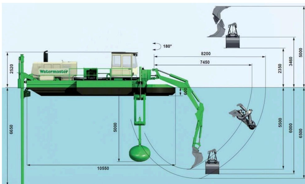
Рисунок 3-15 Водоходный многофункциональный Watermaster – подходит для сухих участков глубиной до 6,5 м; скорость откачки – 600-900 м 3 /час (при 10-30% твердых веществ) с максимальной дальностью откачки до 1,5 км. Коэффициент производства очень сильно зависит от разных условий, например, от состояния почвы, высоты и дальности откачки, наличия обломков или камней, опыта операторов, т.д. ( https://watermaster.fi ).
