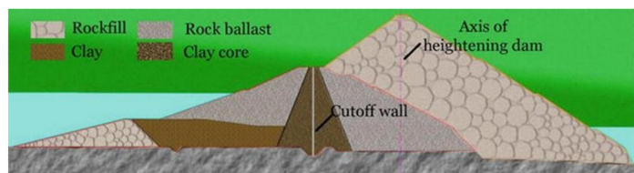
Рисунок 3-10 Повышение плотины Розейрес в Судане (изображение слева - http://pf.bbrnetwork.com/Projects/Manager/media287A-INFOslider_medium.jpg ) и профиль повышения плотины Жушу в Китае (график справа - https://www.intechopen.com/Chapters/71980 )
