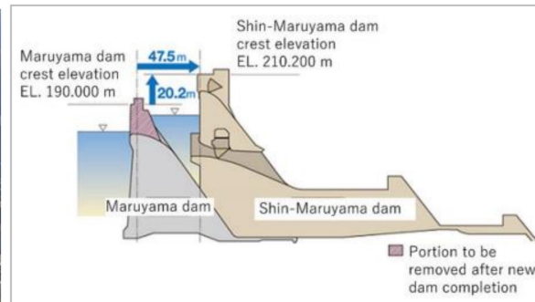
Рисунок 3-9 Опыт по наращиванию (перемещению) плотин в Японии: замена плотины Оюбари более крупной Юбари Шупаро (изображение слева – получено от И. Шимизу) и наращивание плотины Маруяма при помощи Шин-Маруяма (график справа - https://doi.org/10.20965/jdr.2018.p0585 )
