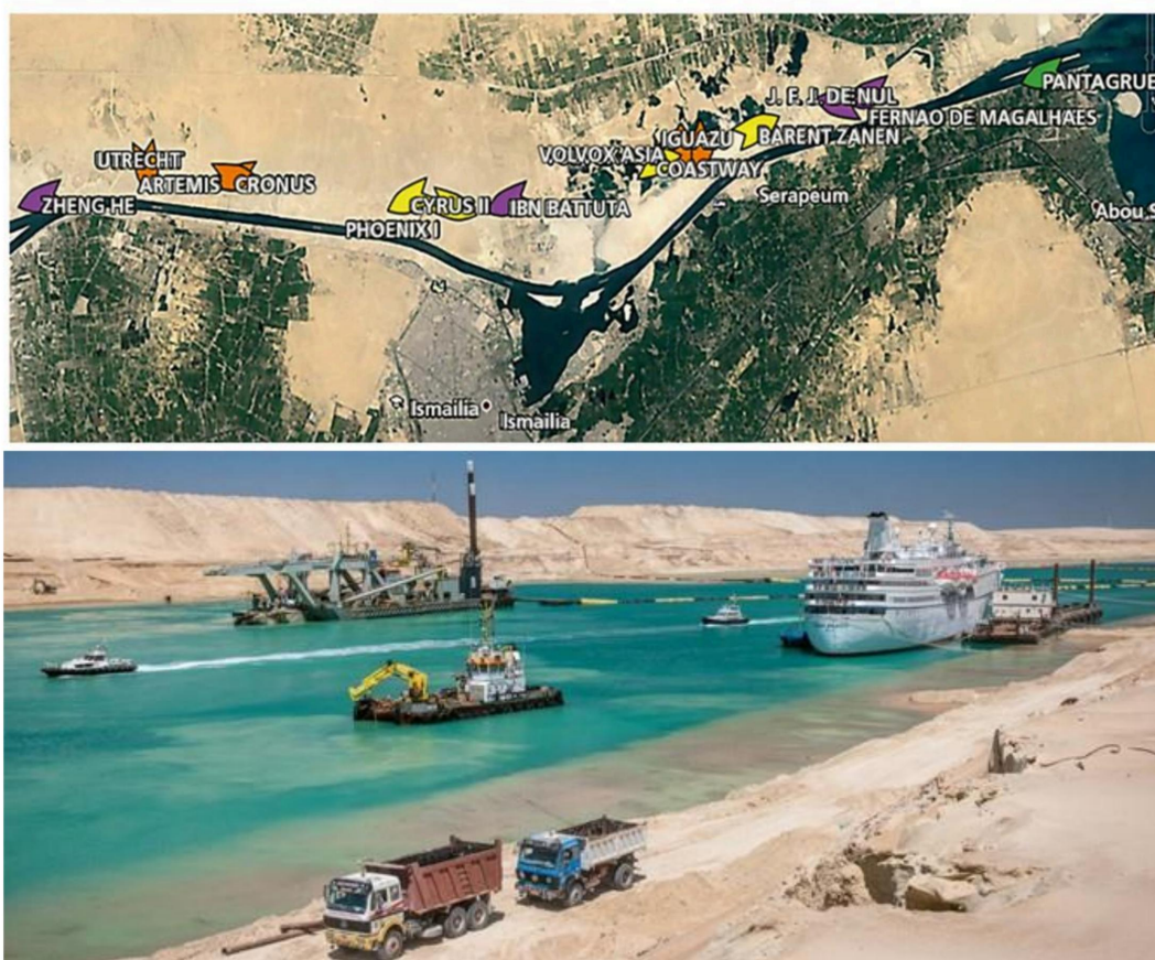
Рисунок 5-29 Спутниковое изображение разных видов землечерпательного оборудования Challenge Consortium на рабочей площадке (сверху) и изображение судов (снизу)
