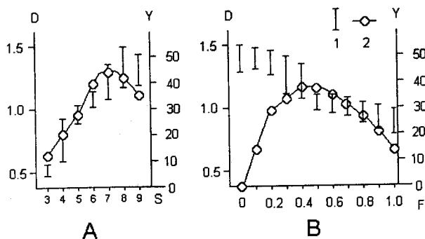
Рис. 4.12. Зависимость вылова ( Y ) и разнообразия генотипов популяции ( D ) в зависимости от селективности (А) и интенсивности (В) промысла. (1 — вариация разнообразия, 2 — вылов)
