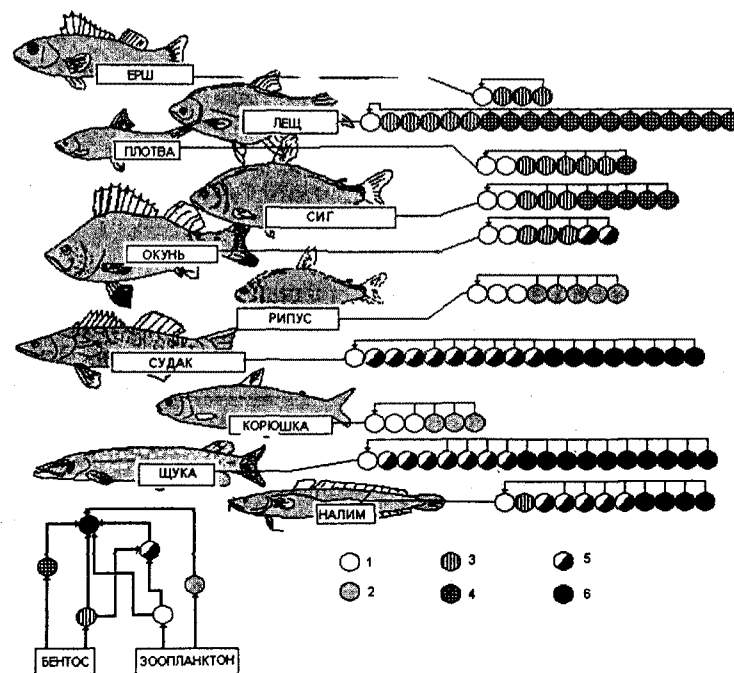
Рис. 6.11. Блок-схема сообщества рыб Ладжского озера (1 — мелкие планктофаги, 2 — крупные планктофаги, 3 — мелкие бентофаги, 4 — крупные бентофаги, 5 — мелкие хищники, 6 — крупные хищники)
