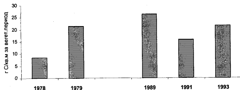
Рис. 5.3. Первичная продукция в заливе Большое Онего за вегетационный период в 1978–1979 и 1989–1993 гг. (по работе Тимаковой, Текановой, 1999)
