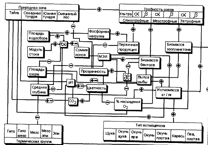
Рис. 1.19. Статистические связи в озерных экосистемах северо-запада России (по данным Китаева, 1986). МЭИ — морфоэдафический индекс (отношение суммы ионов к средней глубине озера), \alpha — коэффициент условного водообмена, \alpha — удельная прозрачность (прозрачность по Секки, деленная на среднюю глубину озера). Знак «+» указывает на проложительность связи, «-» на отрицательность, сочетание этих знаков соответствует многозначным связям
