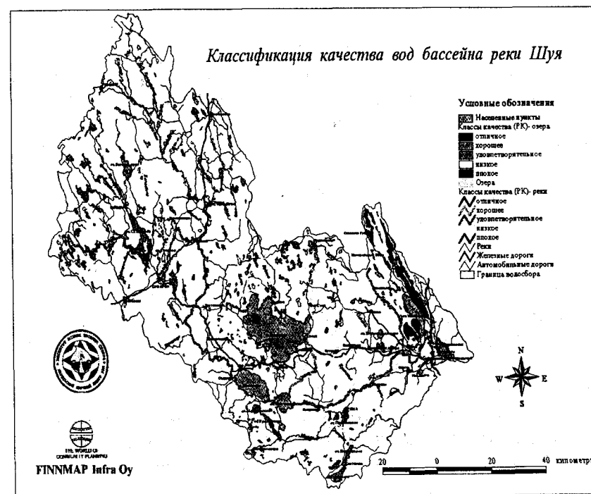
Рис. 6.2.5. Пример классификации водных объектов с использованием ГИС
