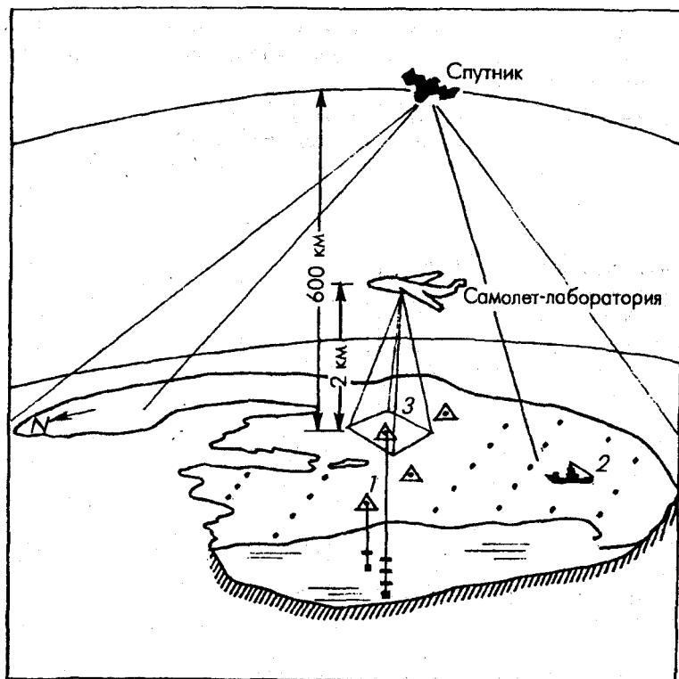
Рис. 6.3.1 Схема проведения эксперимента «Онго». На схеме показаны: спутник, самолет-лаборатория, суда и треугольниками места расположения автономных буйковых станций
