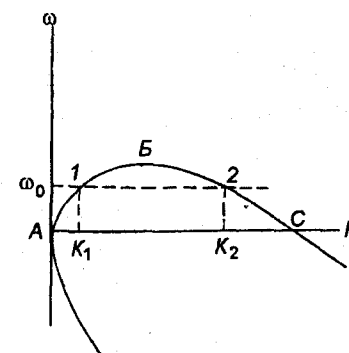
Рис. 4.6.4. Дисперсионное соотношение для гравитационных волн на встречном течении. Б — точка блокировки: 1 — прямая волна ( c_r > 0 ), 2 — отраженная волна
