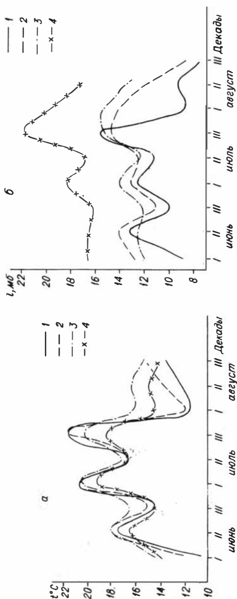
Рис.6. Изменение температуры воздуха (а) и абсолютной влажности (б) по природным комплексам: I - Бердский, 2 - Тальменский, 3 - Барабкинский, 4 - Кадиновский
