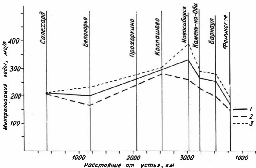
Рис.2. Изменение величины средней за зимний период минерализации воды по длине Оби в различные по водности годы I - средняя за период 1932-1956 гг.; 2 - 1947 г. (многоводный); 3 - 1956 г. (маловодный)
