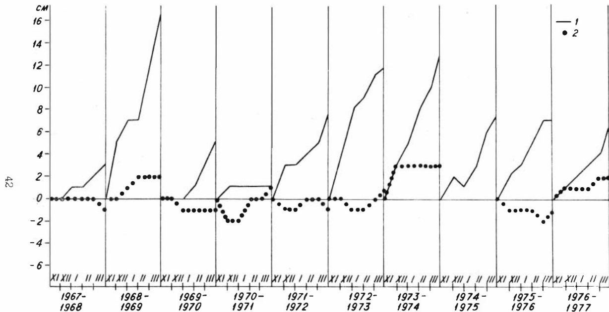
Рис.2. Ход приращения уровней в ледоставный период (ноябрь-март) I - оз. Бол.Чаны - п.Квашнино; 2 - оз.Яркуль (зимой 1974-1975гг. репер на Яркуле был поврежден)
