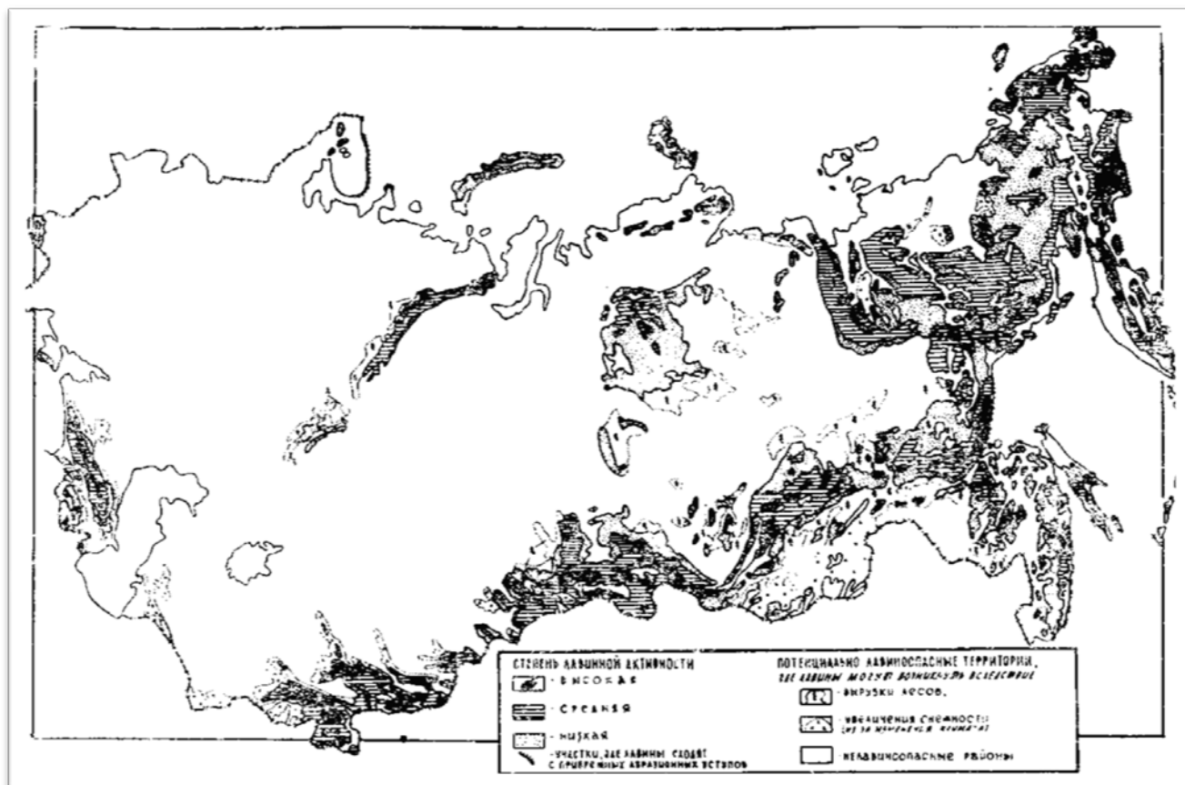
Рис. 48. СССР. Степень лавинной активности (см. табл. 8)
