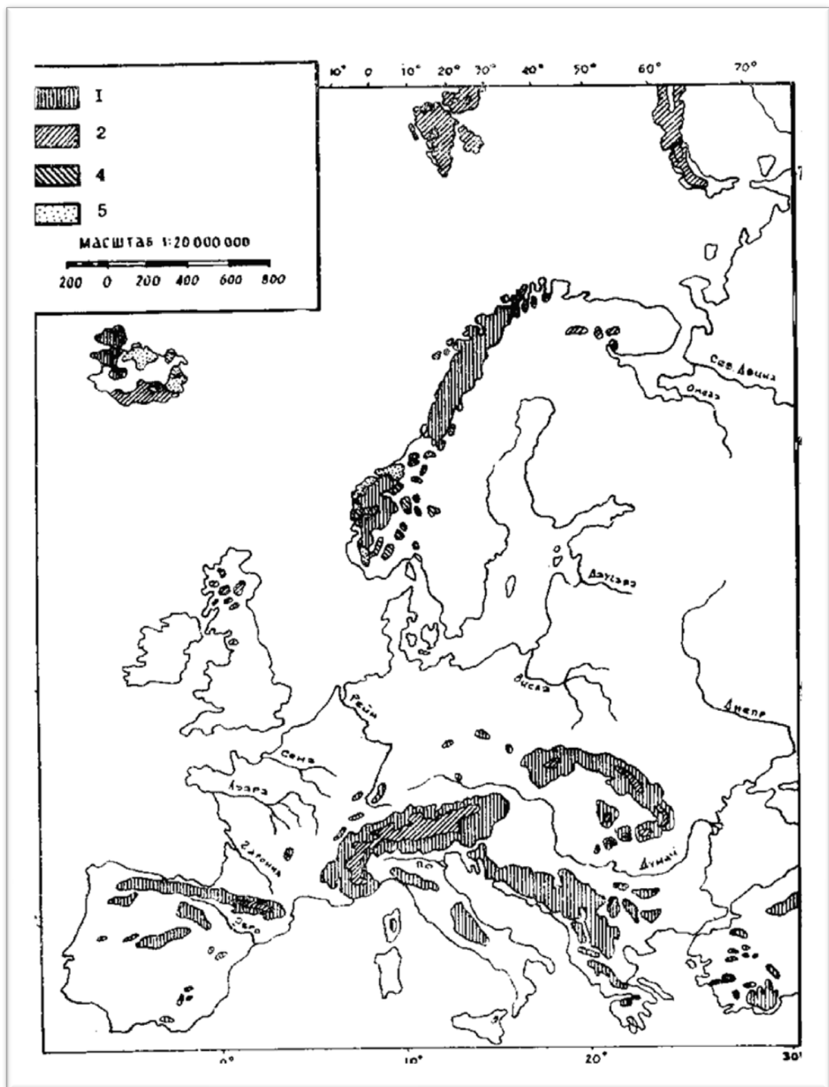
Рис. 34. Европа. Основные факторы лавинообразования: 1 — интенсивные снегопады; 2 — общие, низовые метели; 3 — перекристаллизация снежной толщи; 4 — весеннее снеготаяние; 5 — оттепели
