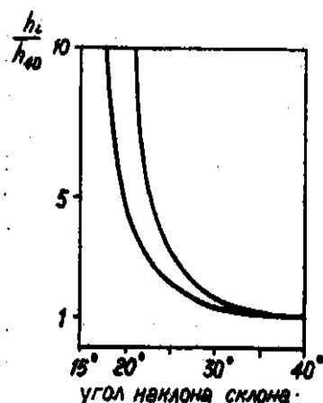
Рис. 1. Отношение критической высоты сухого снежного покрова h_i на склонах с разными углами наклона к его критической высоте на склоне с углом наклона 40^\circ h_{40} при значениях \operatorname{tg} \varphi = 0,36 (правая) и \operatorname{tg} \varphi = 0,30 (левая кривая)
