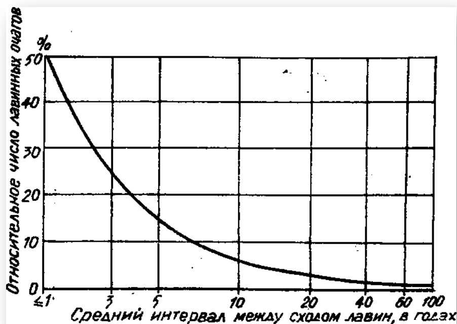
Рис. 6. Относительное число лавинных очагов с различной продолжительностью среднего интервала между сходом лавин, достигающих дна долины, в горах умеренного пояса (по данным К. Л. Абдушлишвили, В. Н. Аккуратова, М. Ч. Залиханова, И. В. Северского и др.)
