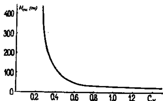
Рис. 22. Коэффициент вариации C_v для разных величин среднего многолетнего значения максимальной декадной высоты снежного покрова H_{ср} . По Е. С. Трошкиной
