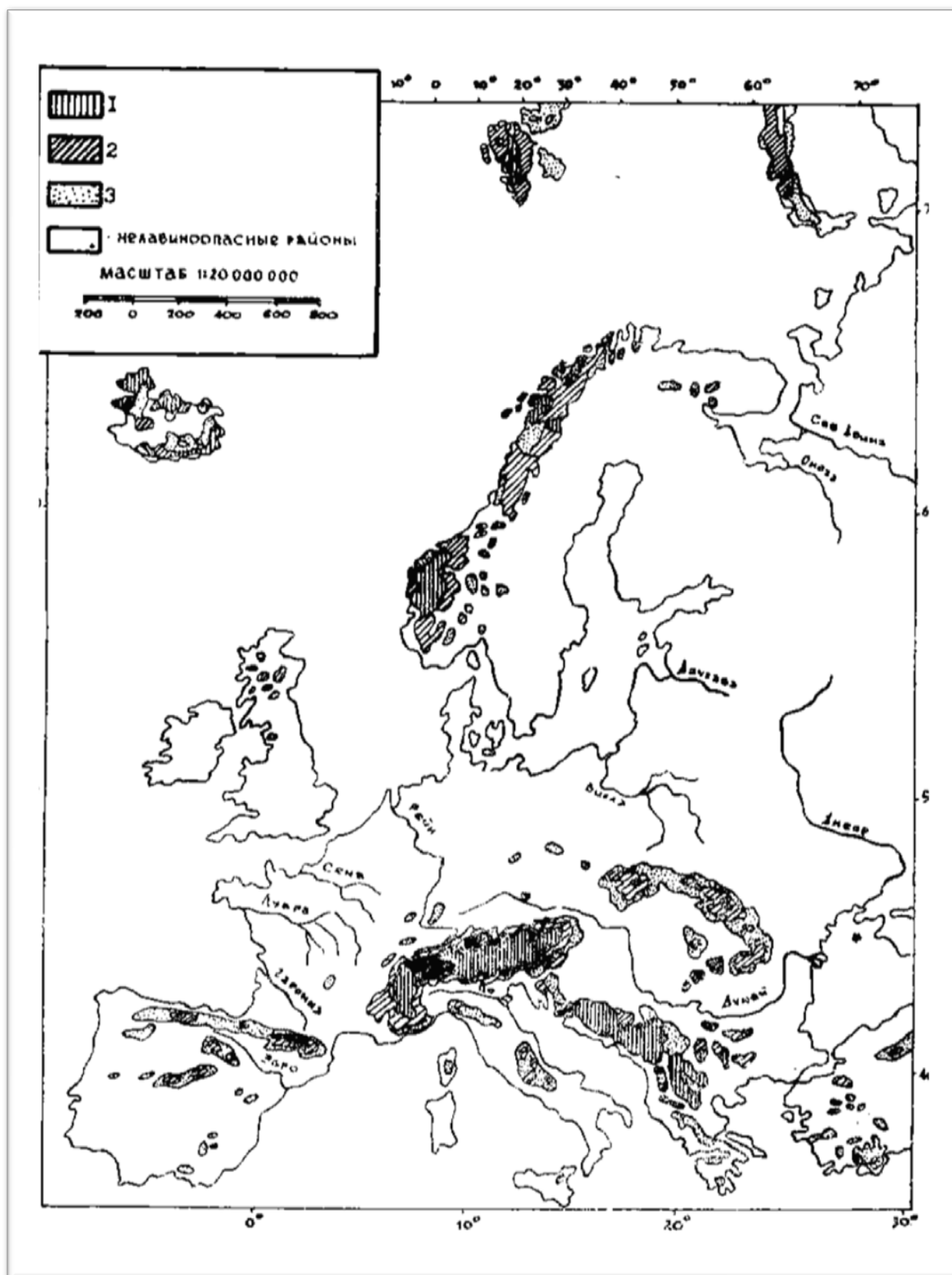
Рис. 35. Европа. Степень лавинной активности: 1 — высокая, 2 — средняя, 3 — низкая (см. табл. 8)
