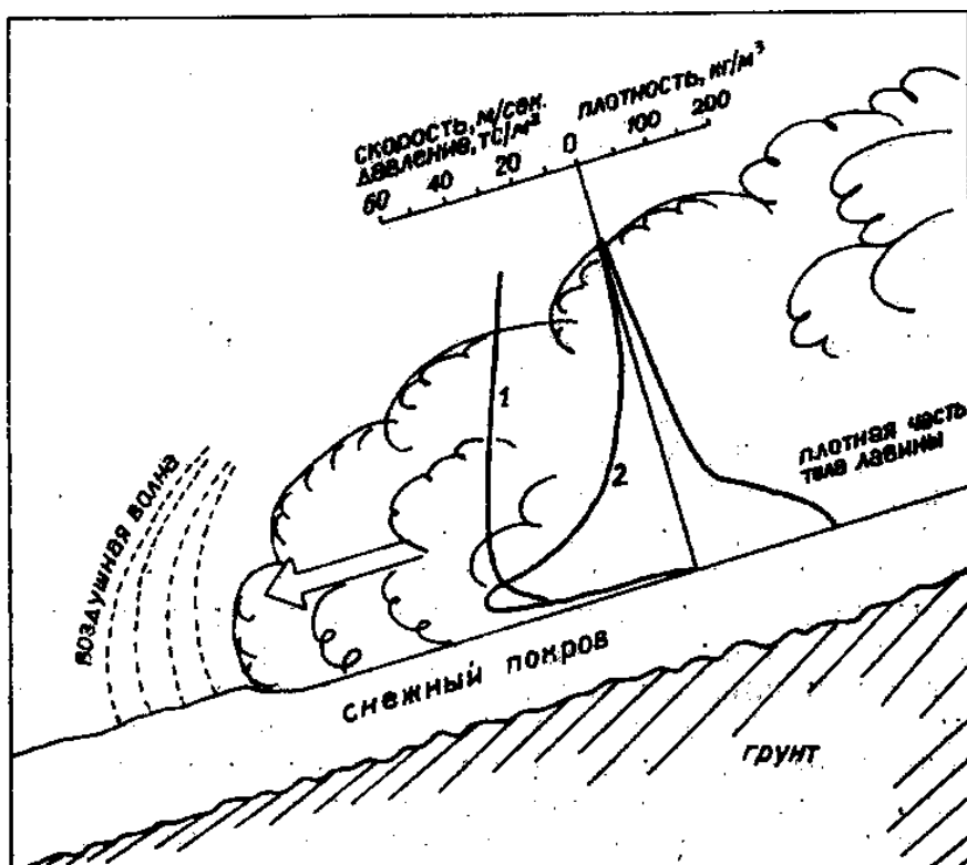
Рис. 5. Вертикальное распределение плотности, скорости, давления на препятствие лавины из сухого снега
