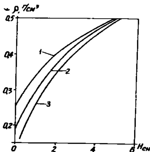
Рис. 18. Характерная плотность снега \rho при различной высоте снежного покрова H_{сн} для районов на 30—49° с. ш. (1), 50—59° с. ш.
