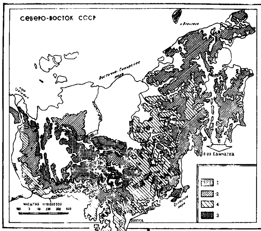
Рис. 65. Северо-Восток России и Камчатка. Основные факторы лавинообразования. Условные обозначения см. рис. 50
