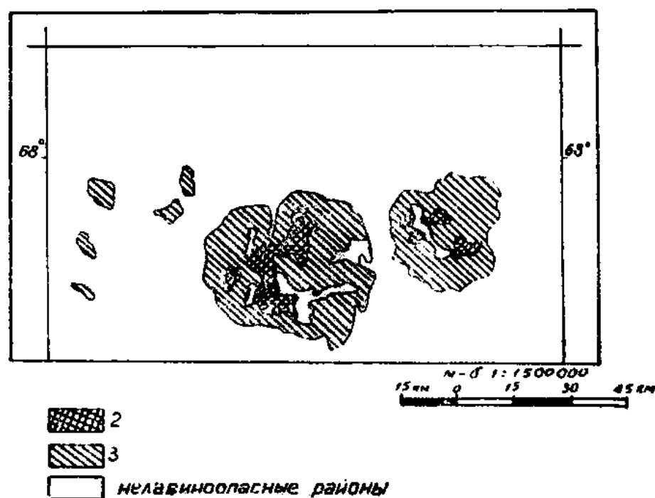
Рис. 52. Хибины, Полярный Урал. Средние суммарные объемы лавин за зиму из очага средних размеров: 1 — более 100 000 м 3 ; 2 — 10 000—100 000 м 3 ; 3 — менее 10 000 м 3
