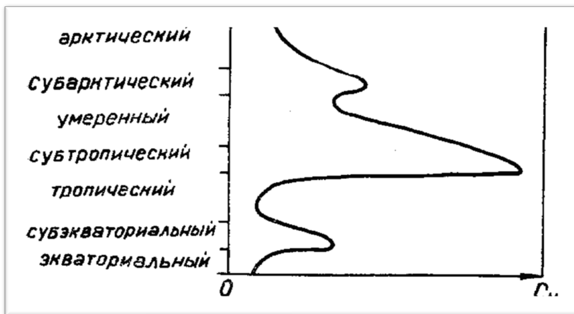
Рис. 26. Схема изменений коэффициентов вариации снежности C_v в горах разных климатических поясов. Сходным должно быть изменение вариабельности и других показателей снеголавинного режима
