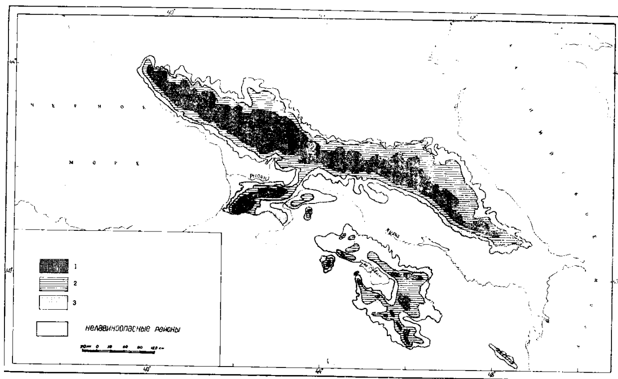
Рис 54. Кавказ. Повторяемость лавин Условные обозначения см. рис. 51
