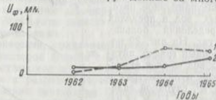
Рис. 33. Совмещенный график инфильтрационного питания грунтовых вод атмосферными осадками за февраль в период 1962—1965 гг. по данным лизиметров с насыпными (1) и монолитными (2) грунтами.
