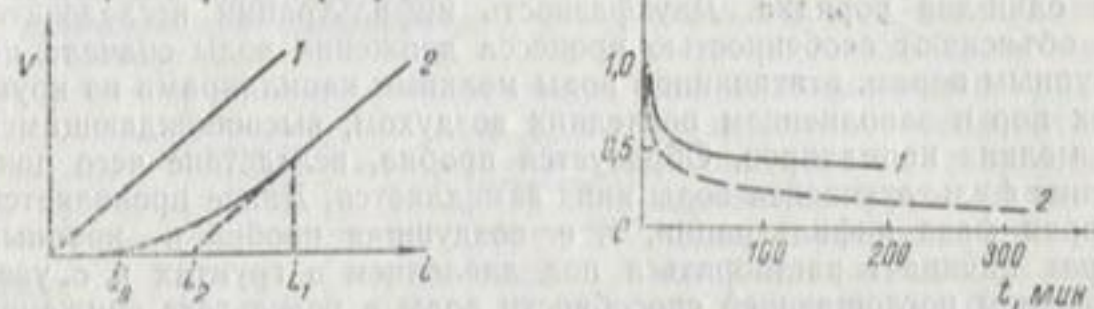
Рис. 27. Зависимость скорости движения воды от градиента (по Ц. Жакену): 1—по закону Дарси; 2—и действительности.
