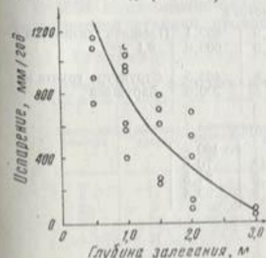
Рис. 5. Зависимость среднегодового испарения грунтовых вод от глубины залегания.
