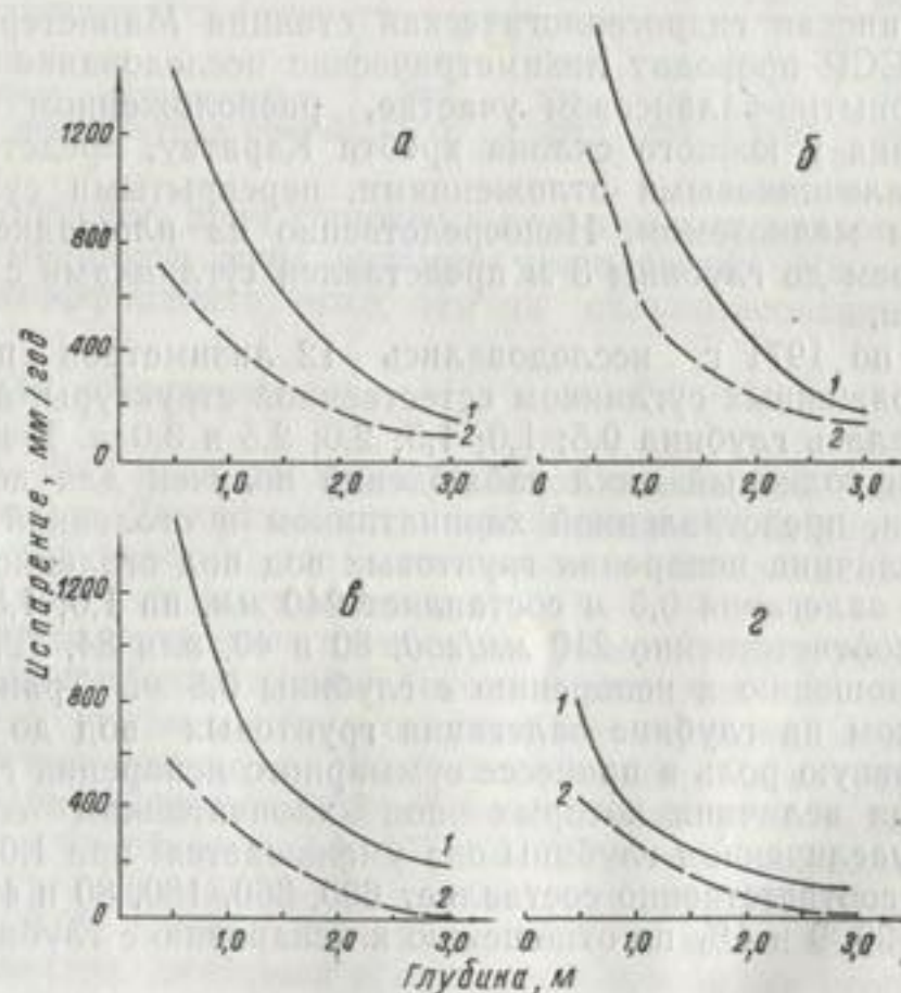
Рис. 10. Совмещенные графики зависимости испарения грунтовых вод от мощности зоны аэрации по зонам ничтожного (1) и скудного (2) увлажнения при различной деятельной поверхности:
