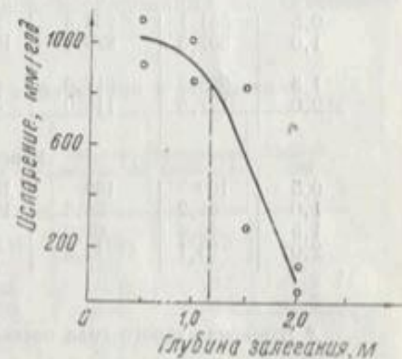
Рис. 5. Зависимость среднегодового испарения грунтовых вод от глубины залегания.
