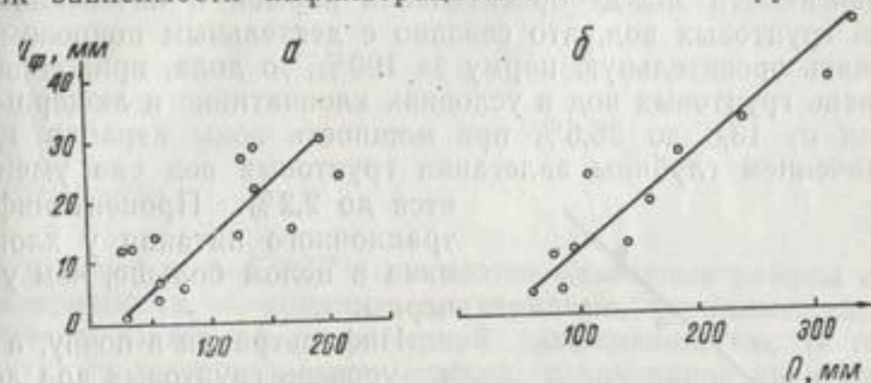
Рис. 42. Зависимость инфильтрационного питания грунтовых вод от месячной суммы оросительной воды:
