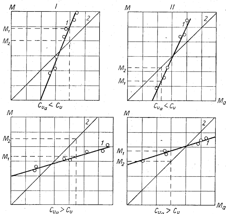
Рис. 7. Влияние смещения линии связи относительно начала координат на величину нормы стока. 1 — фактическая линия связи, ( C_v \cong C_{va} ), 2 — линия связи, проходящая через начало координат ( C_v = C_{va} ).
