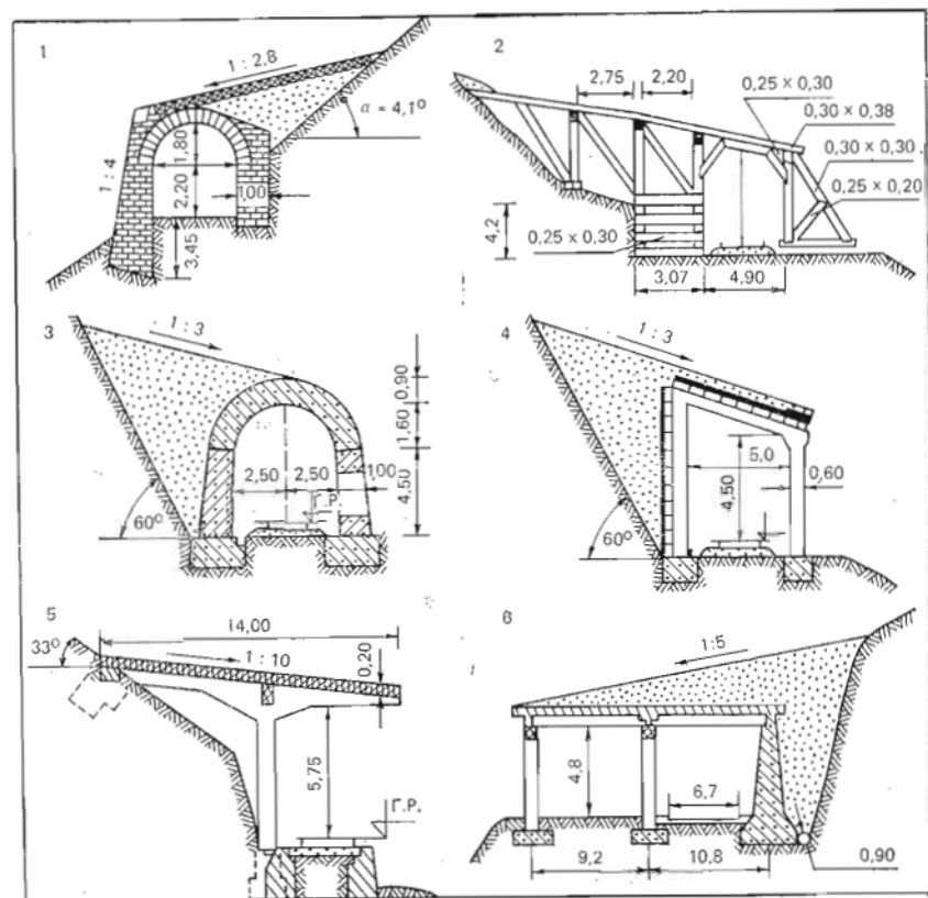
Рис. 11.5. Противолавинные галереи:
