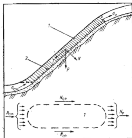
Рис. 4.5. Нарушение устойчивости плиты из плотного снега:
