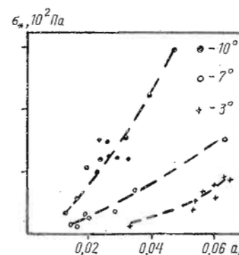
Рис. 3.10. Зависимость сопротивления снега разрыву \sigma от величины относительной контактной поверхности a_k
