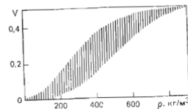
Рис. 3.4. Вероятные пределы изменений коэффициента бокового расширения снега v при одноосном сжатии (заштрихованная область) в зависимости от плотности
