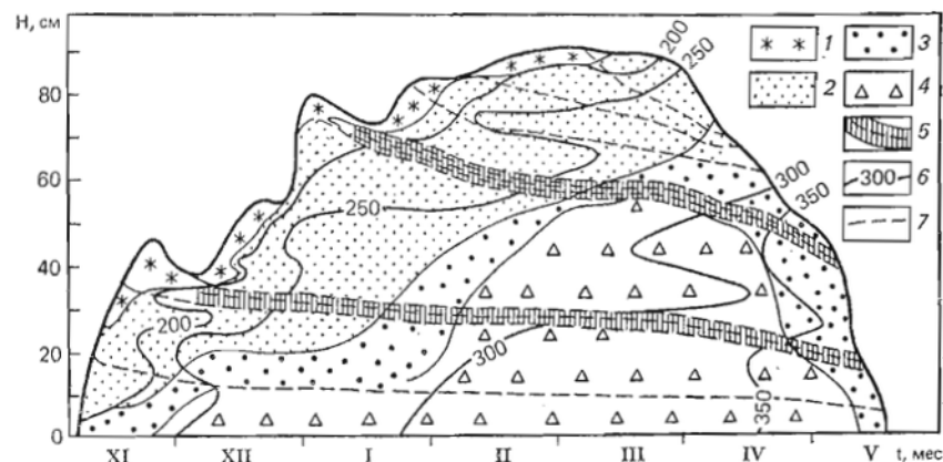
Рис. 2.3. Стратиграфический разрез снежного покрова в Хибинах (по наблюдениям Н. И. Лаптевой):
