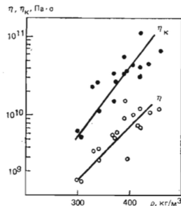
Рис. 3.6. Значения коэффициентов \eta и компрессионного \eta_k вязкости снежного покрова на склонах гор при температуре от -1 до -6^\circ
