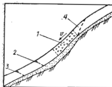
Рис. 4.6. Нарушение устойчивости плиты из слабо уплотненного снега:
