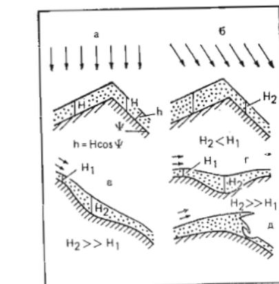
Рис. 2.2. Формирование снежного покрова: а — при снегопаде без ветра; б — при снегопаде со слабым ветром; в, г — при метелевом снегопереносе; д — формирование снежного карниза
