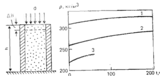
Рис. 3.3. Компрессионное уплотнение снега при \theta = -6^\circ под действием постоянной нагрузки \sigma = 15 \cdot 10^2 Па при начальной плотности \rho_0 : 1 — \rho_0 = 310 кг/м 3 ; 2 — \rho_0 = 260 кг/м 3 ; 3 — \rho_0 = 220 кг/м 3
