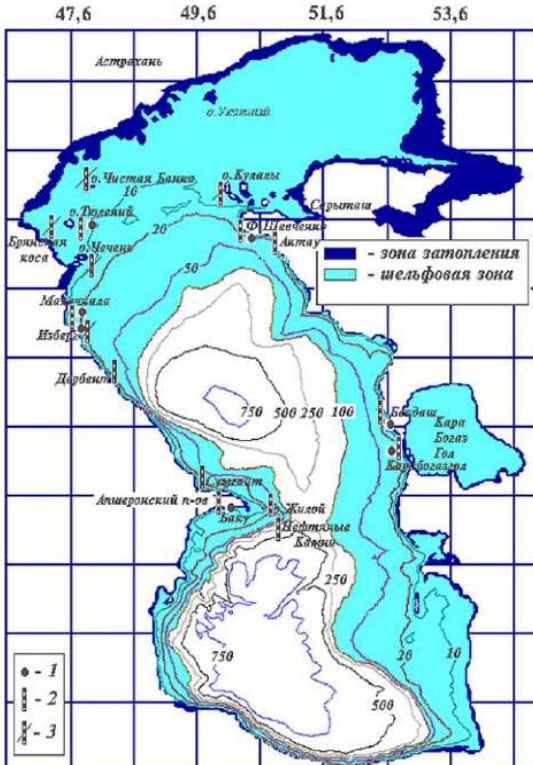
Рис. 2.1. Современная батиметрическая карта Каспийского моря с зонами затопления при положении среднего уровня (-28,00 м БС).
