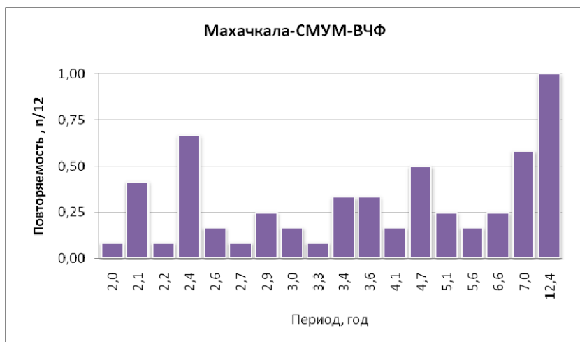
Рис. 4.14. Взаимосвязь между повторяемостью ( n/12 ) и периодом (в годах) гармоник временных рядов среднего месячного уровня моря на посту Махачкала после их модификации путем высокочастотной фильтрации.
