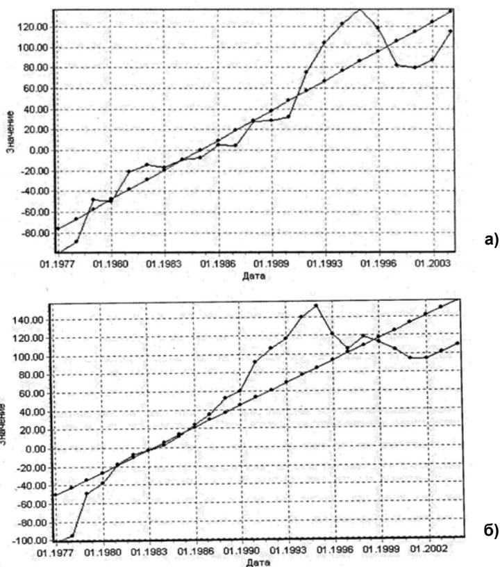
Рис. 3.11. Многолетний ход уровня моря и его тренд на ГМС: о. Тюлений (а); Махачкала (б).
