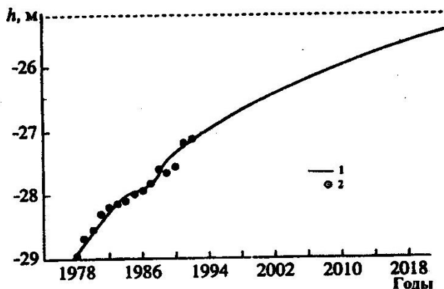
Рис. 8.31. График прогностического хода уровня с 1993 по 2020 г.: прогностическая кривая (1), фактические данные (2) [45].
