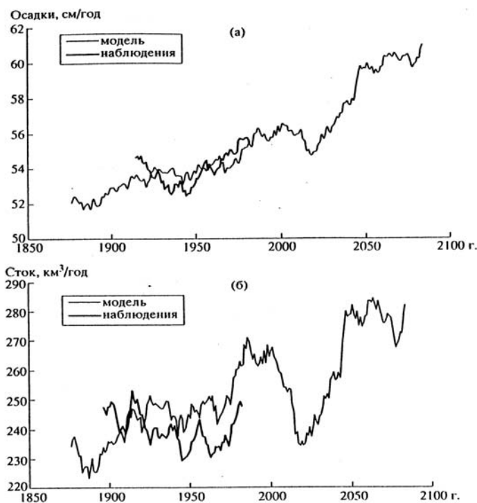
Рис. 8.24. Результаты моделирования с МОЦАО ЕСНАМ4/ОРУСЗ (тонкая линия) и данные наблюдений (30-летнее скользящее сглаживание) (жирная линия) по годовым осадкам на водосборе Волги (а) и ее стоку (б) [105].
