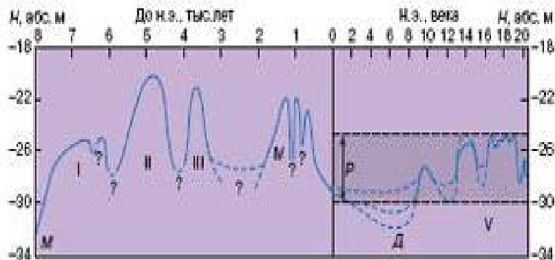
Рис. 4.2. Колебания уровня Каспийского моря за последние 10 тыс. лет [25]. Р – естественный размах колебаний уровня Каспийского моря при климатических условиях, свойственных субатлантической эпохе голоцена (зона риска); I–IV – стадии новокаспийской трансгрессии; М – мангышлакская, Д – дербентская регрессии.
