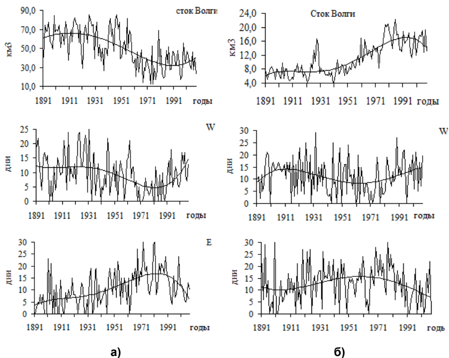
Рис. 6.3. Многолетняя сезонная изменчивость стока Волги (км³) (верхняя панель) и повторяемости атмосферной циркуляции западного (W) и восточного (E) типов (в днях): в июне (а), январе (б).
