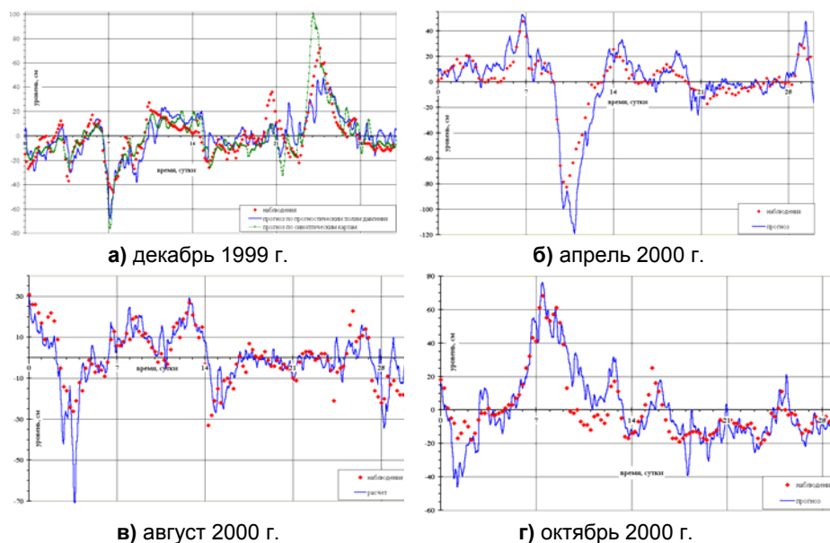
Рис. 9.4. Верификация модели по данным наблюдений на о. Тюлений. Точки – данные наблюдений, синяя линия – результаты расчетов по прогностическим полям приземного атмосферного давления, зеленая линия – результаты расчетов по синоптическим картам.
