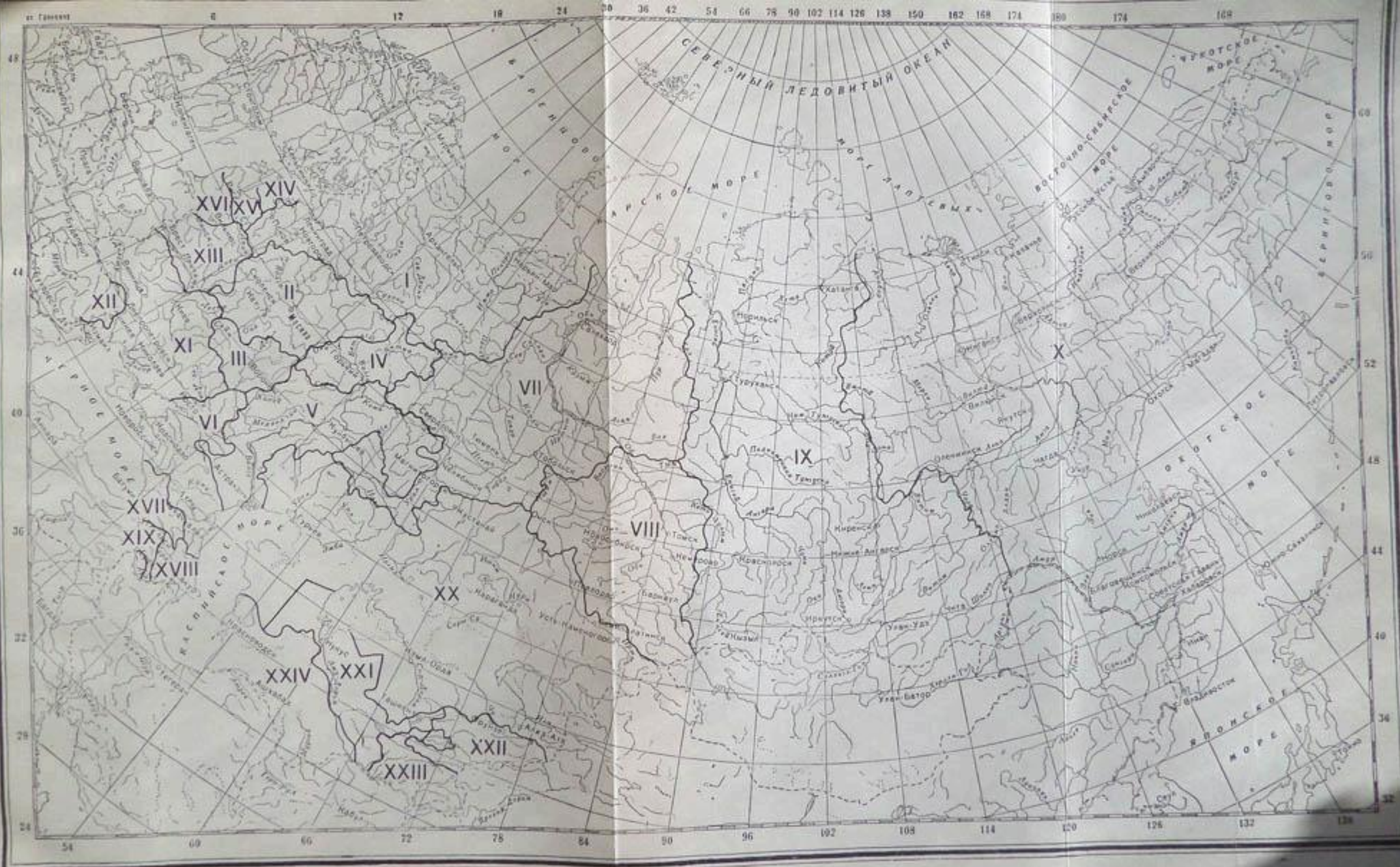
Рис. 4. Схема районов, принятая для расчетов водных ресурсов и водного баланса на территории СССР.
