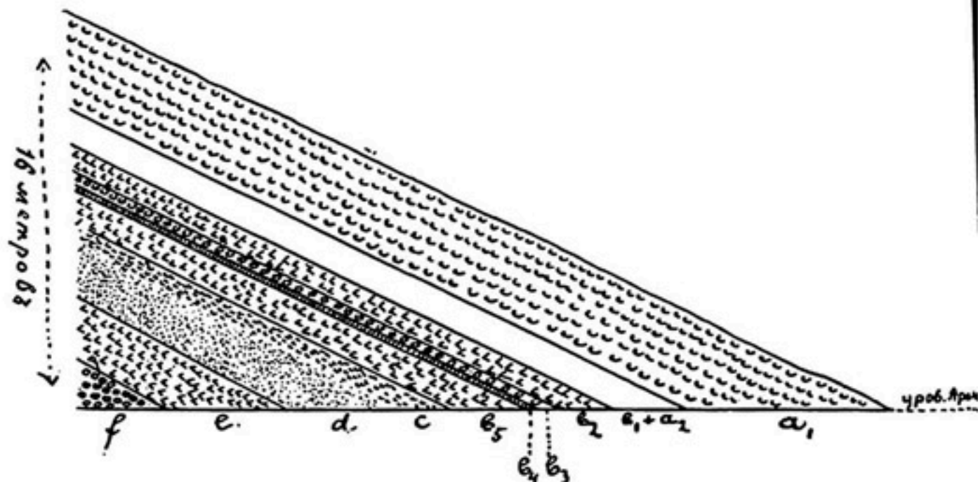
Обнаженіе въ 1½ в. къ западу отъ мыса Икенды на пол. Куланды (ср. фотографіи на стр. 465—466).
