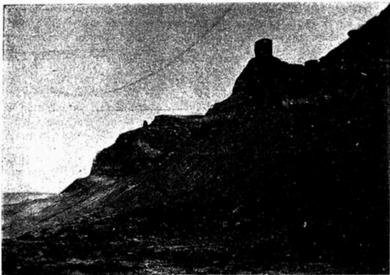
Работа выдуванія на берегу полуострова Каратюнь. Слѣва на заднемъ планѣ—море.
