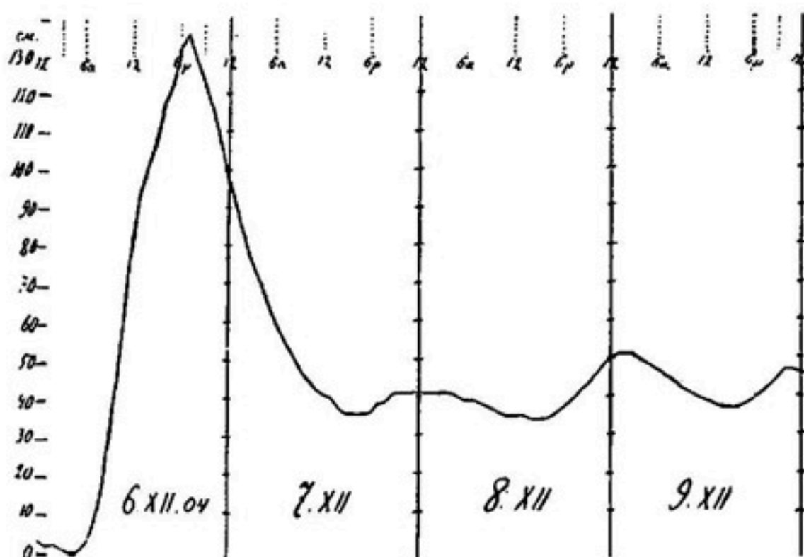
Денивелляція 6 декабря 1904 г. у ст. „Аральское море“, перешедшая на слѣдующіе дни въ сейши. Вертикальный масштаб 1:20.
