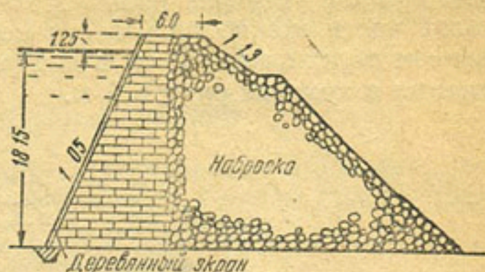
Рис. 24. Профиль плотины Беломорско-Балтийского канала. Экран деревянный
