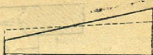
Рис. 44. Распределение нормальных напряжений при отсутствии хвостового утолщения и при его наличии
