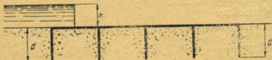
Рис. 139. Многошпунтовый контур
