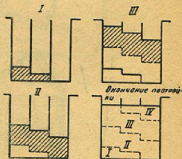
Рис. 194. Способ возведения плотины методом гребенки
