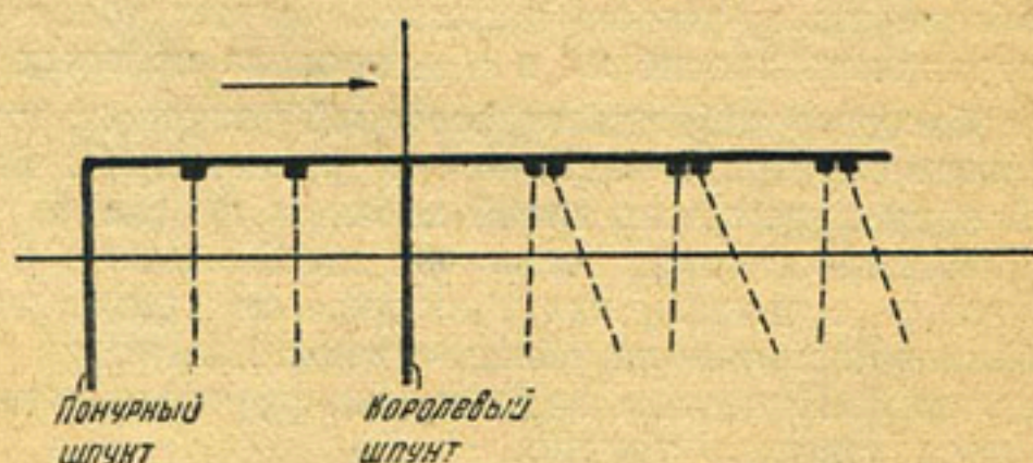
Рис. 181. Флютбет с козловыми сваями
