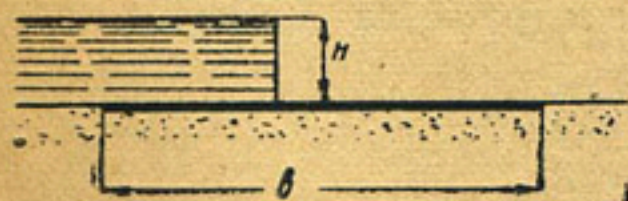
Рис. 132. Бесшпунтовый фильтрационный контур (№ 1)
