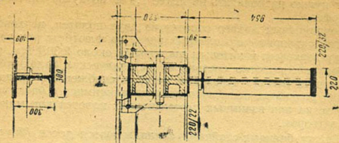
Рис. 184. Опорные части затвора
