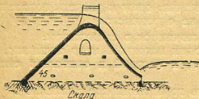
Рис. 92. Полый железобетонный водослив на скале (профиль)
