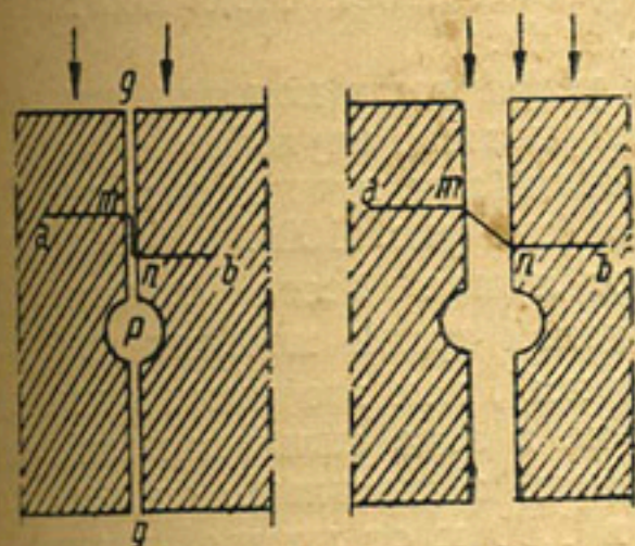
Рис. 99. Простейшее уплотнение
