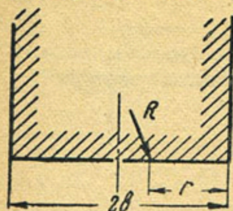
Рис. 116. Уменьшение расчетной ширины фундамента по Герсеванову
