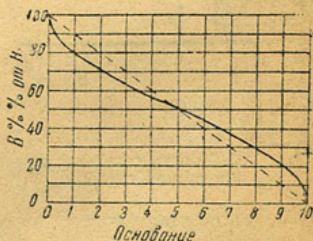
Рис. 141. Эшюра фильтрационного давления для бесшпунтового контура № 1
