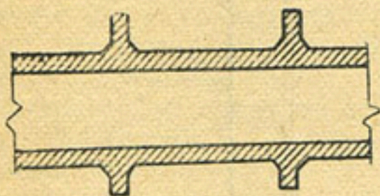
Рис. 61. Труба водоспуска
