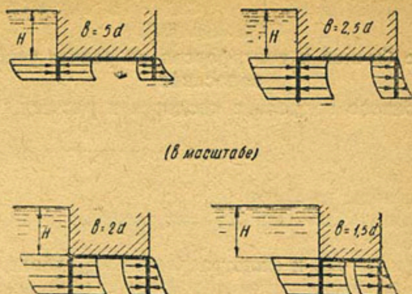
Рис. 158. Статические условия работы шпунтовых рядов в двухшпунтовом контуре при различном соотношении ширины флютбета и глубины шпунта
