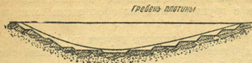
Рис. 5. Сопряжение земляной плотины с основанием и с берегами
