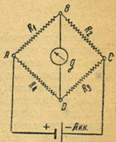
Рис. 131. Метод ЭГДА
