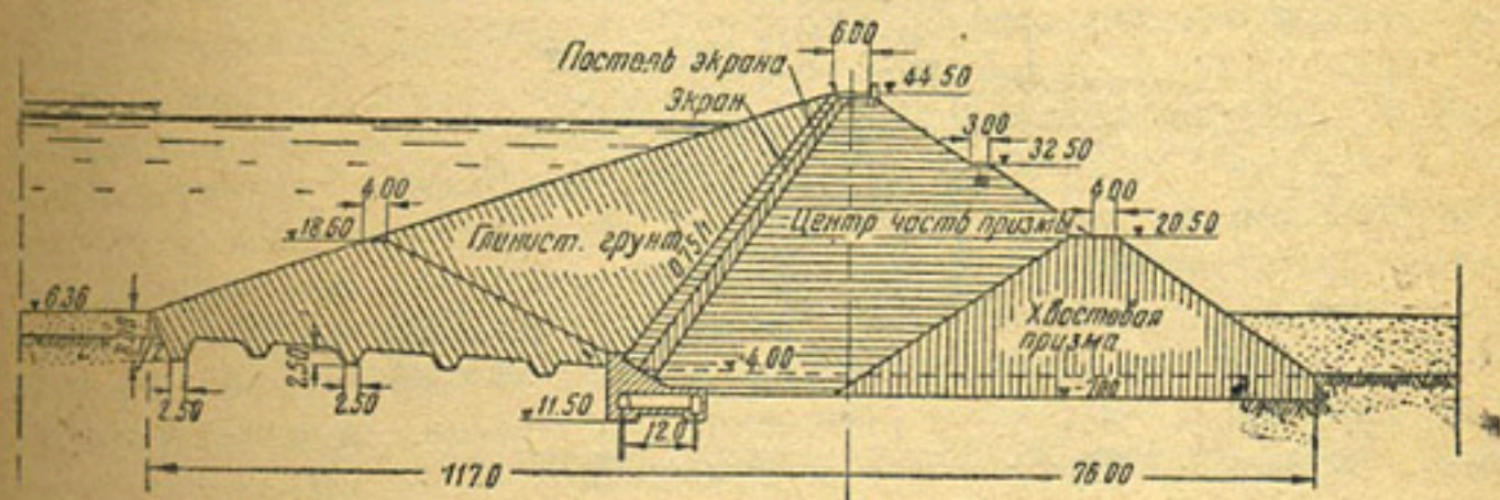
Рис. 25 Профиль плотины Гайо
