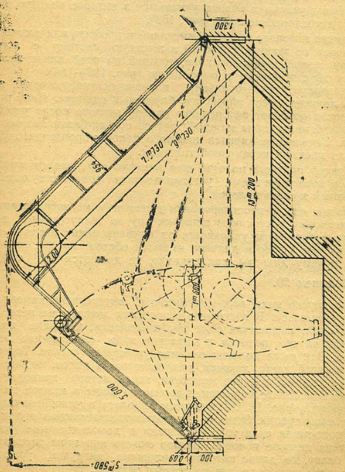
Ғис, 183. Затлор дахвер
