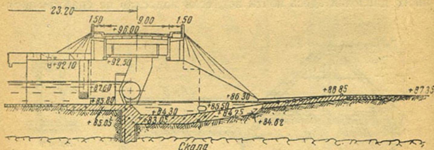
Рис. 113. Плотина с упором верхового зуба в скалу
