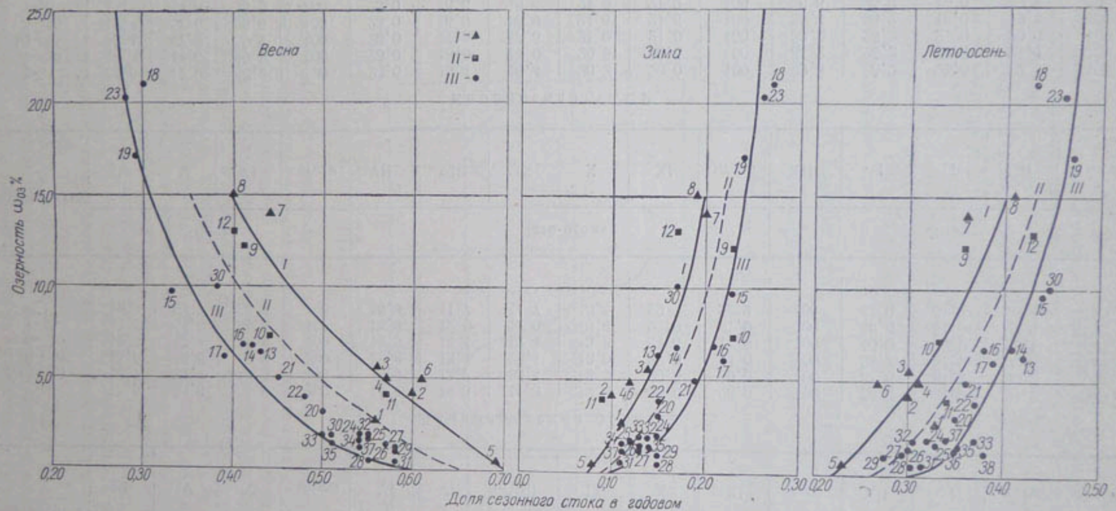
Рис. 9. Зависимость средней величины сезонного стока (в долях от годового) от озерности водосбора [номера точек по табл. 7 в работе (В. Г. Андреев, 1957а)]. 1 — реки Кольского полуострова, 2 — реки Северной Карелии 3 — прочие озерные реки Северо-запада Европейской территории Союза ССР.
