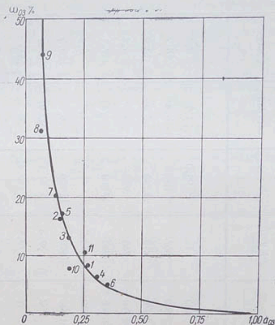
Рис. 7. Зависимость коэффициента уменьшения средней годовой амплитуды уровня озера a_{03} от озерности водосбора \omega_{03} (номера точек по табл. 17).
