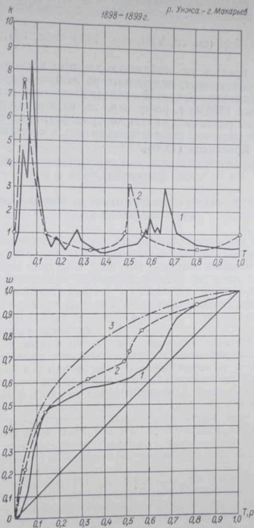
Рис. 44. Гидрографы и интегральные кривые стока по р. Унже у г. Макарьева за 1898/99 г.
