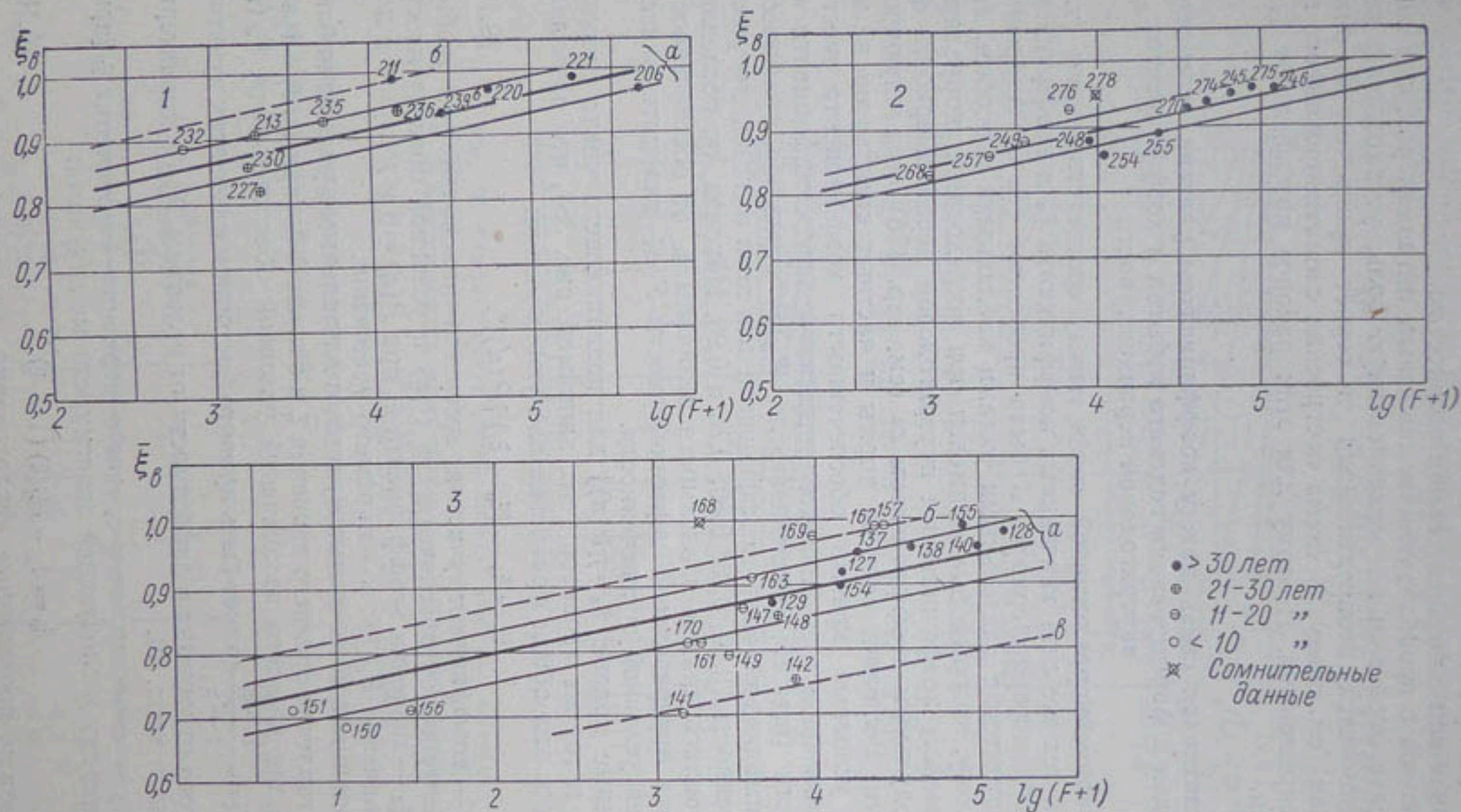
Рис. 37. Районные графики зависимости среднемноголетних значений коэффициента участия весеннего половодья в годовом избытке \bar{\xi}_в от величины площади водосбора F .
