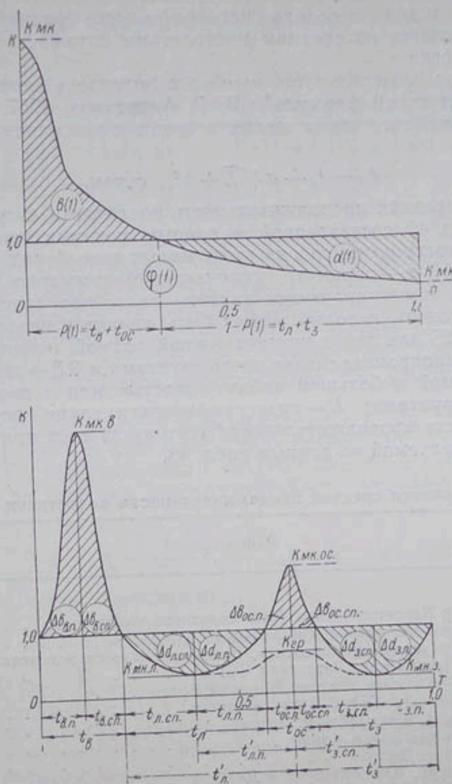
Рис. 41. Схема построения расчетного гидрографа при заданной внутригодовой неравномерности стока d .
