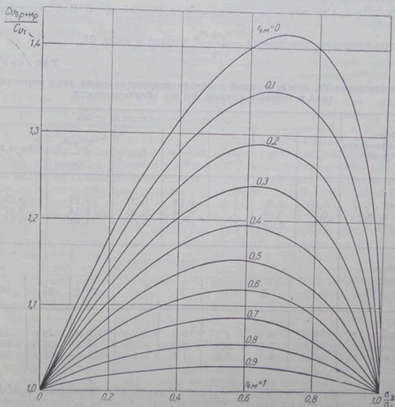
Рис. 19. График зависимости отношения коэффициентов вариации суммы равнообеспеченных величин стока весны и межени C_{v_{Bp+Mp}} и годового стока C_{v_{\Gamma}} от отношения среднеквадратических отклонений стока весны \sigma_B и года \sigma_{\Gamma} и от коэффициента корреляции r_{BM} .
