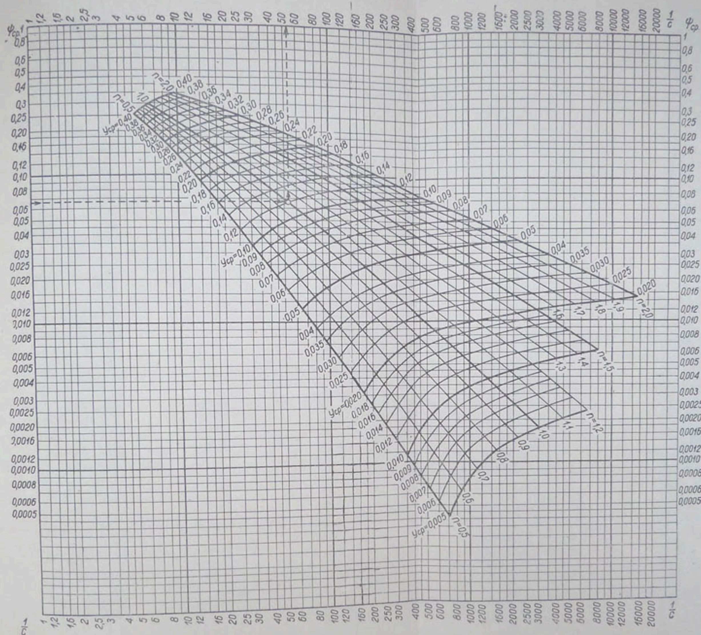
Рис. 47. Номограмма для определения параметров \frac{1}{c} и n уравнения кривых продолжительности расходов по заданным величинам Q_{ср} и \psi_{ср} .
