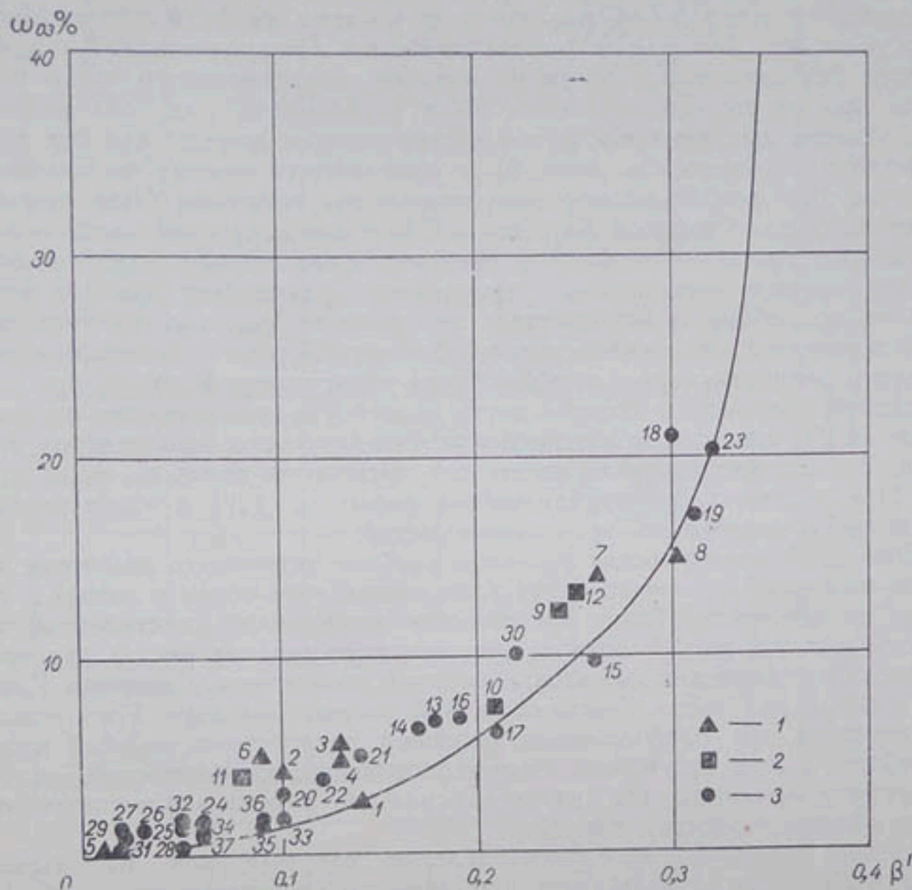
Рис. 8. Зависимость относительной величины средней регулирующей емкости озер на водосборе \beta' от озерности \omega_{03}
