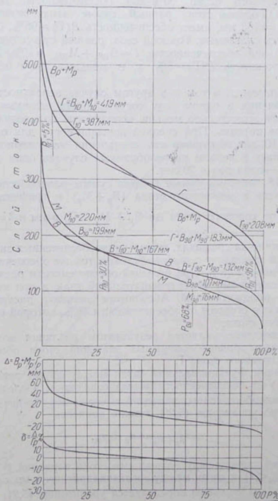
Рис. 18. Кривые обеспеченности годового ( \Gamma ), весеннего ( V ) и межениго ( M ) стока; графики суммы равнообеспеченных значений весеннего и межениго стока ( B_p + M_p ) и ее отклонений от годового стока той же обеспеченности: \Delta = B_p + M_p - \Gamma_p и \delta = \frac{\Delta}{\Gamma_p} \% (р. Тихвинка у д. Горелухи).
