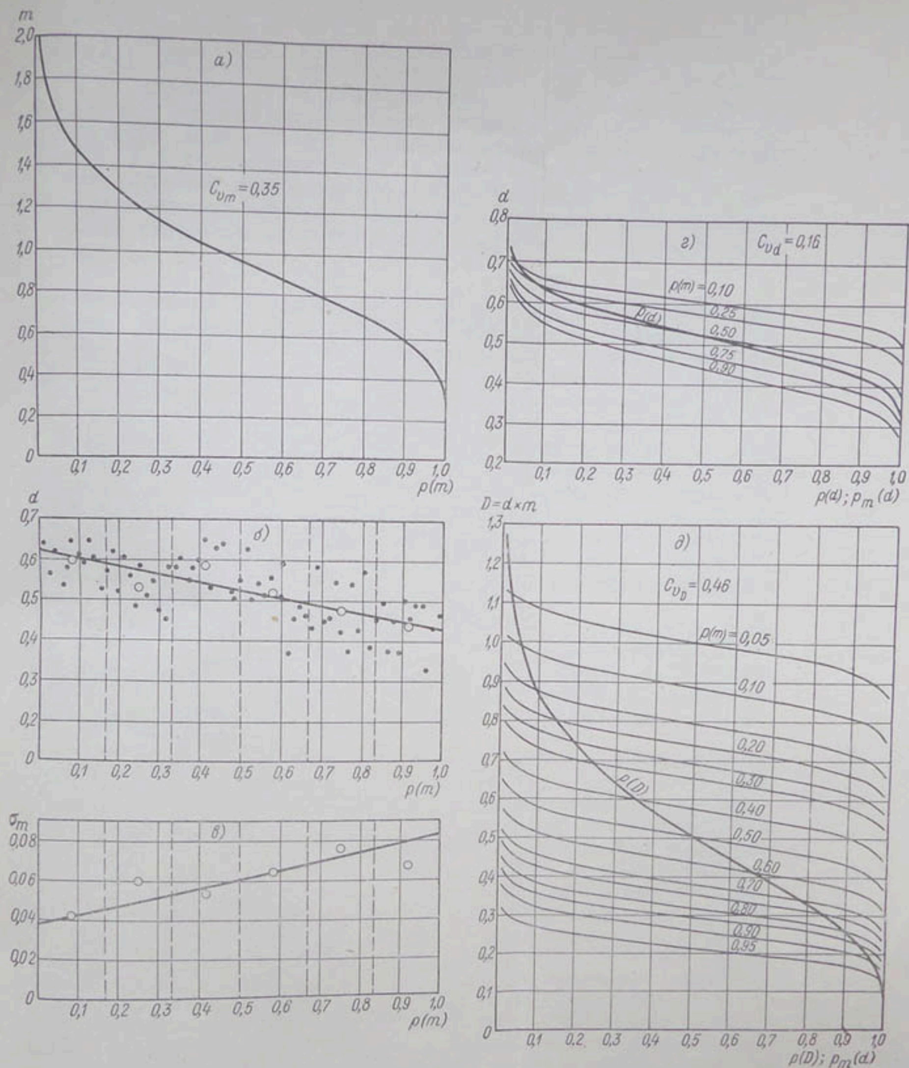
Рис. 30. Характеристика внутригодовой неравномерности стока в зависимости от водности года на примере р. Дона у г. Калача.
