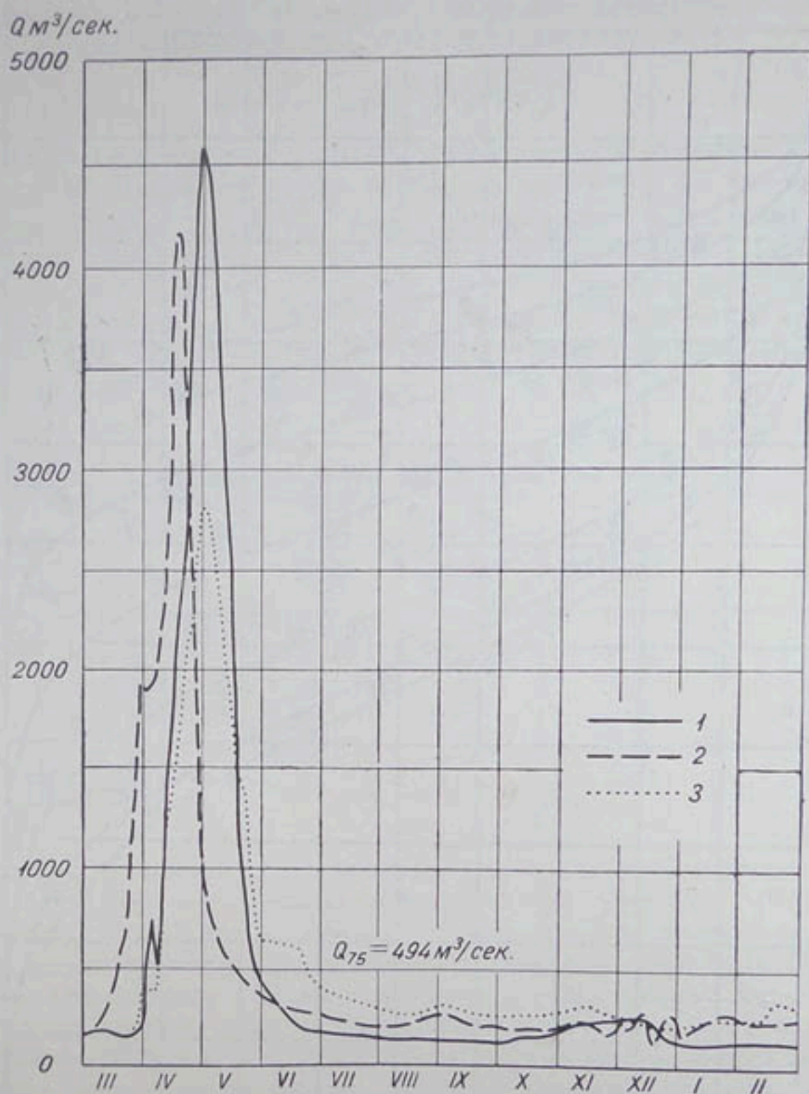
Рис. 40. Гидрографы трех характерных лет р. Дона у г. Калача с обеспеченностью годового стока P(m) \cong 75\% и различной условной обеспеченностью внутригодовой неравномерности.
