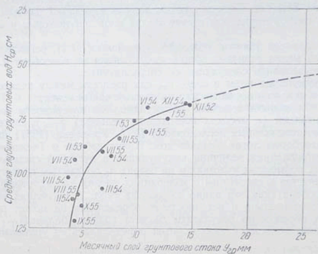
Рис. 3. Зависимость месячного слоя грунтового стока р. Полонети в створе с. Яжелбицы U_{гр} от средней глубины воды в скважинах на логах Усадьевском и Таежном H_{ср}
