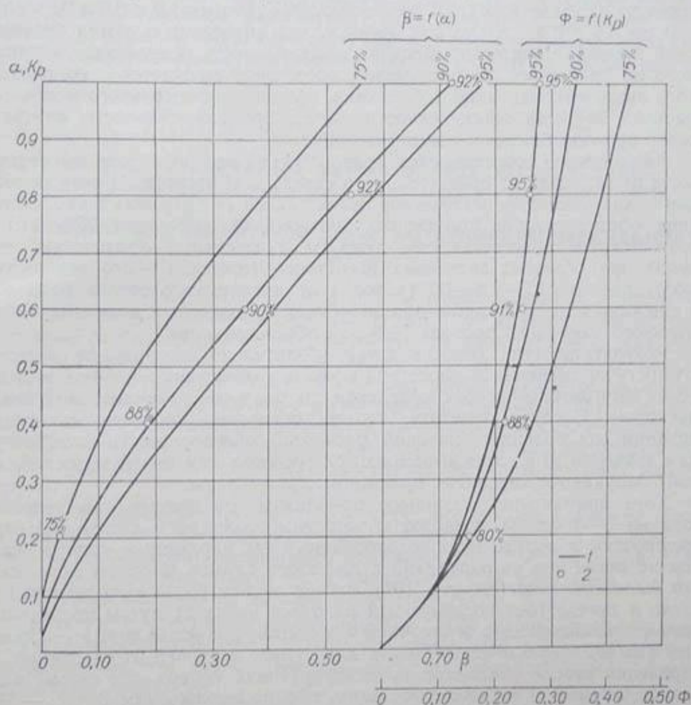
Рис. 22. Кривые зависимости емкости сезонного регулирования \beta от расхода \alpha гарантированной отдачи и полезно используемой годовой отдачи \Phi от расчетного расхода K_p по р. Шелони у с. Заполья для 75%-ной обеспеченности.
