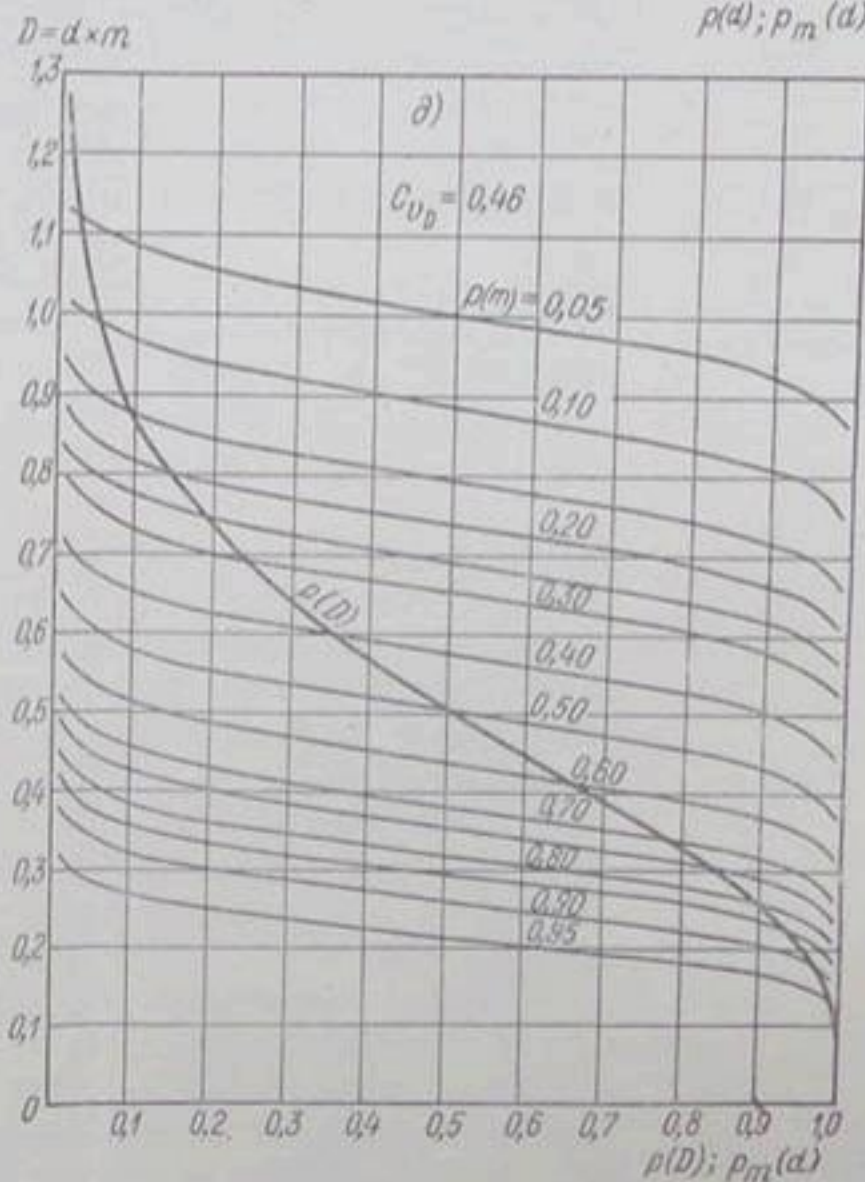
Рис. 30. Характеристика внутригодовой неравномерности стока в зависимости от водности года на примере р. Дона у г. Калача.
