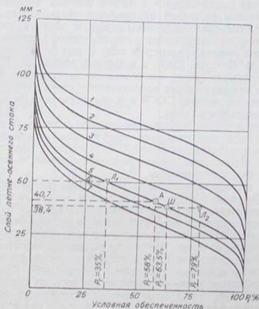
Рис. 20. Условные кривые обеспеченности летне-осеннего стока при фиксированном годовом стоке по р. Сож у г. Славгорода с показанием результатов расчета межсезонного распределения стока для заданной обеспеченности 75% по разным методам
