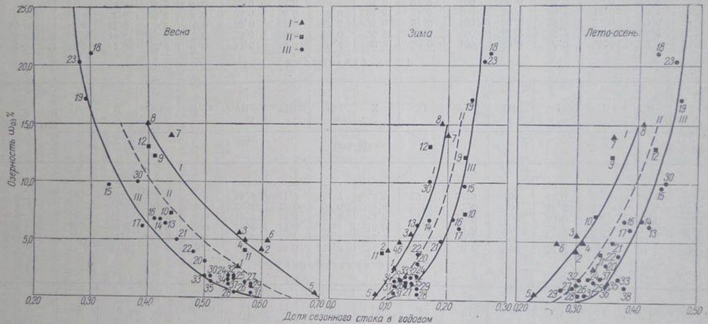
Рис. 9. Зависимость средней величины сезонного стока (в долях от годового) от озерности водосбора [номера точек по табл. 7 в работе (В. Г. Андреянов, 1957а)]. 1 — реки Кольского полуострова, 2 — реки Северной Карелии 3 — прочие озерные реки Северо-запада Европейской территории Союза ССР.
