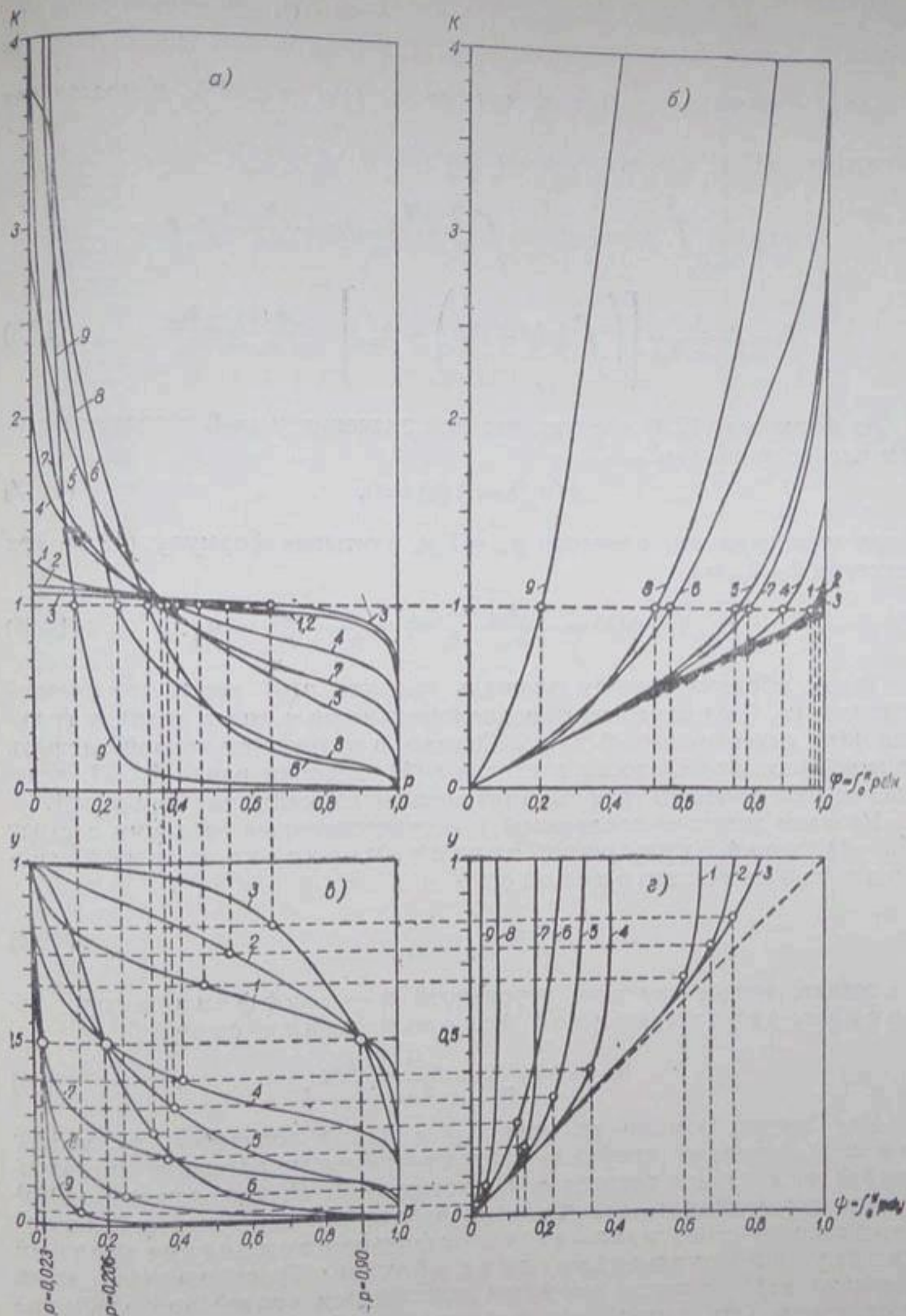
Рис. 46. Графики кривой продолжительности расходов и кривой использования стока при разных значениях параметров c и n . а — кривые продолжительности расходов p(k) ; б — кривые использования стока \varphi(k) ; в — приведенные кривые продолжительности расходов p(y) ; г — приведенные кривые использования стока \varphi(y) . Параметры кривых см. в табл. 49.
