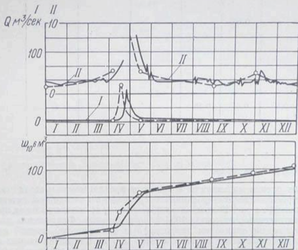
Рис. 43. Гидрограф и календарная интегральная кривая стока для 1934 года по р. Боровке у х. Паника.
