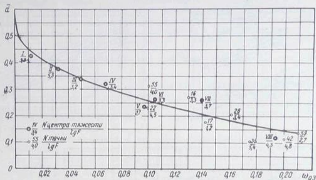
Рис. 27. График зависимости среднегодовых значений коэффициента внутригодовой неравномерности \bar{d} от озерности водосбора \omega_{03} .
