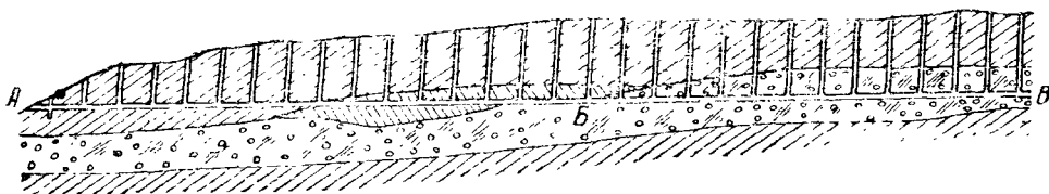
Рис. 75. Кяриз
