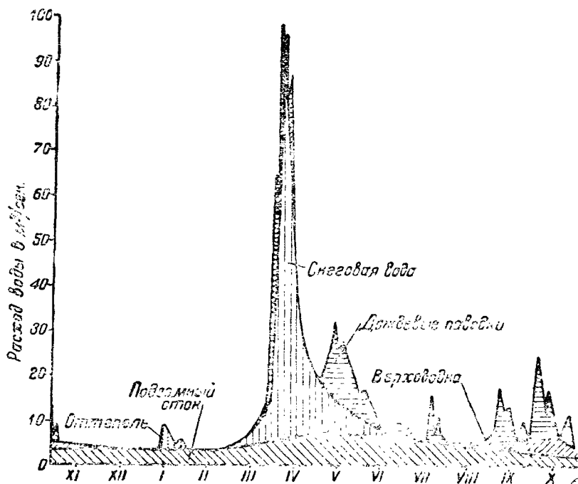
Рис. 7. Годовой гидрограф р. Ижоры (по В. С. Советову)
