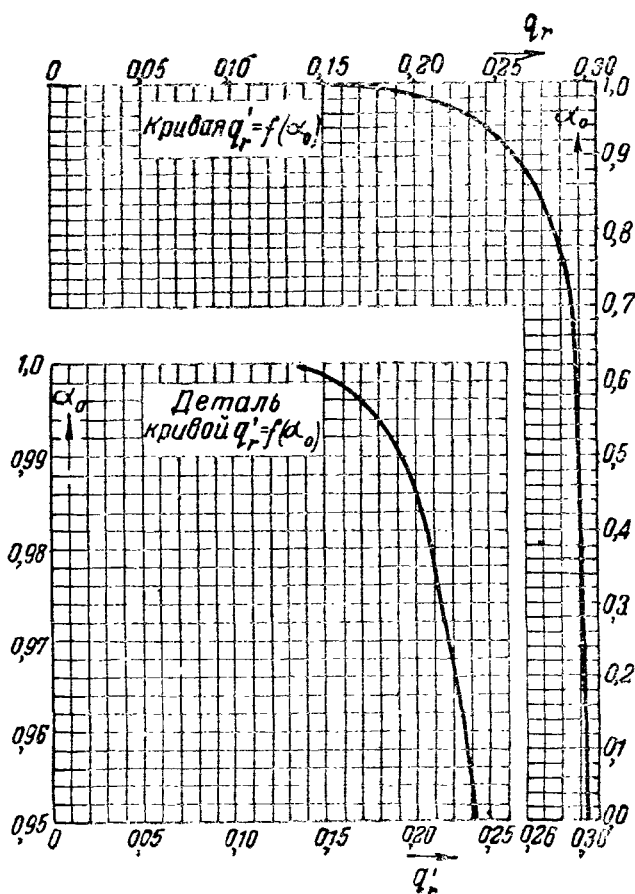
Рис. 83. График для нахождения величины q_r'
