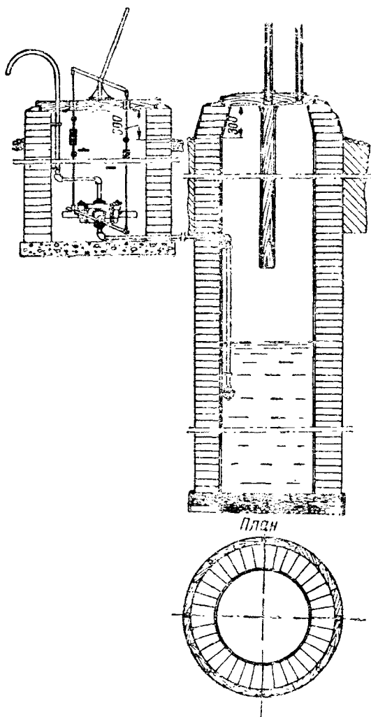
Рис. 55. Кирпичный колодец
