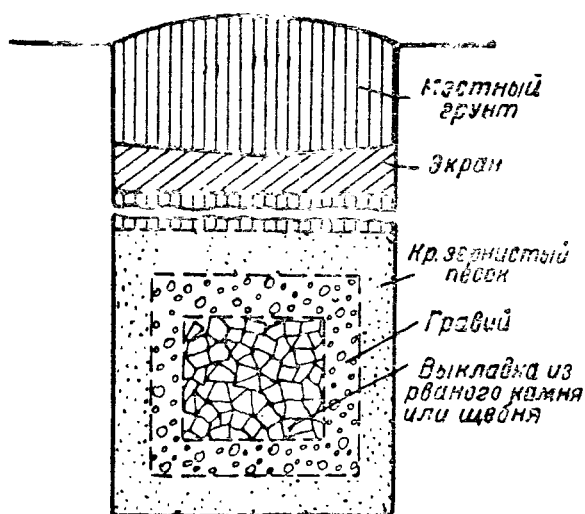
Рис. 69. Каменно-щебеночный водозабор
