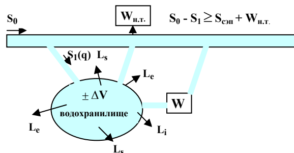
Рис. 1. Расчетная схема имитационной модели
