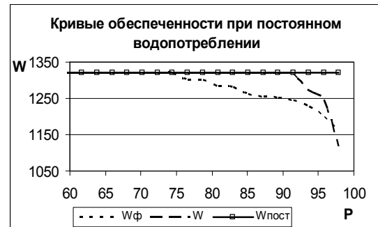
Рис. 11. График кривых до и после диспетчерского графика
