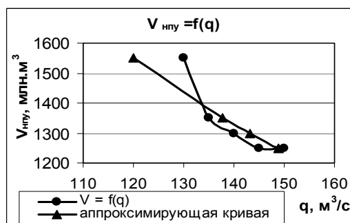
Рис.8. График зависимости емкости водохранилища от пропускной способности тракта при P_{\text{пр}} = 86\%
