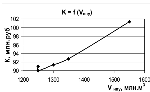
Рис. 9. Графики зависимости капитальных вложений от емкости водохранилища, если подводящий тракт канал и трубопровод соответственно
