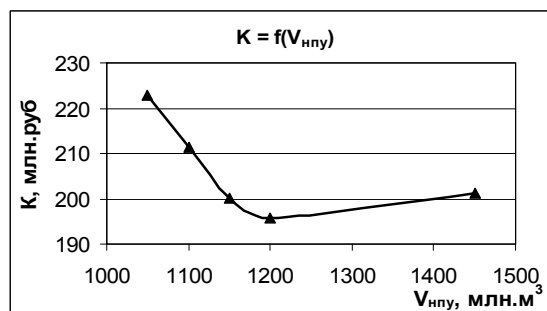
Рис. 9. Графики зависимости капитальных вложений от емкости водохранилища, если подводящий тракт канал и трубопровод соответственно
