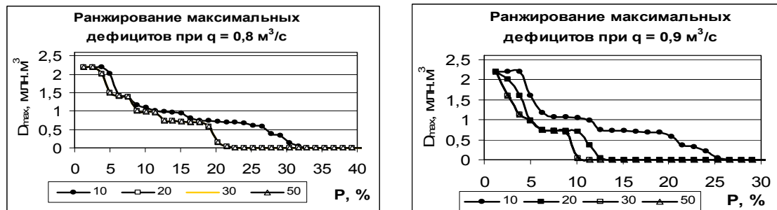
Рис. 14. Графики, показывающие кривые максимальных дефицитов при q = 0,8 и 0,9 \text{ м}^3/\text{с} .
