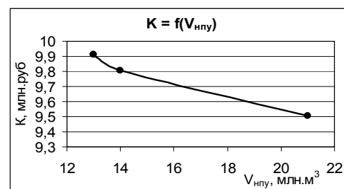
Рис. 16. График зависимости капитальных вложений от емкости
