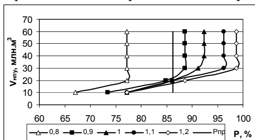
Рис. 15. График изменений емкости водохранилища в зависимости от обеспеченности потребителей водой
