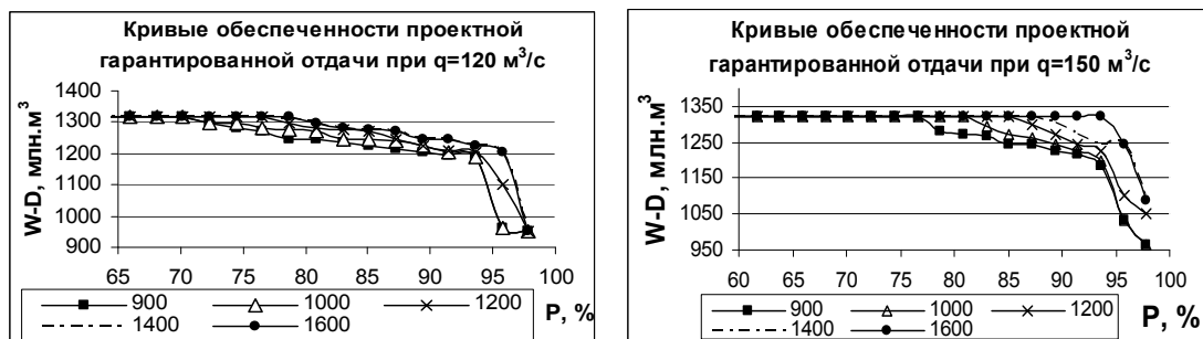
Рис. 5. Кривые обеспеченности проектной гарантированной отдачи при пропускной способности тракта q = 120 и 150 м³/с.
