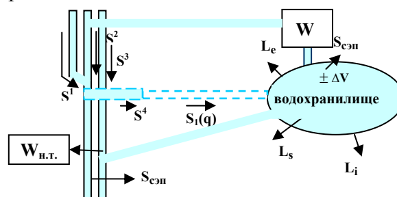
Рис. 12. Расчетная схема для наливного водохранилища Полиатис
