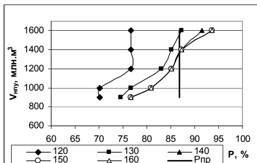
Рис. 7. График изменений емкости водохранилища в зависимости от обеспеченности потребителей водой
