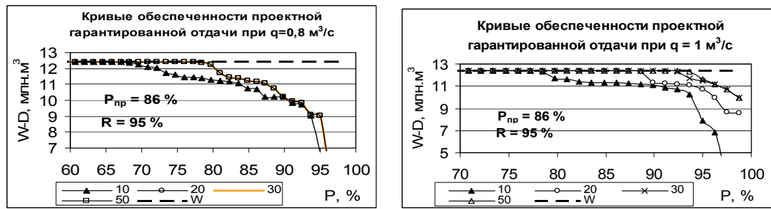
Рис. 13. Кривые обеспеченности проектной гарантированной отдачи при пропускной способности тракта q = 0,8 и 1,0 \text{ м}^3/\text{с} .
