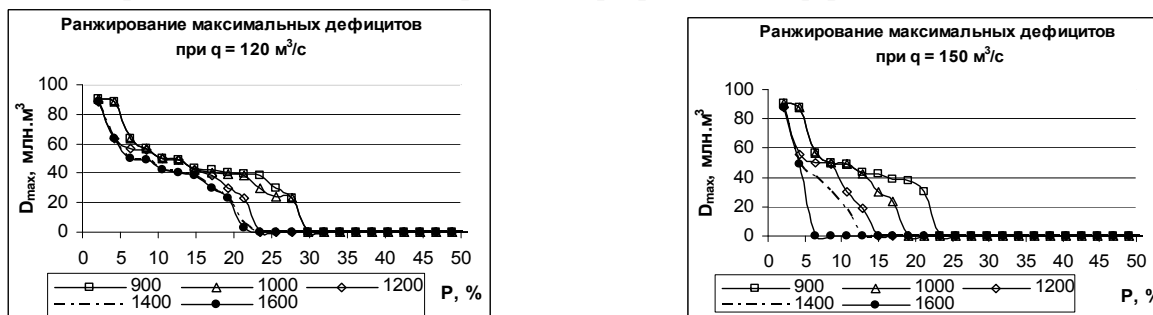
Рис. 6. Графики, показывающие кривые максимальных дефицитов при q = 120 и 150 м³/с.
