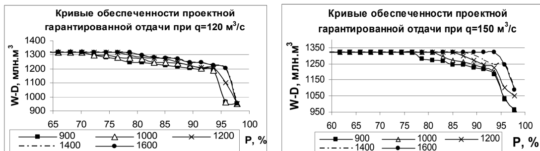
Рис. 5. Кривые обеспеченности проектной гарантированной отдачи при пропускной способности тракта q = 120 и 150 м 3 /с.
