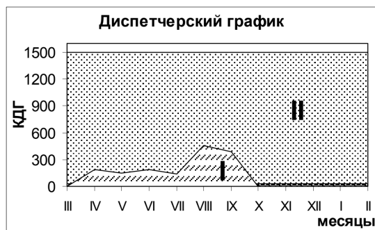
Рис. 10. Диспетчерский график для обеспечения наливного водохранилища на реке Самур:
