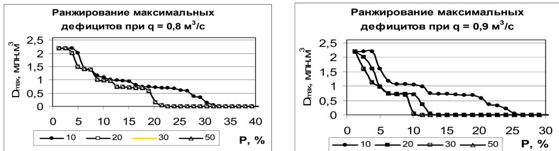
Рис. 14. Графики, показывающие кривые максимальных дефицитов при q = 0,8 и 0,9 м³/с.
