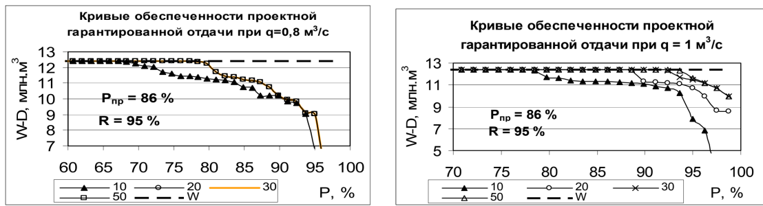
Рис. 13. Кривые обеспеченности проектной гарантированной отдачи при пропускной способности тракта q = 0,8 и 1,0 м³/с.
