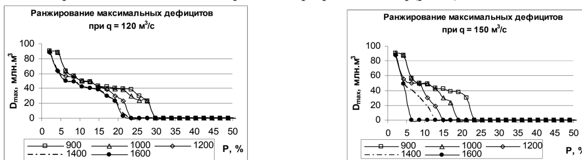
Рис. 6. Графики, показывающие кривые максимальных дефицитов при q = 120 и 150 м 3 /с.
