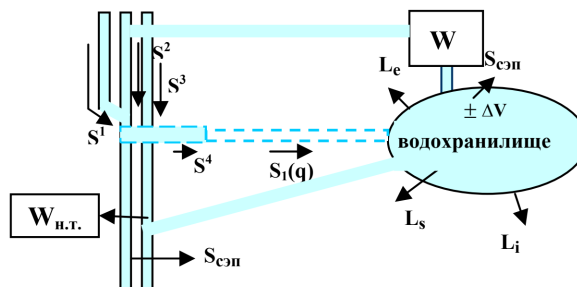
Рис. 12. Расчетная схема для наливного водохранилища Полиатис
