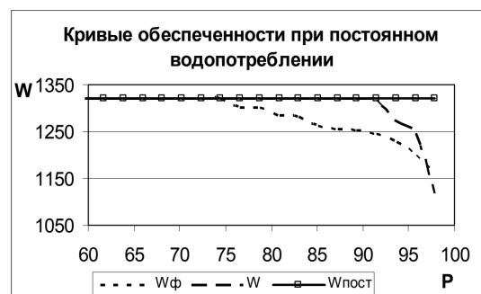
Рис. 11. График кривых до и после диспетчерского графика
