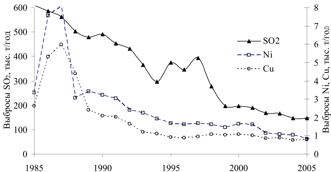
Рисунок 6. Снижение выбросов диоксида серы, никеля и меди комбинатами концерна «Никель» на Кольском Севере.
