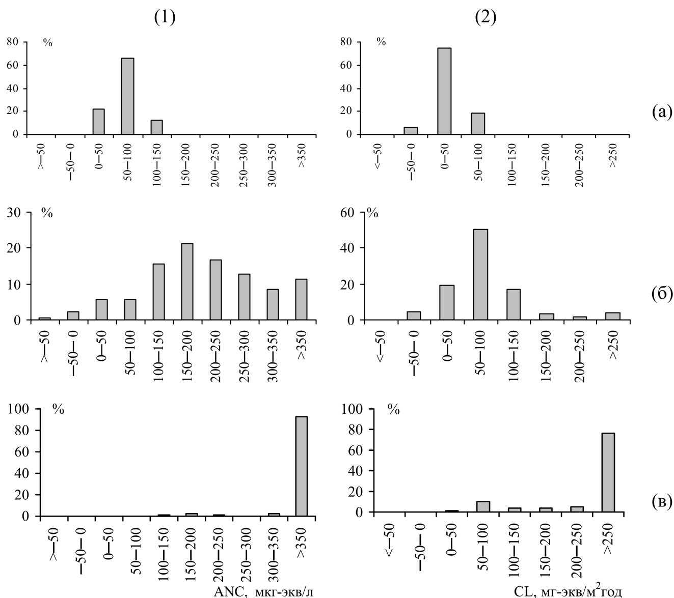
Рис. 3. Распределение озер (%) в природно-климатических зонах (а – тундра и лесотундра, б – северная и средняя тайга, в – смешанные и широколиственные леса) по значениям кислотонейтрализующей способности вод (1 – ANC, мкг-экв/л) и значениям критических нагрузок (2 – CL, мг-экв/м 2 год) выпадений кислотообразующих веществ.
