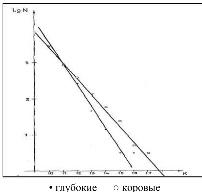
Рис. 2.2 – Поверхностные и глубокие землетрясения на Памире в 1895-1991 гг. [12]
