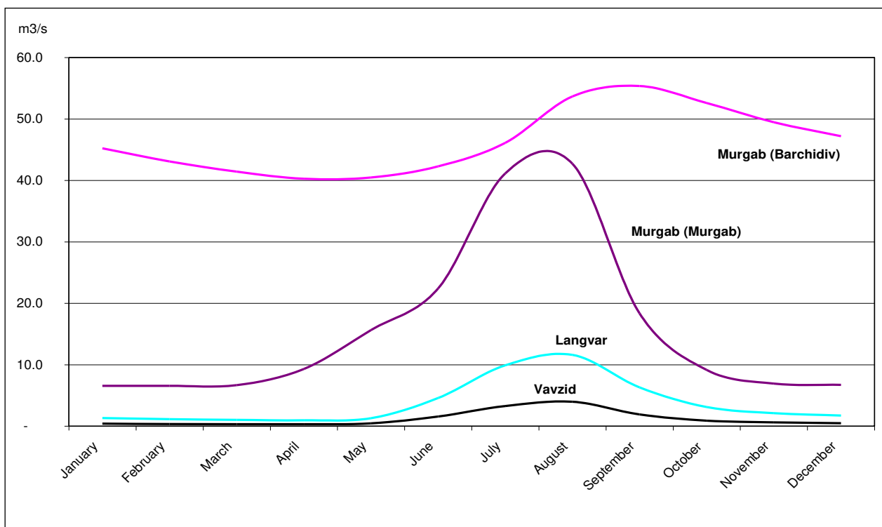
Рис. 1.8 – Среднемесячный расход рек Вавзид, Лангвар и Мургаб (м³/сек)
