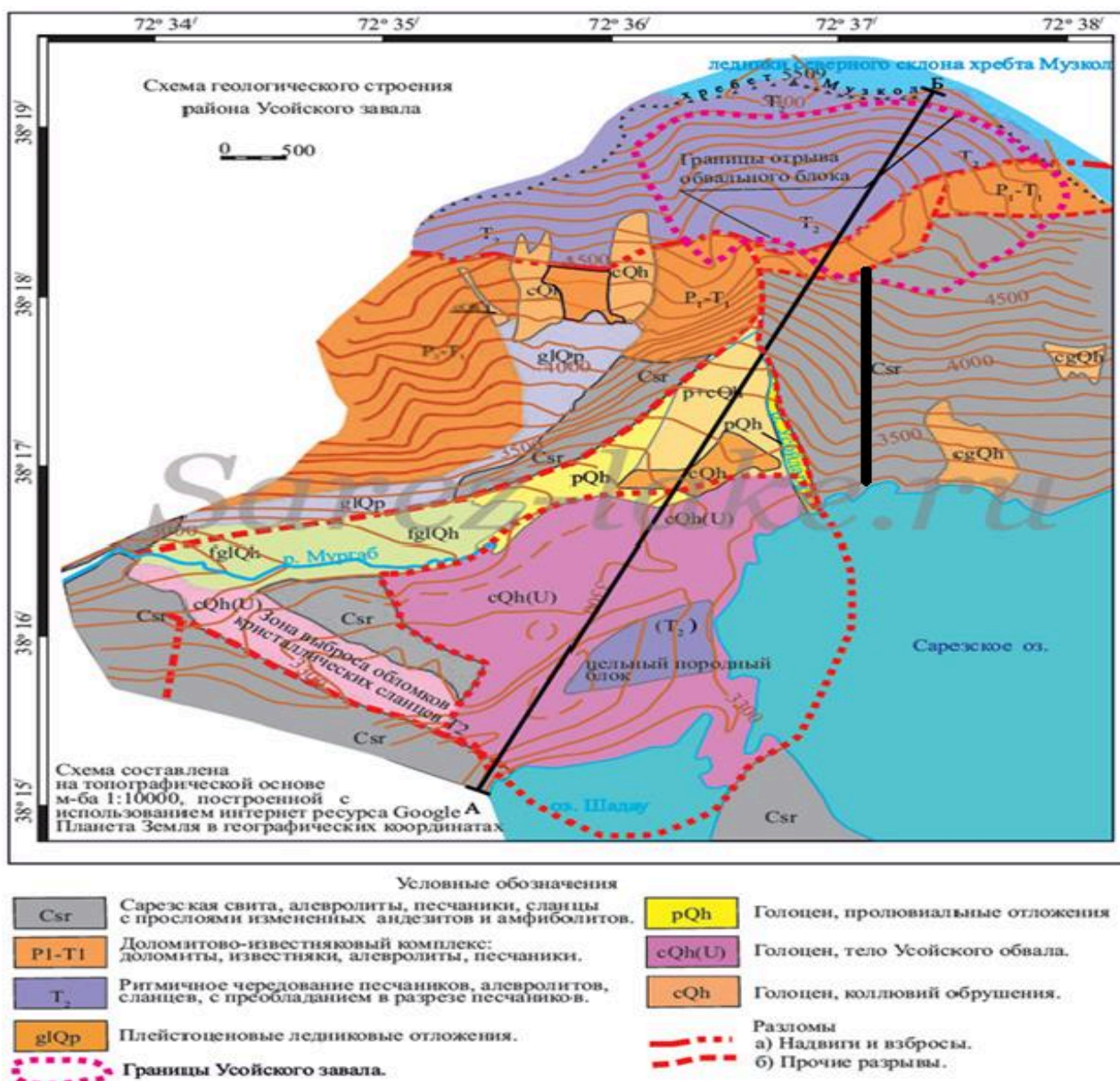
Рис. 4.3 – Схема геологического строения района Усойского завала
