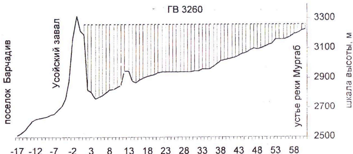
Рис. 1.5 – Продольный профиль реки Бартанг в районе Сарезского озера [11]
