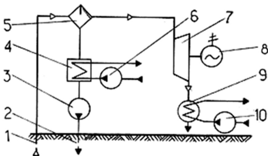
Рисунок 2.8. Тепловая схема одноконтурной ГеоТЭС
