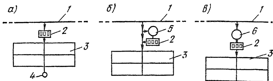
Рис. VIII.2. Схема подключения внутризаводской водопроводной сети к городскому водопроводу
