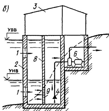
Рис. VI.2. Схемы водозаборных сооружений берегового типа
