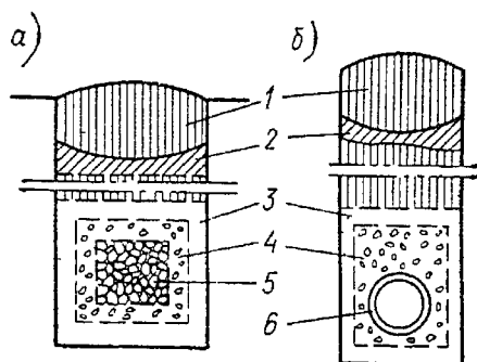
Рис VII 20 Траншейные водозаборы
