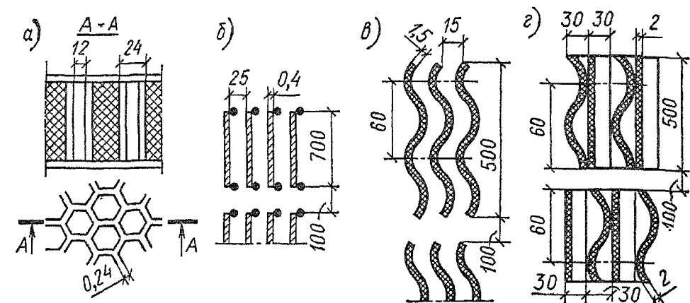
Рис. VIII.17. Пленочные оросители из пластмасс
