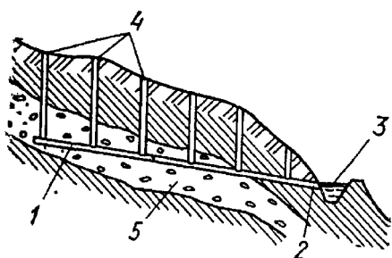
Рис. VII 19 Схема кяриза
