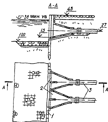
Рис. VI 11. Затапливаемый водо- приемник
