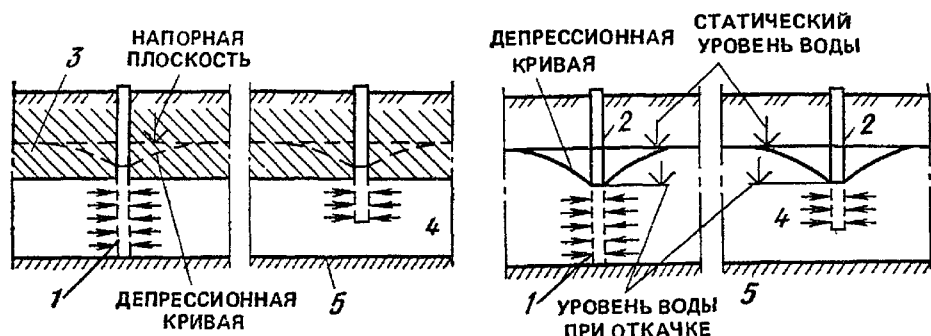
Рис. VII.12. Типы скважин
