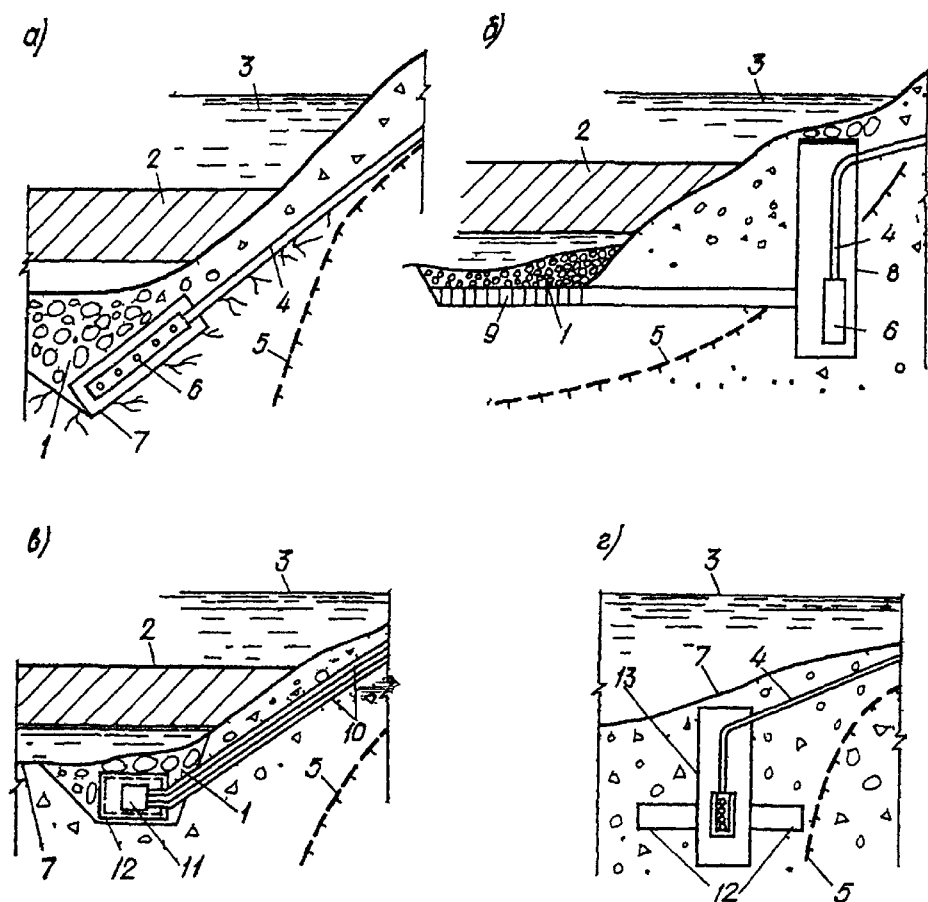
Рис VI 28 Водозаборные сооружения, оборудованные погружными насосами на реках с большим колебанием уровня воды
