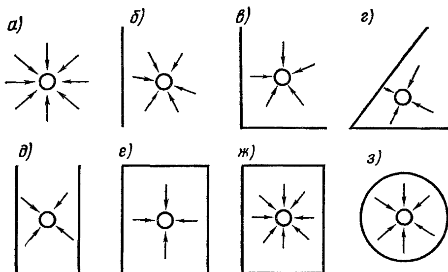
Рис. VII.14. Расчетные схемы водоносных пластов (план)
