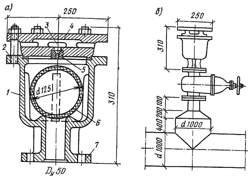
Рис. IV.13. Общий вид вантуза эксплуатационного D_y=50 мм (а) и схема установки его на водоводе D_y=1000 мм (б)
