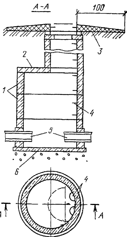
Рис. IV 22. Водопроводный колодец
