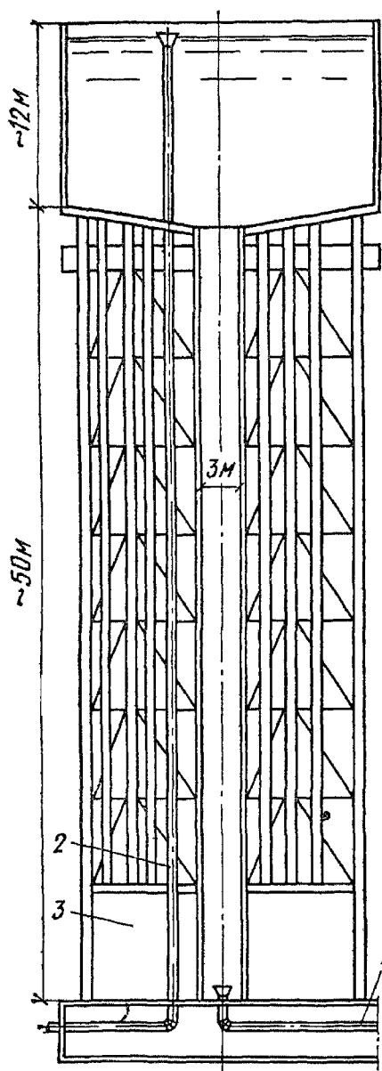
Рис. V.2. Схема водонапорной башни вместимостью 3600 м 3
