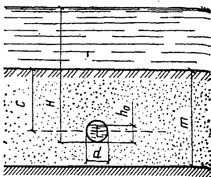
Рис. VII.24. Схема к расчету подруслового водозабора
