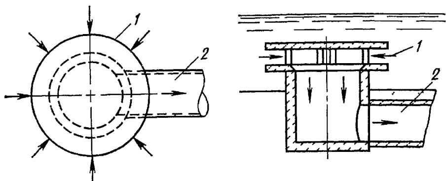
Рис VI 30 Морской затопленный водоприемник с круговым приемом воды
