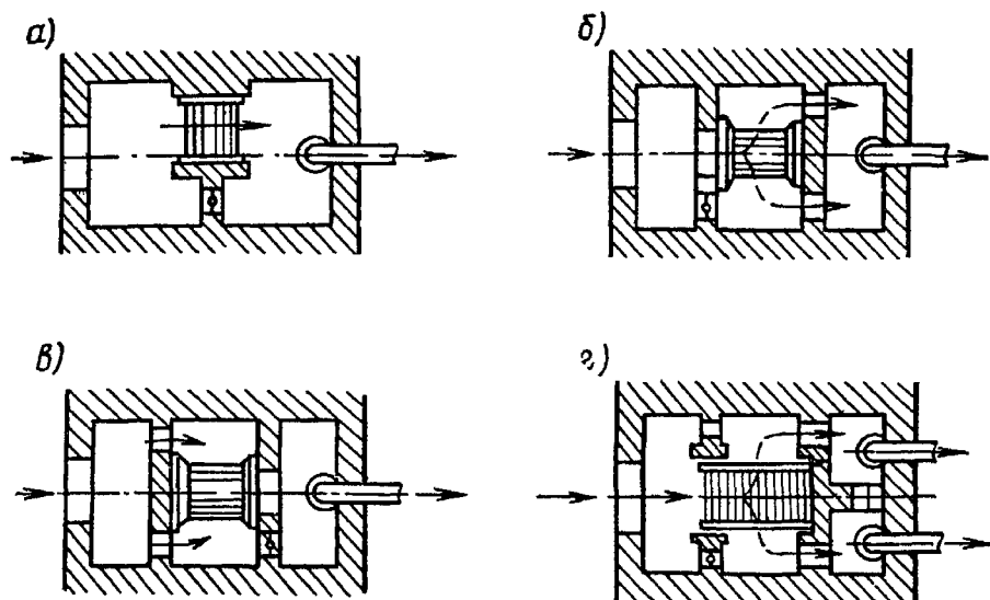
Рис. VI.21. Схемы подвода воды к вращающимся сеткам
