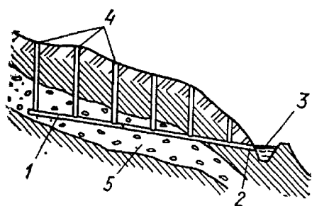
Рис. VII 19 Схема кяриза
