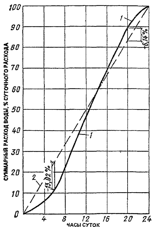
Рис II.9 Совмещенный график работы насосной станции I и II подъема
