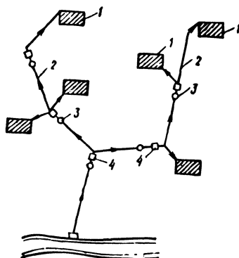
Рис. 2.2. Схема групповой (районной) системы водоснабжения: 1 — предприятие, поселок и т. п.; 2 — водовод; 3 — резервуар; 4 — насосная станция
