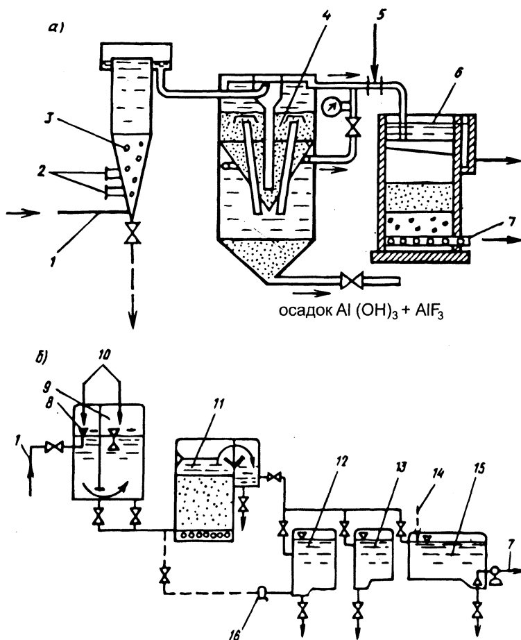
Рис. 5.32. Схема дефторирования воды сорбцией на свежееобразованном гидроксиде алюминия (а) и фильтрованием через зернистую загрузку, заряженную сульфат-ионами (б):
