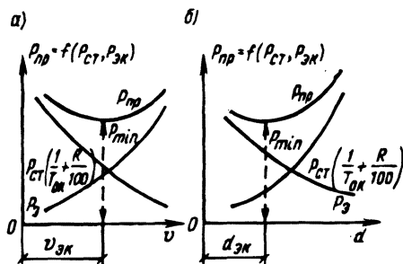
Рис. 3.5. Характер изменения приведенных затрат в функции скорости (а) и диаметра (б)
