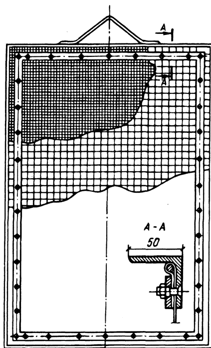
Рис. 4.16. Водоочистная плоская сетка для отверстий размером от 0,4 \times 0,6 до 1 \times 1,25 \text{ м}
