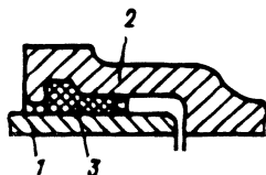
Рис. 3.10. Раструбное соединение чугунных труб на резиновых уплотнителях
