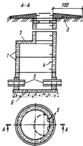
Рис. 3.23. Водопроводный колодец:
