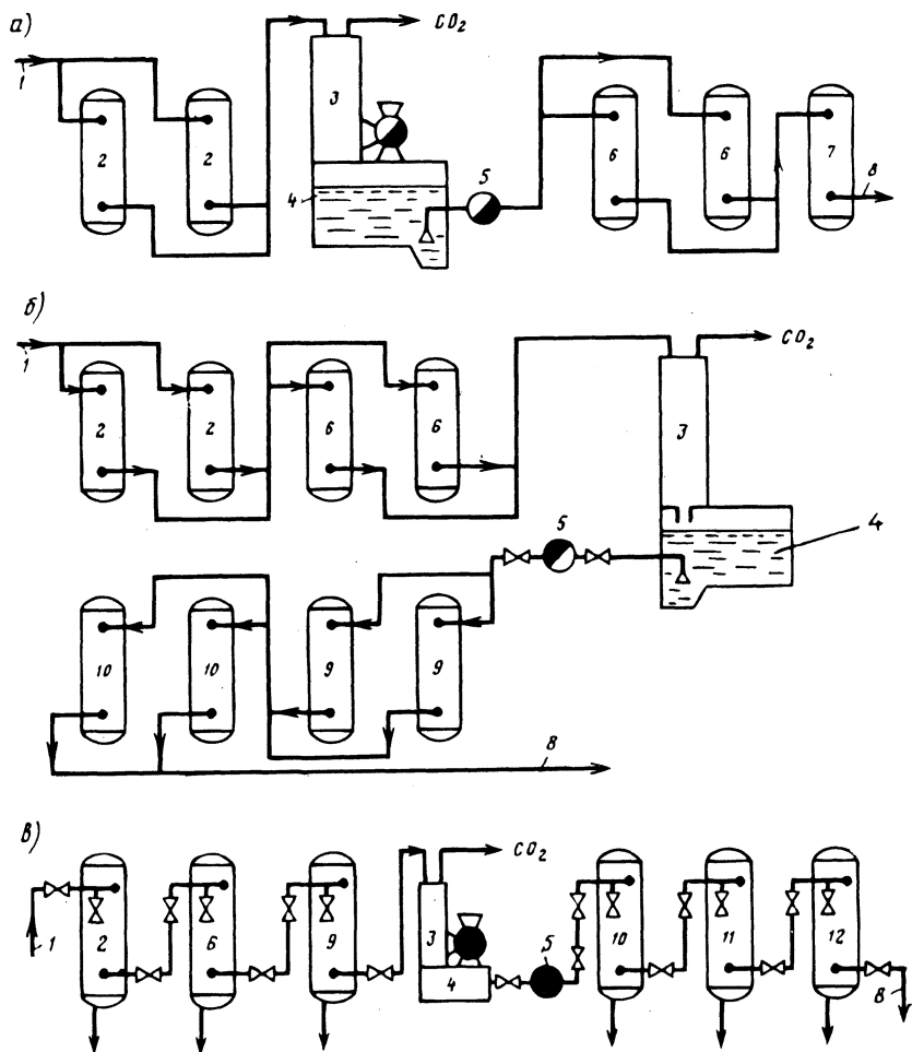
Рис. 5.30. Технологические схемы ионитового обессоливания воды: а — одноступенчатая; б — двухступенчатая; в — трехступенчатая; 1, 8 — подача исходной и отвод обессоленной воды; 2 — водород-катионитовые фильтры; 3 — дегазатор; 4 — промежуточный резервуар; 5 — насос; 6 — анионитовые фильтры; 7 — буферный натрий-катионитовый фильтр; 9 — водород-катионитовые фильтры II ступени; 10 — анионитовые фильтры II ступени (с сильноосновным анионитом); 11 — водород-катионитовые фильтры III ступени; 12 — анионитовые фильтры III ступени
