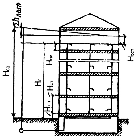
Рис. 2.5. Схема подачи воды в здание
