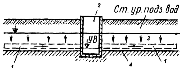
Рис. 4.7. Горизонтальный водозабор:
