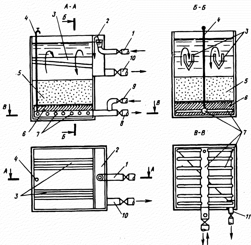
Рис. 5.19. Скорый открытый фильтр:
