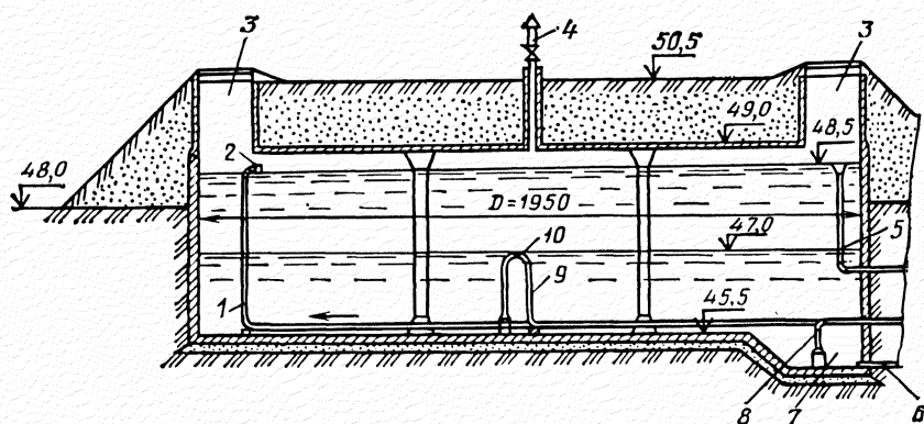
Рис. 2.13. Резервуар чистой воды:
