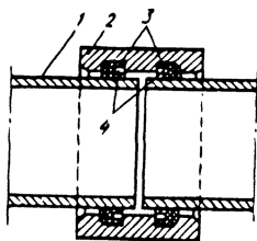
Рис. 3.13. Стык с асбестоцементной муфтой:
