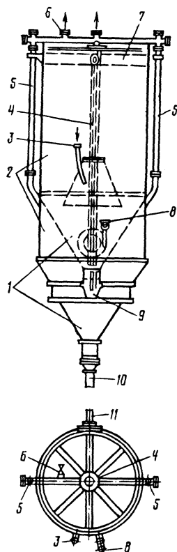
Рис. 5.5. Схема двухкамерного сатуратора «Струя»:
