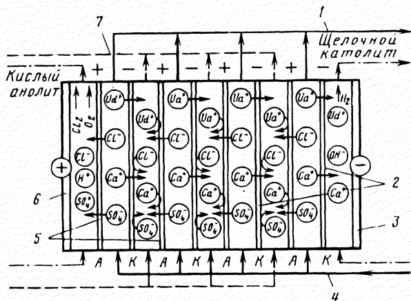
Рис. 5.31. Схема многокамерного электродиализного аппарата: 1, 4 — отвод обессоленной и подача исходной воды; 2, 5 — ионоселективные катионитовые и анионитовые мембраны; 3 — катод; 6 — анод; 7 — отвод концентрата
