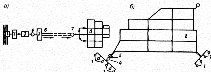
Рис. 2.1. Общая схема систем водоснабжения из поверхностного (а) и подземного (б) источников:
