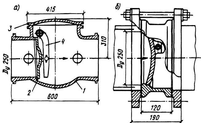
Рис. 3.20. Клапан обратный с нерегулируемым закрытием: а — типа «захлопка»; б — безударный; 1 — корпус; 2 — тарель клапана; 3 — крышка корпуса; 4 — рычаг
