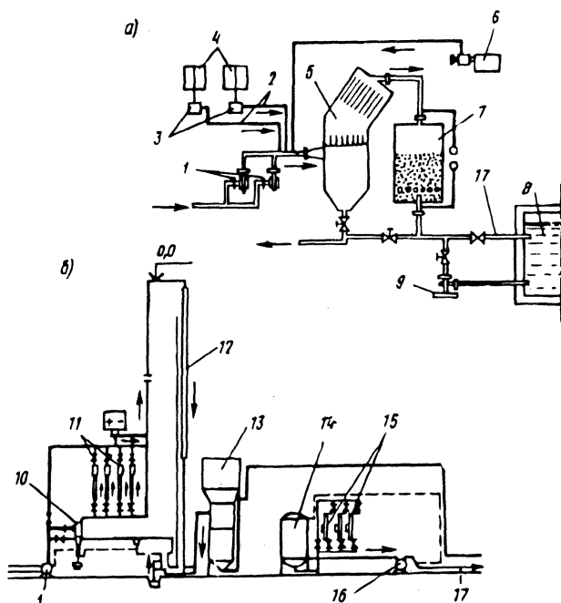
Рис. 5.34. Схема установки АзНИИ ВП «Струя» (а) и ВНИИГиМ (б): 1 — насос I подъема; 2 — подача реагентов; 3 — насос-дозатор; 4 — реагентное хозяйство; 5 — тонкослойный отстойник; 6 — электролизер для обеззараживания воды; 7 — напорный скорый фильтр; 8 — резервуар чистой воды; 9 — промывной насос; 10 — гидроциклон; 11 — электрокоагулятор; 12 — воздухоохладитель; 13 — самопромывающийся скорый фильтр; 14 — пневматический бак; 15 — бактерицидная установка; 16 — электронасос; 17 — отвод обработанной воды
