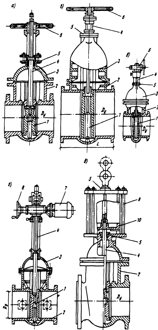
Рис. 3.16. Схемы задвижек:
