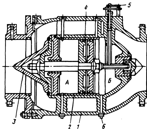
Рис. 3.17. Кольцевая задвижка:
