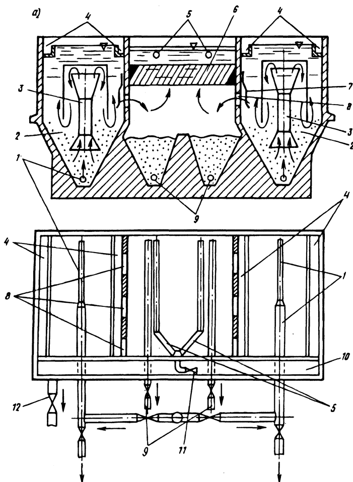
Рис. 5.16. Осветлитель коридорного типа с рециркуляцией осадка и тонкослойными модулями (а), с поддонным (б) и выносным (в) осадкоуплотнителями:
