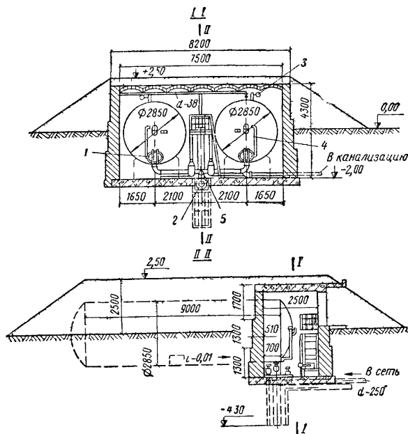
1 — люк (400×300 мм), 2 — подводящая и разводящая труба диаметром 250 мм, 3 — предохранительный клапан на 8 кгс/см 2 , 4 — водомерное стекло, 5 — поплавковый предохранительный клапан
