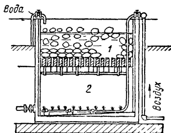
Поперечный разрез
