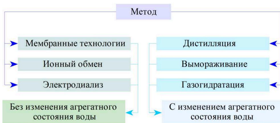
Рисунок 2 – Классификация методов опреснения вод
