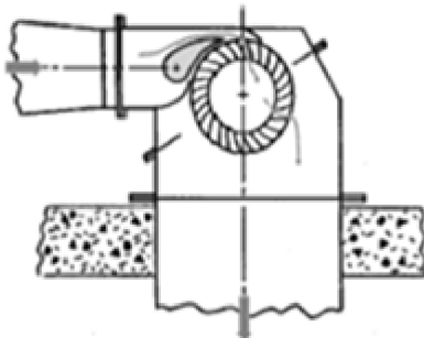
Рис. 2. Поперечно-струйная турбина Банки
