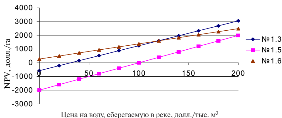
Рис. 1. Цена на воду, сберегаемую в реке, и показатель NPV у водосберегающих мероприятий и технологий в орошаемой зоне 1 Нишанского района (на уровень первых лет XXI в.)
