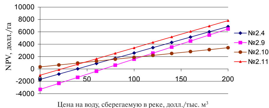
Рис. 2. Цена на воду, сберегаемую в реке, и показатель NPV у водосберегающих мероприятий и технологий в орошаемой зоне 2 Нишанского района (на уровень первых лет XXI в.)
