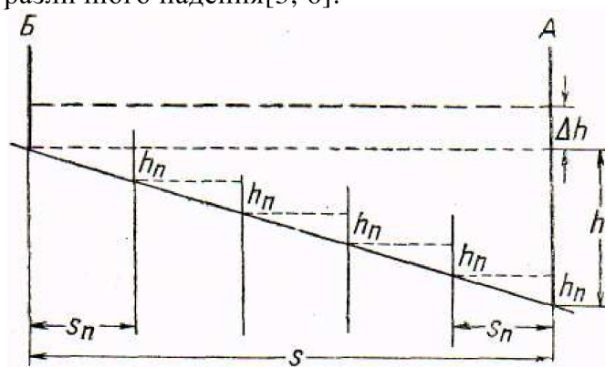
Рис. 1. Схема размещения точек однодневной связи (ТОС)
