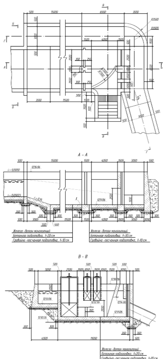
Рисунок 4 – Конструкция запроектированного напорного бассейна для каскада деривационных ГЭС на реке Усех
