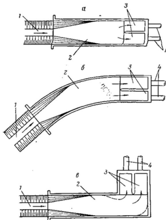
Рисунок 2 – Схемы подвода воды к водопримным камерам напорного бассейна: а – прямолинейный подвод воды; б – криволинейный подвод воды; в – подвод воды под углом 90°. 1 – деривационный канал; 2 – аванкамера; 3 – водопримные камеры; 4 – турбинный трубопровод
