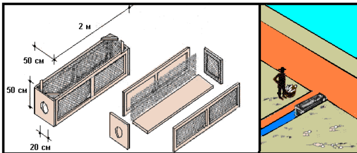
Рис. 21. Схема переносного рыбоуловителя и его установки.
