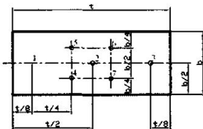
Рис. И.1 Схема измерения остаточных толщин листа (схема 1 - по трем точкам, схема 2 - по семи точкам)
