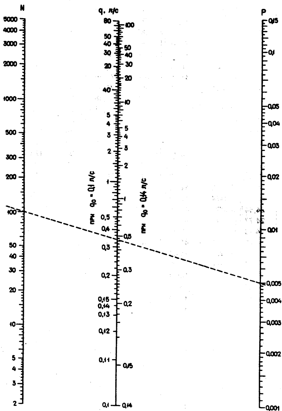
Черт. 1. Номограмма для определения секундных расходов воды q при q_0 = 0,1 и 0,14 \text{ л/с} и P \leq 0,15
