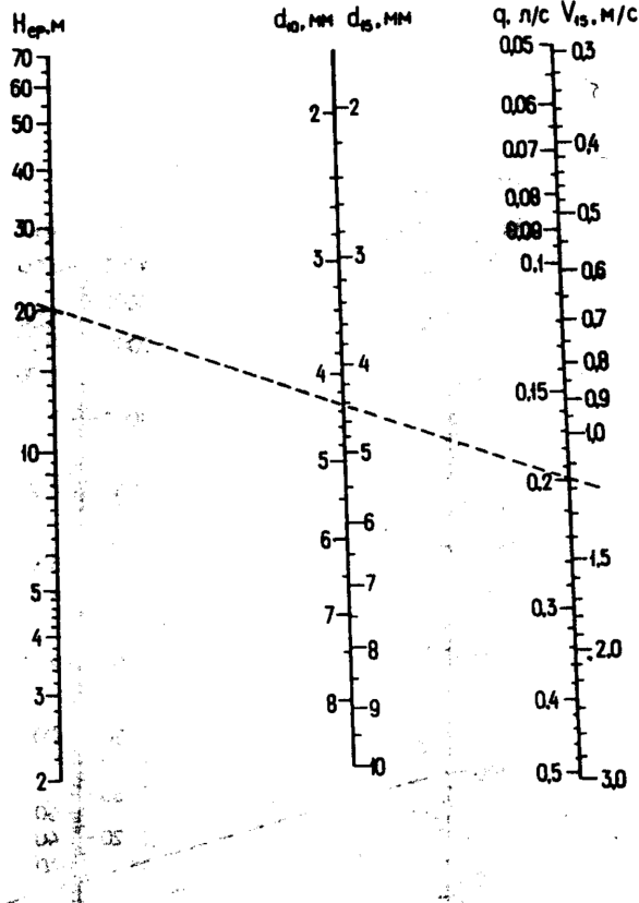
Черт. 6. Номограмма для определения диаметров отверстий диафрагм, устанавливаемых у смесителей водоразборной арматуры санитарных приборов
