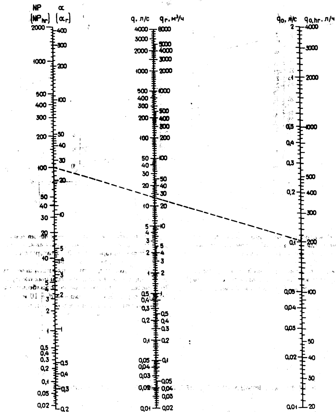
Черт. 4. Номограмма для определения секундных и часовых расходов воды в зависимости от NP ( NP_{\text{hr}} ) при различных значениях q_0, \text{л/с} , q_{0, \text{hr}}, \text{л/ч}
