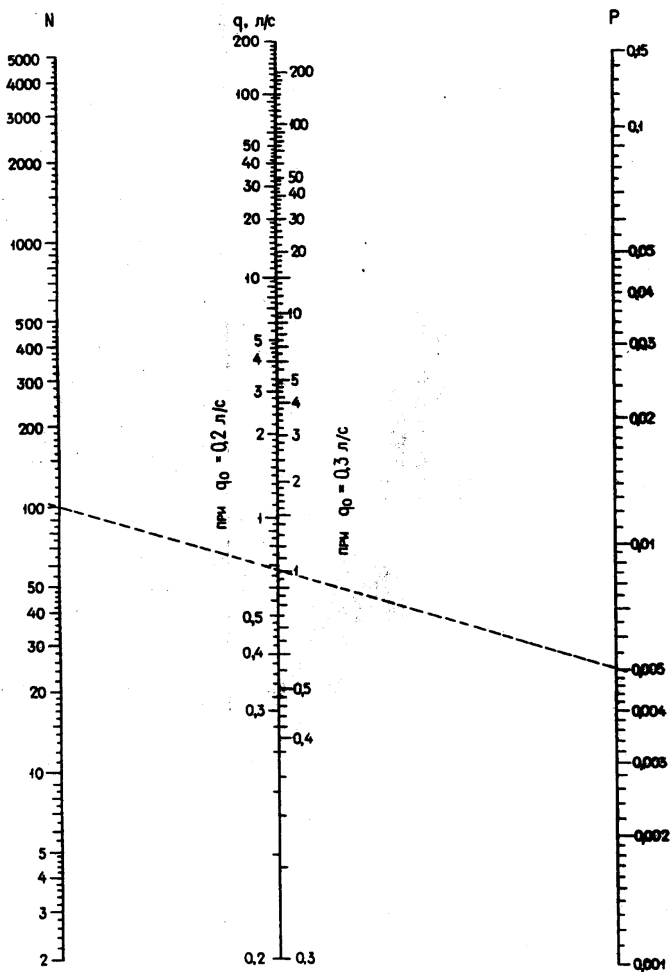
Черт. 2. Номограмма для определения секундных расходов воды q при q_0 = 0,2 и 0,14 л/с и P \leq 0,15
