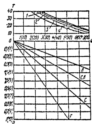
Рис. 2. Номограмма для определения рабочего давления в трубопроводе из РВП в зависимости от срока службы трубопровода и температуры транспортируемой среды
