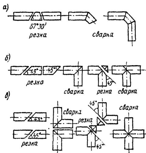
Рис. 22. Схема процесса изготовления фасонных частей контактной стыковой сваркой а — отводы и колена, б — тройники; в — крестовины
