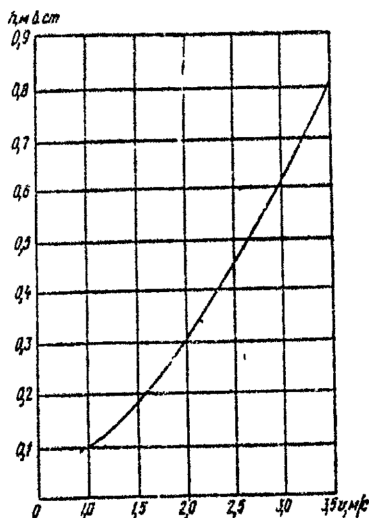
Рис. 7. Потери напора в односегментном крене
