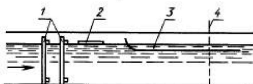
Средства для стабилизации потока в открытом канале
