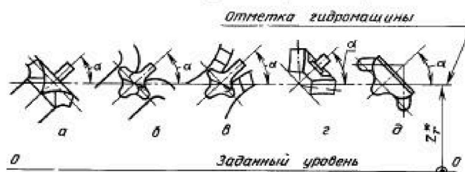
Схема отметки гидромашин ( 0^\circ \leq \alpha \leq 90^\circ )
