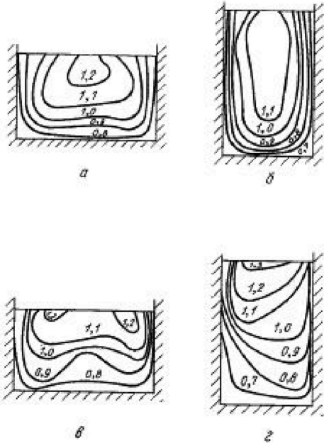
a, б — поля скоростей нормального распределения; в, г — поля скоростей с отклонением от нормального распределения, приводящим к предельным погрешностям определению расхода
