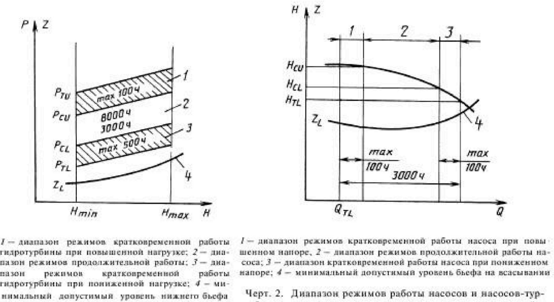
Черт. 1. Диапазоны режимов работы гидротурбин
