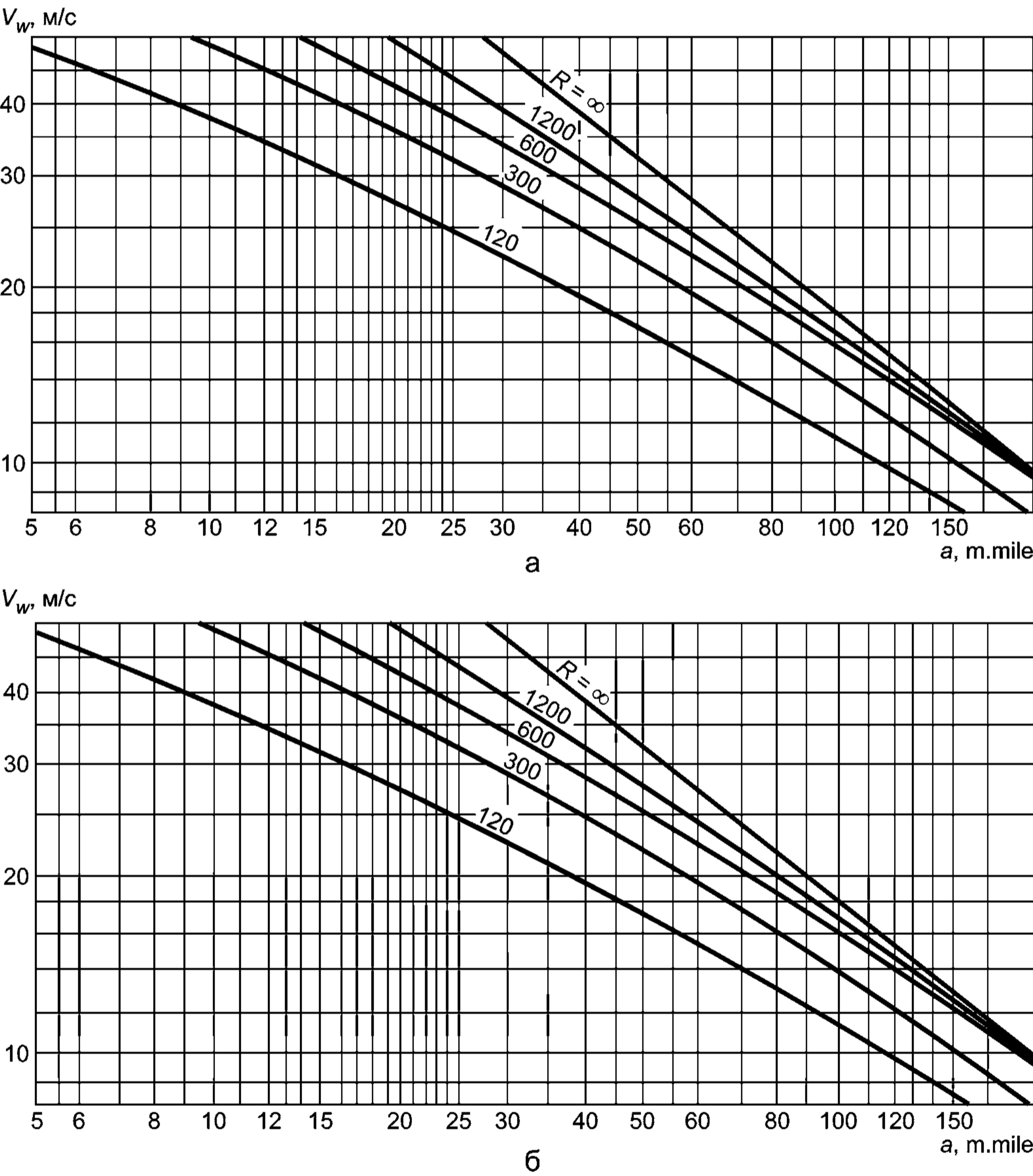
а – \varphi \geq 50^\circ с.ш.; б – \varphi \geq 35^\circ - 49^\circ с.ш.
