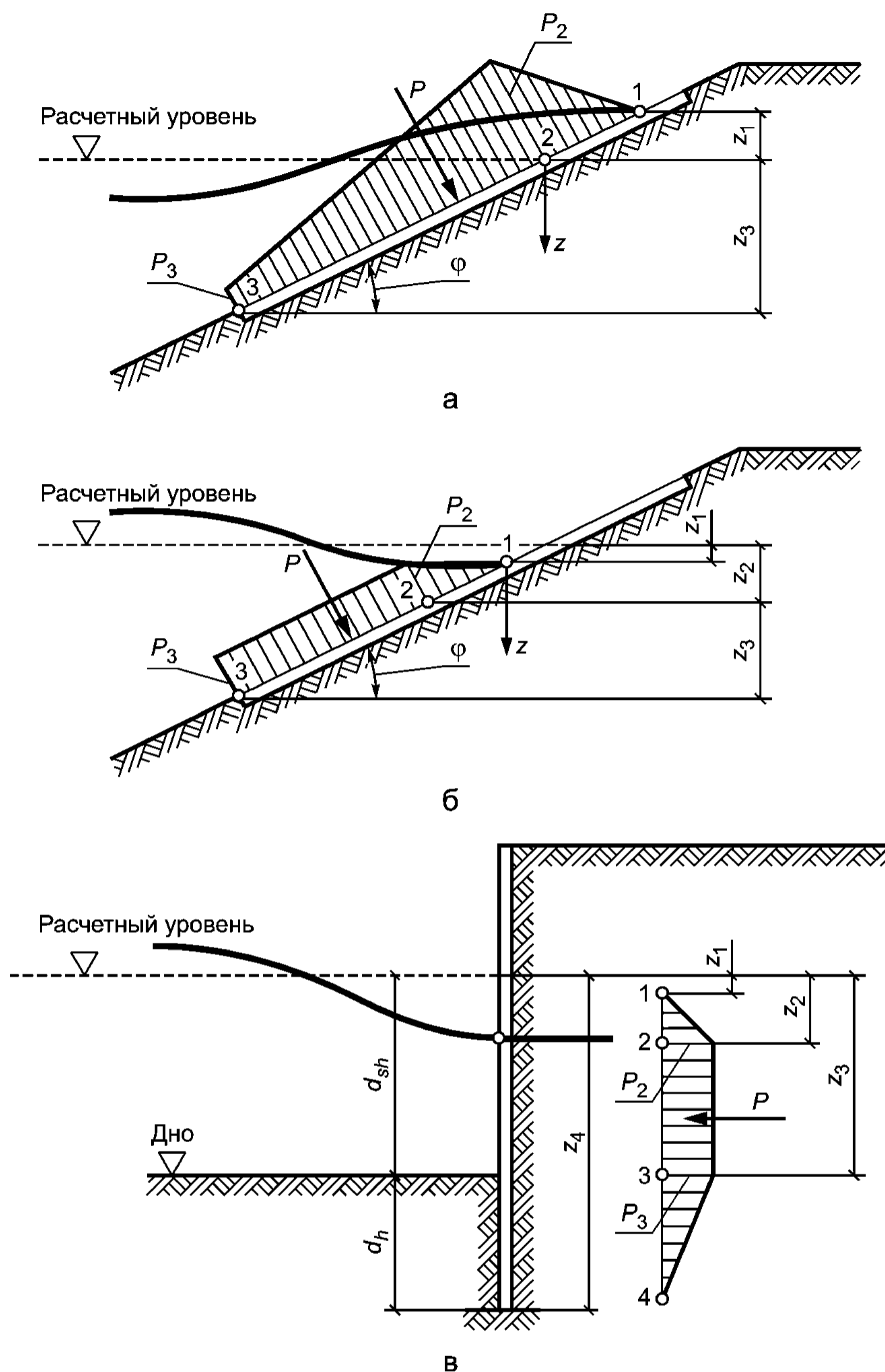
а — при накате волны на откос; б — при откате волны с откоса; в — при ложбине волны у вертикальной стены
