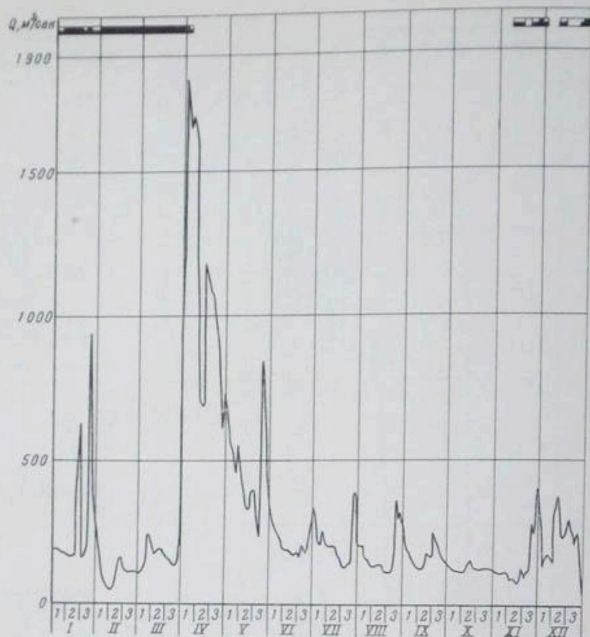
Рис. 1.9д. Гидрограф р. Днестра у с. Каменка за 1956 г.
