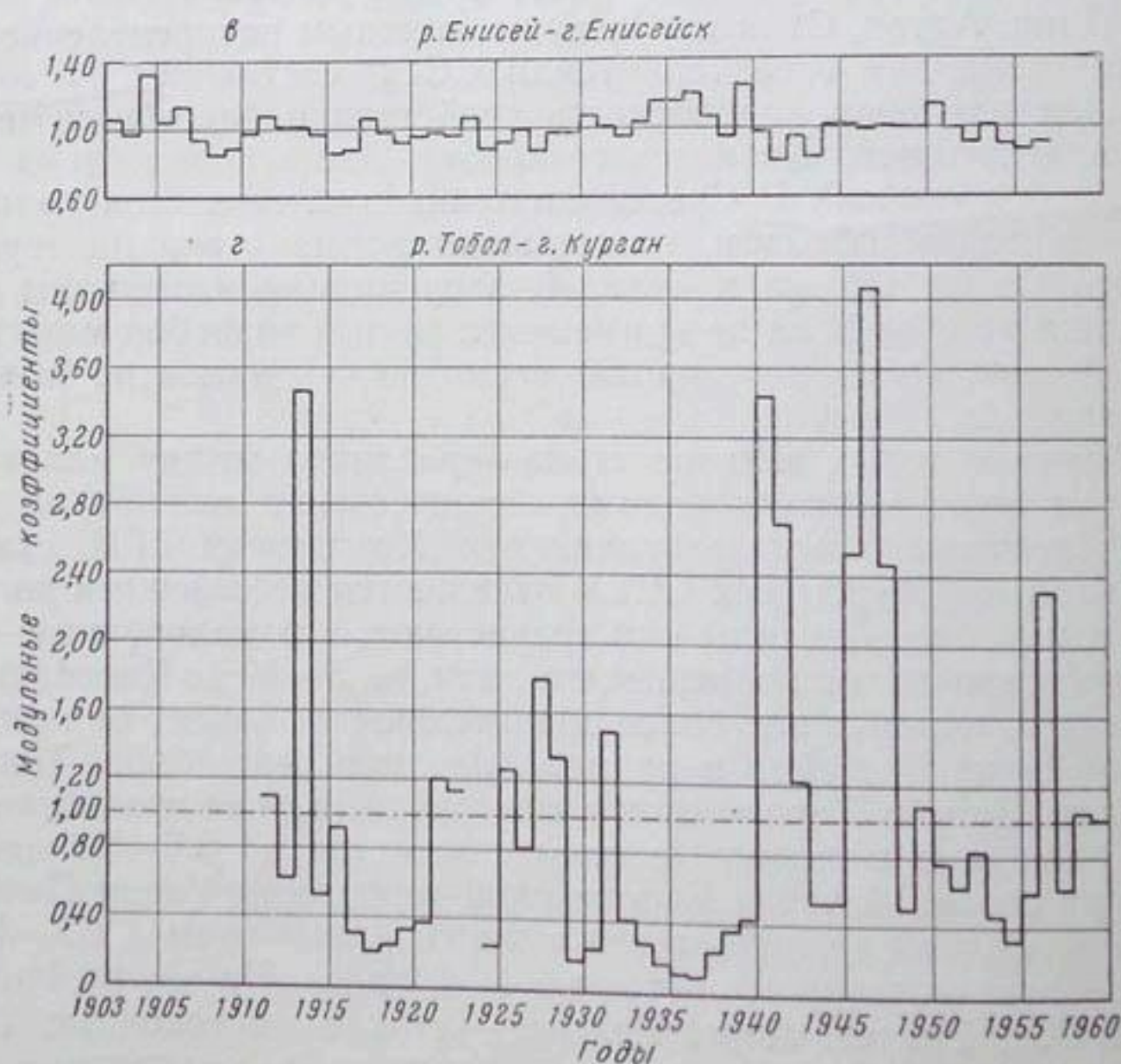
Рис. 1.7. Диаграмма многолетних колебаний средних годовых расходов воды рек а — Дона; б — Волги; в — Енисея; г — Тобола
