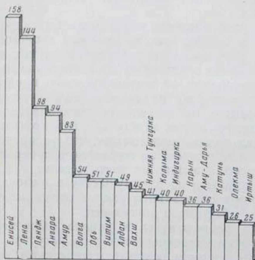
Рис. II.4. Потенциальные гидроэнергетические ресурсы наиболее мощных рек СССР (в млрд. кВт·ч)
