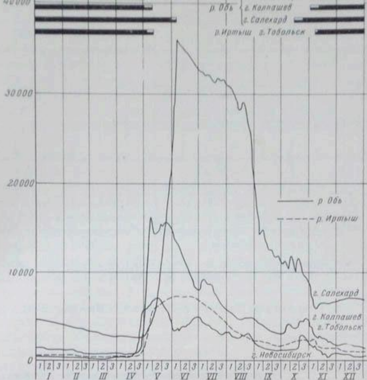
Рис. 1.9ж. Гидрограф р. Оби у г. Новосибирска, г. Ковпашёва и г. Салехарда и р. Иртыша у г. Тобольска за 1942 г.
