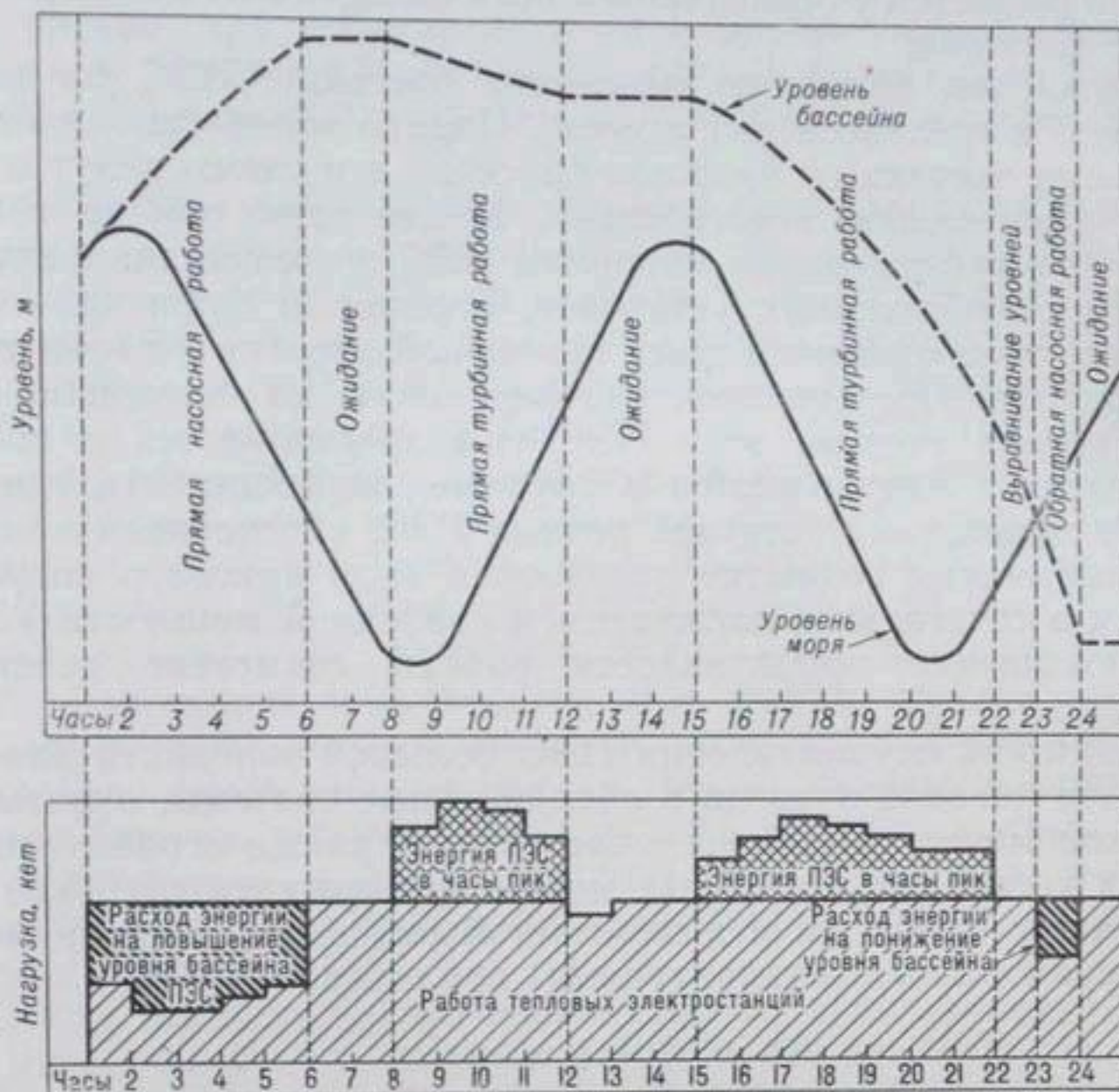
Рис. VI.6. Пример работы ПЭС в пиковом режиме. В ночные часы свободная мощность ТЭС используется для насосной работы турбин по подкачке уровня бассейна, который сбрасывается в часы пик
