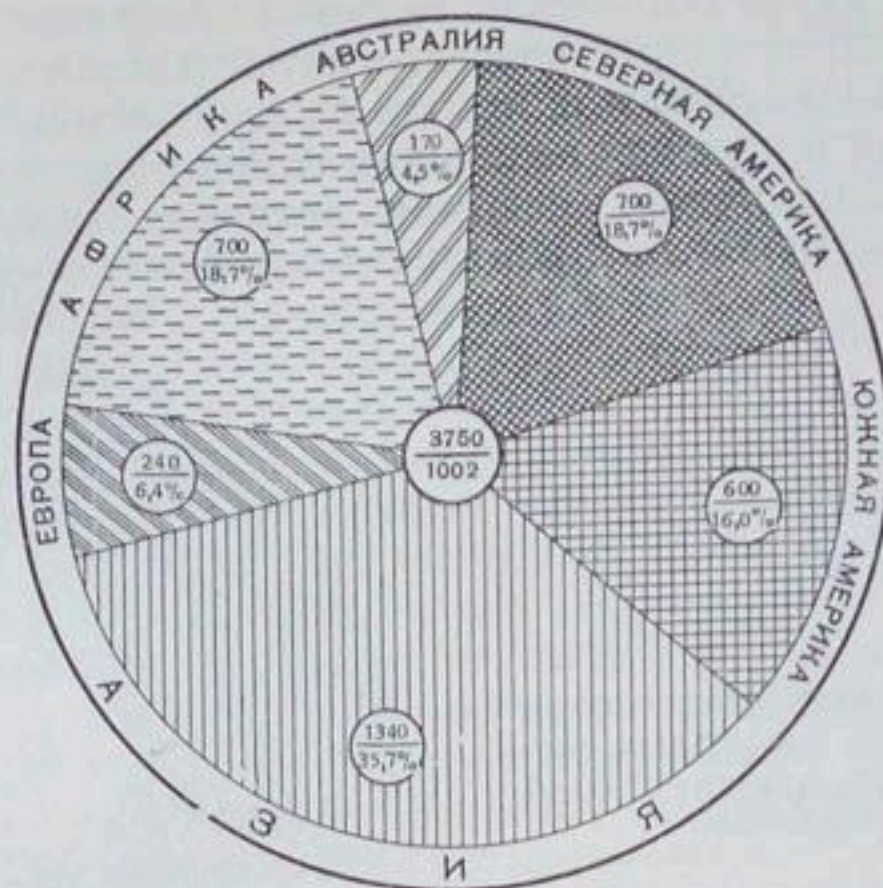
Рис. VII.2. Валовой потенциал энергии речного стока отдельных континентов (в млн. квт и в процентах от общего потенциала)
