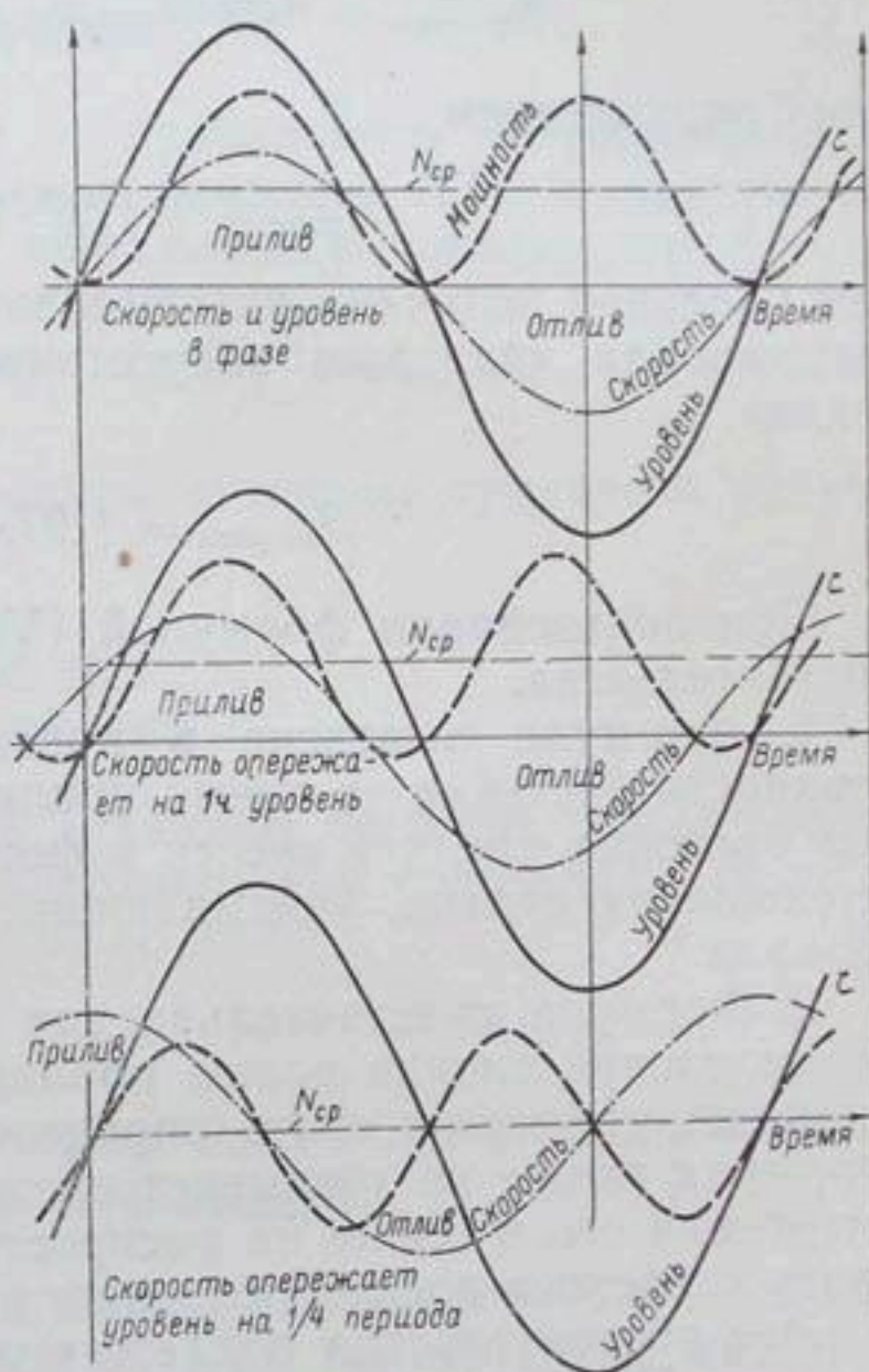
Рис. VI.7. Кривые мощности, уровня и скорости прилива
