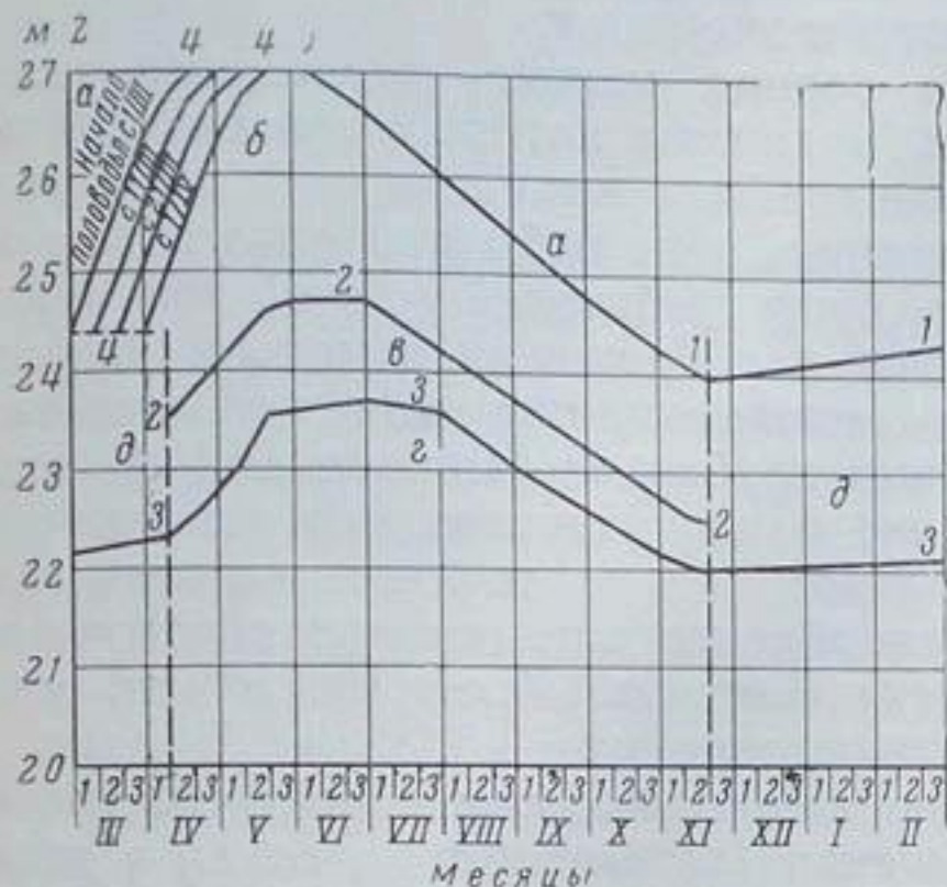
Рис. X.4. Диспетчерский график работы Цимлянского водохранилища. Первый этап эксплуатации
