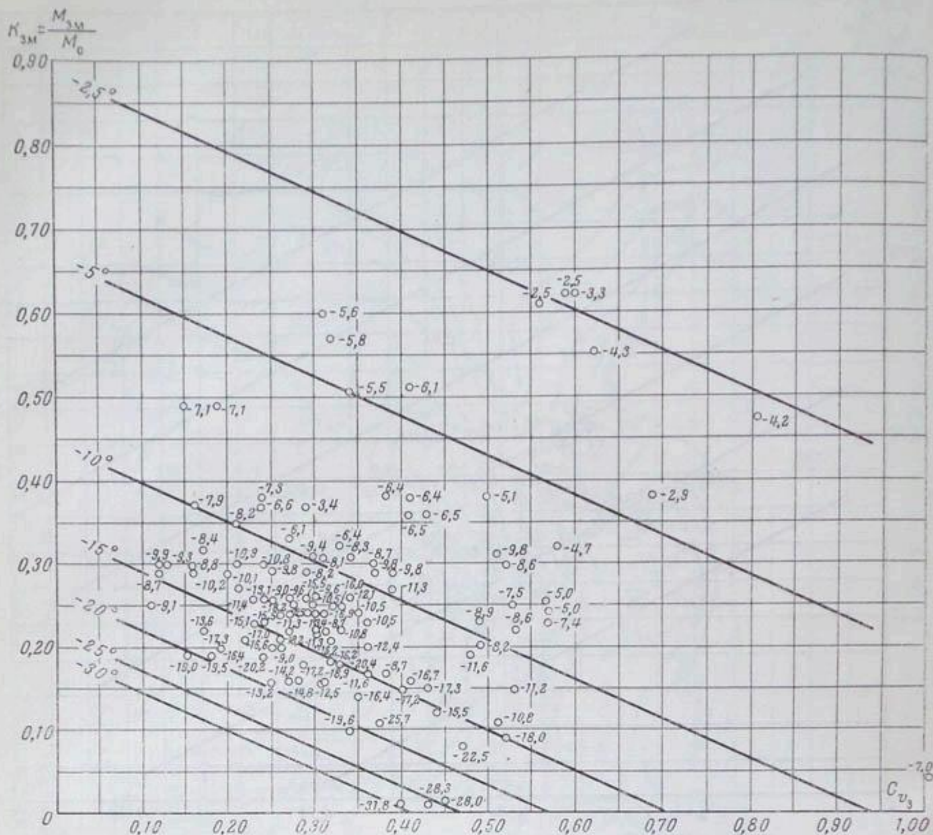
Рис. IV.6. Связь C_v и K среднемесячного зимнего стока
