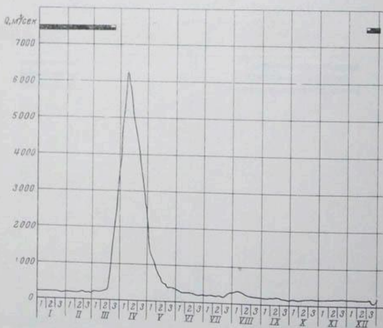
Рис. 1.9е. Гидрограф р. Дона у г. Калач за 1913 г.
