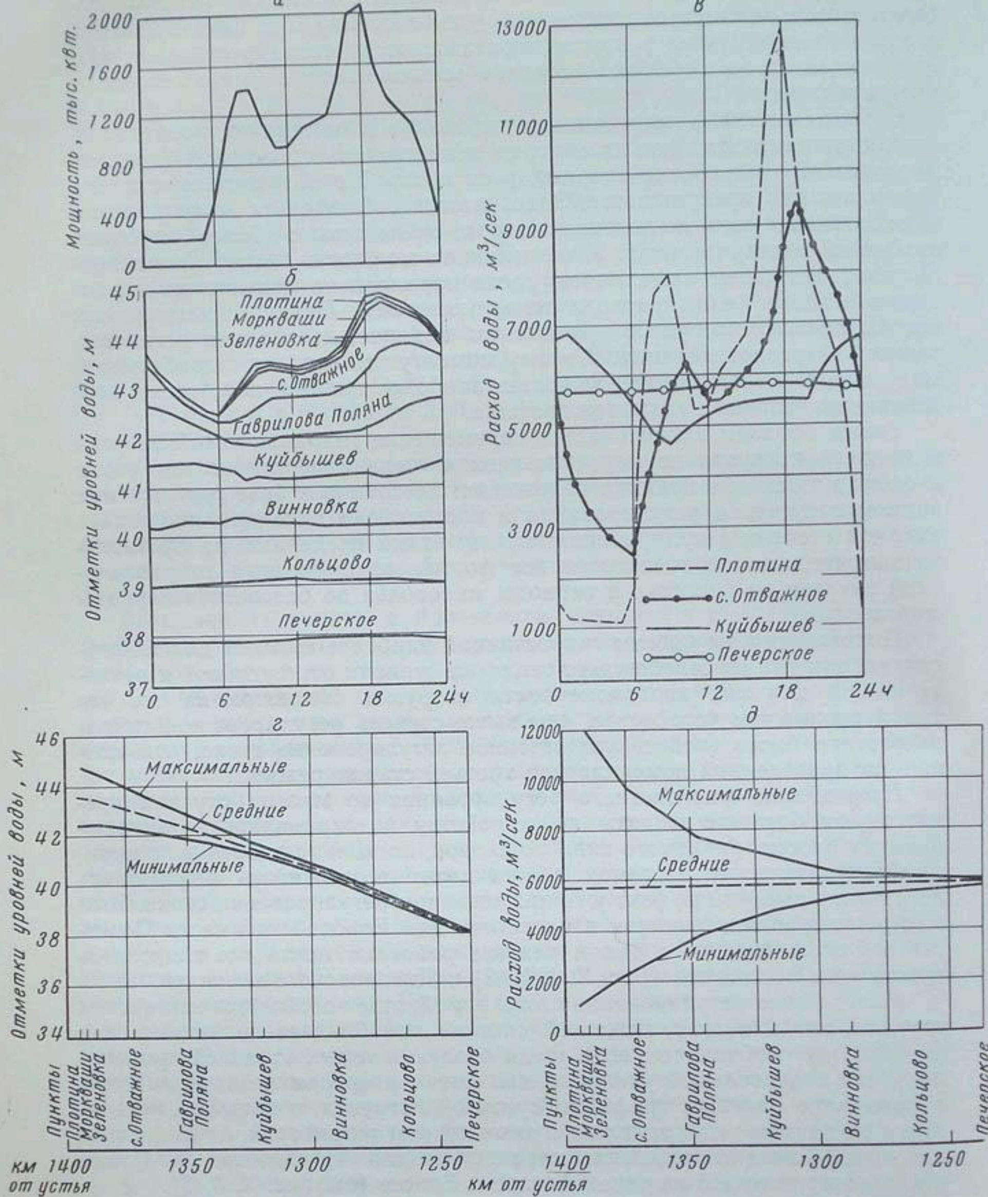
Рис. X.1. Режим нижнего бьефа Волжской ГЭС имени В.И. Ленина при суточном регулировании в декабре маловодного года при неподпертом бьефе
