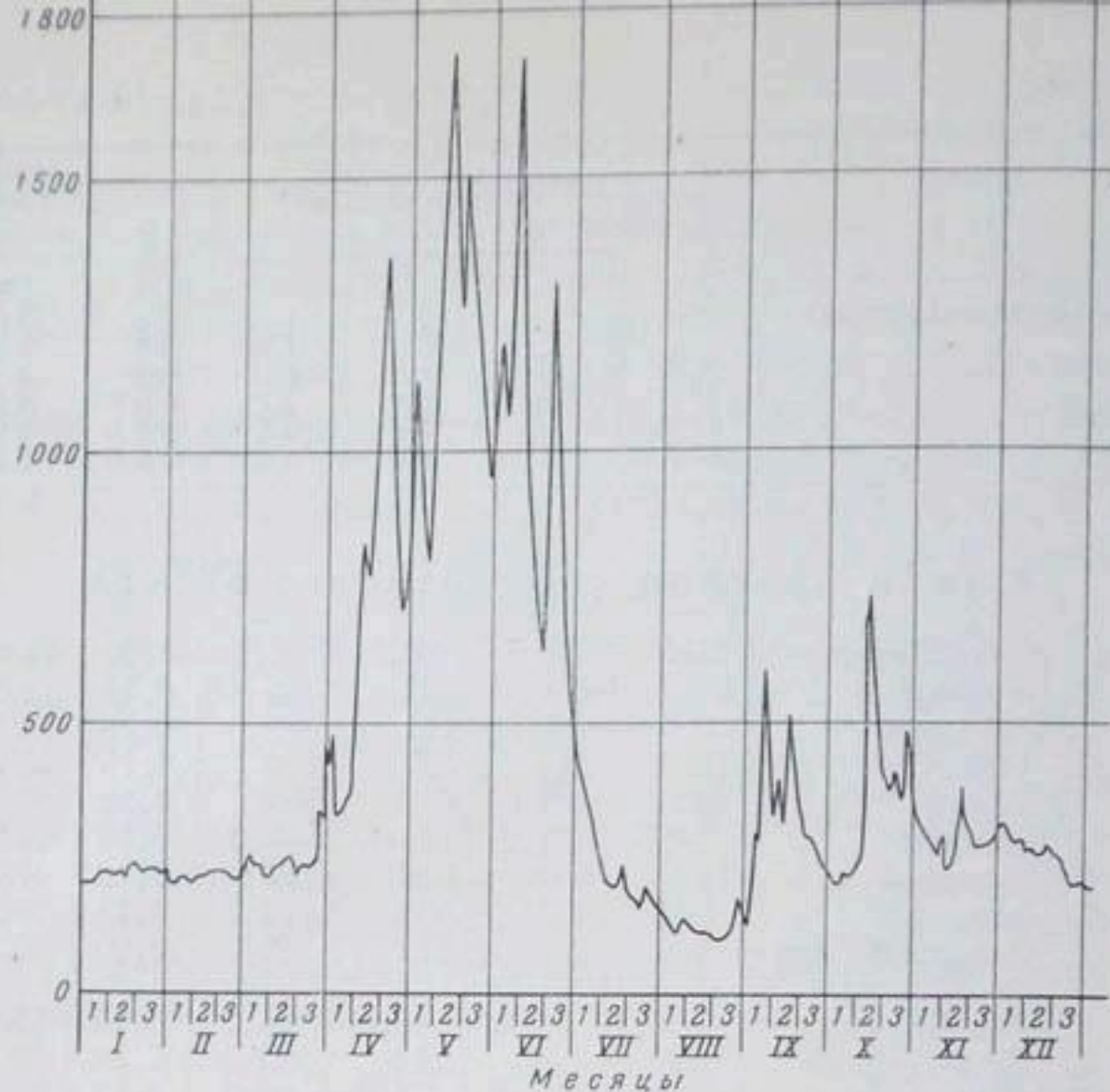
Рис. 1.9а. Гидрограф р. Куры у с. Мингечаур за 1948 г.
