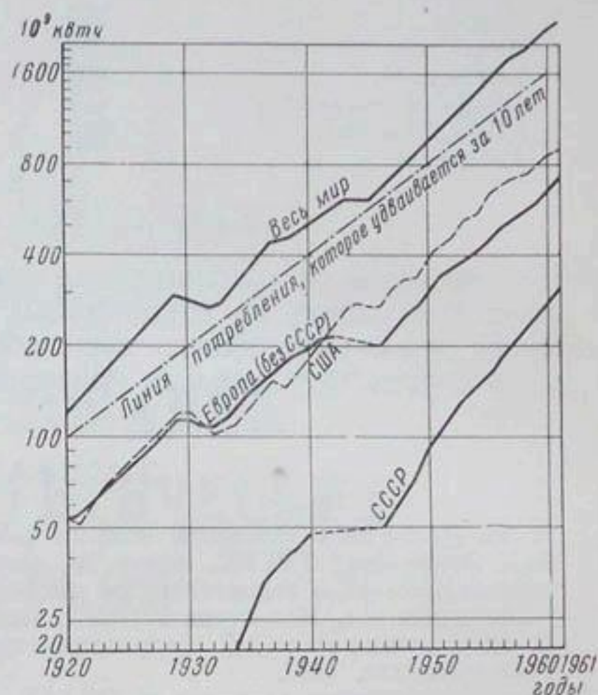
Рис. VII.3. Кривые валового потребления электроэнергии всего мира, Европы (без СССР), СССР и США за 1920—1961 гг. (полулогарифмическая шкала)
