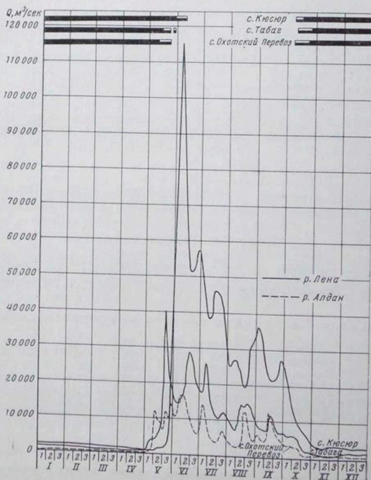
Рис. 1.9б. Гидрографы р. Лены у с. Кюсюр и с. Габага и р. Алдана у с. Охотский Перевоз за 1952 г.
