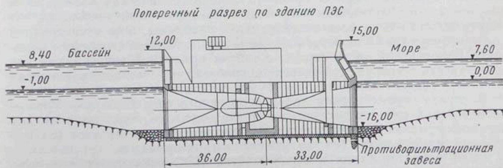
Рис. VI.10. Здание Лумбовской ПЭС (проект 1964 г.)
