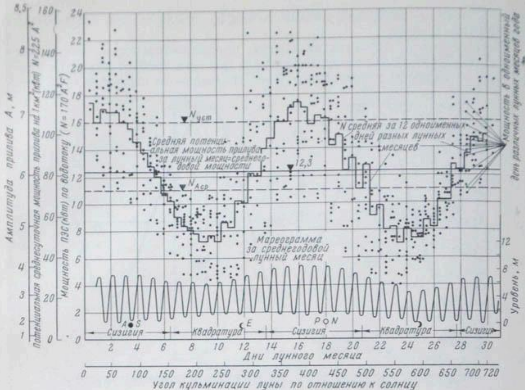
Рис. VI.4. Изменение мощности прилива за лунный (синодический) месяц. Район Беломорской ПЭС [1]. Коэффициент прилива принят равным 2 по отношению к основному пункту Сосновец
