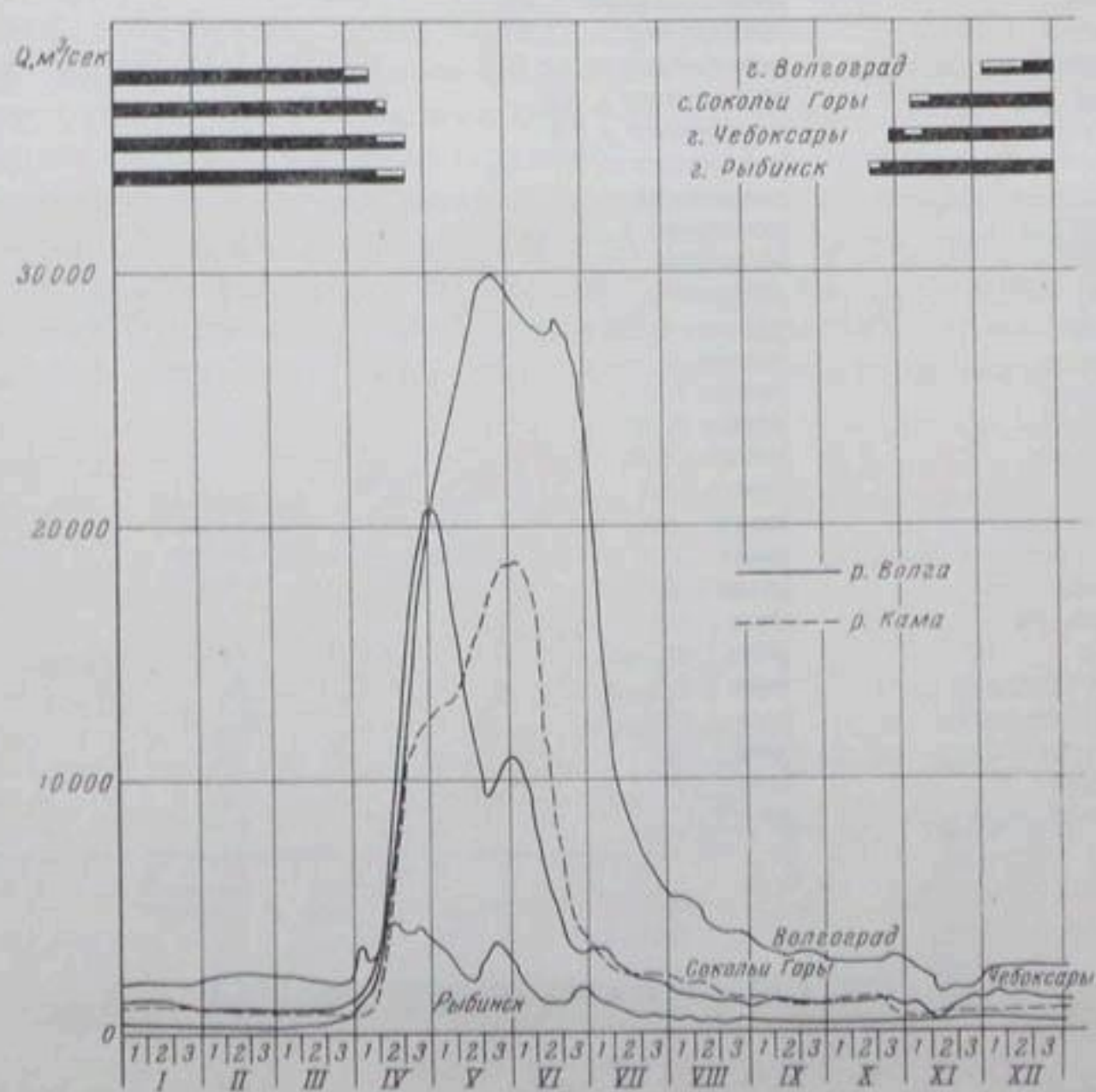
Рис. 1.9з. Гидрографы р. Волги у г. Рыбинска, г. Чебоксары и г. Волгограда и р. Камы у с. Соколы Горы за 1912 г.
