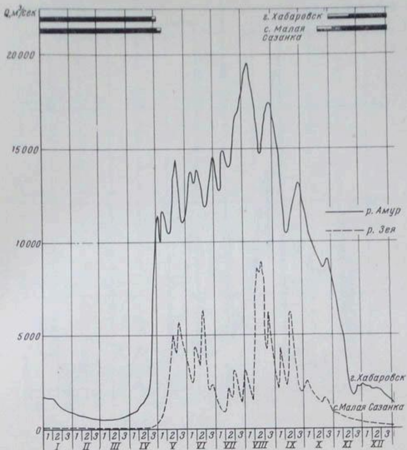
Рис. 1.9в. Гидрографы р. Амура у г. Хабаровска и р. Зеи у с. Малая Сазанка за 1942 г.
