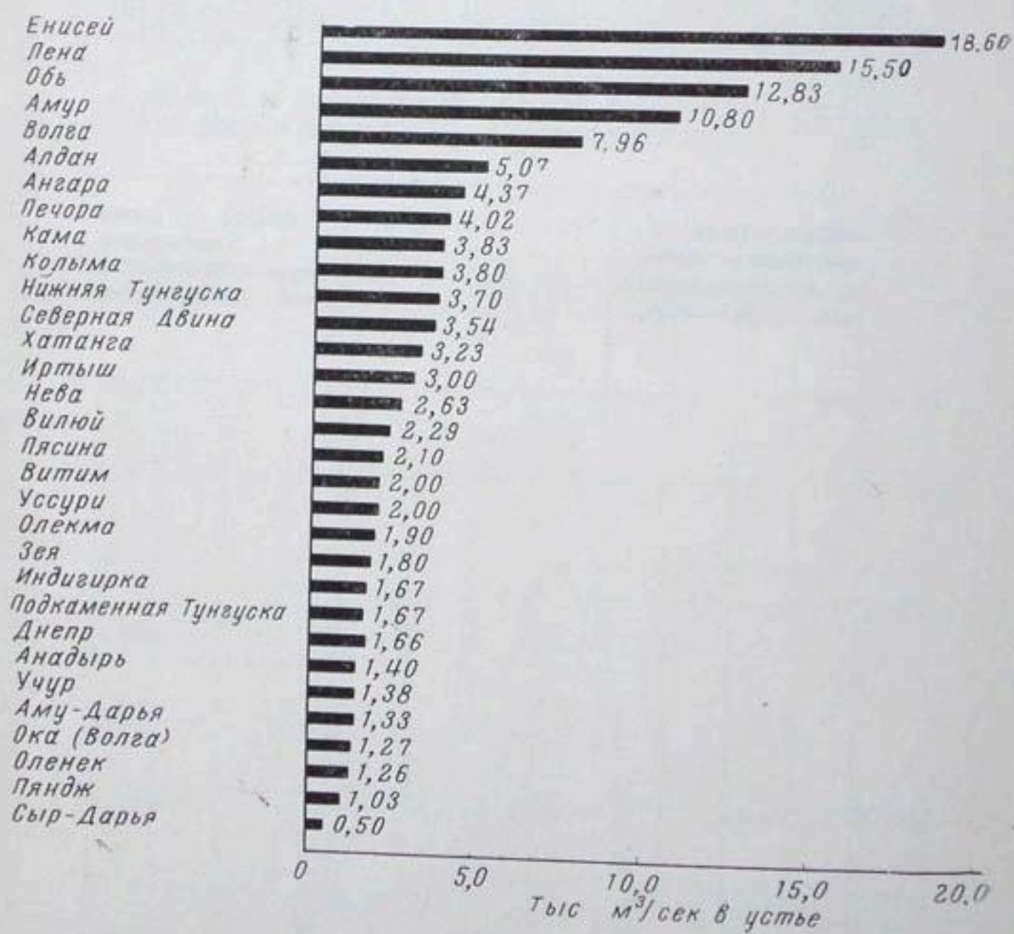
Рис. 1.10. Диаграмма водности рек СССР
