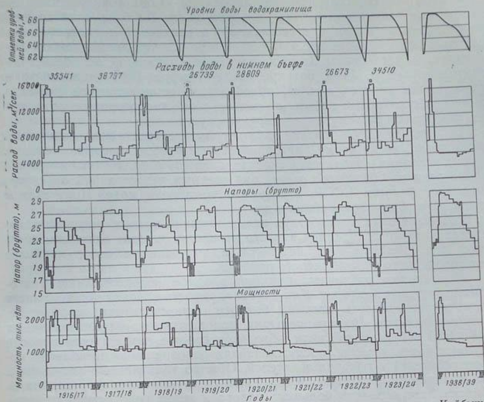
Рис. X.2. Хронологические графики изменения основных элементов режима Куйбышевского водохранилища и Волжской ГЭС имени В. И. Ленина. Начальный этап работы
