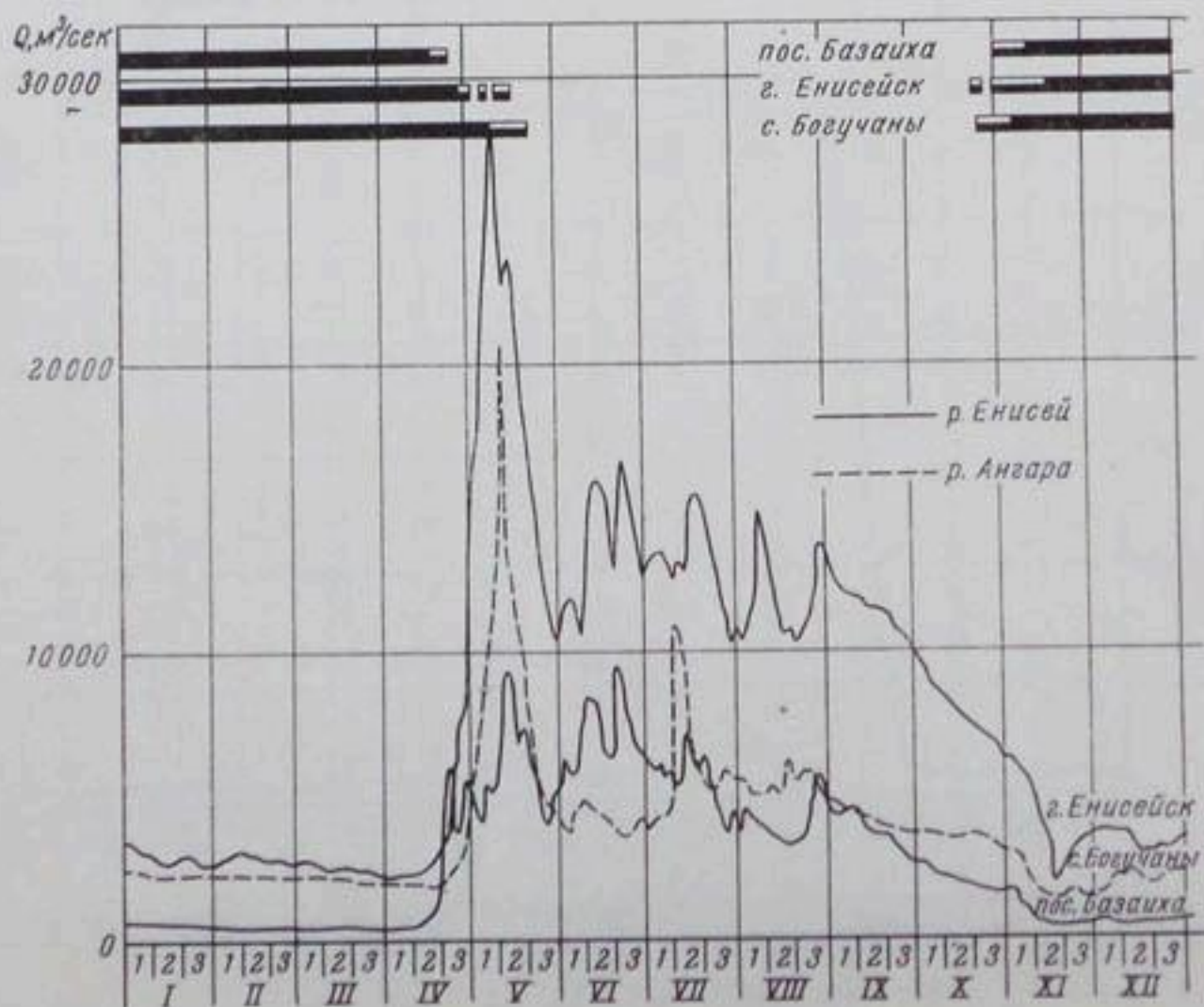
Рис. 1.9г. Гидрографы р. Енисея у г. Енисейска и пос. Базайха за 1949 г. и р. Ангара у с. Богучаны за 1953 г.
