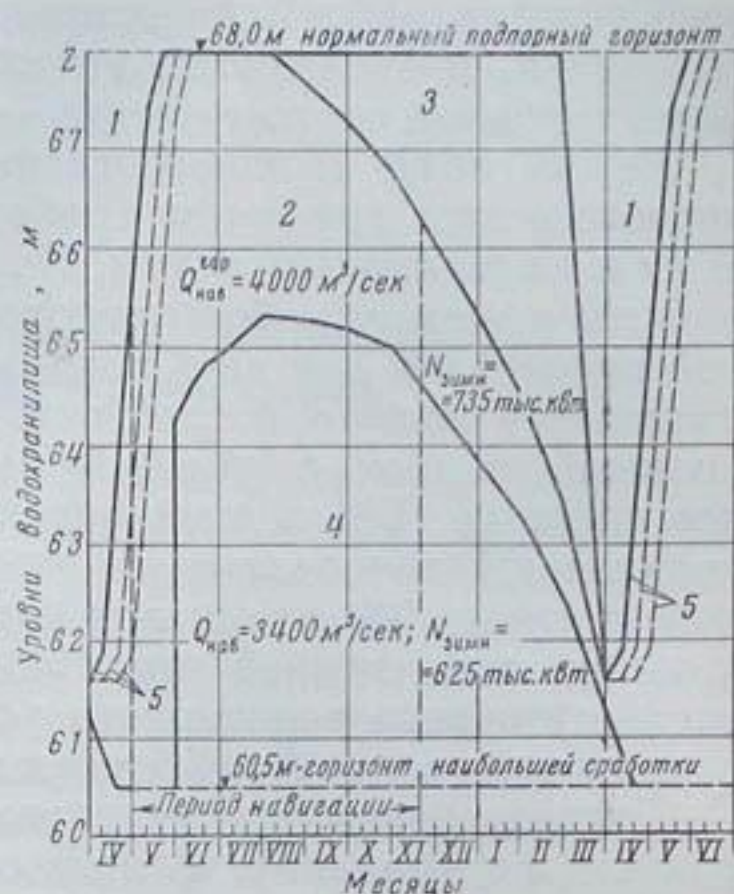
Рис. X.5. Диспетчерский график работы Куйбышевского водохранилища для ближайшего этапа его эксплуатации
