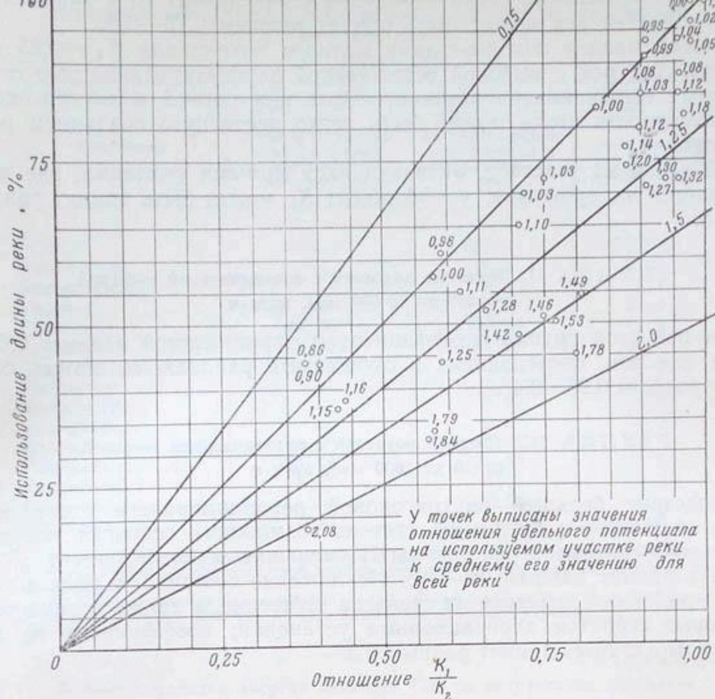
Рис. III.2. Зависимость между использованием длины реки и отношением K_1/K_2
