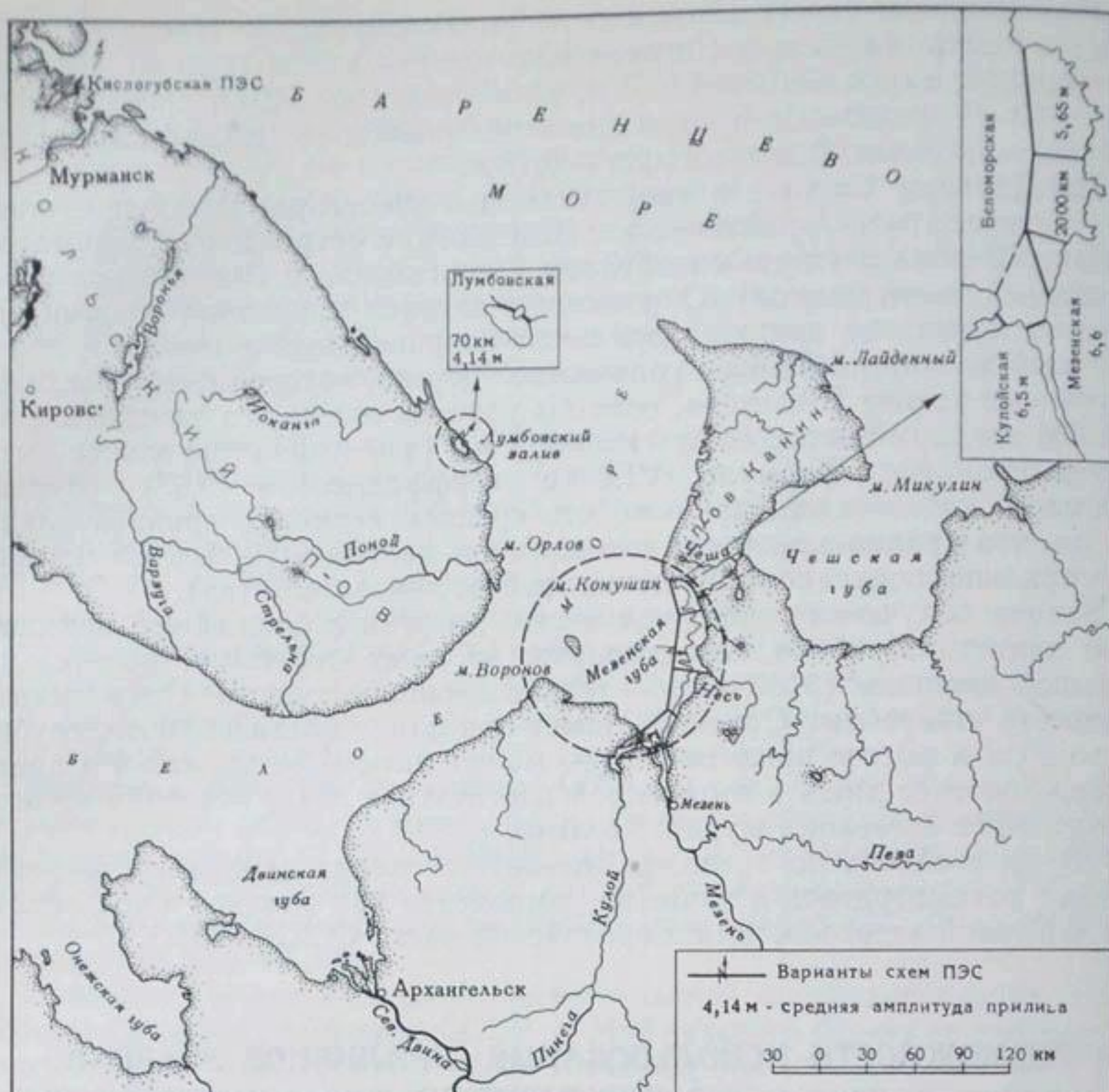
Рис. VI.8. Варианты приливных электростанций на побережье Белого моря
