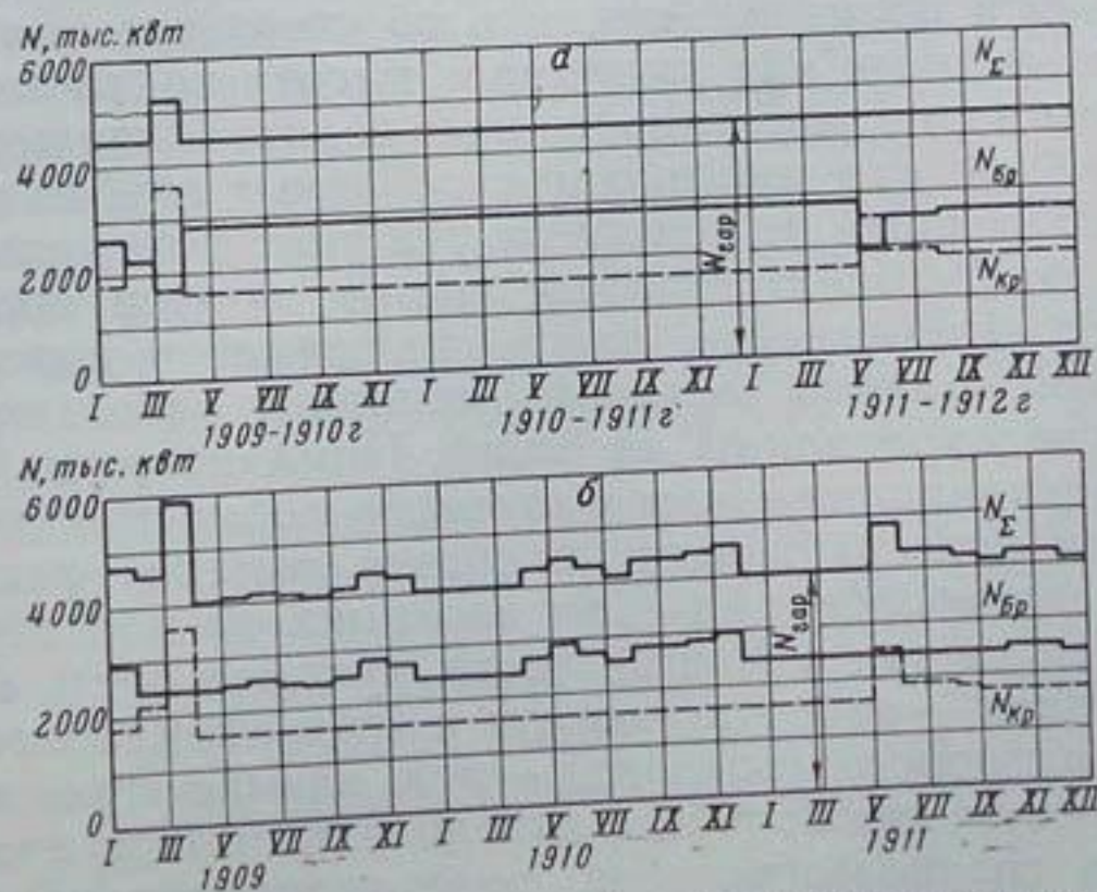
Рис. X.3. Хронологический график среднемесячных мощностей Братской ( N_{Бр} ) и Красноярской ( N_{Кр} ) ГЭС при их совместной (а) и раздельной (б) работе
