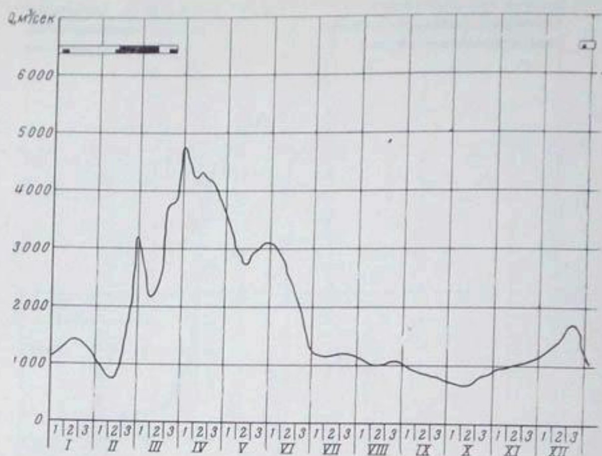
Рис. 1.9н. Гидрограф р. Днепра у с. Лоцманская Каменка за 1923 г.
