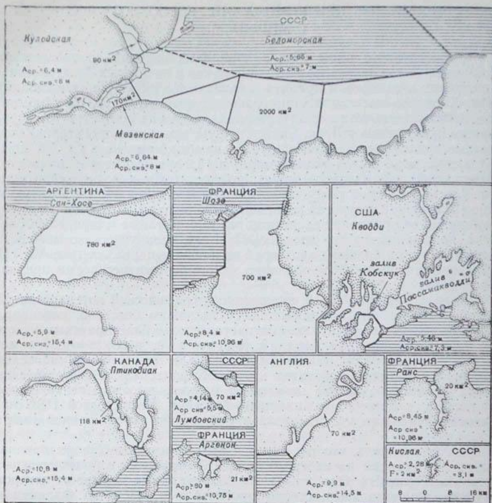
Рис. VI.11. Планы заливов, в которых проектируются приливные электростанции [1].
