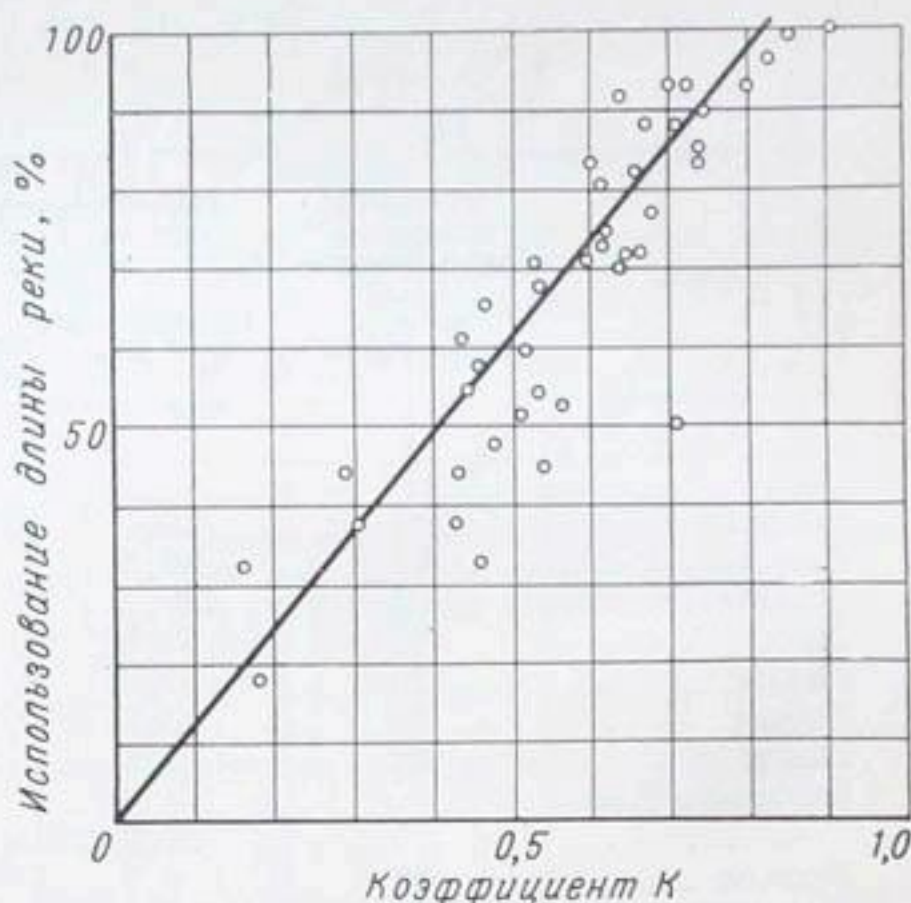
Рис. III.1. Зависимость коэффициента K_1 от используемой длины реки
