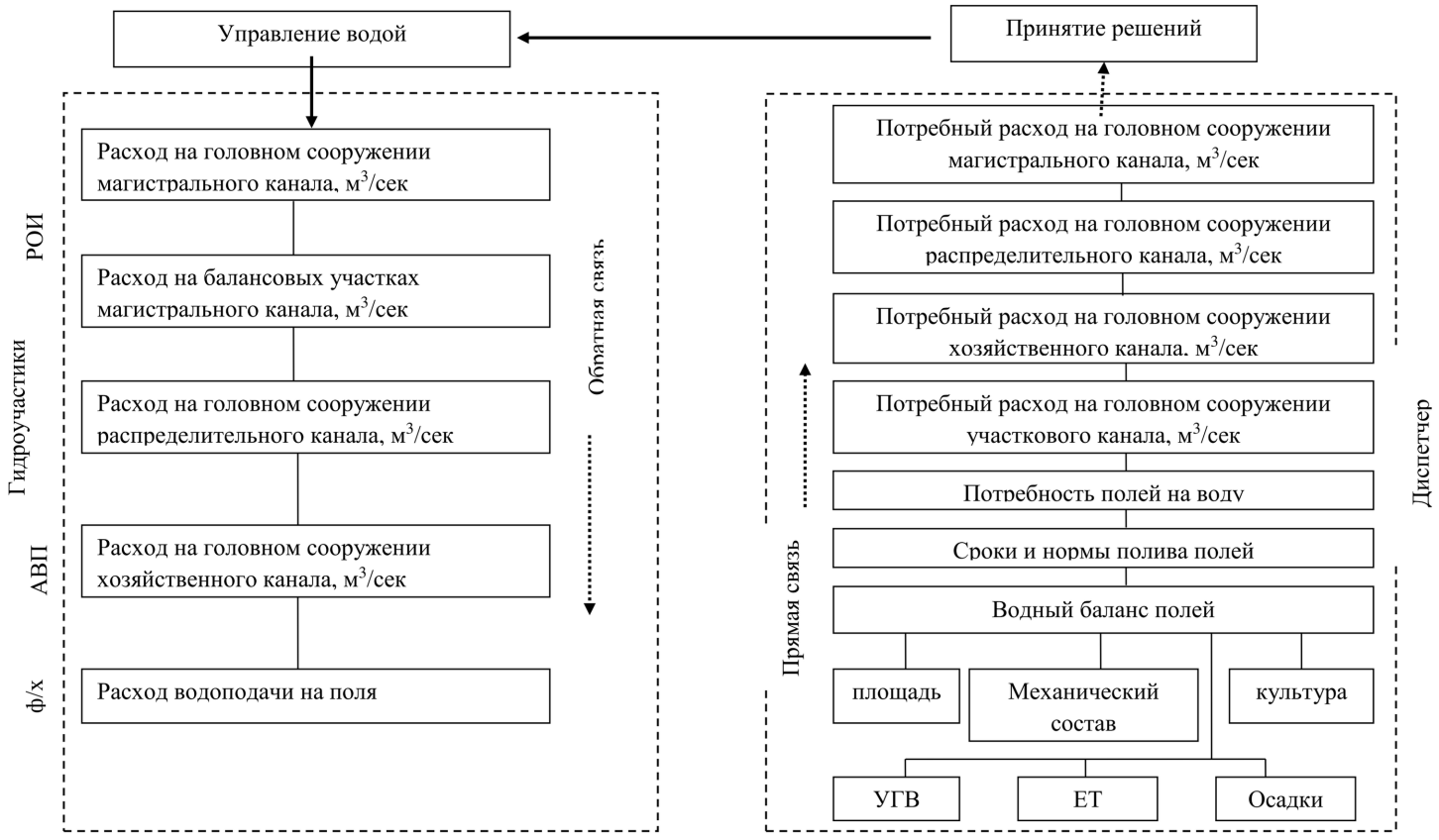
Рисунок 1.1. Рекомендуемая схема планирования и распределения воды.
