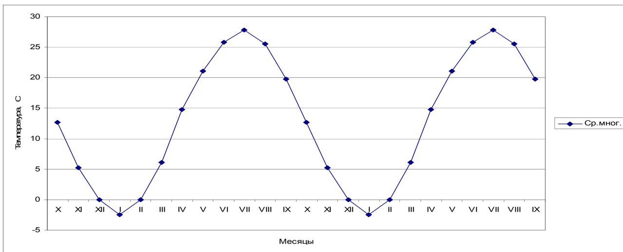
Рис.1.1. Сезонное изменение температуры воздуха по среднегодовым данным (осредненно по 11 метеостанциям региона)
