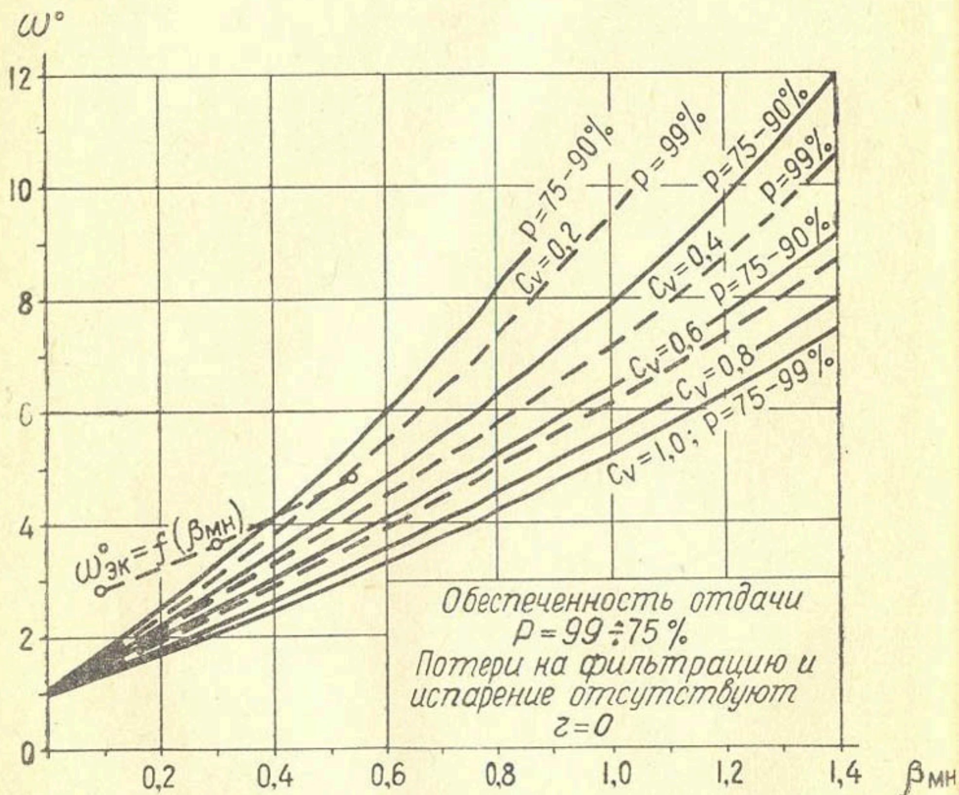
Рис. 13. Графики для определения потребной полезной емкости водохранилища многолетнего регулирования стока рек на 1 \text{ м}^3 увеличения годовой гарантированной отдачи воды.
