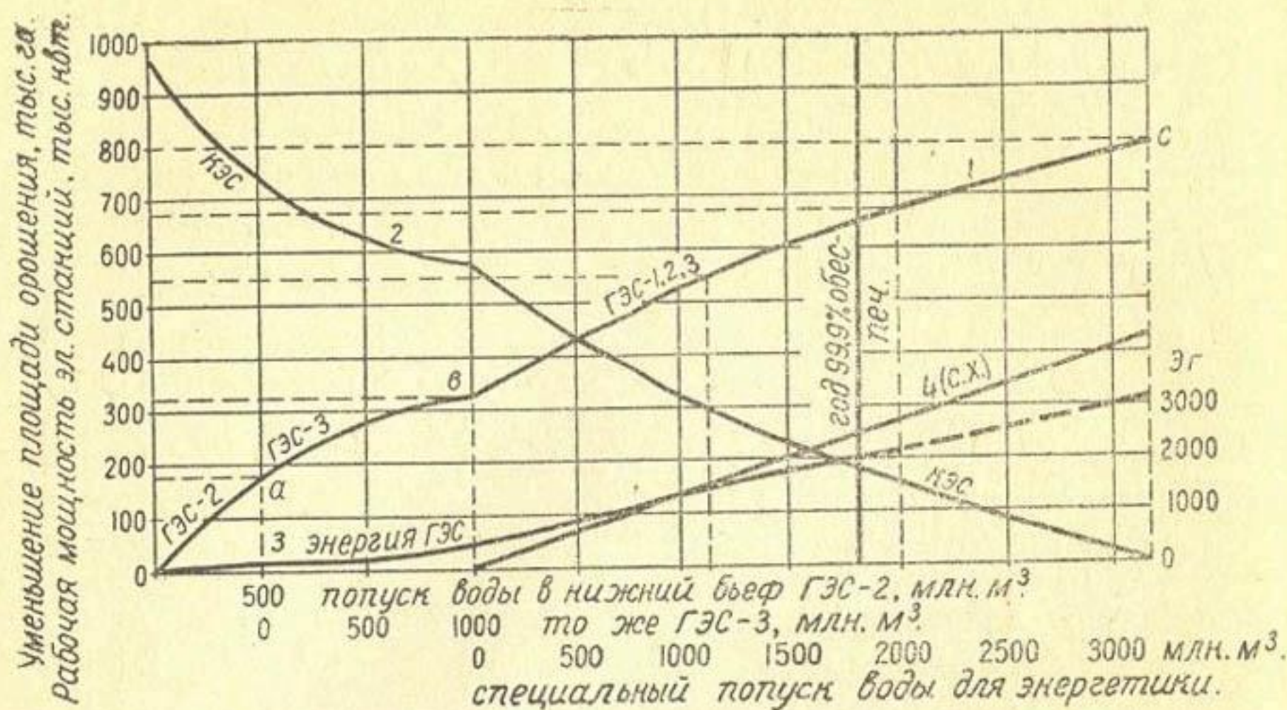
Рис. 50. Зависимости рабочей мощности 1 и средней многолетней выработки энергии 2 проектируемого каскада ГЭС, мощности заменяющей КЭС 3 и снижения величины площади орошения 4 от потребности воды ГЭС за невегетационный период года.
