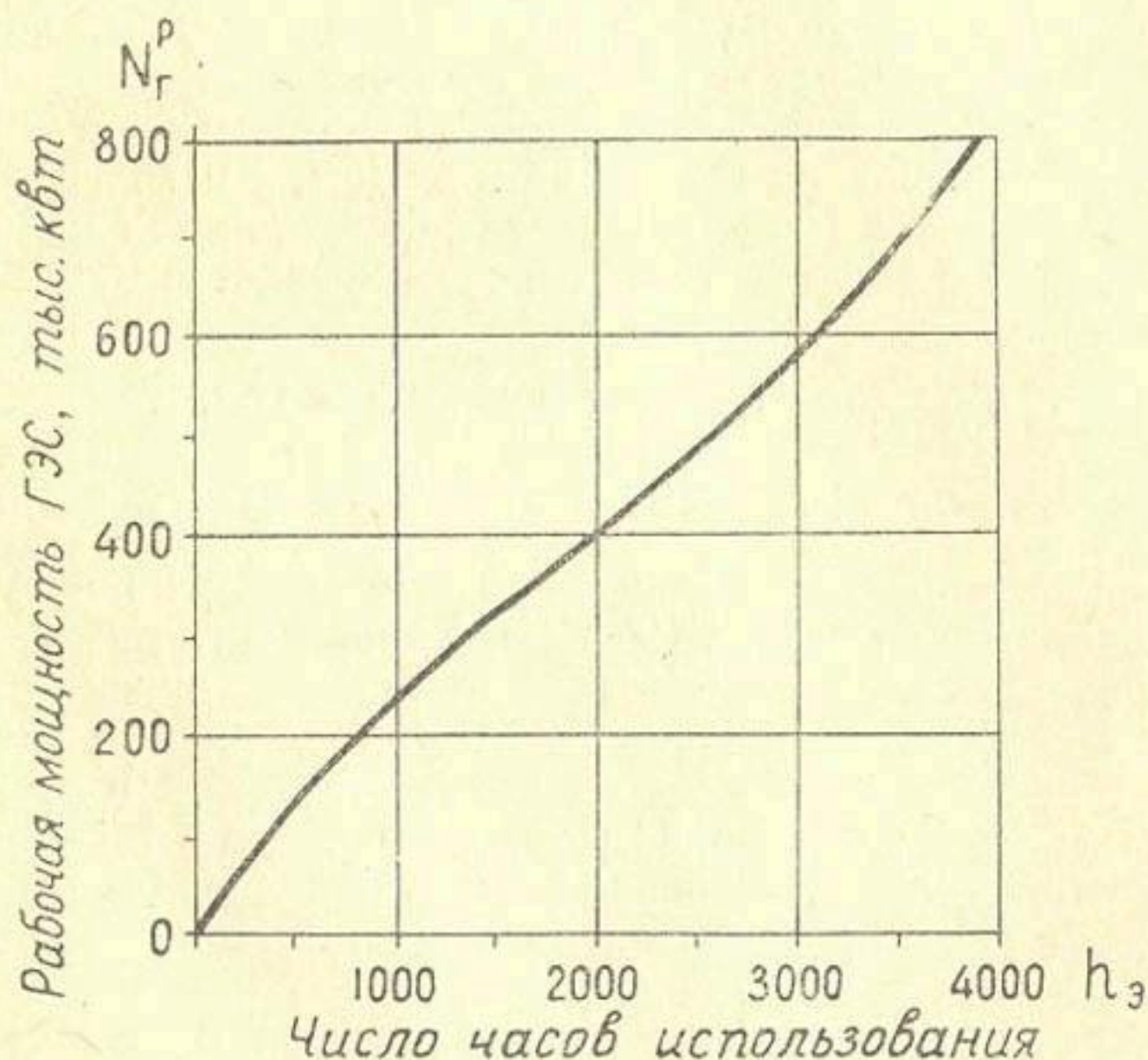
Рис. 56. Зависимость числа часов использования дополнительного киловатта проектируемой ГЭС в графике нагрузки энергосистемы за невегетационный период года h_z от величины ее рабочей мощности N_r^p
