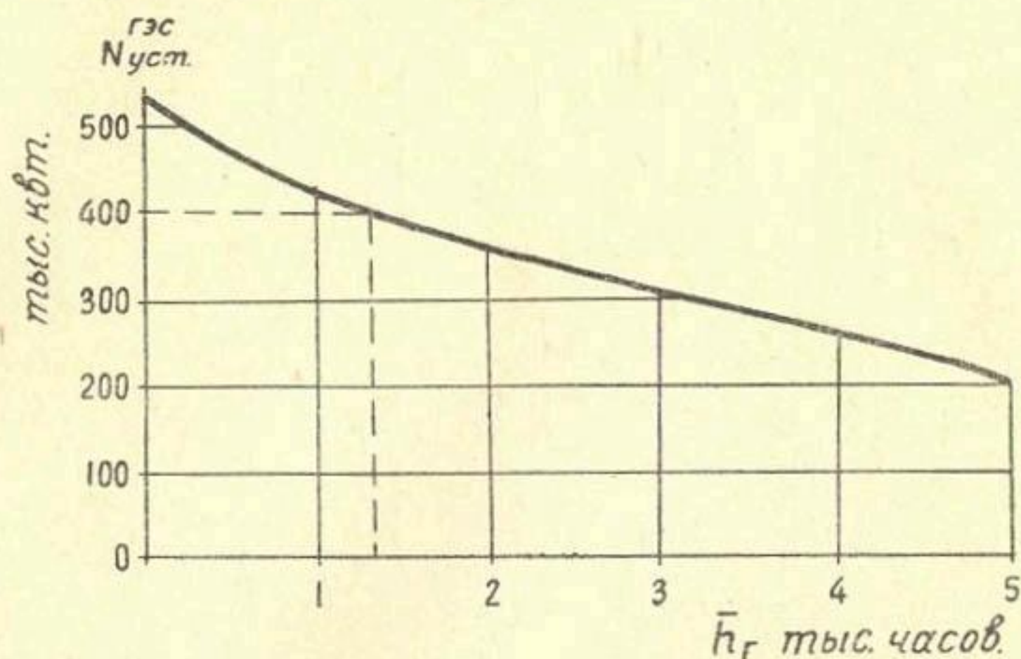
Рис. 37. Зависимость среднего многолетнего числа часов использования дополнительного киловатта \bar{h}_r от установленной мощности ГЭС N_{уст}
