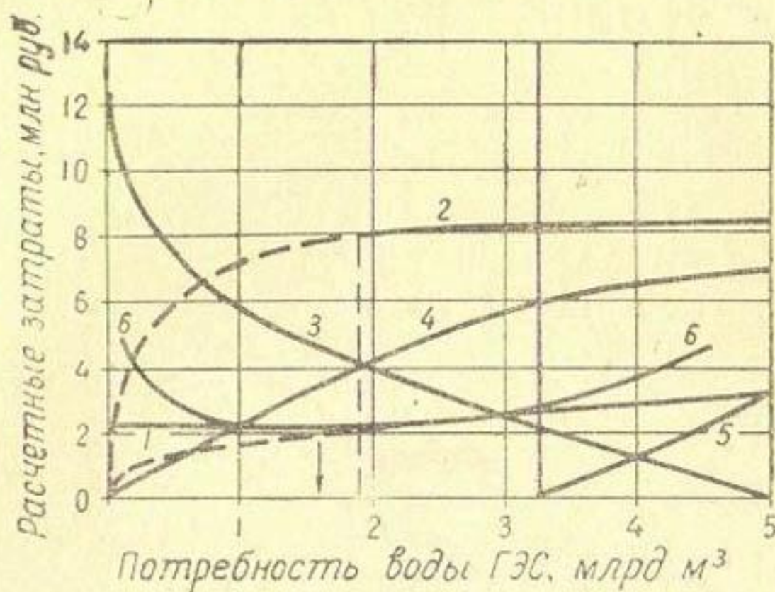
Рис. 36. Среднегодовые расчетные затраты в ГЭС 1, сэкономленное топливо 2, в заменяющую КЭС 3, дополнительные затраты в сельское хозяйство 4, компенсацию дефицита электроэнергии в системе 5 и сумма 6 в зависимости от годовой потребности воды ГЭС для покрытия гарантируемой зоны графика нагрузки энергосистемы (схема II-а).
