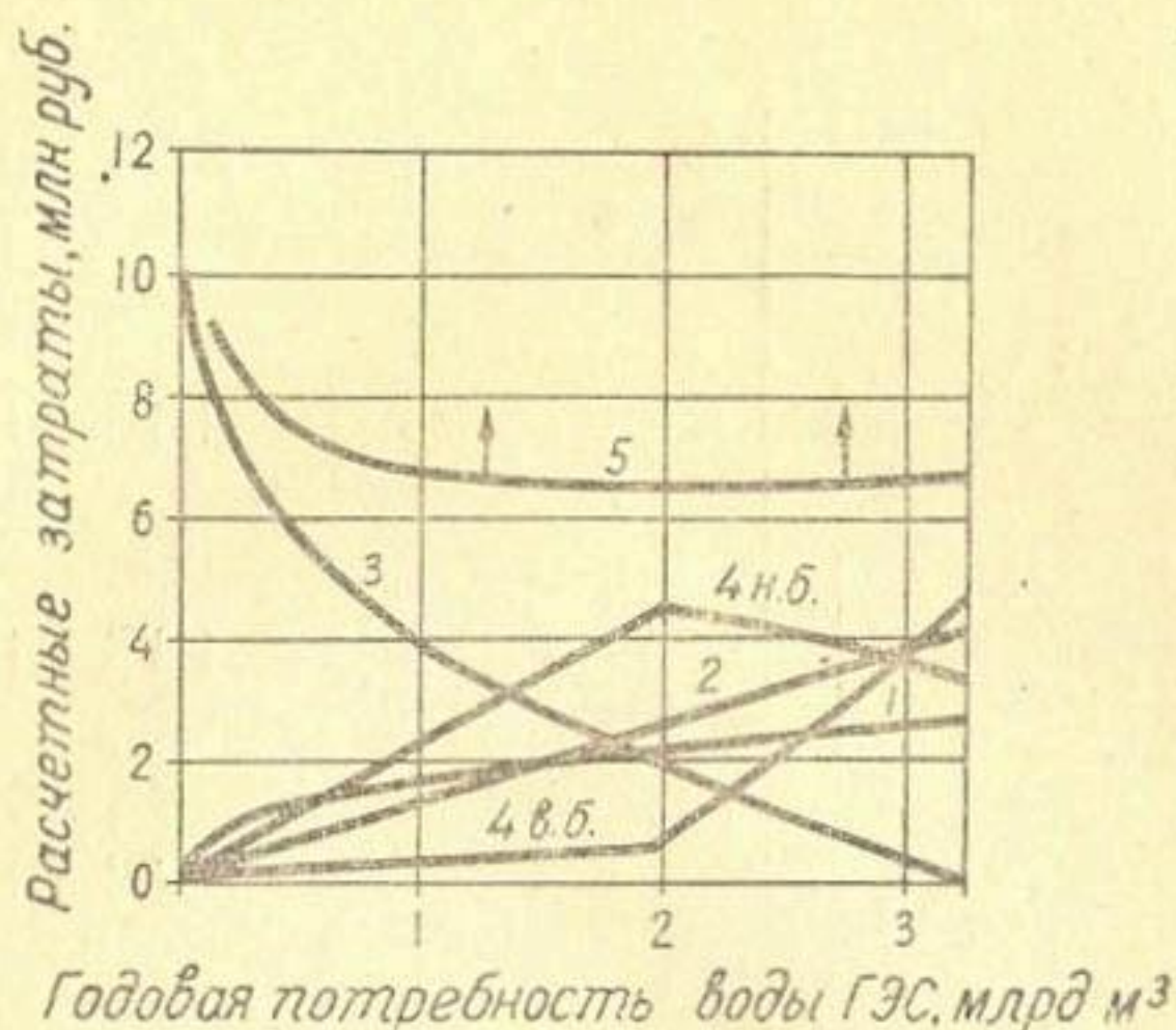
Рис. 40. Среднегодовые расчетные затраты в ГЭС 1, сэкономленное топливо 2, заменяющую КЭС 3, дополнительные затраты в сельское хозяйство (4 н. б. — от снижения площади орошения в нижнем и 4 в. б. — верхнем бьефе ГЭС) и их сумма 5 в зависимости от годовой потребности воды ГЭС для покрытия заданного графика нагрузки (схема III).
