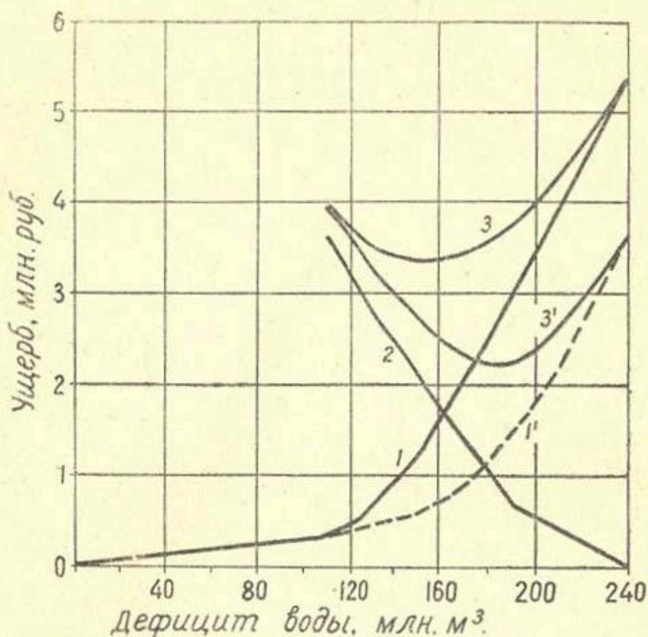
Рис. 61. Зависимости ущерба от ограничений в воде: 1—производственно-энергетической системы (без ограничения коммунально-бытовой нагрузки системы); 1'—то же с учетом ограничения коммунально-бытовой нагрузки; 2—сельскохозяйственных потребителей; 3—суммарные государственные ущербы от ограничений в воде без учета ограничений коммунально-бытовой нагрузки энергосистемы; 3' — то же с учетом этих ограничений.
