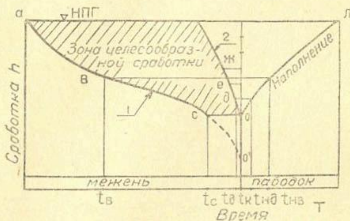
Рис. 24. К выбору оптимального режима сработки водохранилища.
