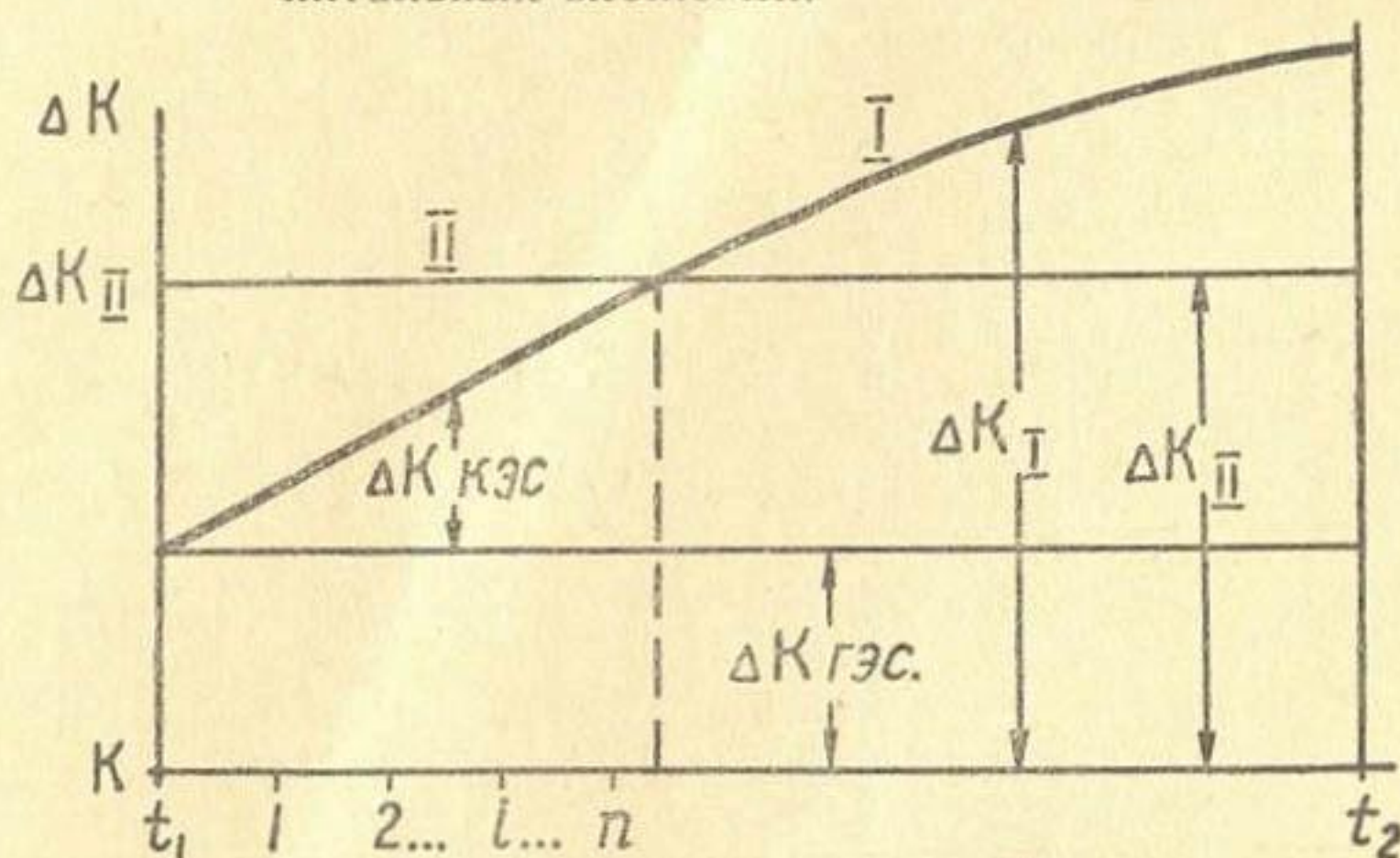
Рис. 5. Динамика изменения капитальных вложений по вариантам: I — на ГЭС к первому расчетному уровню t_1 устанавливается полная мощность N_r с последующей компенсацией ее снижения, наращиванием тепловой мощности; II — на уровне t_1 устанавливается мощность ГЭС, равная N_r , и дополнительная мощность ТЭС — \alpha_N \Delta N_r
