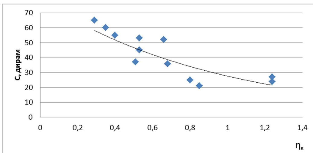
Рис. 2. - Зависимость удельных эксплуатационных затрат от показателя \eta_k
