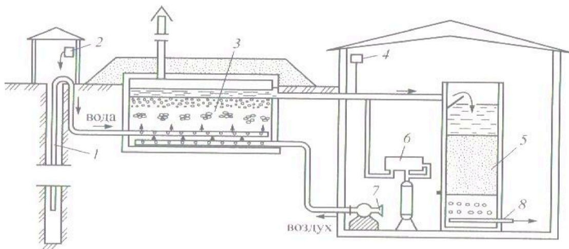
Рис. 5. - Установка биохимического извлечения сероводорода из воды:
