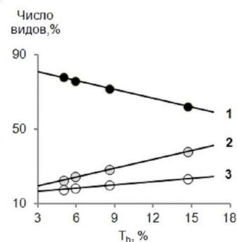
Рис. 5. Линейные тренды по данным 1947–1981 гг.: 1 – H ; 2 – ( T + T h ); 3 – T
