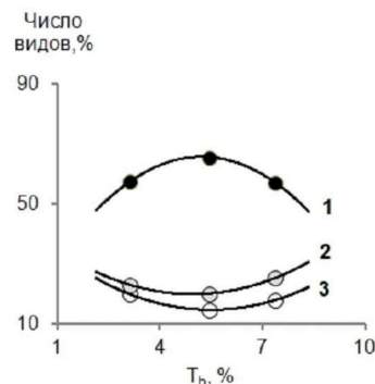
Рис. 6. Полиномиальные тренды по данным 1990–2000 гг.: 1 – H ; 2 – ( T + T h ); 3 – T
